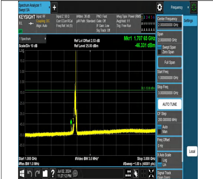
Band66-20MHz-QPSK-132572-1RB#99-1000~3000-PASS
