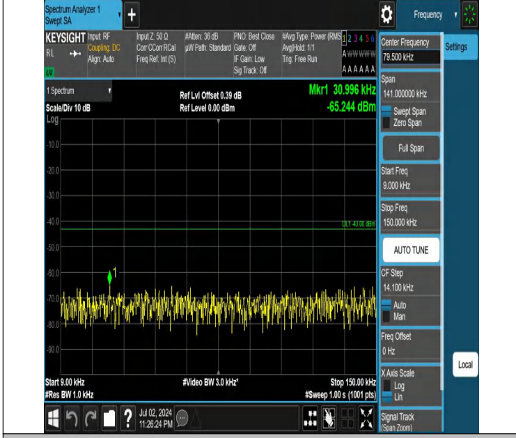
Band66-20MHz-QPSK-132572-1RB#0-0.009~0.15-PASS
