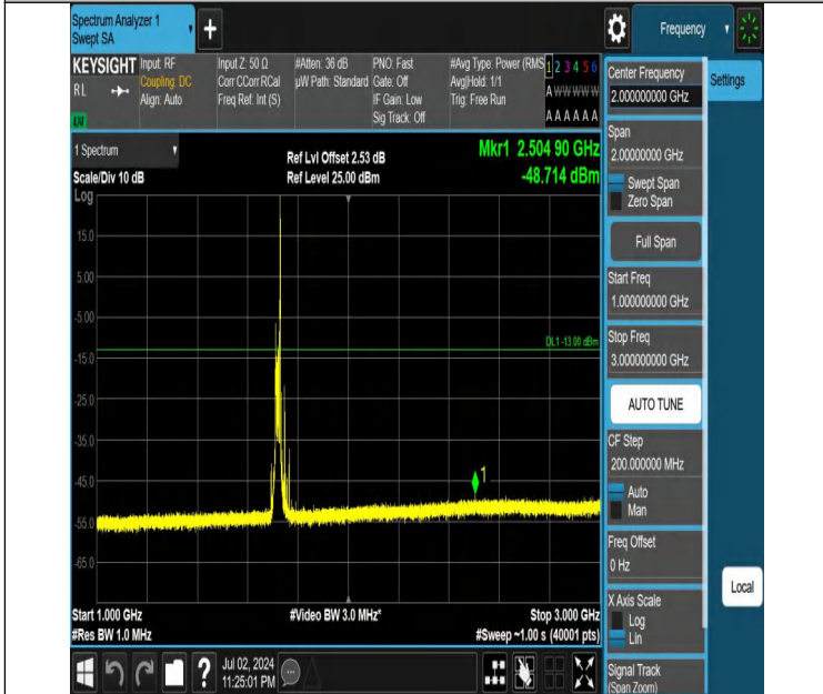
Band66-20MHz-QPSK-132072-1RB#99-1000~3000-PASS
