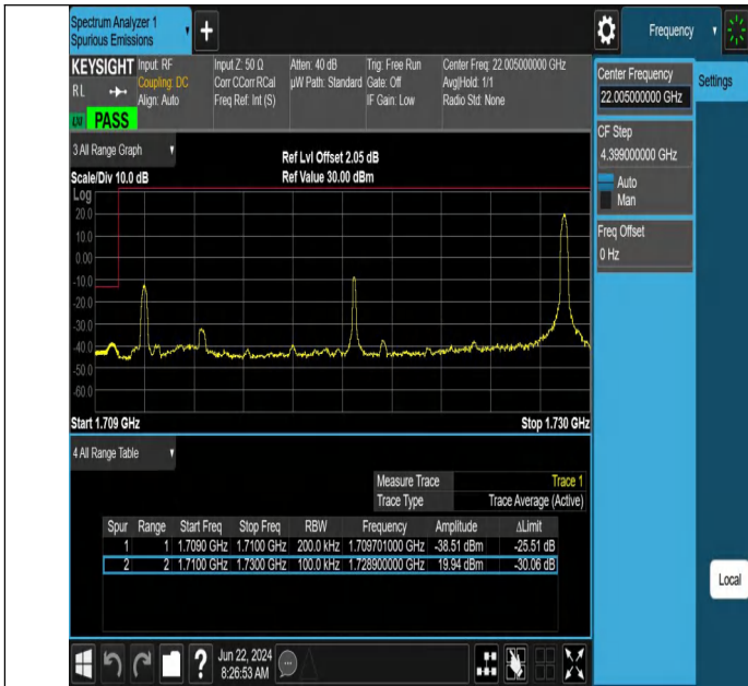
Band66-20MHz-QPSK-132072-1RB#99-PASS
