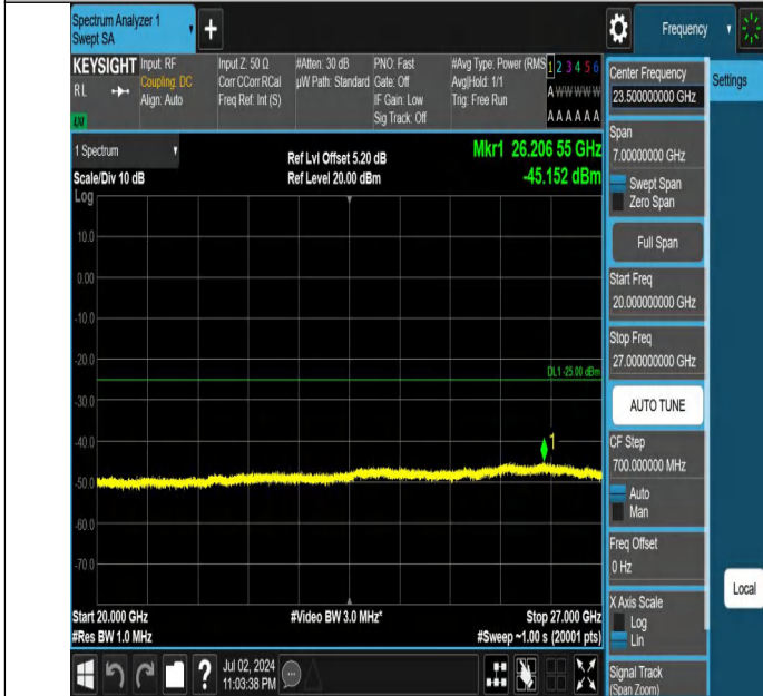
Band7-20MHz-QPSK-20850-1RB#0-20000~27000-PASS
