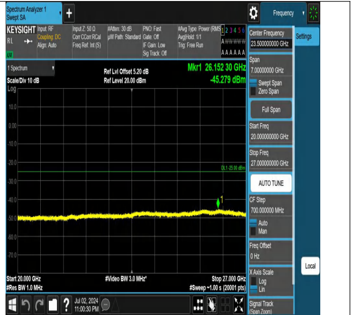
Band7-15MHz-QPSK-20825-1RB#74-20000~27000-PASS
