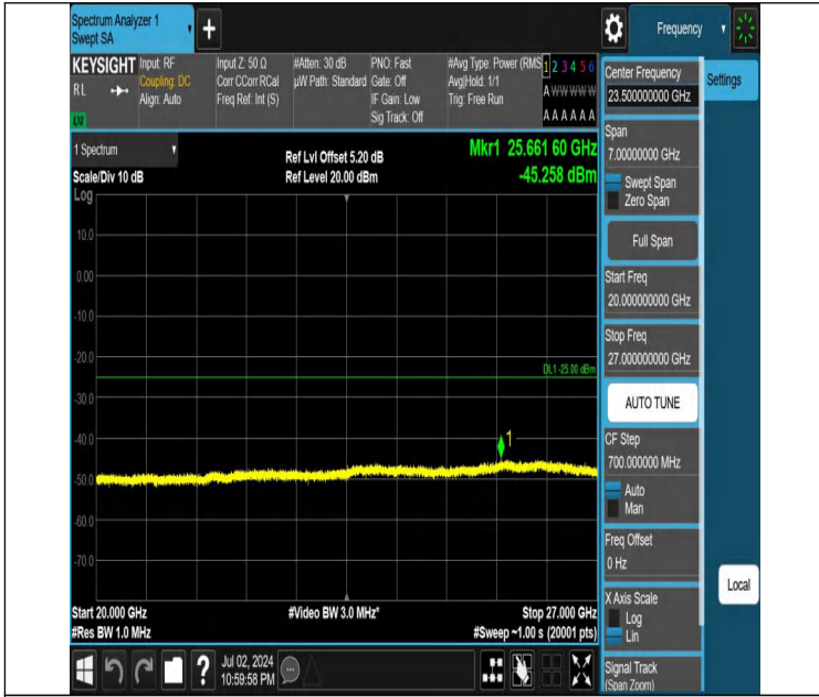
Band7-15MHz-QPSK-20825-1RB#0-20000~27000-PASS
