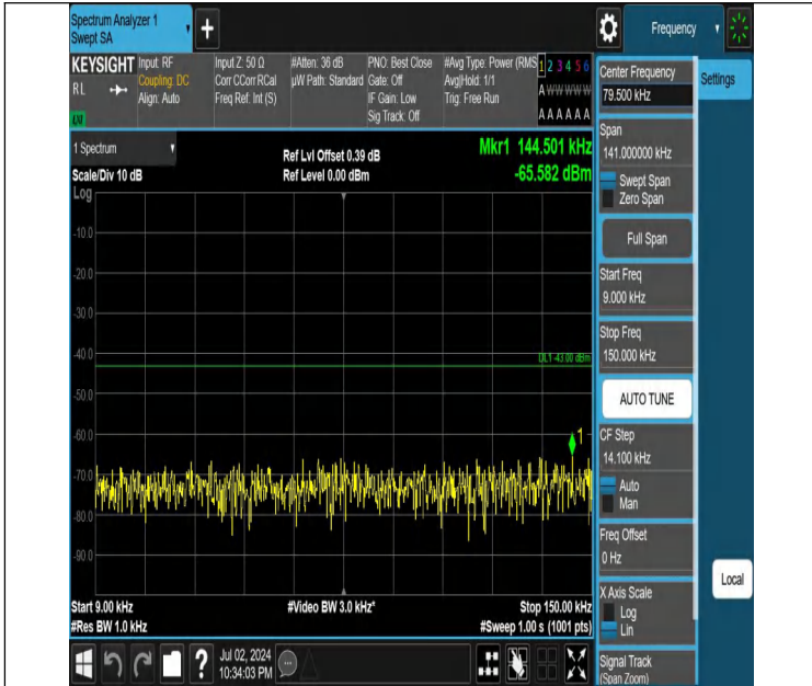
Band4-20MHz-QPSK-20175-1RB#0-0.009~0.15-PASS
