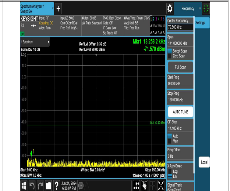
GPRS1900-661-0-0.009~0.15MHz-PASS
