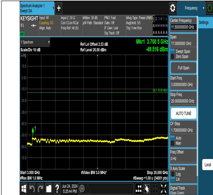
GSM1900-512-0-3000~20000MHz-PASS
