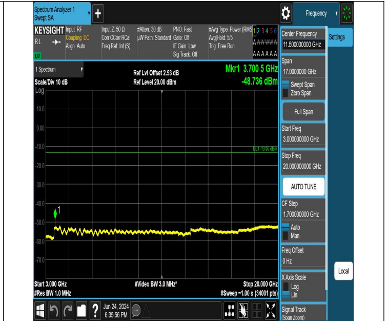
GPRS1900-512-0-3000~20000MHz-PASS
