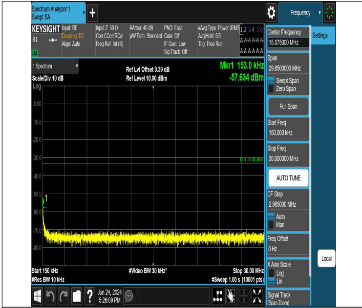
GSM1900-661-0-0.15~30MHz-PASS
