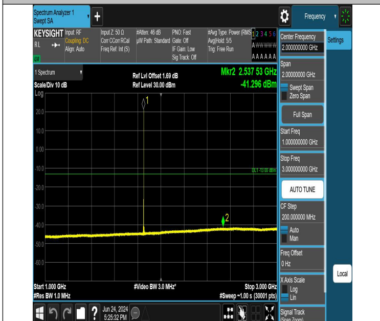
GSM1900-512-0-1000~3000MHz-PASS
