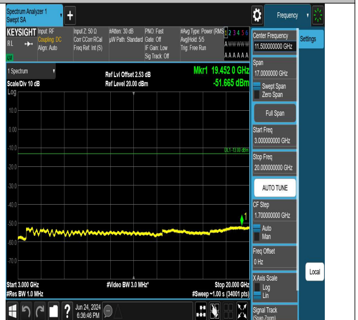
GPRS1900-661-0-3000~20000MHz-PASS
