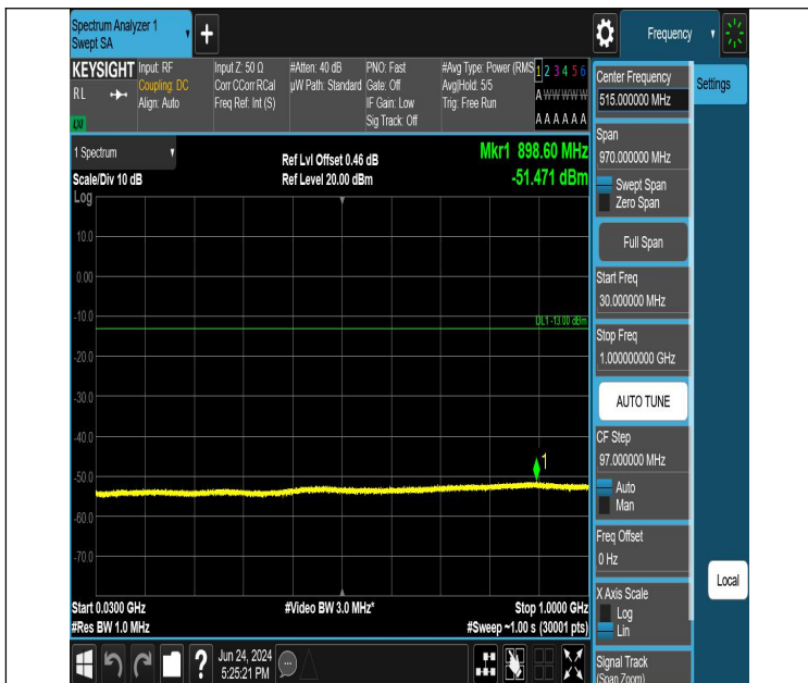
GSM1900-512-0-30~1000MHz-PASS
