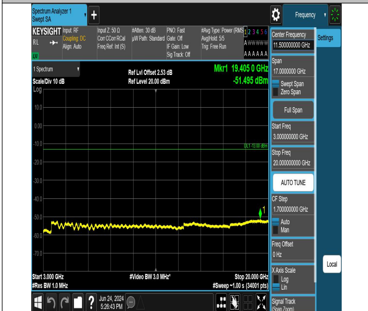
GSM1900-661-0-3000~20000MHz-PASS
