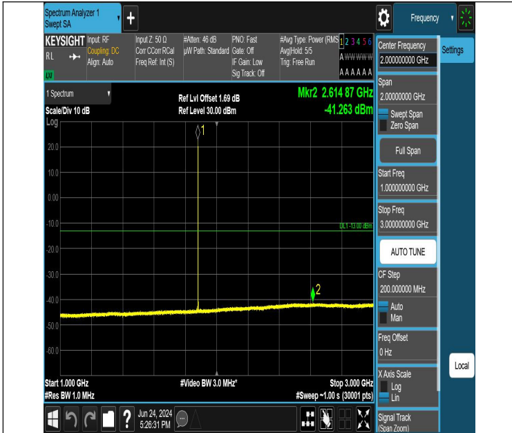
GSM1900-661-0-1000~3000MHz-PASS
