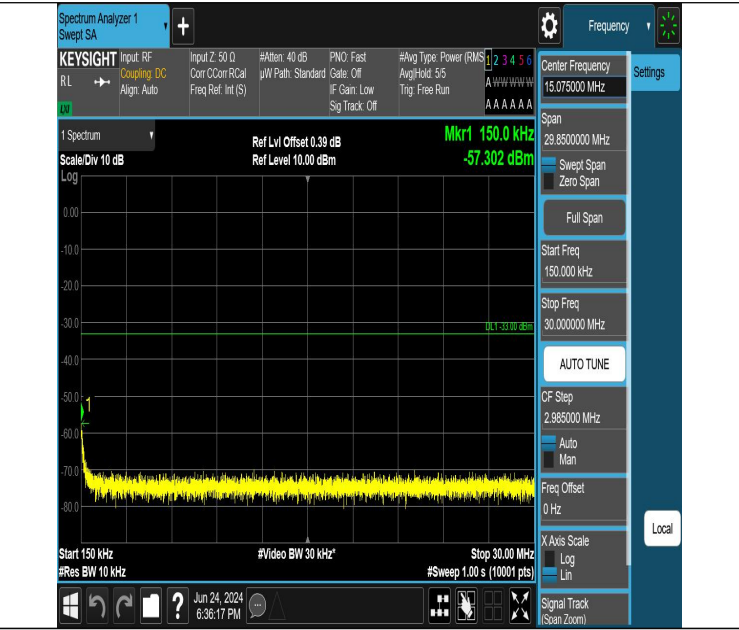
GPRS1900-661-0-0.15~30MHz-PASS
