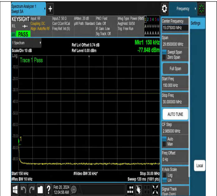
NTNV-N78-3700-3800-PC2-30-10-L-DFT-QPSK-Edge_1RB_L eft-Ant1-PASS
