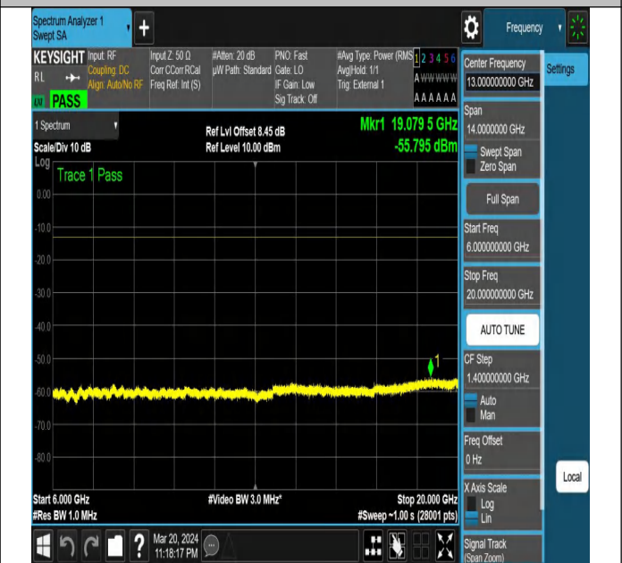
NTNV-N78-3450-3550-PC2-30-40-L-DFT-QPSK-Edge_1RB_L eft-Ant1-PASS
