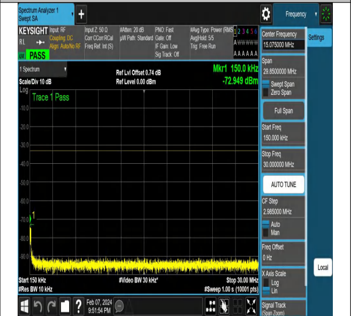
NTNV-N78-3450-3550-PC2-30-40-L-DFT-QPSK-Edge_1RB_L eft-Ant1-PASS
