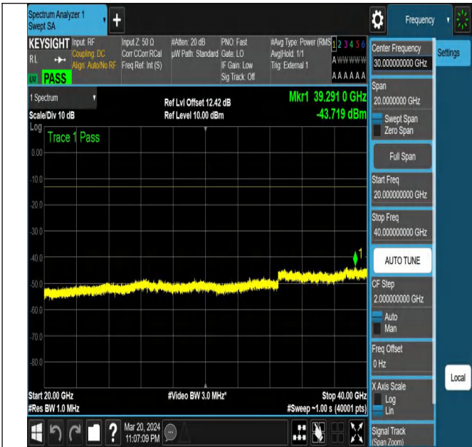
NTNV-N78-3450-3550-PC2-30-20-M-DFT-QPSK-Edge_1RB_
