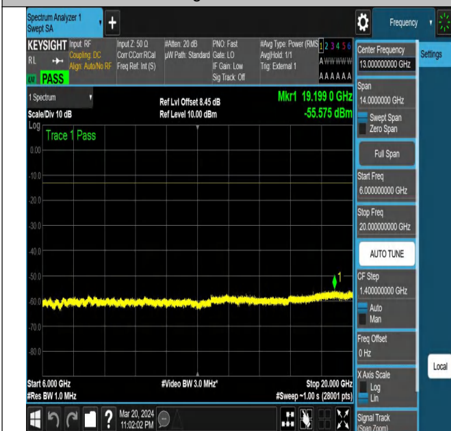
NTNV-N78-3450-3550-PC2-30-20-L-DFT-QPSK-Edge_1RB_
