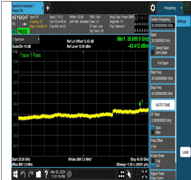
NTNV-N78-3450-3550-PC2-30-20-L-DFT-QPSK-Edge_1RB_ eft-Ant1-PASS
