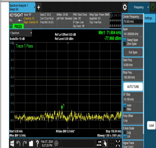
NTNV-N78-3450-3550-PC2-30-20-L-DFT-QPSK-Edge_1RB_L eft-Ant1-PASS
