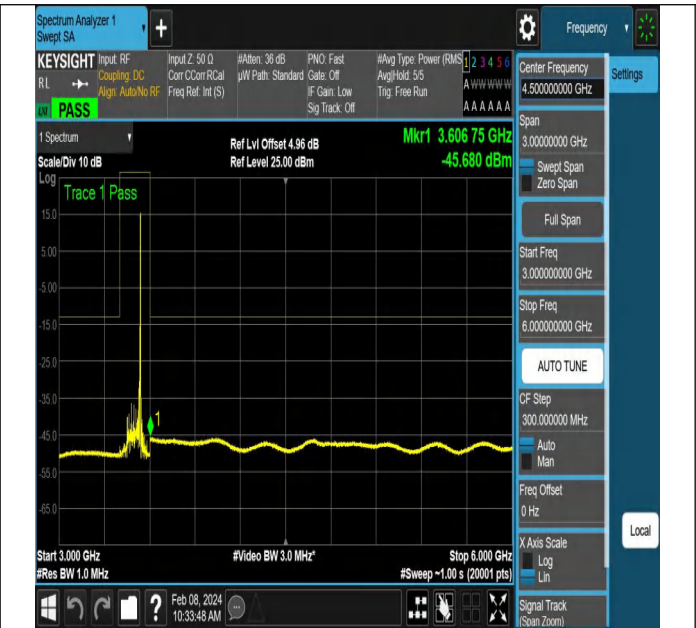
NTNV-N78-3450-3550-PC2-30-90-L-DFT-QPSK-Edge_1RB_
