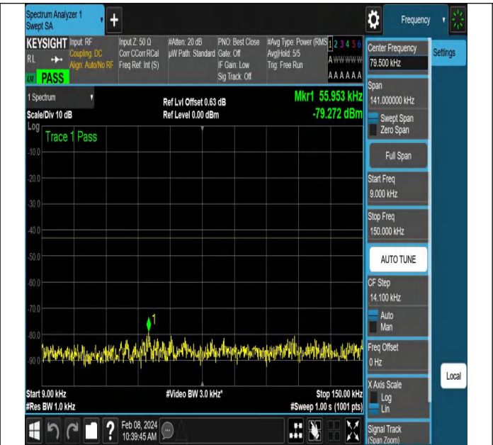
NTNV-N78-3450-3550-PC2-30-90-M-DFT-QPSK-Edge_1RB_
