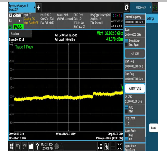
NTNV-N78-3450-3550-PC2-30-90-L-DFT-QPSK-Edge_1RB_
