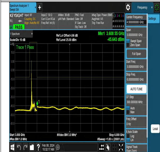
NTNV-N78-3450-3550-PC2-30-90-L-DFT-QPSK-Edge_1RB_L eft-Ant1-PASS
