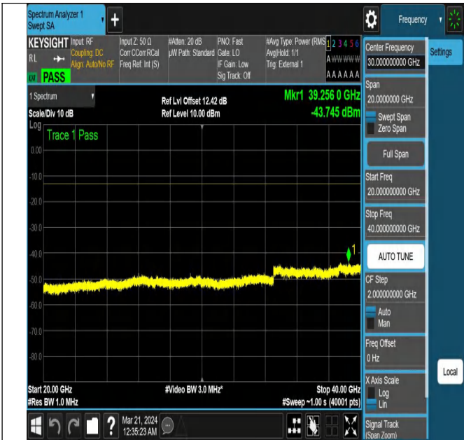
NTNV-N78-3450-3550-PC2-30-90-M-DFT-QPSK-Edge_1RB_
