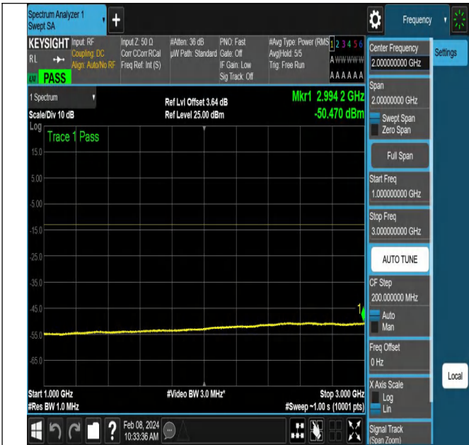
NTNV-N78-3450-3550-PC2-30-90-L-DFT-QPSK-Edge_1RB_
