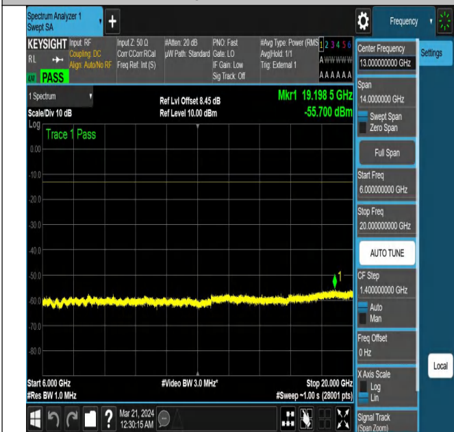
NTNV-N78-3450-3550-PC2-30-90-L-DFT-QPSK-Edge_1RB_
