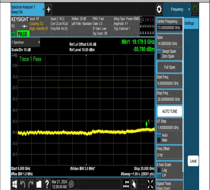
NTNV-N78-3450-3550-PC2-30-90-L-DFT-QPSK-Edge_1RB_L eft-Ant1-PASS
