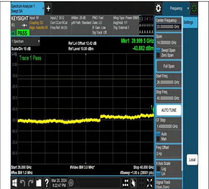
NTNV-N77-3700-3980-PC2-30-20-L-DFT-QPSK-Edge_1RB_L eft-Ant1-PASS
