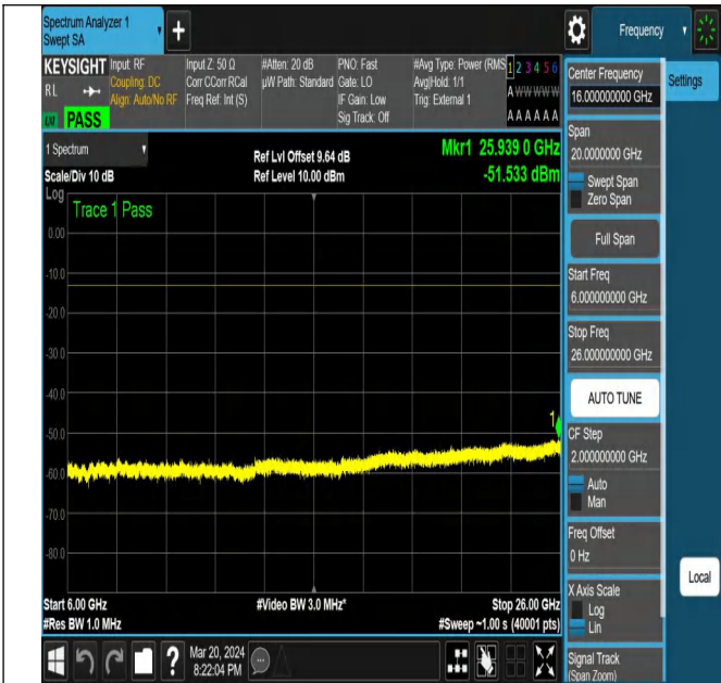
NTNV-N77-3700-3980-PC2-30-20-L-DFT-QPSK-Edge_1RB_L eft-Ant1-PASS
