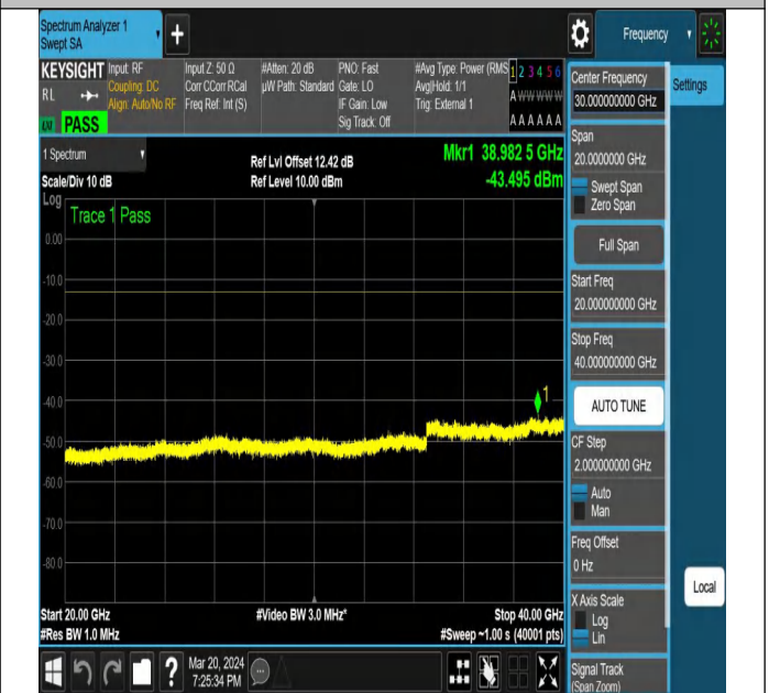
NTNV-N77-3450-3550-PC2-30-90-L-DFT-QPSK-Edge_1RB_L eft-Ant1-PASS
