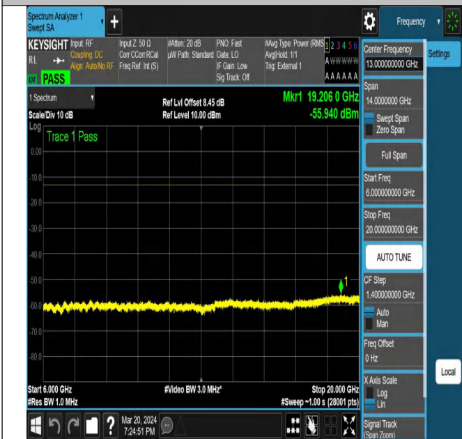
NTNV-N77-3450-3550-PC2-30-90-L-DFT-QPSK-Edge_1RB_L eft-Ant1-PASS
