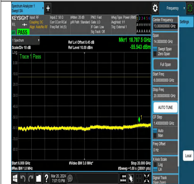
NTNV-N77-3450-3550-PC2-30-60-L-DFT-QPSK-Edge_1RB_L eft-Ant1-PASS
