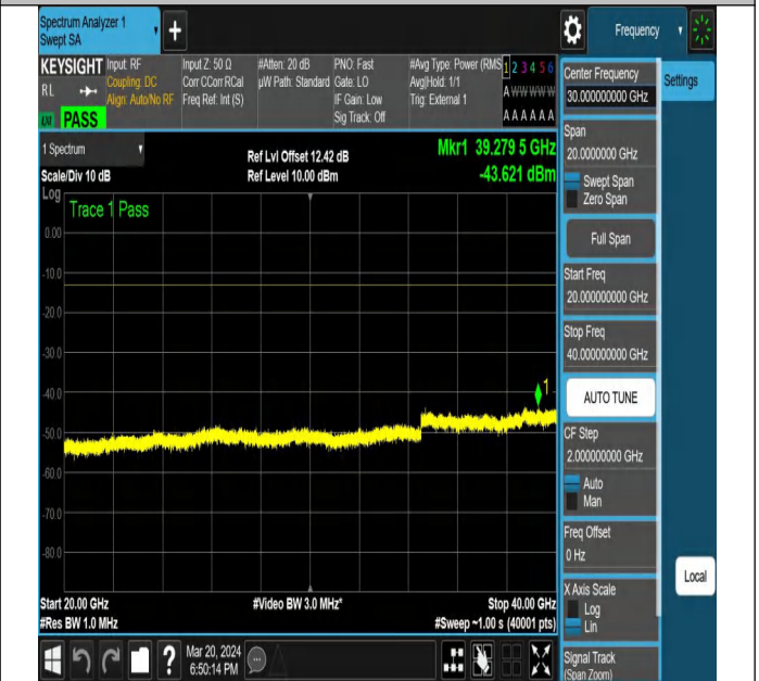
NTNV-N77-3450-3550-PC2-30-80-L-DFT-QPSK-Edge_1RB_L eft-Ant1-PASS
