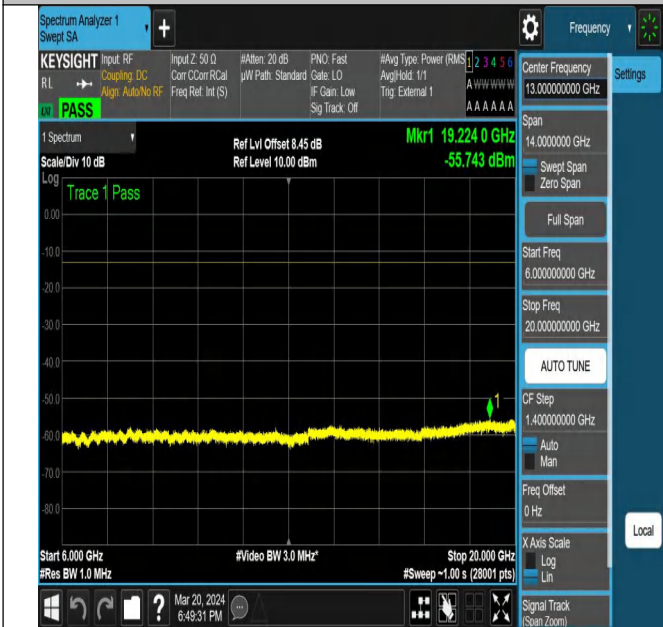
NTNV-N77-3450-3550-PC2-30-80-L-DFT-QPSK-Edge_1RB_L eft-Ant1-PASS
