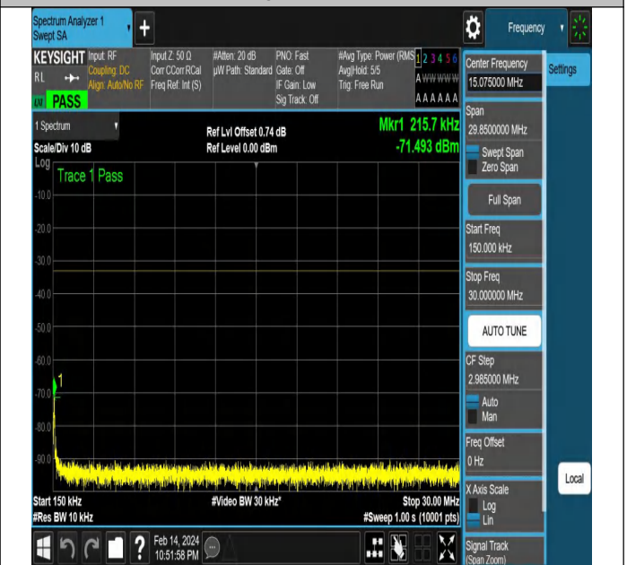
NTNV-N77-3450-3550-PC2-30-40-L-DFT-QPSK-Edge_1RB_L eft-Ant1-PASS
