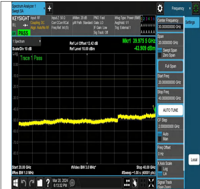
NTNV-N77-3450-3550-PC2-30-40-L-DFT-QPSK-Edge_1RB_L eft-Ant1-PASS
