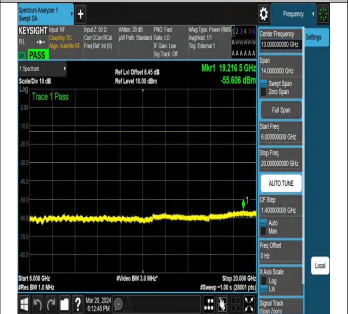
NTNV-N77-3450-3550-PC2-30-40-L-DFT-QPSK-Edge_1RB_L eft-Ant1-PASS
