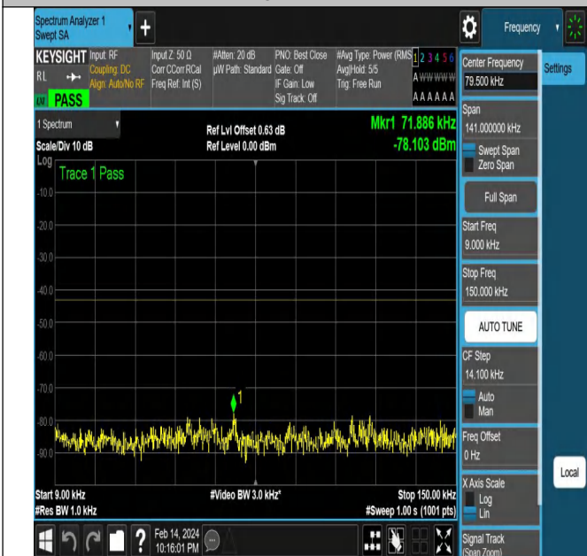
NTNV-N77-3450-3550-PC2-30-20-L-DFT-QPSK-Edge_1RB_L eft-Ant1-PASS
