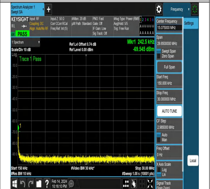
NTNV-N77-3450-3550-PC2-30-20-L-DFT-QPSK-Edge_1RB_L eft-Ant1-PASS
