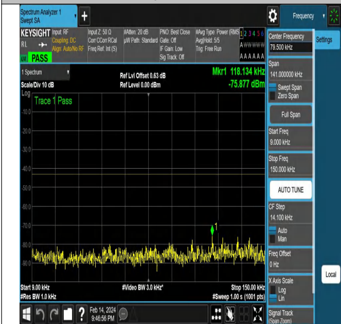
NTNV-N77-3450-3550-PC2-30-15-L-DFT-QPSK-Edge_1RB_L eft-Ant1-PASS
