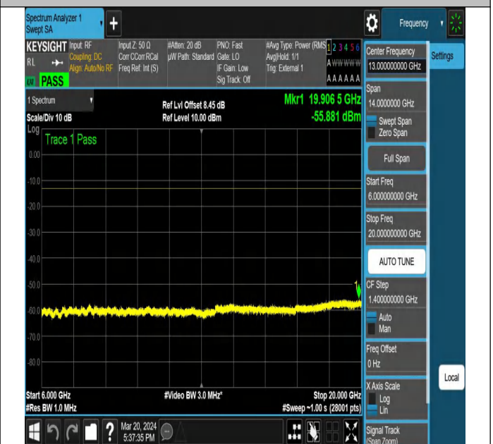
NTNV-N77-3450-3550-PC2-30-15-L-DFT-QPSK-Edge_1RB_L eft-Ant1-PASS
