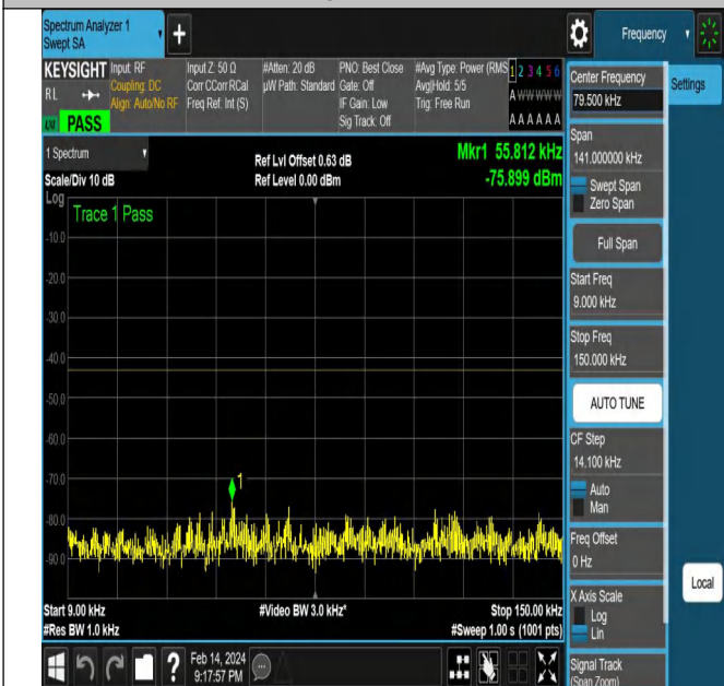
NTNV-N77-3450-3550-PC2-30-10-L-DFT-QPSK-Edge_1RB_L eft-Ant1-PASS
