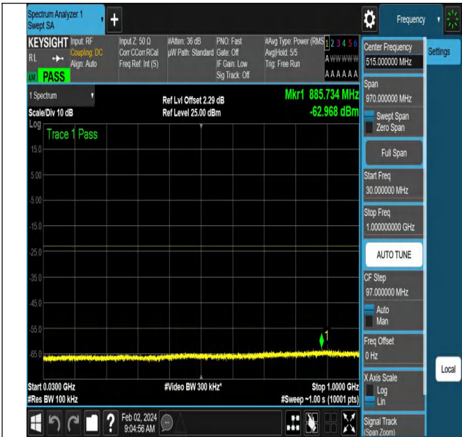
NTNV-N66-PC3-15-20-M-DFT-QPSK-Edge_1RB_Right-Ant1-
