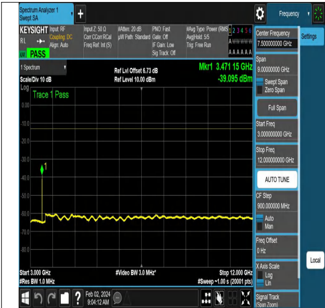
NTNV-N66-PC3-15-20-M-DFT-QPSK-Edge_1RB_Left-Ant1-P
