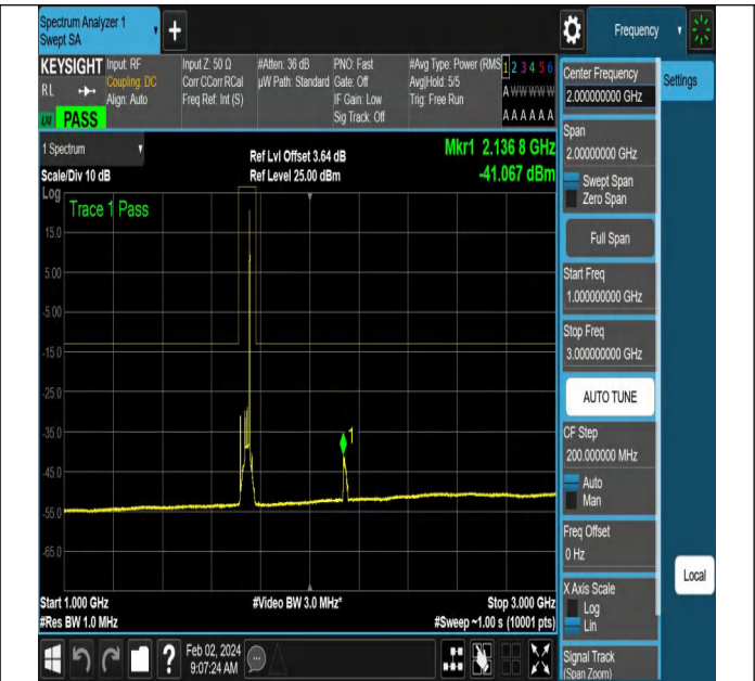
NTNV-N66-PC3-15-20-M-CP-QPSK-Edge_1RB_Right-Ant1-P ASS
