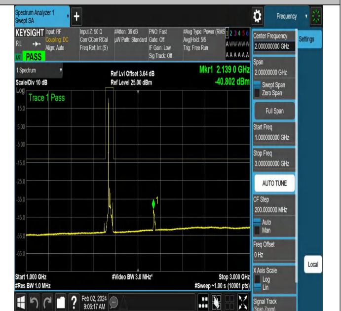
NTNV-N66-PC3-15-20-M-CP-QPSK-Edge_1RB_Left-Ant1-PA
