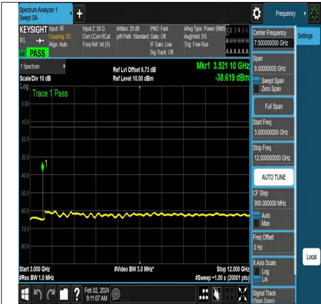
NTNV-N66-PC3-15-20-H-DFT-QPSK-Edge_1RB_Left-Ant1-P ASS
