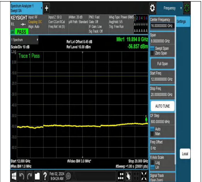
NTNV-N66-PC3-15-20-M-DFT-QPSK-Edge_1RB_Left-Ant1-P
