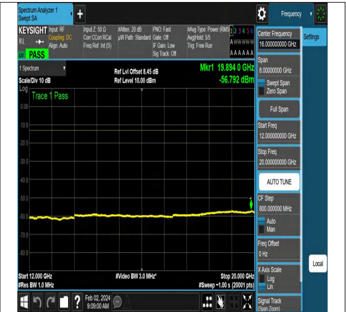
NTNV-N66-PC3-15-20-H-DFT-PI2BPSK-Edge_1RB_Left-Ant1 -PASS
