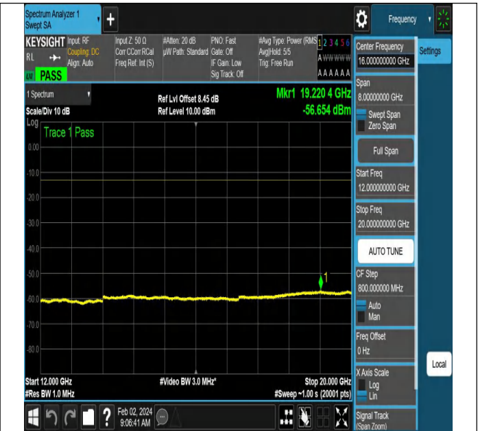
NTNV-N66-PC3-15-20-M-CP-QPSK-Edge_1RB_Left-Ant1-PA
