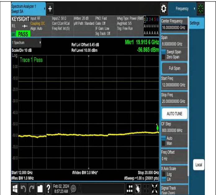
NTNV-N66-PC3-15-20-L-DFT-QPSK-Edge_1RB_Left-Ant1-PA
