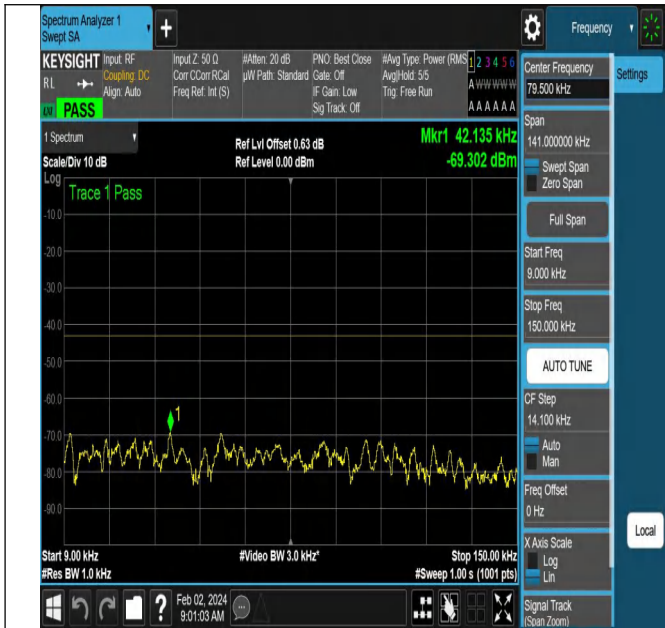
NTNV-N66-PC3-15-20-M-DFT-PI2BPSK-Edge_1RB_Left-Ant1
