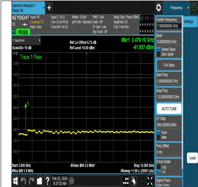
NTNV-N66-PC3-15-15-M-DFT-PI2BPSK-Edge_1RB_Left-Ant1 -PASS
