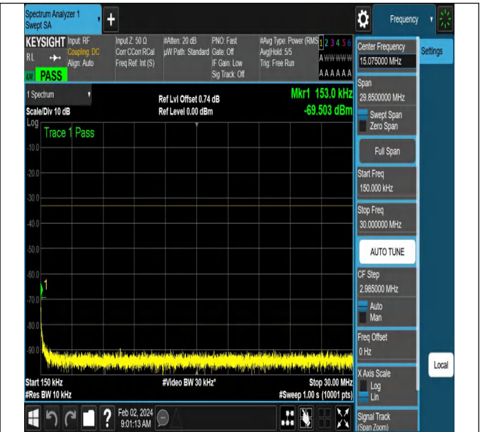
NTNV-N66-PC3-15-20-M-DFT-PI2BPSK-Edge_1RB_Left-Ant1
