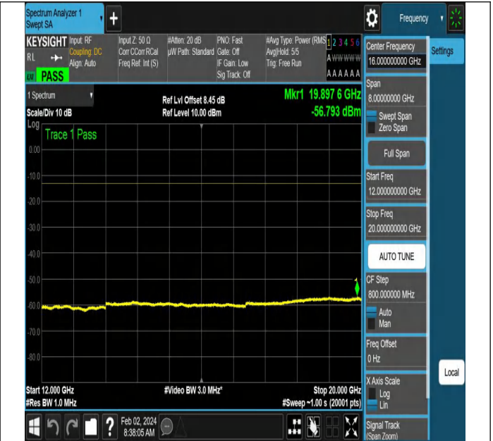
NTNV-N66-PC3-15-15-M-DFT-PI2BPSK-Edge_1RB_Left-Ant1 -PASS
