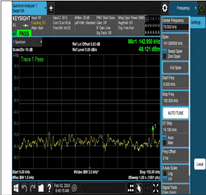
NTNV-N66-PC3-15-15-M-DFT-QPSK-Edge_1RB_Left-Ant1-P ASS
