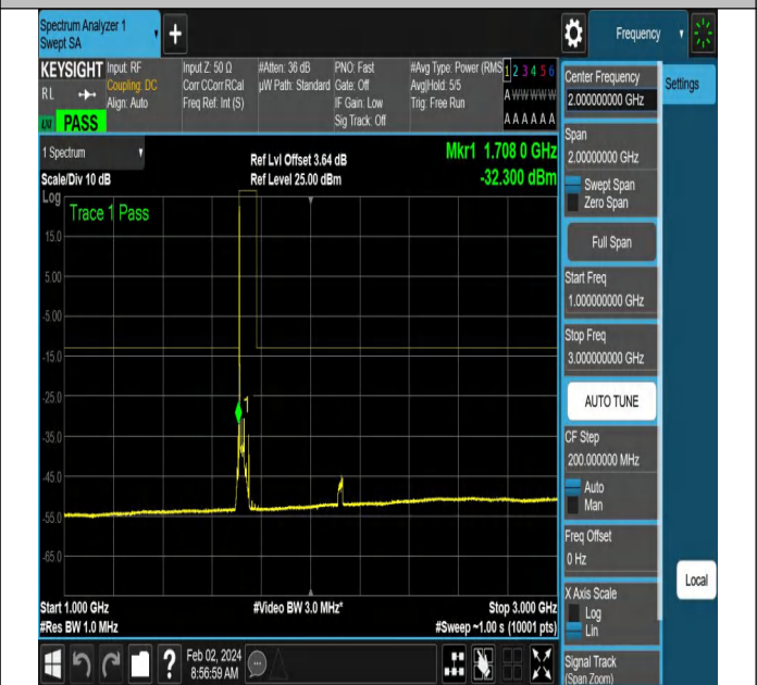
NTNV-N66-PC3-15-20-L-DFT-QPSK-Edge_1RB_Left-Ant1-PA
