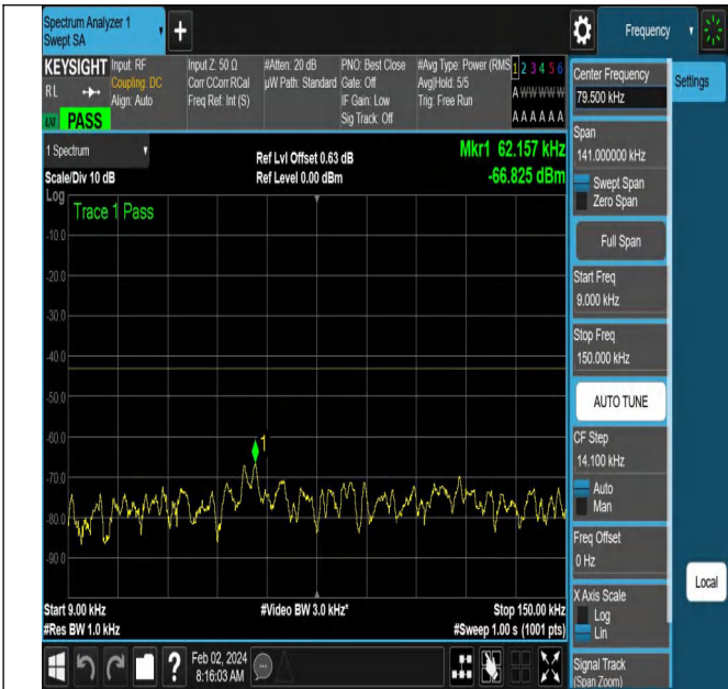
NTNV-N66-PC3-15-10-M-DFT-QPSK-Edge_1RB_Left-Ant1-P ASS
