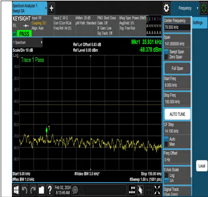
NTNV-N66-PC3-15-10-M-DFT-PI2BPSK-Edge_1RB_Left-Ant1
