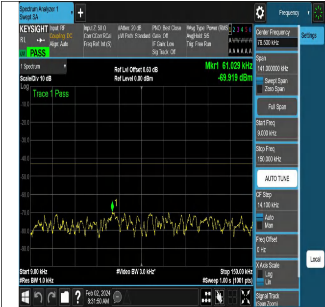
NTNV-N66-PC3-15-15-L-DFT-QPSK-Edge_1RB_Left-Ant1-PA
