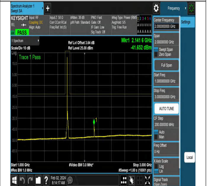
NTNV-N66-PC3-15-10-M-DFT-PI2BPSK-Edge_1RB_Left-Ant1
