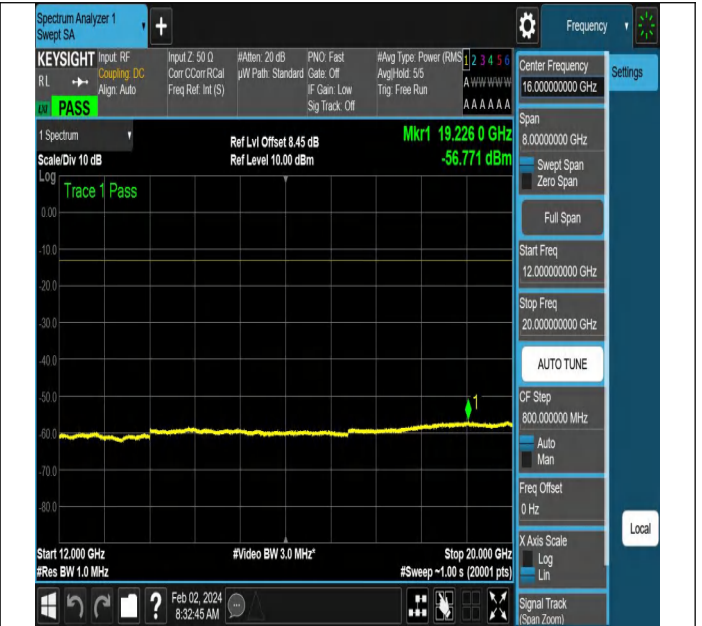
NTNV-N66-PC3-15-15-L-DFT-QPSK-Edge_1RB_Left-Ant1-PA
