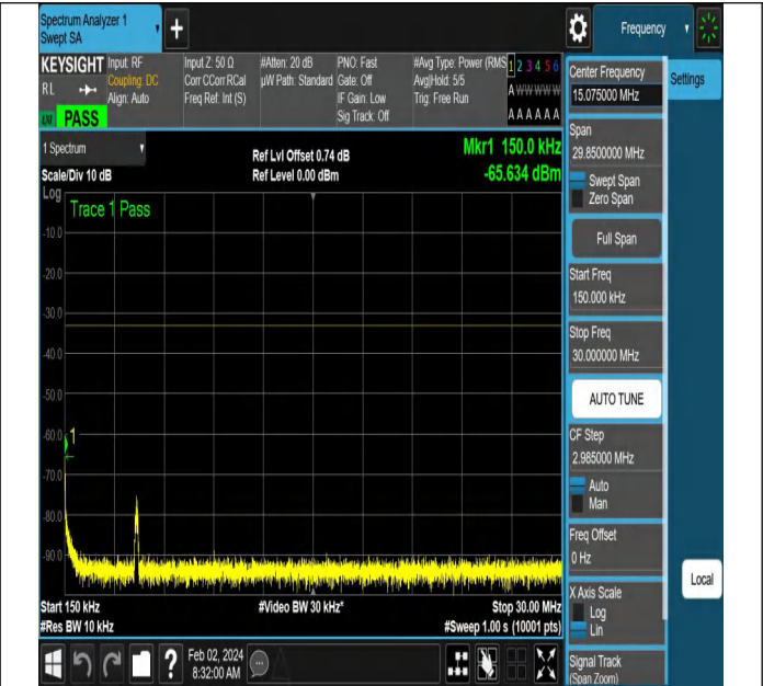
NTNV-N66-PC3-15-15-L-DFT-QPSK-Edge_1RB_Left-Ant1-PA
