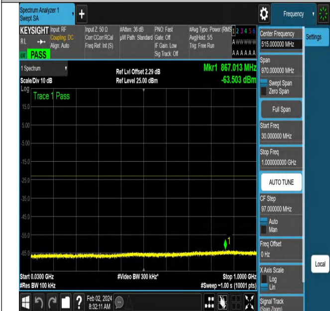
NTNV-N66-PC3-15-15-L-DFT-QPSK-Edge_1RB_Left-Ant1-PA
