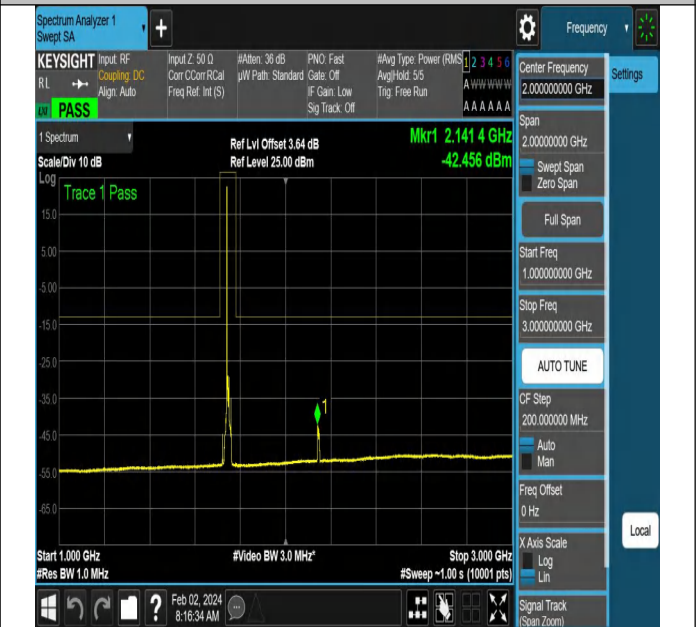
NTNV-N66-PC3-15-10-M-DFT-QPSK-Edge_1RB_Left-Ant1-P ASS
