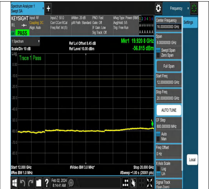
NTNV-N66-PC3-15-10-M-DFT-PI2BPSK-Edge_1RB_Left-Ant1 -PASS
