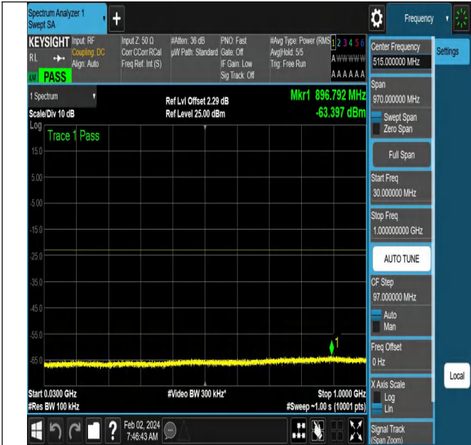
NTNV-N66-PC3-15-5-L-DFT-PI2BPSK-Edge_1RB_Right-Ant1 -PASS
