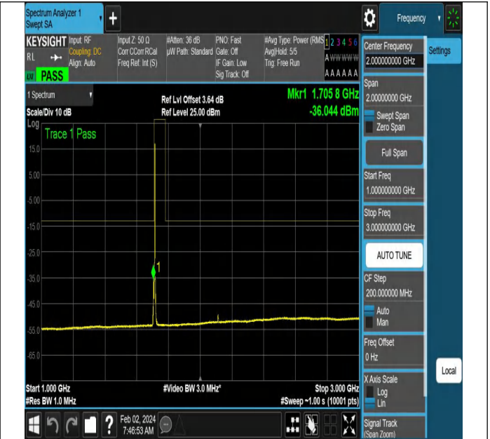
NTNV-N66-PC3-15-5-L-DFT-PI2BPSK-Edge_1RB_Right-Ant1 -PASS
