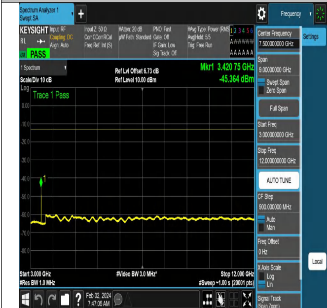
NTNV-N66-PC3-15-5-L-DFT-PI2BPSK-Edge_1RB_Right-Ant1 -PASS
