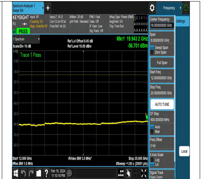
NTNV-N12-PC3-15-10-M-DFT-PI2BPSK-Edge_1RB_Left-Ant1 -PASS
