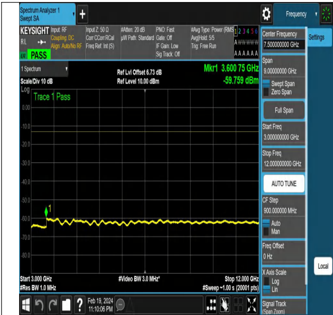
NTNV-N12-PC3-15-10-M-DFT-PI2BPSK-Edge_1RB_Left-Ant1 -PASS
