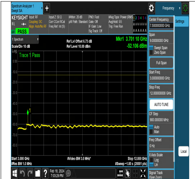
NTNV-DC_5A_n2A-PC3-15-5+10-M+L-QPSK-DFT-QPSK-Edge
