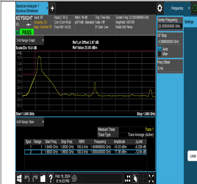
NTNV-DC_5A_n2A-PC3-15-5+10-M+L-QPSK-DFT-QPSK-Edge_ 1RB_Left-PASS
