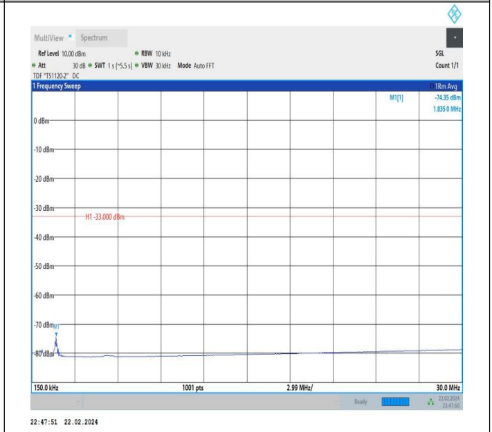
66-66-20MHz-20MHz-QPSK-QPSK-132072-132270-1RB#99-0 RB#0-0.15~30MHz-PASS
