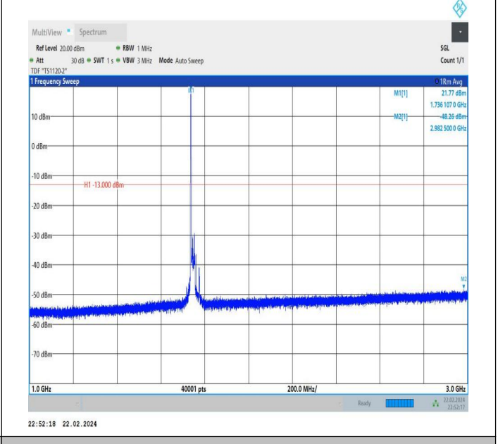
66-66-20MHz-20MHz-QPSK-QPSK-132323-132521-1RB#0-0 RB#0-1000~3000MHz-PASS
