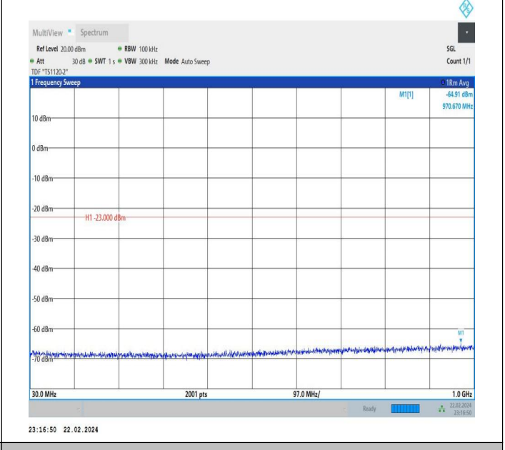
66-66-20MHz-20MHz-QPSK-QPSK-132374-132572-1RB#0-1 RB#99-30~1000MHz-PASS
