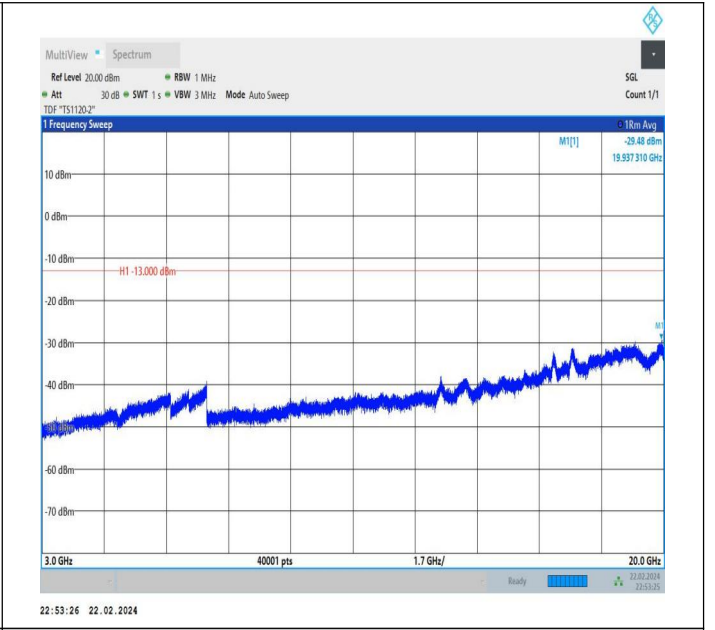
66-66-20MHz-20MHz-QPSK-QPSK-132323-132521-1RB#99-0 RB#0-3000~20000MHz-PASS
