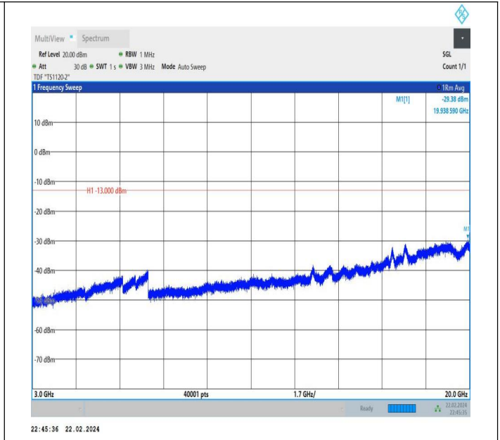
66-66-20MHz-20MHz-QPSK-QPSK-132072-132270-1RB#0-0 RB#0-3000~20000MHz-PASS
