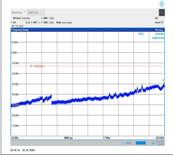
66-66-20MHz-20MHz-QPSK-QPSK-132323-132521-1RB#0-1 RB#99-3000~20000MHz-PASS
