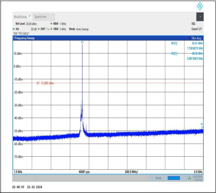
66-66-20MHz-20MHz-QPSK-QPSK-132072-132270-1RB#99-0 RB#0-1000~3000MHz-PASS
