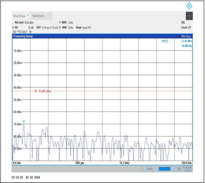
66-66-20MHz-20MHz-QPSK-QPSK-132374-132572-1RB#0-1 RB#99-0.009~0.15MHz-PASS
