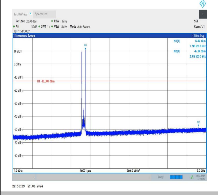
66-66-20MHz-20MHz-QPSK-QPSK-132072-132270-1RB#0-1 RB#99-1000~3000MHz-PASS
