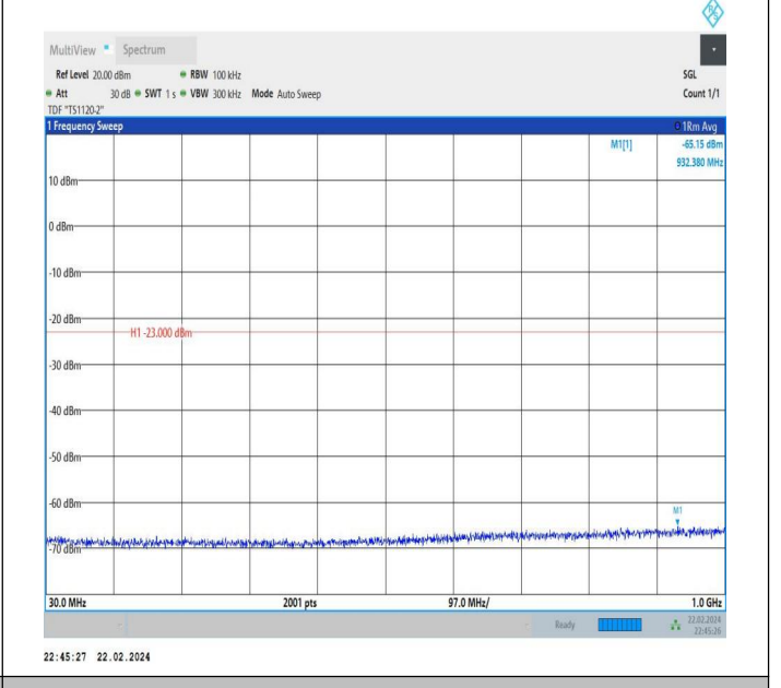
66-66-20MHz-20MHz-QPSK-QPSK-132072-132270-1RB#0-0 RB#0-30~1000MHz-PASS
