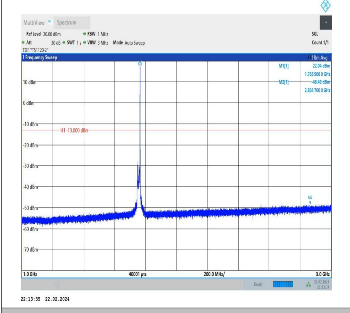
66-66-20MHz-15MHz-QPSK-QPSK-132423-132594-1RB#99-0 RB#0-1000~3000MHz-PASS
