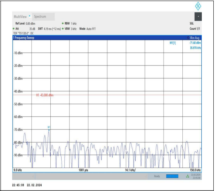
66-66-20MHz-20MHz-QPSK-QPSK-132072-132270-1RB#0-0 RB#0-0.009~0.15MHz-PASS
