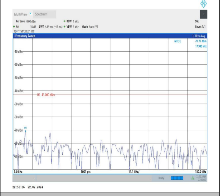
66-66-20MHz-20MHz-QPSK-QPSK-132072-132270-1RB#0-1 RB#99-0.009~0.15MHz-PASS
