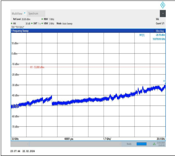
66-66-20MHz-20MHz-QPSK-QPSK-132374-132572-1RB#99-0 RB#0-3000~20000MHz-PASS
