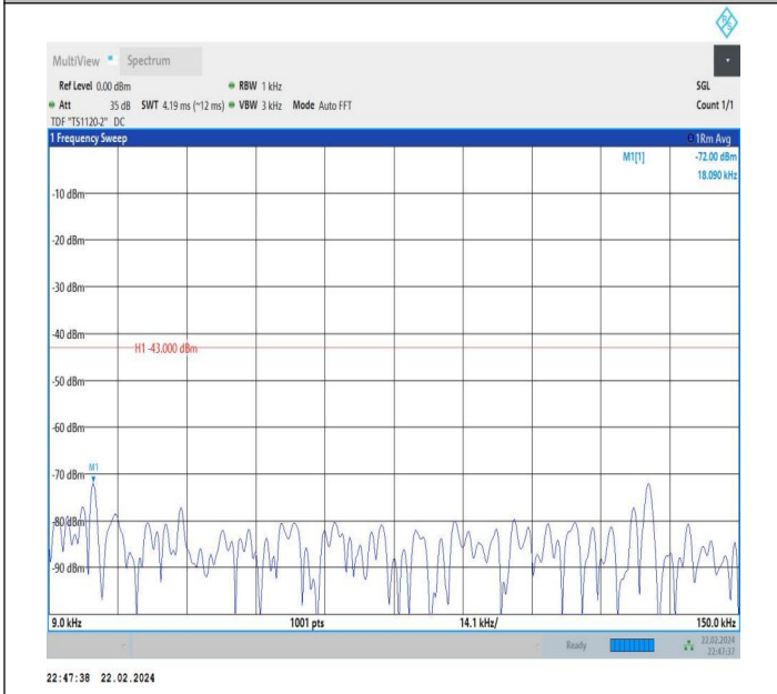
66-66-20MHz-20MHz-QPSK-QPSK-132072-132270-1RB#99-0 RB#0-0.009~0.15MHz-PASS
