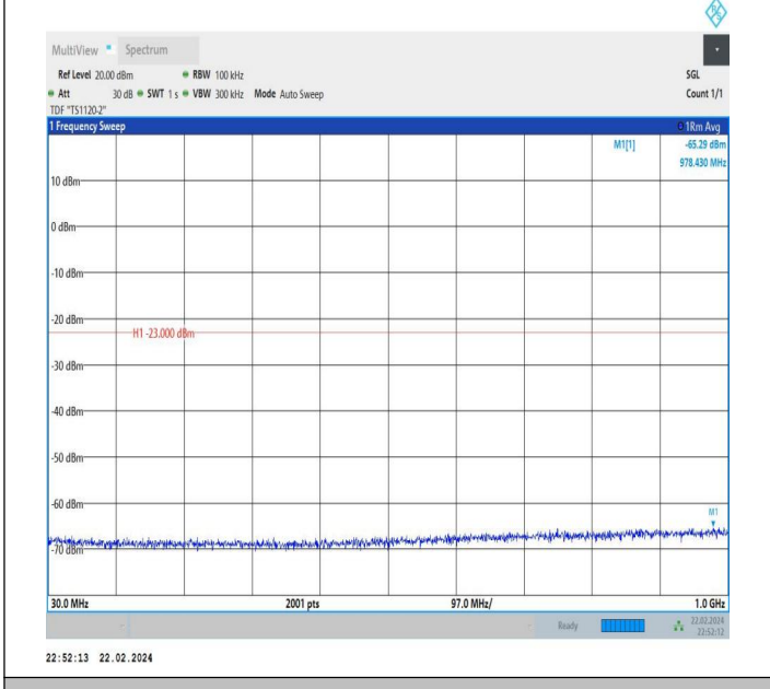
66-66-20MHz-20MHz-QPSK-QPSK-132323-132521-1RB#0-0 RB#0-30~1000MHz-PASS
