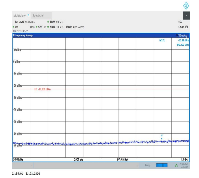
66-66-20MHz-20MHz-QPSK-QPSK-132323-132521-1RB#0-1 RB#99-30~1000MHz-PASS
