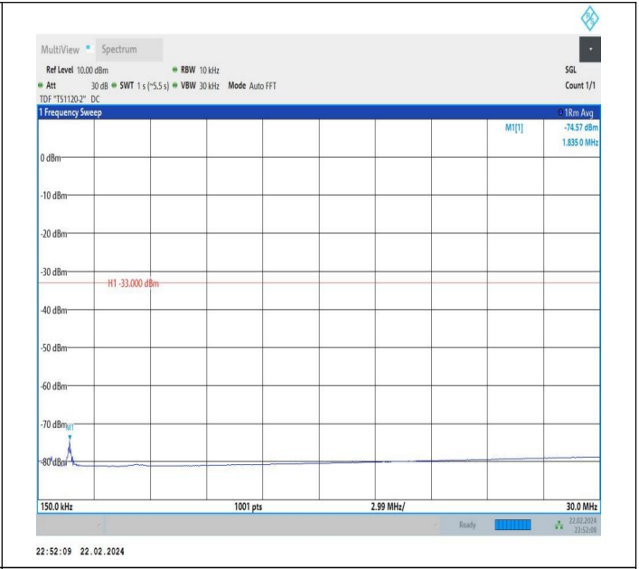
66-66-20MHz-20MHz-QPSK-QPSK-132323-132521-1RB#0-0 RB#0-0.15~30MHz-PASS
