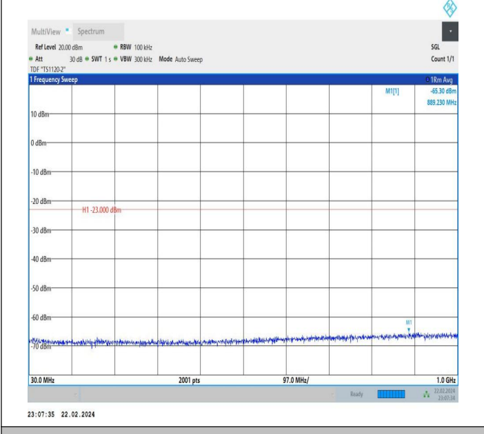
66-66-20MHz-20MHz-QPSK-QPSK-132374-132572-1RB#99-0 RB#0-30~1000MHz-PASS
