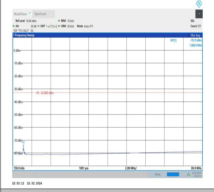
66-66-20MHz-20MHz-QPSK-QPSK-132323-132521-1RB#99-0 RB#0-0.15~30MHz-PASS
