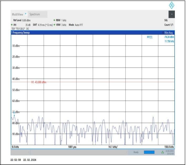
66-66-20MHz-20MHz-QPSK-QPSK-132323-132521-1RB#99-0 RB#0-0.009~0.15MHz-PASS
