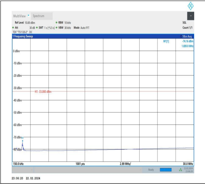
66-66-20MHz-20MHz-QPSK-QPSK-132374-132572-1RB#0-0 RB#0-0.15~30MHz-PASS
