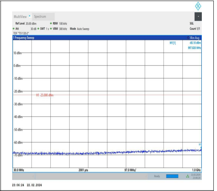
66-66-20MHz-20MHz-QPSK-QPSK-132374-132572-1RB#0-0 RB#0-30~1000MHz-PASS
