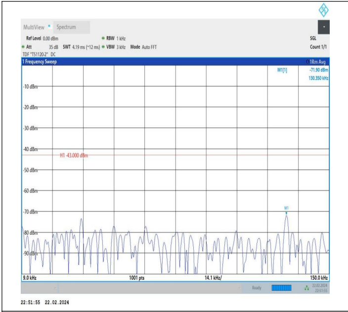
66-66-20MHz-20MHz-QPSK-QPSK-132323-132521-1RB#0-0 RB#0-0.009~0.15MHz-PASS
