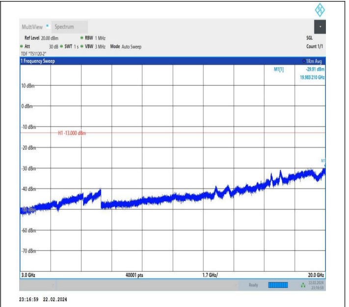
66-66-20MHz-20MHz-QPSK-QPSK-132374-132572-1RB#0-1 RB#99-3000~20000MHz-PASS
