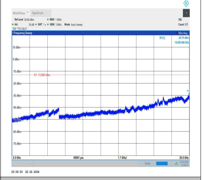
66-66-20MHz-20MHz-QPSK-QPSK-132374-132572-1RB#0-0 RB#0-3000~20000MHz-PASS
