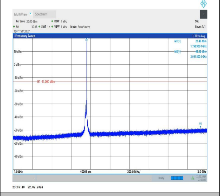
66-66-20MHz-20MHz-QPSK-QPSK-132374-132572-1RB#99-0 RB#0-1000~3000MHz-PASS
