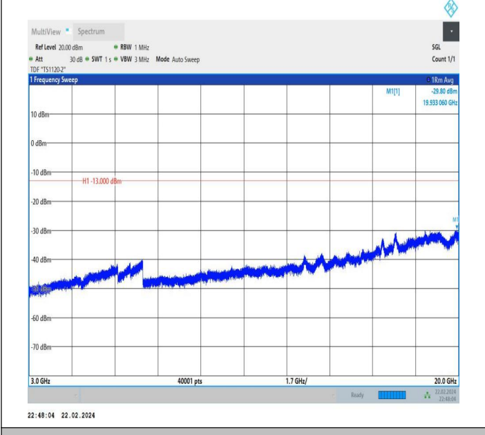
66-66-20MHz-20MHz-QPSK-QPSK-132072-132270-1RB#99-0 RB#0-3000~20000MHz-PASS
