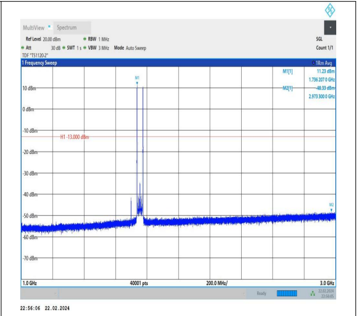
66-66-20MHz-20MHz-QPSK-QPSK-132323-132521-1RB#0-1 RB#99-1000~3000MHz-PASS
