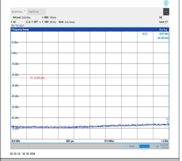
66-66-20MHz-20MHz-QPSK-QPSK-132323-132521-1RB#99-0 RB#0-30~1000MHz-PASS
