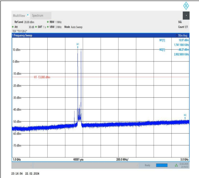
66-66-20MHz-20MHz-QPSK-QPSK-132374-132572-1RB#0-1 RB#99-1000~3000MHz-PASS
