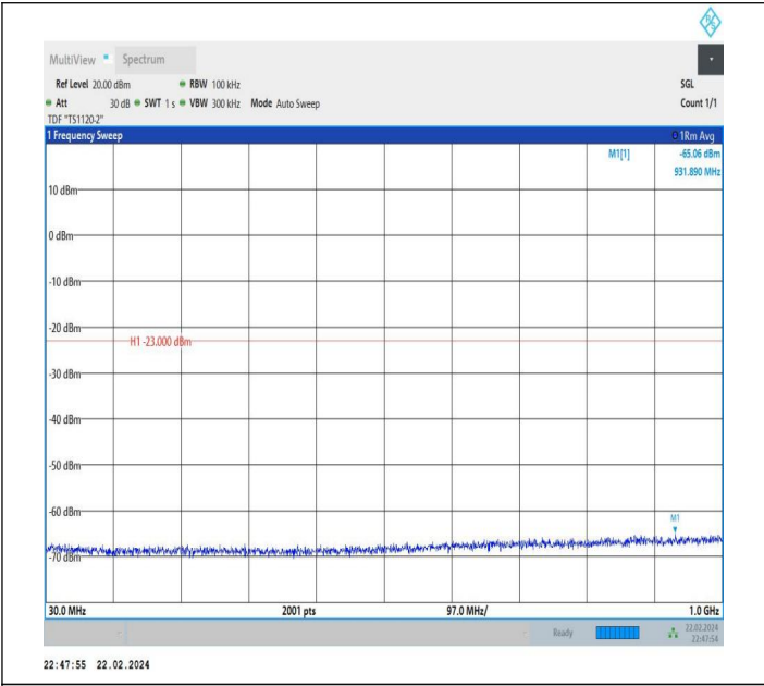
66-66-20MHz-20MHz-QPSK-QPSK-132072-132270-1RB#99-0 RB#0-30~1000MHz-PASS
