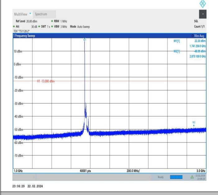
66-66-20MHz-20MHz-QPSK-QPSK-132374-132572-1RB#0-0 RB#0-1000~3000MHz-PASS
