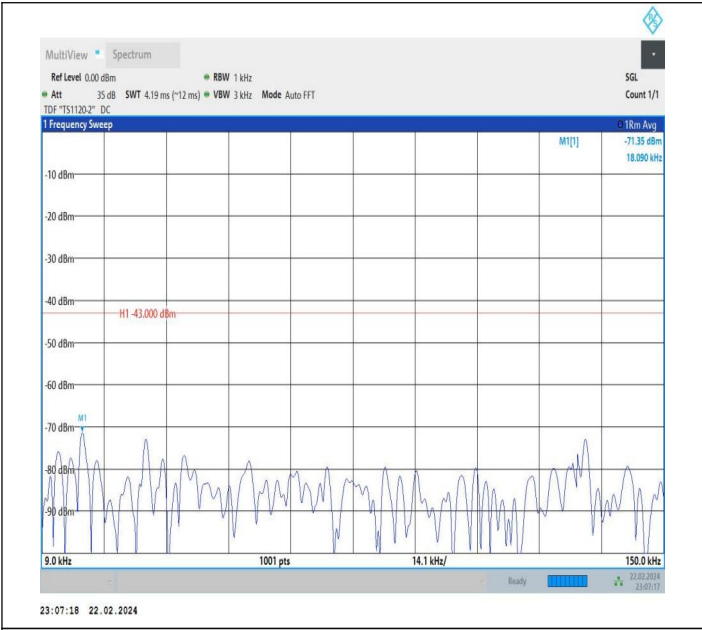
66-66-20MHz-20MHz-QPSK-QPSK-132374-132572-1RB#99-0 RB#0-0.009~0.15MHz-PASS
