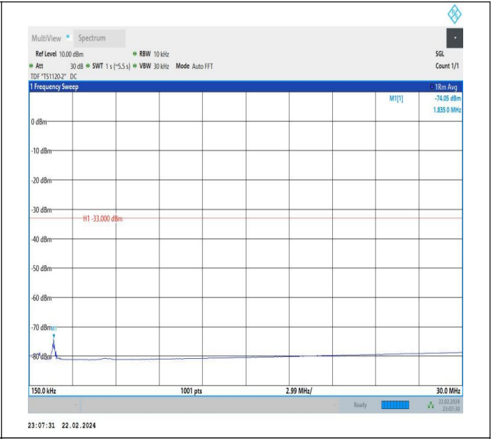
66-66-20MHz-20MHz-QPSK-QPSK-132374-132572-1RB#99-0 RB#0-0.15~30MHz-PASS
