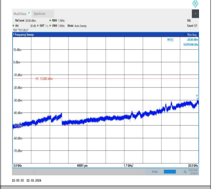
66-66-20MHz-20MHz-QPSK-QPSK-132072-132270-1RB#0-1 RB#99-3000~20000MHz-PASS
