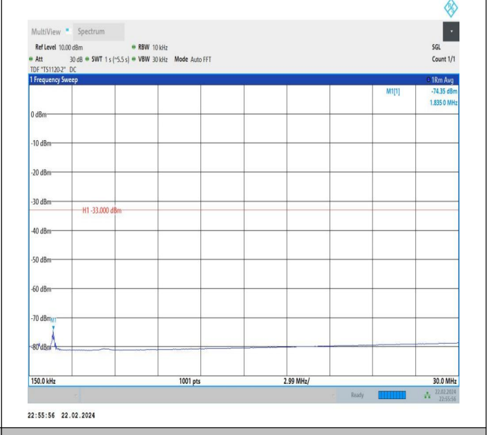
66-66-20MHz-20MHz-QPSK-QPSK-132323-132521-1RB#0-1 RB#99-0.15~30MHz-PASS
