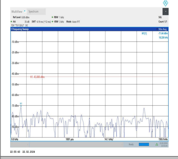
66-66-20MHz-20MHz-QPSK-QPSK-132323-132521-1RB#0-1 RB#99-0.009~0.15MHz-PASS
