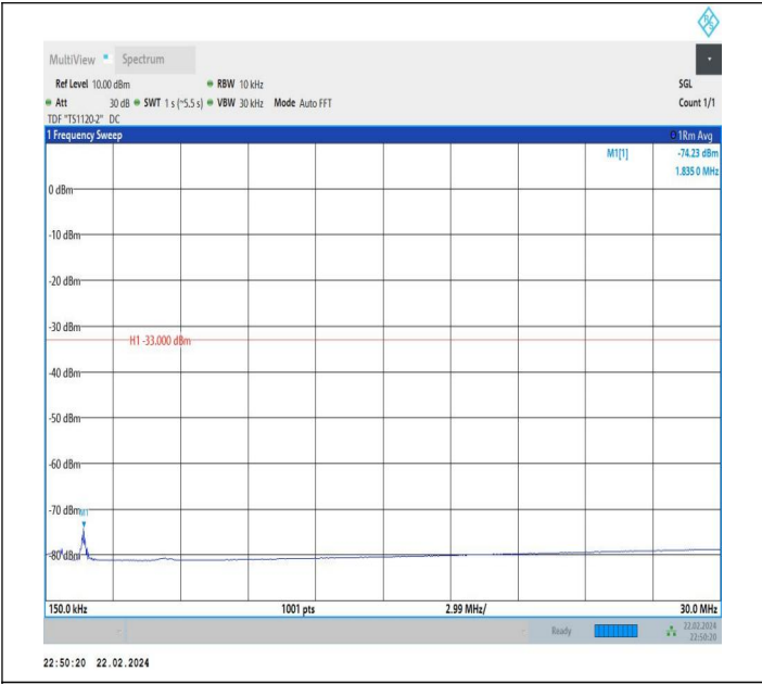
66-66-20MHz-20MHz-QPSK-QPSK-132072-132270-1RB#0-1 RB#99-0.15~30MHz-PASS
