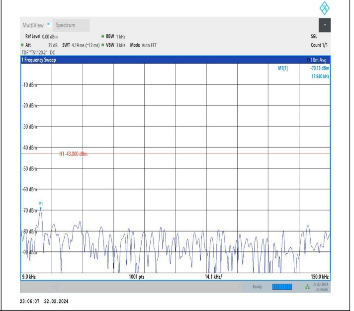
66-66-20MHz-20MHz-QPSK-QPSK-132374-132572-1RB#0-0 RB#0-0.009~0.15MHz-PASS
