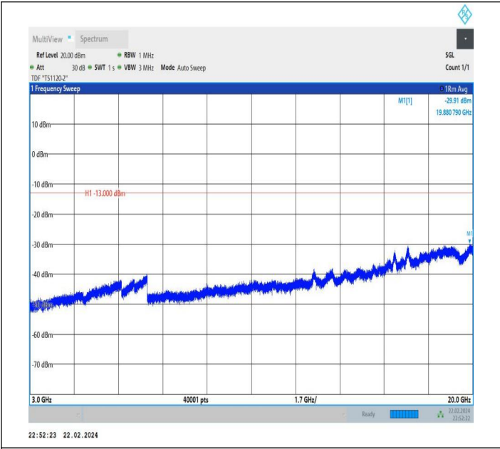
66-66-20MHz-20MHz-QPSK-QPSK-132323-132521-1RB#0-0 RB#0-3000~20000MHz-PASS
