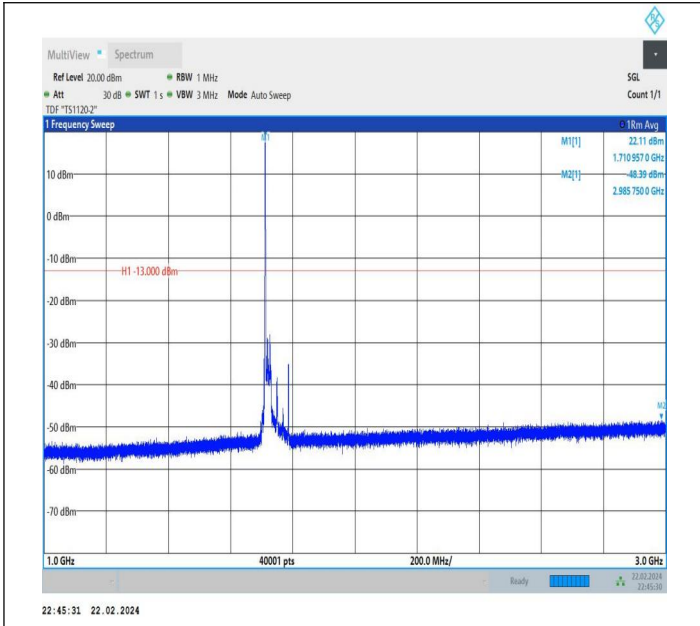
66-66-20MHz-20MHz-QPSK-QPSK-132072-132270-1RB#0-0 RB#0-1000~3000MHz-PASS
