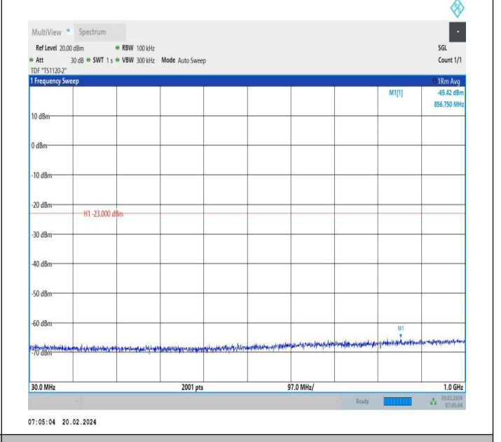
66-66-20MHz-10MHz-QPSK-QPSK-132473-132617-1RB#0-0 RB#0-30~1000MHz-PASS
