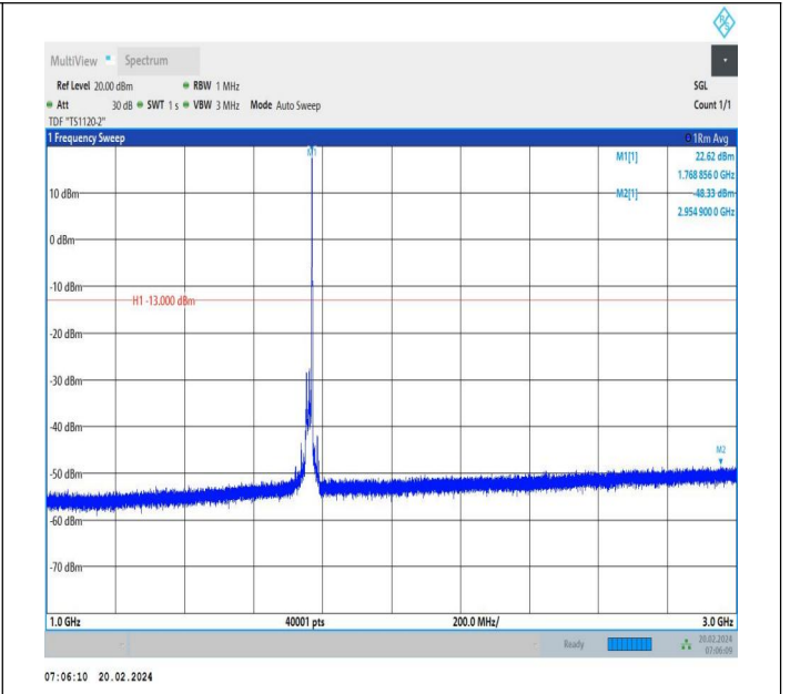
66-66-20MHz-10MHz-QPSK-QPSK-132473-132617-1RB#99-0 RB#0-1000~3000MHz-PASS
