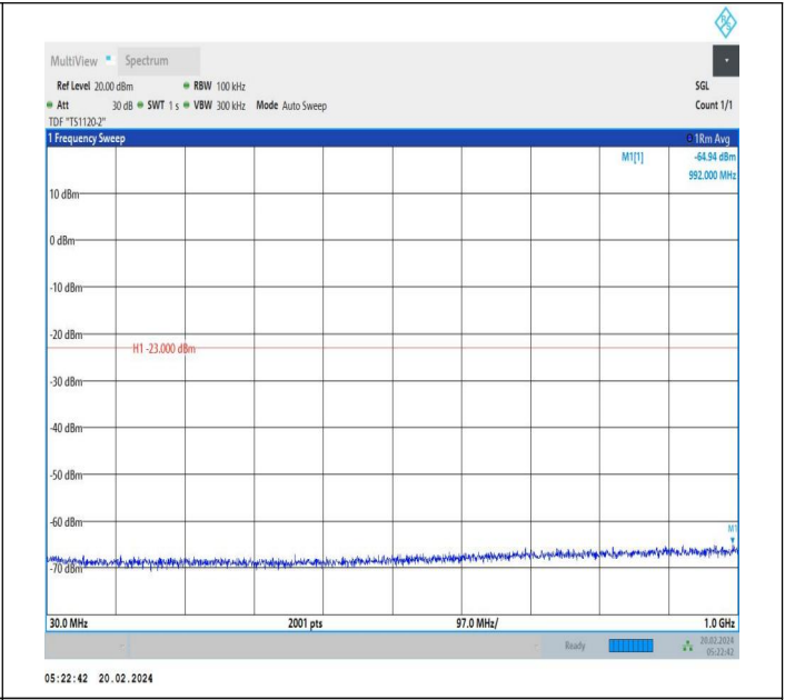
66-66-15MHz-20MHz-QPSK-QPSK-132401-132572-1RB#0-0 RB#0-30~1000MHz-PASS
