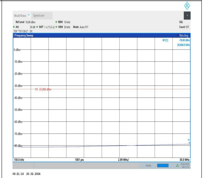
66-66-20MHz-5MHz-QPSK-QPSK-132397-132514-1RB#99-0 RB#0-0.15~30MHz-PASS
