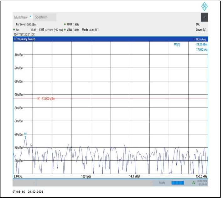
66-66-20MHz-10MHz-QPSK-QPSK-132473-132617-1RB#0-0 RB#0-0.009~0.15MHz-PASS
