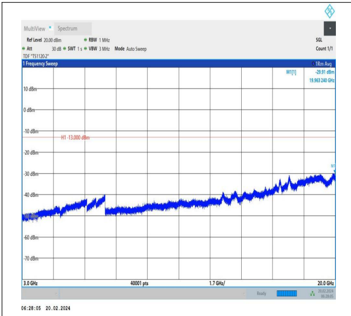
66-66-20MHz-5MHz-QPSK-QPSK-132522-132639-1RB#0-0R B#0-3000~20000MHz-PASS
