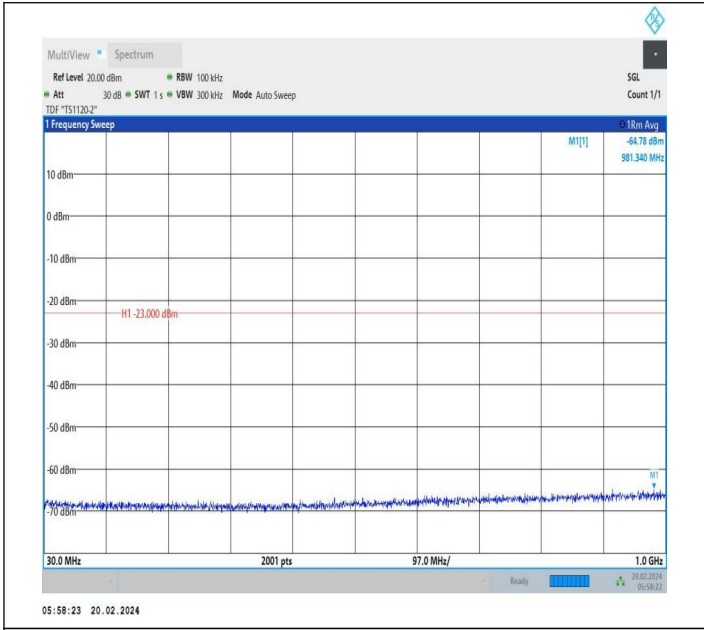
66-66-20MHz-5MHz-QPSK-QPSK-132072-132189-1RB#0-0R B#0-30~1000MHz-PASS
