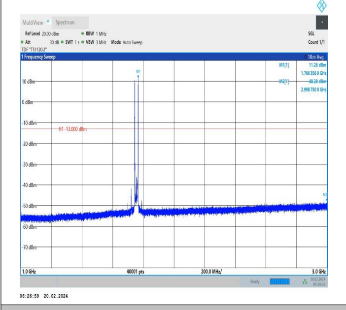
66-66-20MHz-5MHz-QPSK-QPSK-132397-132514-1RB#0-1R B#24-1000~3000MHz-PASS
