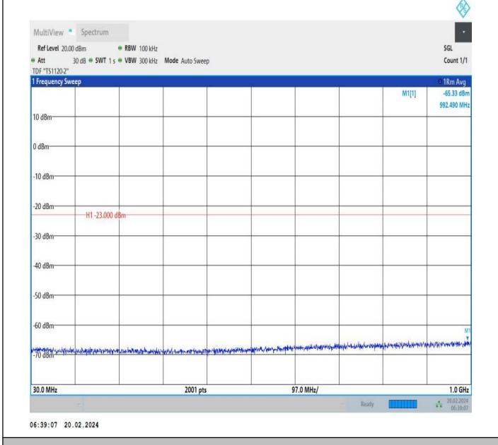
66-66-20MHz-10MHz-QPSK-QPSK-132072-132216-1RB#99-0 RB#0-30~1000MHz-PASS
