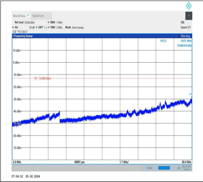
66-66-20MHz-10MHz-QPSK-QPSK-132373-132517-1RB#0-1 RB#49-3000~20000MHz-PASS
