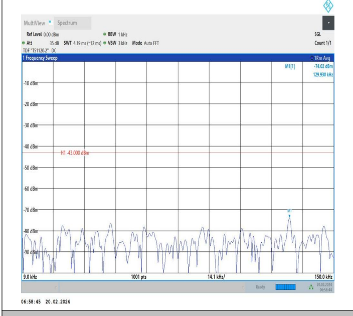
66-66-20MHz-10MHz-QPSK-QPSK-132373-132517-1RB#0-0 RB#0-0.009~0.15MHz-PASS
