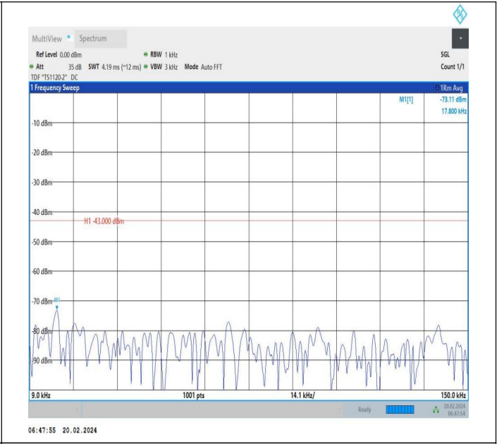
66-66-20MHz-10MHz-QPSK-QPSK-132072-132216-1RB#0-1 RB#49-0.009~0.15MHz-PASS
