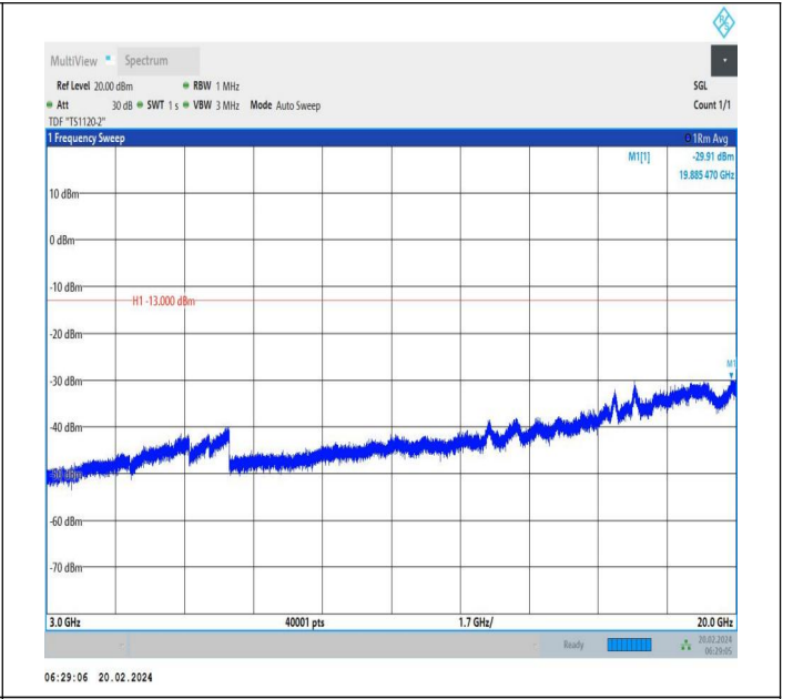
66-66-20MHz-5MHz-QPSK-QPSK-132522-132639-1RB#99-0 RB#0-3000~20000MHz-PASS
