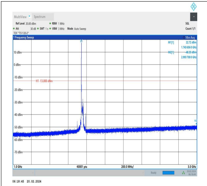
66-66-20MHz-5MHz-QPSK-QPSK-132397-132514-1RB#0-0R B#0-1000~3000MHz-PASS
