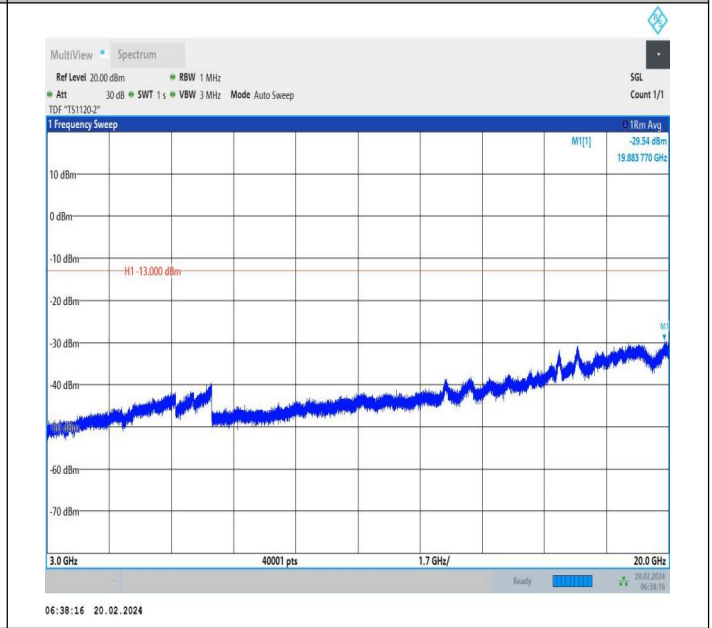
66-66-20MHz-10MHz-QPSK-QPSK-132072-132216-1RB#0-0 RB#0-3000~20000MHz-PASS
