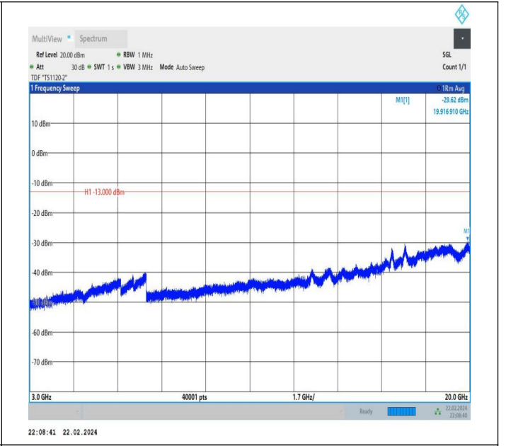
66-66-20MHz-15MHz-QPSK-QPSK-132072-132243-1RB#99-0 RB#0-3000~20000MHz-PASS
