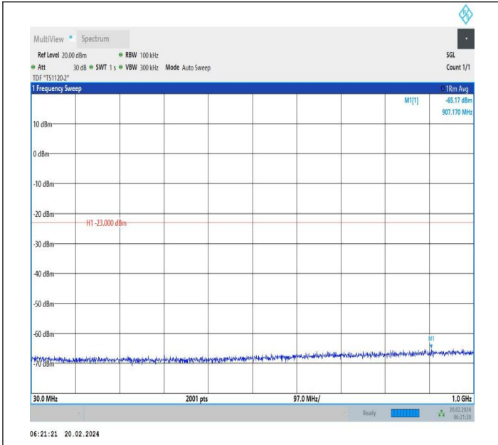
66-66-20MHz-5MHz-QPSK-QPSK-132397-132514-1RB#99-0 RB#0-30~1000MHz-PASS
