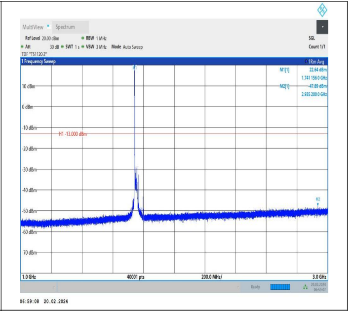
66-66-20MHz-10MHz-QPSK-QPSK-132373-132517-1RB#0-0 RB#0-1000~3000MHz-PASS
