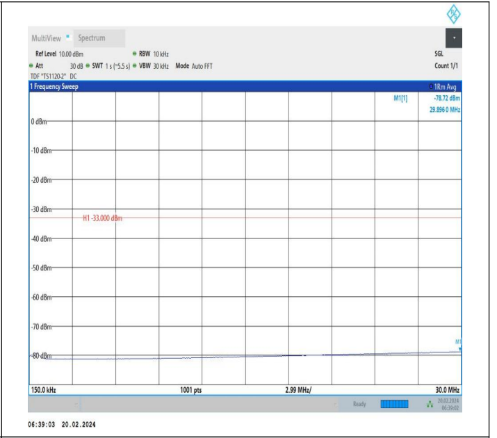
66-66-20MHz-10MHz-QPSK-QPSK-132072-132216-1RB#99-0 RB#0-0.15~30MHz-PASS
