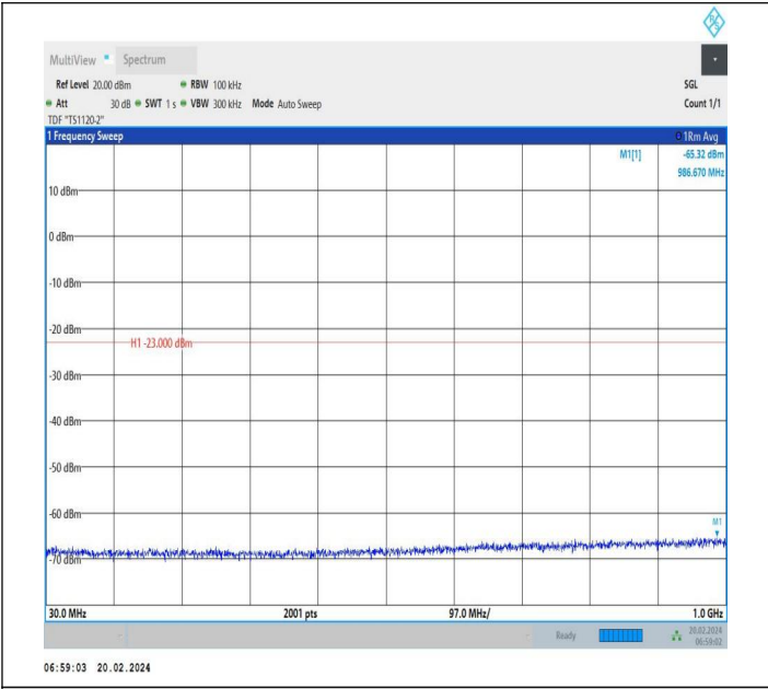
66-66-20MHz-10MHz-QPSK-QPSK-132373-132517-1RB#0-0 RB#0-30~1000MHz-PASS
