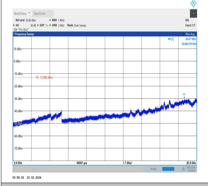
66-66-20MHz-5MHz-QPSK-QPSK-132072-132189-1RB#0-0R B#0-3000~20000MHz-PASS
