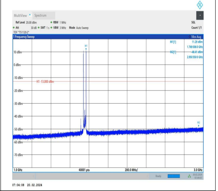
66-66-20MHz-10MHz-QPSK-QPSK-132373-132517-1RB#0-1 RB#49-1000~3000MHz-PASS
