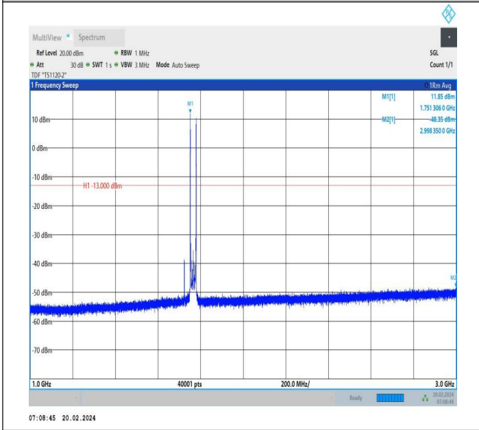
66-66-20MHz-10MHz-QPSK-QPSK-132473-132617-1RB#0-1 RB#49-1000~3000MHz-PASS
