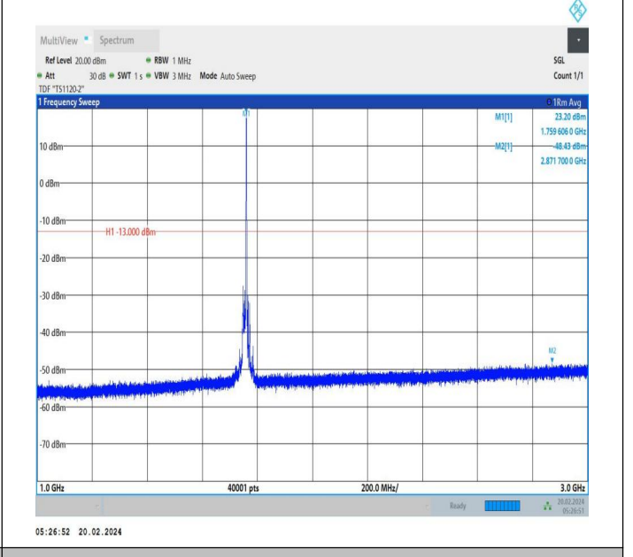
66-66-15MHz-20MHz-QPSK-QPSK-132401-132572-1RB#74-0 RB#0-1000~3000MHz-PASS
