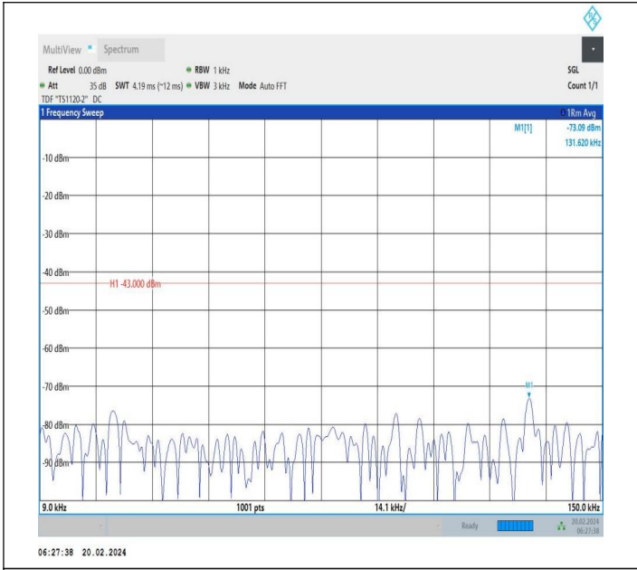
66-66-20MHz-5MHz-QPSK-QPSK-132522-132639-1RB#0-0R B#0-0.009~0.15MHz-PASS
