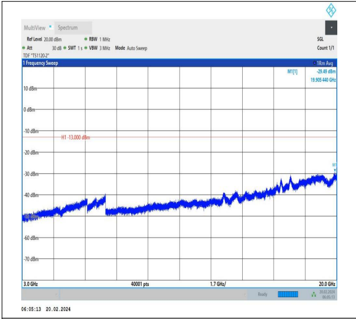
66-66-20MHz-5MHz-QPSK-QPSK-132072-132189-1RB#0-1R B#24-3000~20000MHz-PASS
