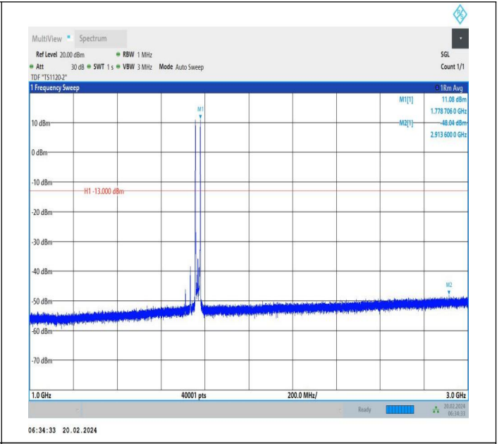
66-66-20MHz-5MHz-QPSK-QPSK-132522-132639-1RB#0-1R B#24-1000~3000MHz-PASS
