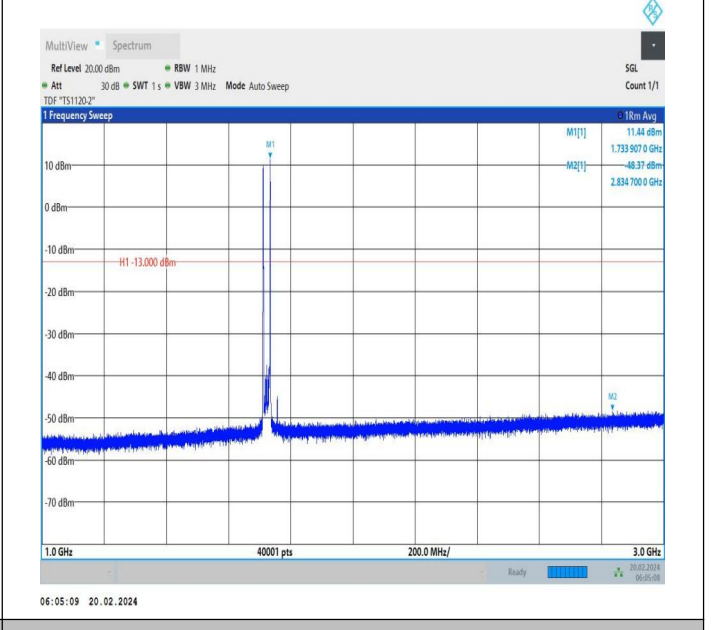
66-66-20MHz-5MHz-QPSK-QPSK-132072-132189-1RB#0-1R B#24-1000~3000MHz-PASS
