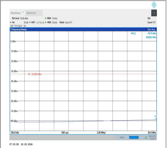
66-66-20MHz-10MHz-QPSK-QPSK-132373-132517-1RB#0-1 RB#49-0.15~30MHz-PASS
