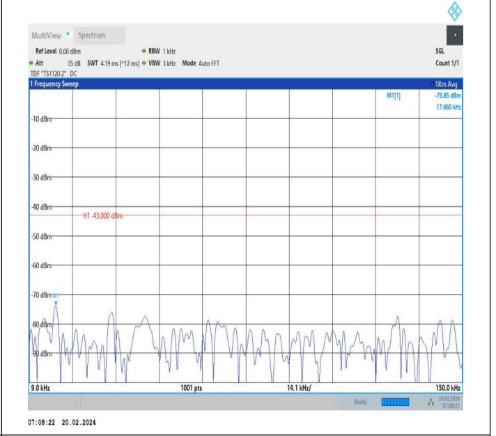
66-66-20MHz-10MHz-QPSK-QPSK-132473-132617-1RB#0-1 RB#49-0.009~0.15MHz-PASS
