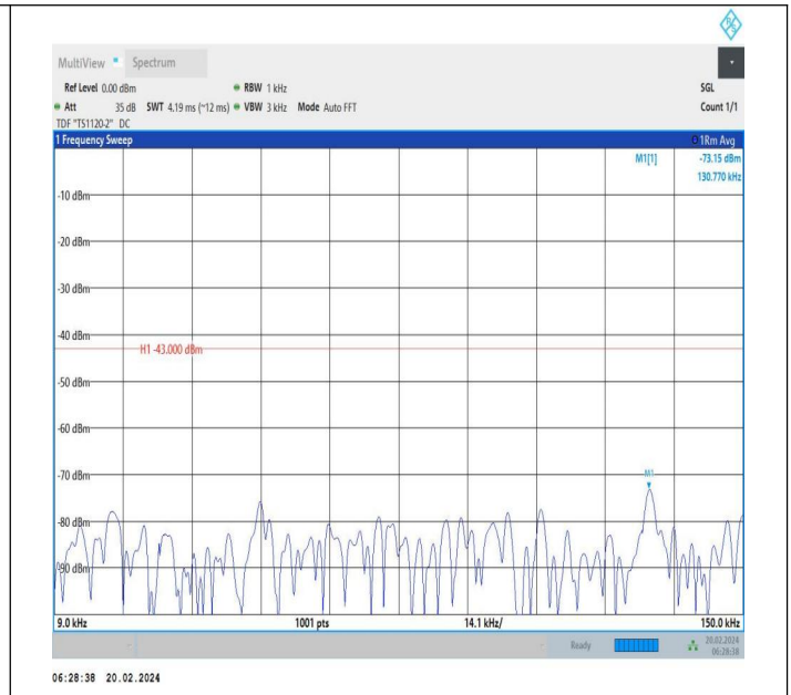
66-66-20MHz-5MHz-QPSK-QPSK-132522-132639-1RB#99-0 RB#0-0.009~0.15MHz-PASS
