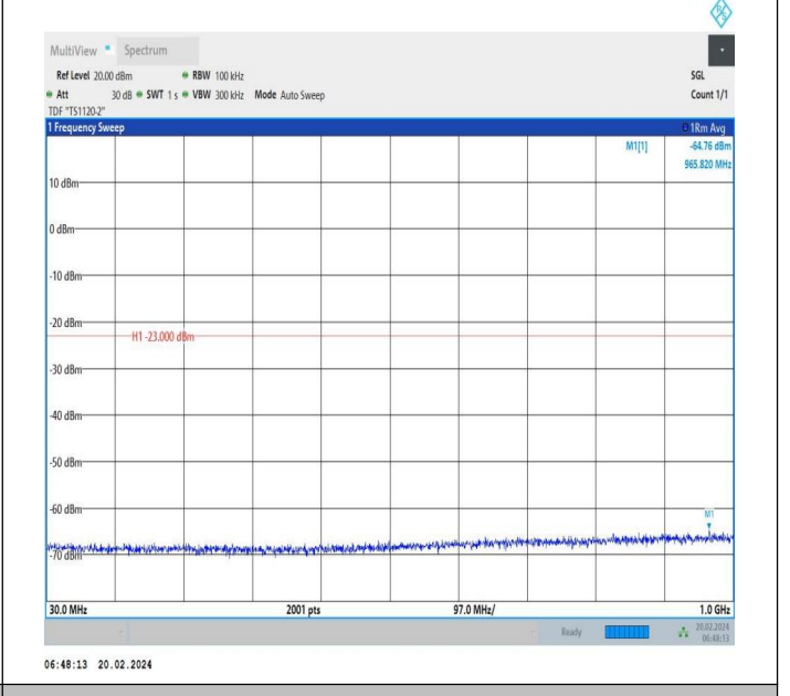
66-66-20MHz-10MHz-QPSK-QPSK-132072-132216-1RB#0-1 RB#49-30~1000MHz-PASS
