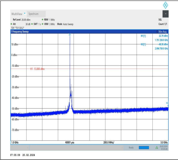
66-66-20MHz-10MHz-QPSK-QPSK-132473-132617-1RB#0-0 RB#0-1000~3000MHz-PASS
