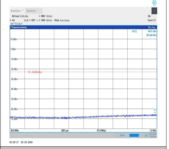
66-66-15MHz-20MHz-QPSK-QPSK-132401-132572-1RB#0-1 RB#99-30~1000MHz-PASS
