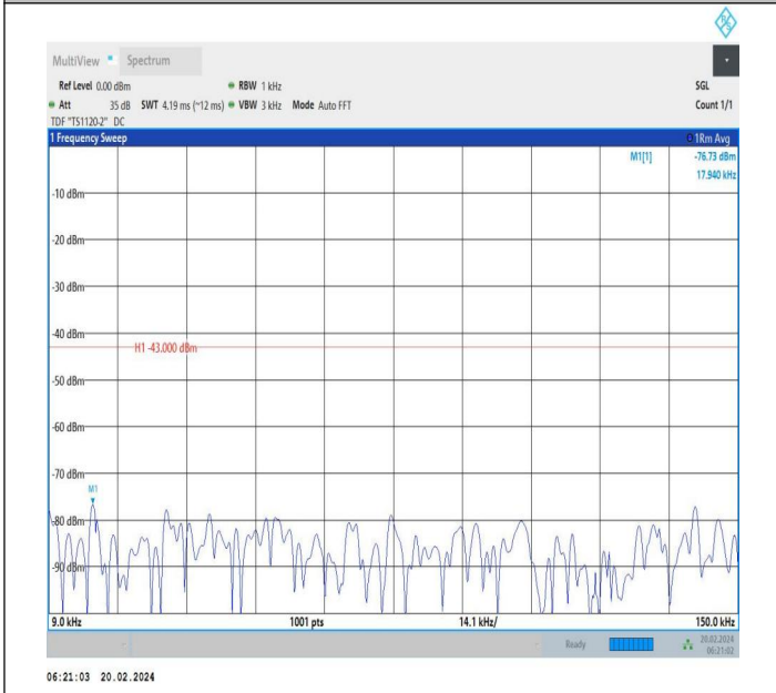
66-66-20MHz-5MHz-QPSK-QPSK-132397-132514-1RB#99-0 RB#0-0.009~0.15MHz-PASS
