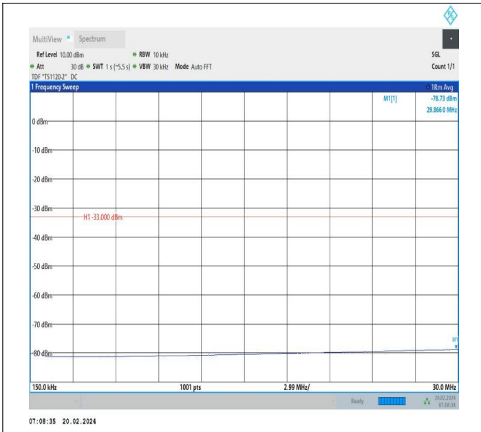
66-66-20MHz-10MHz-QPSK-QPSK-132473-132617-1RB#0-1 RB#49-0.15~30MHz-PASS
