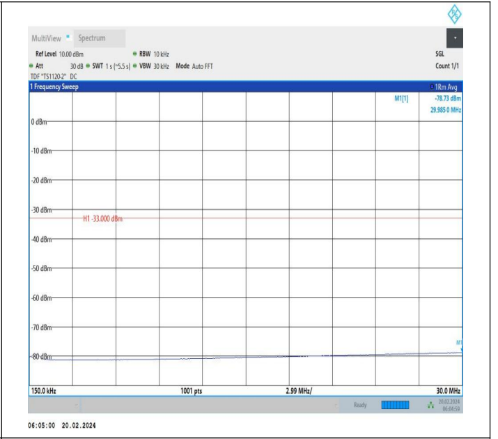
66-66-20MHz-5MHz-QPSK-QPSK-132072-132189-1RB#0-1R B#24-0.15~30MHz-PASS
