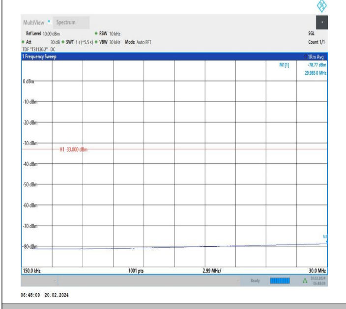
66-66-20MHz-10MHz-QPSK-QPSK-132072-132216-1RB#0-1 RB#49-0.15~30MHz-PASS
