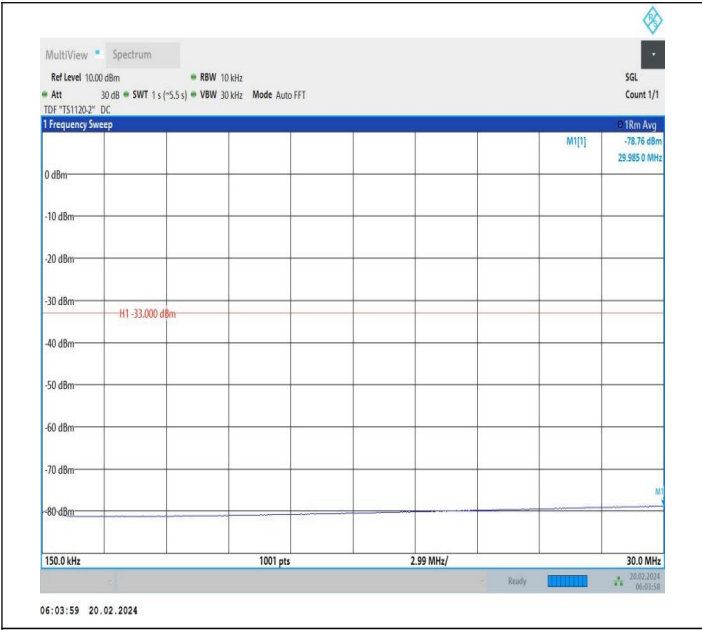
66-66-20MHz-5MHz-QPSK-QPSK-132072-132189-1RB#99-0 RB#0-0.15~30MHz-PASS
