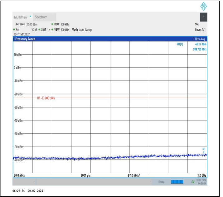
66-66-20MHz-5MHz-QPSK-QPSK-132397-132514-1RB#0-1R B#24-30~1000MHz-PASS
