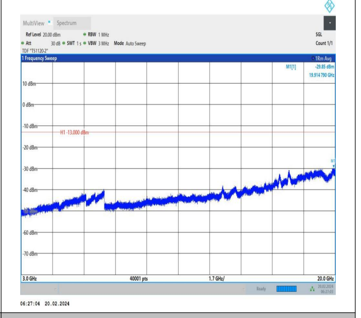
66-66-20MHz-5MHz-QPSK-QPSK-132397-132514-1RB#0-1R B#24-3000~20000MHz-PASS
