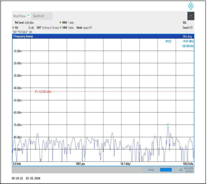
66-66-20MHz-5MHz-QPSK-QPSK-132397-132514-1RB#0-0R B#0-0.009~0.15MHz-PASS
