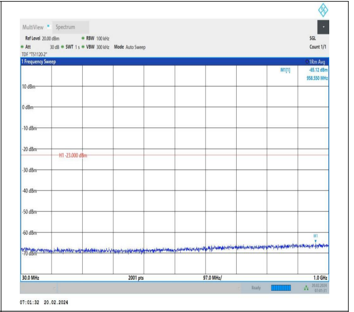
66-66-20MHz-10MHz-QPSK-QPSK-132373-132517-1RB#99-0 RB#0-30~1000MHz-PASS
