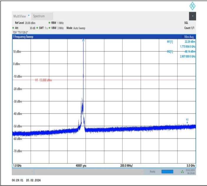
66-66-20MHz-5MHz-QPSK-QPSK-132522-132639-1RB#99-0 RB#0-1000~3000MHz-PASS
