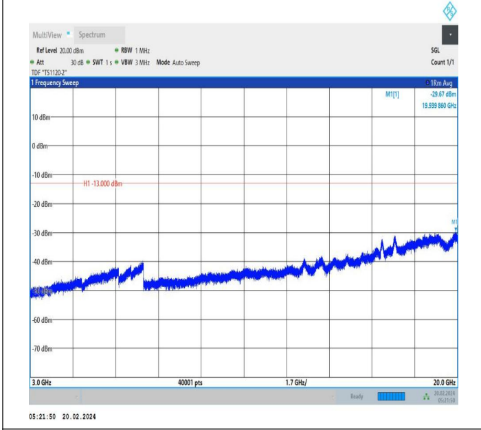
66-66-15MHz-20MHz-QPSK-QPSK-132325-132496-1RB#0-1 RB#99-3000~20000MHz-PASS
