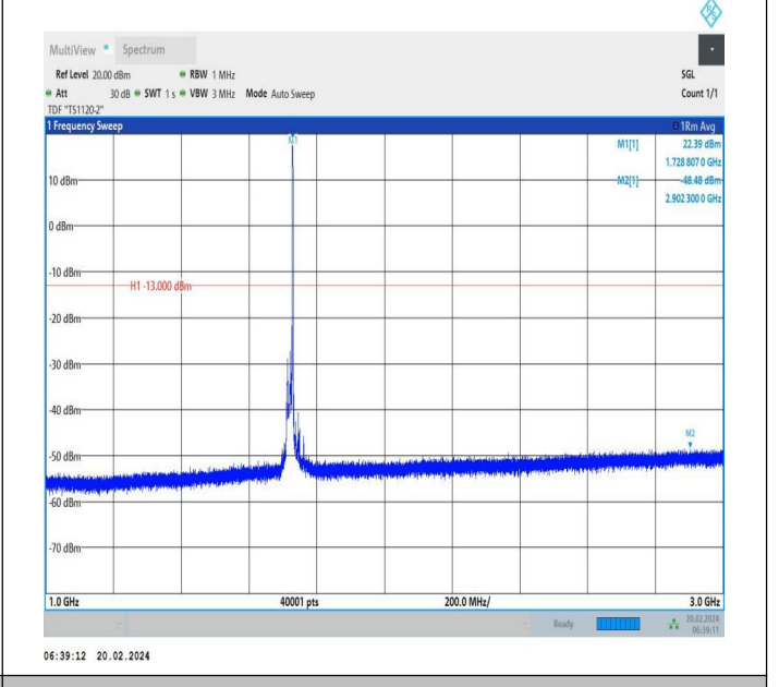
66-66-20MHz-10MHz-QPSK-QPSK-132072-132216-1RB#99-0 RB#0-1000~3000MHz-PASS
