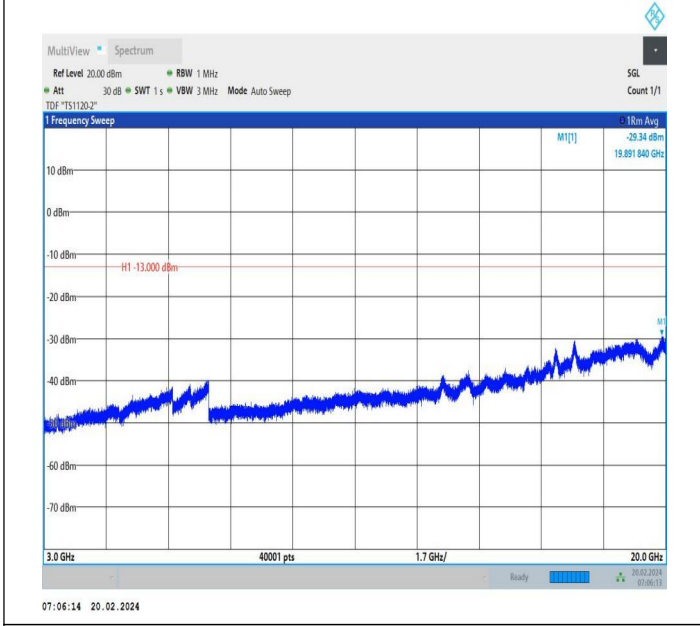
66-66-20MHz-10MHz-QPSK-QPSK-132473-132617-1RB#99-0 RB#0-3000~20000MHz-PASS
