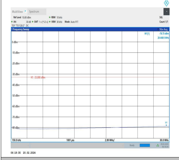
66-66-20MHz-5MHz-QPSK-QPSK-132397-132514-1RB#0-0R B#0-0.15~30MHz-PASS
