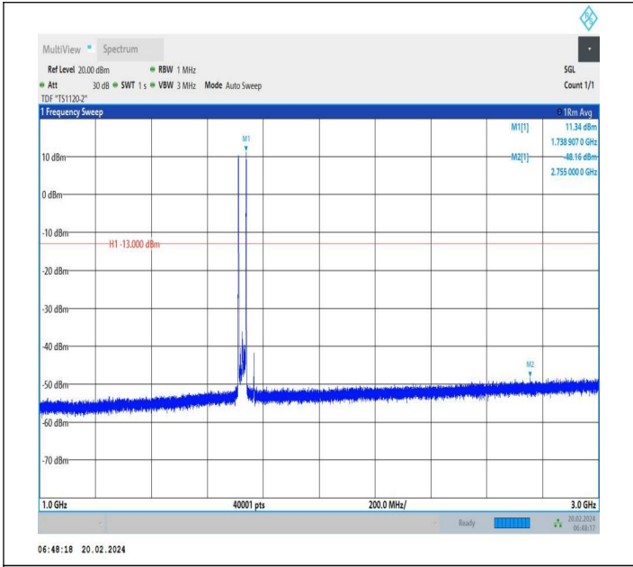
66-66-20MHz-10MHz-QPSK-QPSK-132072-132216-1RB#0-1 RB#49-1000~3000MHz-PASS
