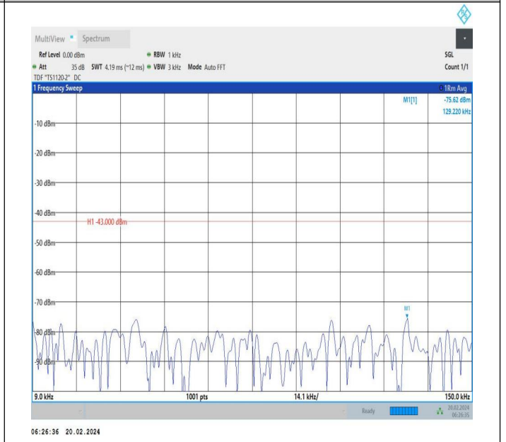
66-66-20MHz-5MHz-QPSK-QPSK-132397-132514-1RB#0-1R B#24-0.009~0.15MHz-PASS
