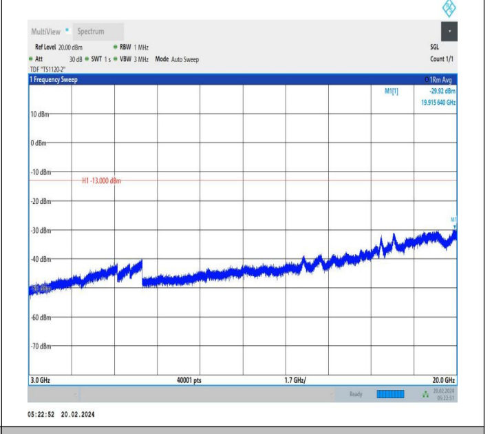
66-66-15MHz-20MHz-QPSK-QPSK-132401-132572-1RB#0-0 RB#0-3000~20000MHz-PASS
