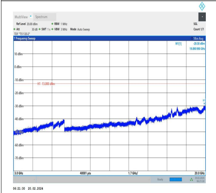
66-66-20MHz-5MHz-QPSK-QPSK-132397-132514-1RB#99-0 RB#0-3000~20000MHz-PASS
