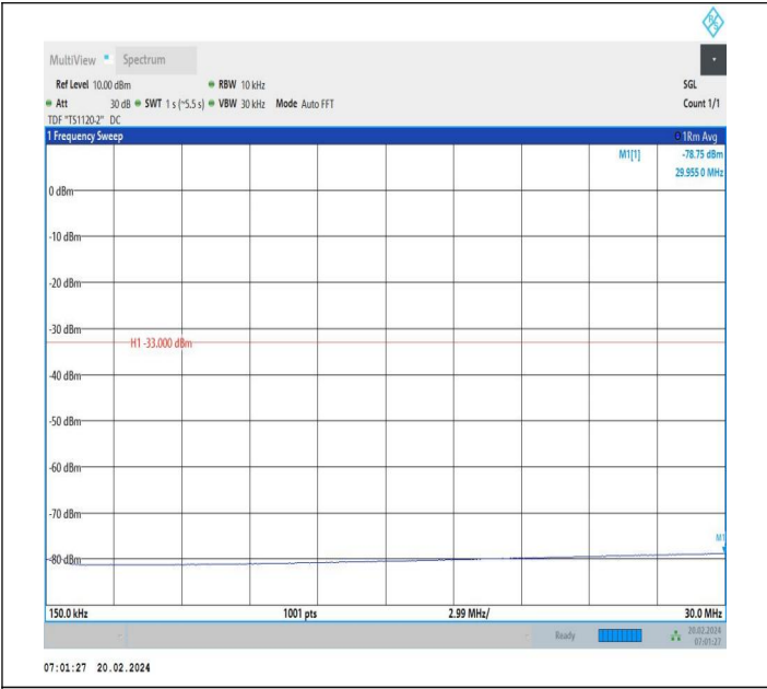
66-66-20MHz-10MHz-QPSK-QPSK-132373-132517-1RB#99-0 RB#0-0.15~30MHz-PASS
