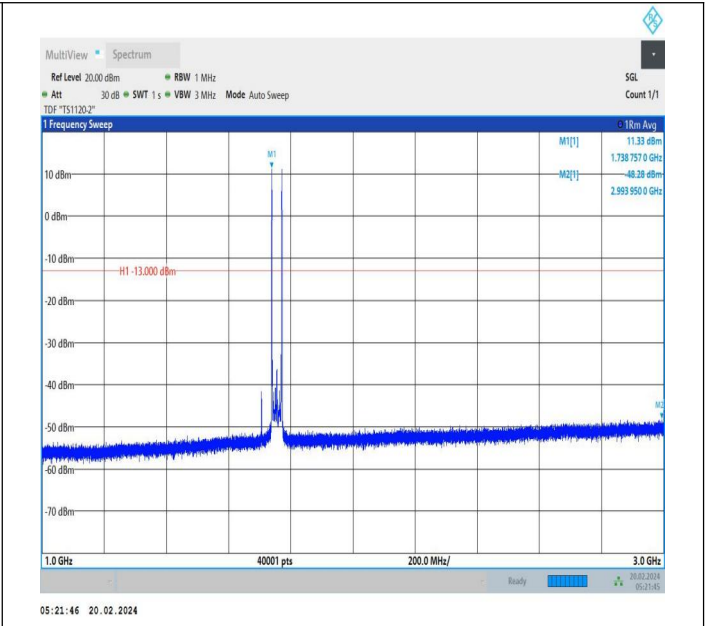
66-66-15MHz-20MHz-QPSK-QPSK-132325-132496-1RB#0-1 RB#99-1000~3000MHz-PASS
