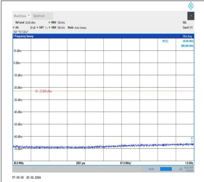
66-66-20MHz-10MHz-QPSK-QPSK-132473-132617-1RB#99-0 RB#0-30~1000MHz-PASS
