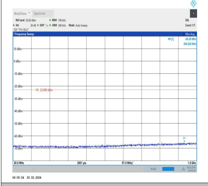
66-66-20MHz-5MHz-QPSK-QPSK-132072-132189-1RB#0-1R B#24-30~1000MHz-PASS
