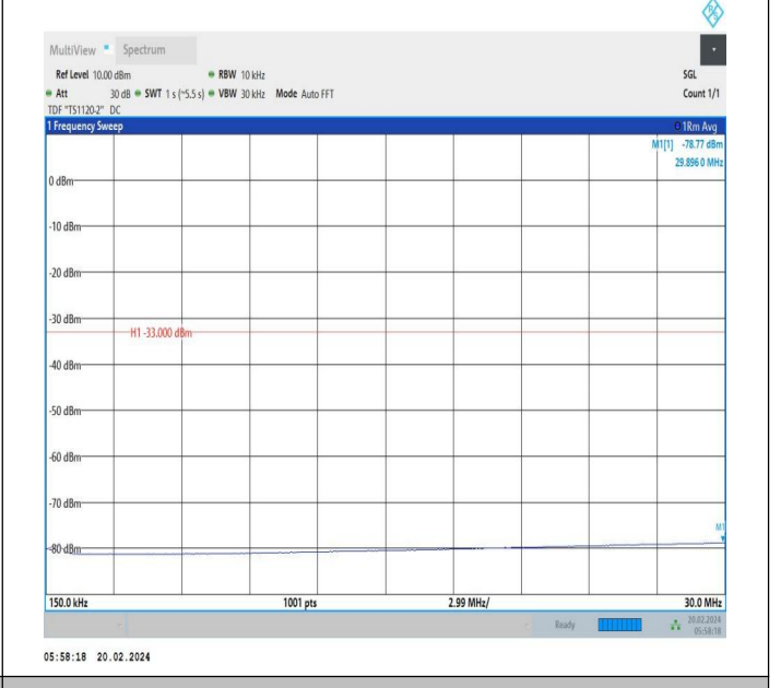
66-66-20MHz-5MHz-QPSK-QPSK-132072-132189-1RB#0-0R B#0-0.15~30MHz-PASS
