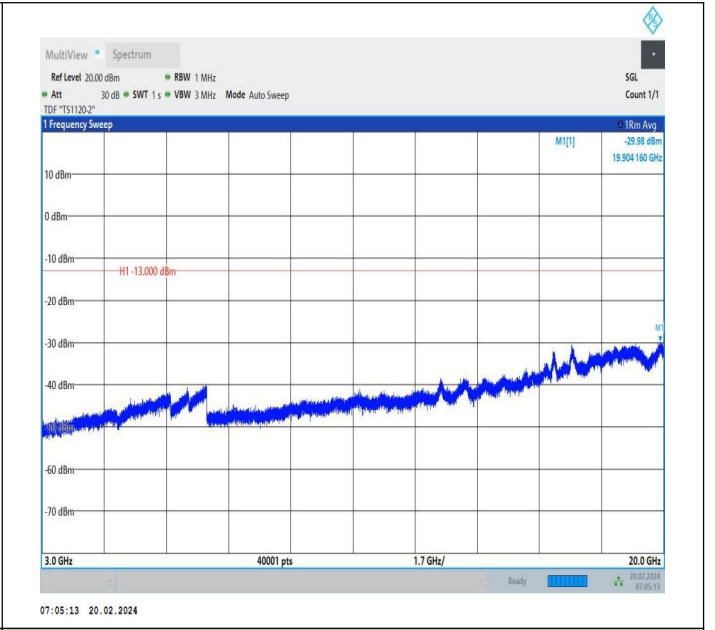
66-66-20MHz-10MHz-QPSK-QPSK-132473-132617-1RB#0-0 RB#0-3000~20000MHz-PASS
