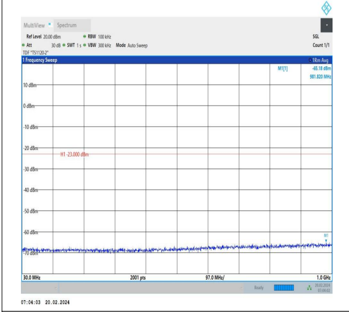
66-66-20MHz-10MHz-QPSK-QPSK-132373-132517-1RB#0-1 RB#49-30~1000MHz-PASS
