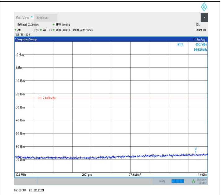
66-66-20MHz-10MHz-QPSK-QPSK-132072-132216-1RB#0-0 RB#0-30~1000MHz-PASS
