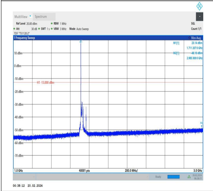
66-66-20MHz-10MHz-QPSK-QPSK-132072-132216-1RB#0-0 RB#0-1000~3000MHz-PASS
