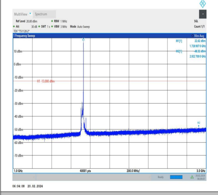
66-66-20MHz-5MHz-QPSK-QPSK-132072-132189-1RB#99-0 RB#0-1000~3000MHz-PASS
