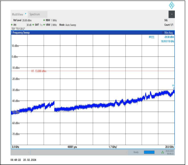
66-66-20MHz-10MHz-QPSK-QPSK-132072-132216-1RB#0-1 RB#49-3000~20000MHz-PASS
