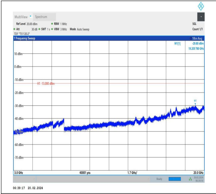
66-66-20MHz-10MHz-QPSK-QPSK-132072-132216-1RB#99-0 RB#0-3000~20000MHz-PASS
