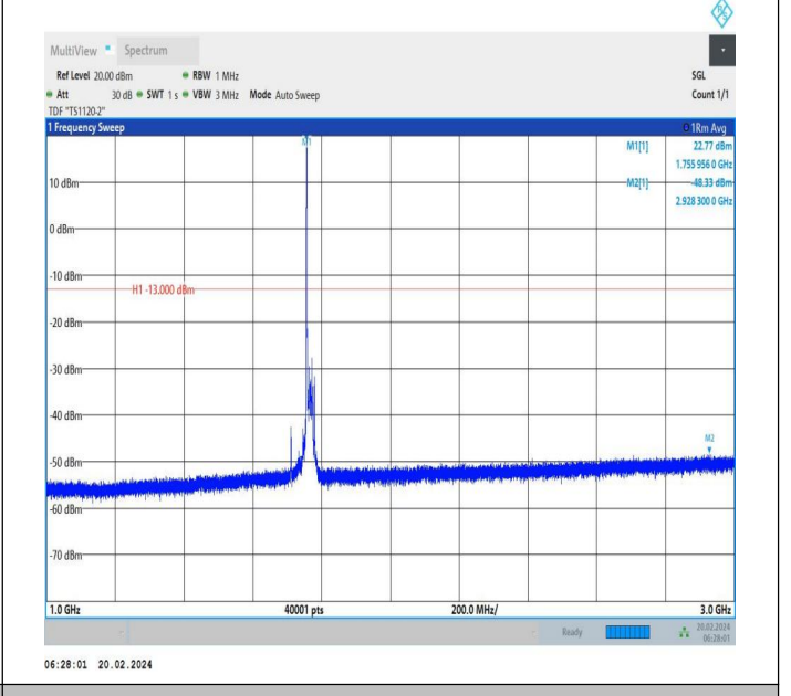
66-66-20MHz-5MHz-QPSK-QPSK-132522-132639-1RB#0-0R B#0-1000~3000MHz-PASS
