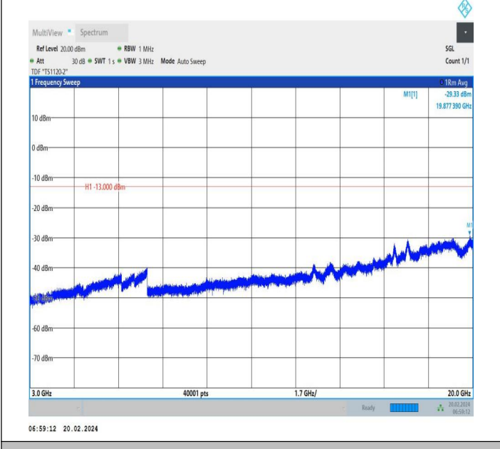
66-66-20MHz-10MHz-QPSK-QPSK-132373-132517-1RB#0-0 RB#0-3000~20000MHz-PASS
