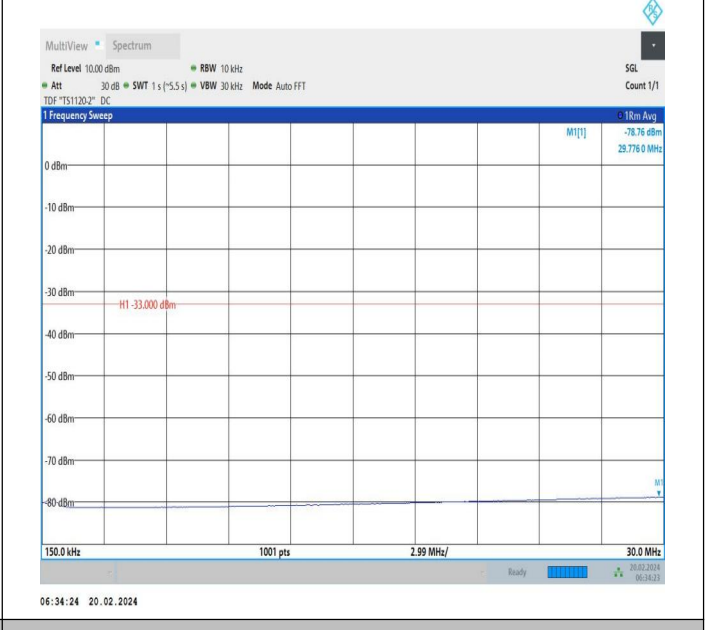
66-66-20MHz-5MHz-QPSK-QPSK-132522-132639-1RB#0-1R B#24-0.15~30MHz-PASS
