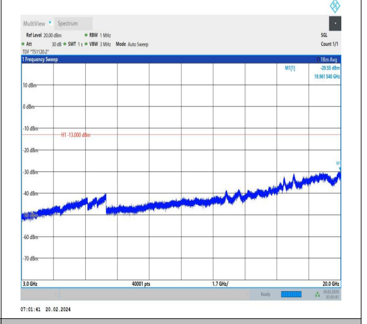
66-66-20MHz-10MHz-QPSK-QPSK-132373-132517-1RB#99-0 RB#0-3000~20000MHz-PASS
