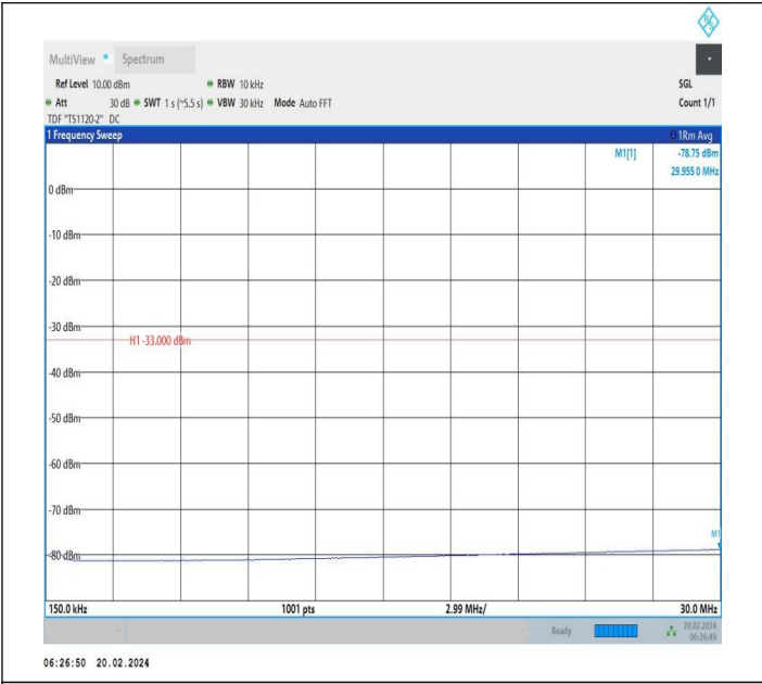
66-66-20MHz-5MHz-QPSK-QPSK-132397-132514-1RB#0-1R B#24-0.15~30MHz-PASS
