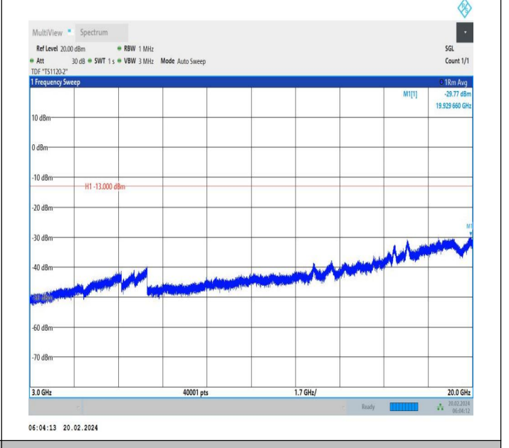
66-66-20MHz-5MHz-QPSK-QPSK-132072-132189-1RB#99-0 RB#0-3000~20000MHz-PASS
