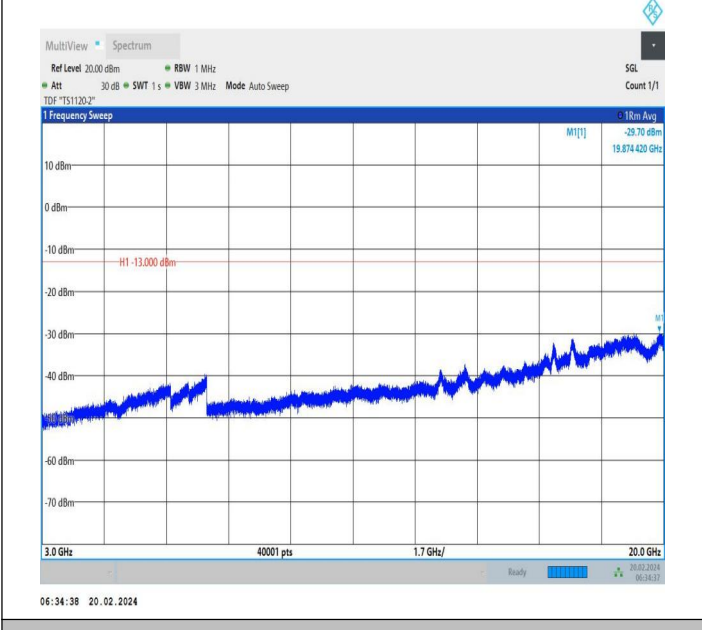
66-66-20MHz-5MHz-QPSK-QPSK-132522-132639-1RB#0-1R B#24-3000~20000MHz-PASS
