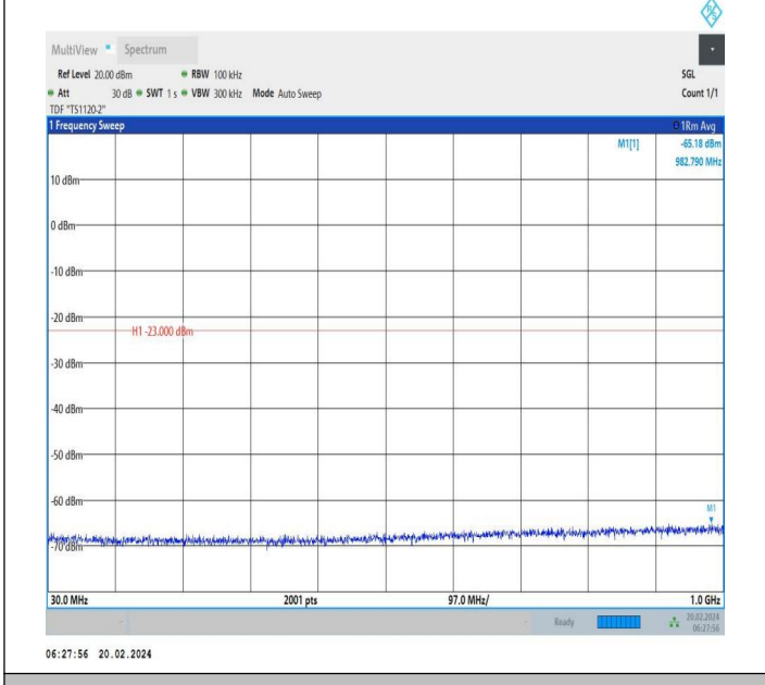
66-66-20MHz-5MHz-QPSK-QPSK-132522-132639-1RB#0-0R B#0-30~1000MHz-PASS
