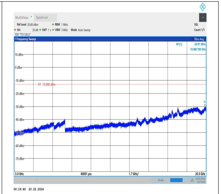
66-66-20MHz-5MHz-QPSK-QPSK-132397-132514-1RB#0-0R B#0-3000~20000MHz-PASS
