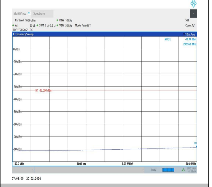
66-66-20MHz-10MHz-QPSK-QPSK-132473-132617-1RB#99-0 RB#0-0.15~30MHz-PASS
