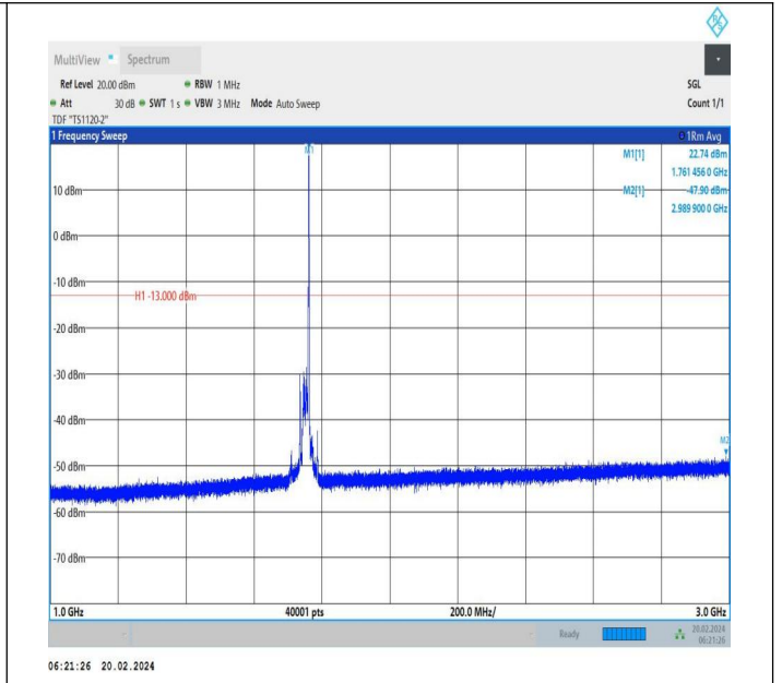
66-66-20MHz-5MHz-QPSK-QPSK-132397-132514-1RB#99-0 RB#0-1000~3000MHz-PASS
