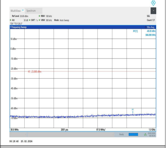
66-66-20MHz-5MHz-QPSK-QPSK-132397-132514-1RB#0-0R B#0-30~1000MHz-PASS
