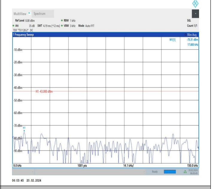
66-66-20MHz-5MHz-QPSK-QPSK-132072-132189-1RB#99-0 RB#0-0.009~0.15MHz-PASS
