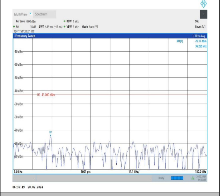
66-66-20MHz-10MHz-QPSK-QPSK-132072-132216-1RB#0-0 RB#0-0.009~0.15MHz-PASS
