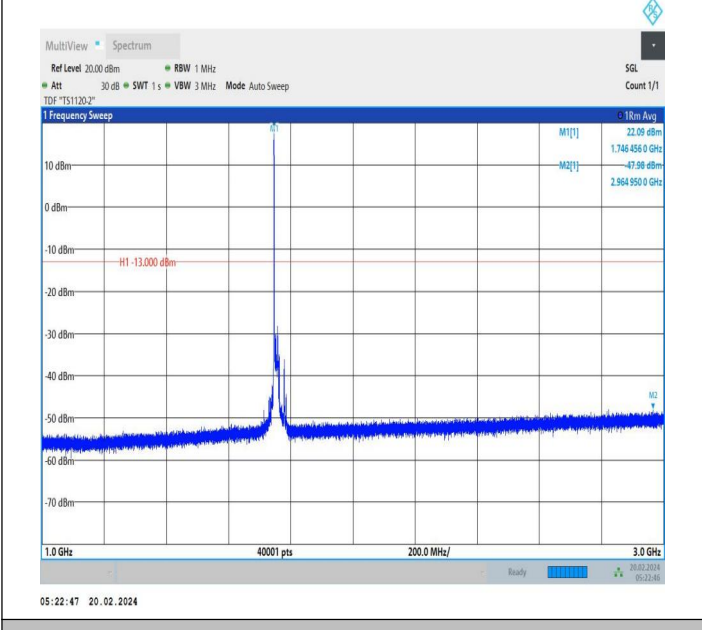
66-66-15MHz-20MHz-QPSK-QPSK-132401-132572-1RB#0-0 RB#0-1000~3000MHz-PASS
