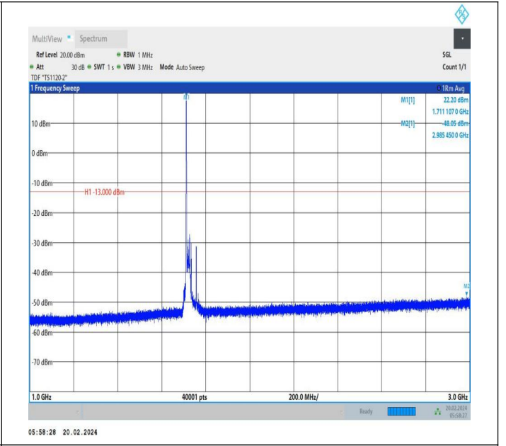
66-66-20MHz-5MHz-QPSK-QPSK-132072-132189-1RB#0-0R B#0-1000~3000MHz-PASS
