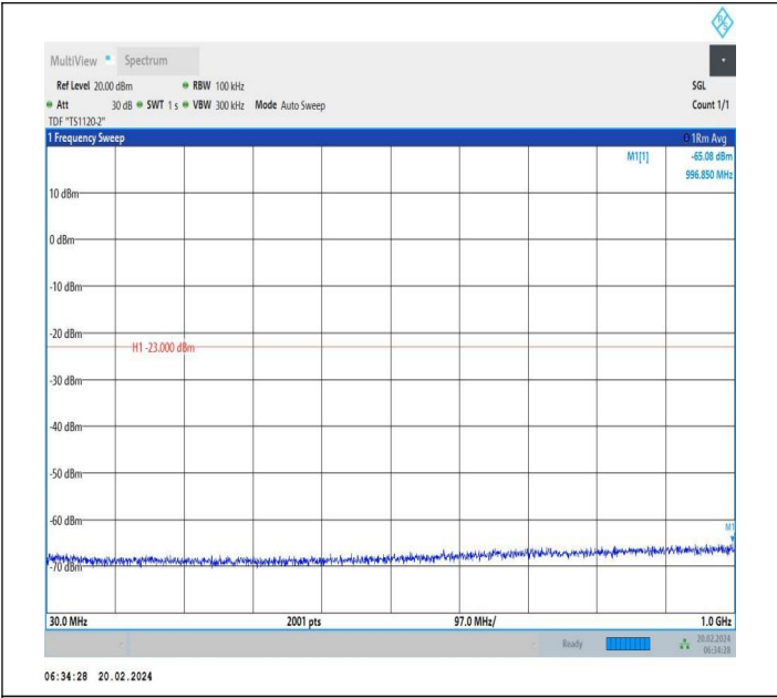
66-66-20MHz-5MHz-QPSK-QPSK-132522-132639-1RB#0-1R B#24-30~1000MHz-PASS
