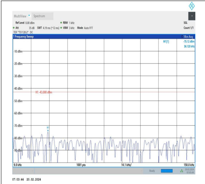
66-66-20MHz-10MHz-QPSK-QPSK-132373-132517-1RB#0-1 RB#49-0.009~0.15MHz-PASS
