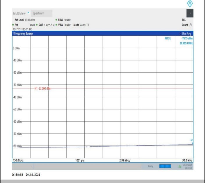
66-66-20MHz-10MHz-QPSK-QPSK-132373-132517-1RB#0-0 RB#0-0.15~30MHz-PASS
