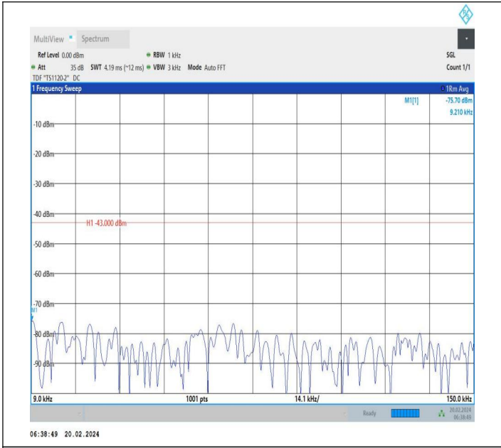
66-66-20MHz-10MHz-QPSK-QPSK-132072-132216-1RB#99-0 RB#0-0.009~0.15MHz-PASS
