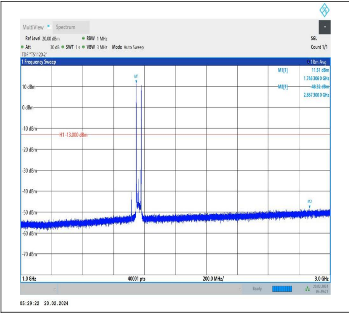
66-66-15MHz-20MHz-QPSK-QPSK-132401-132572-1RB#0-1 RB#99-1000~3000MHz-PASS
