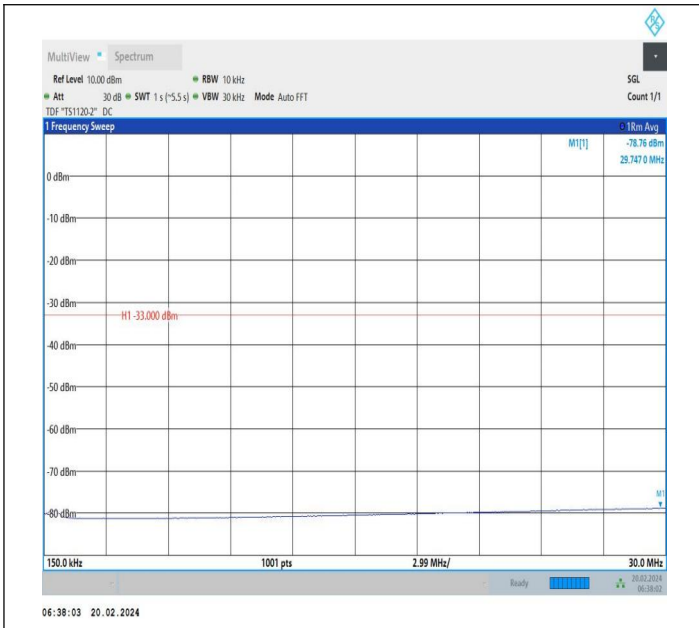
66-66-20MHz-10MHz-QPSK-QPSK-132072-132216-1RB#0-0 RB#0-0.15~30MHz-PASS
