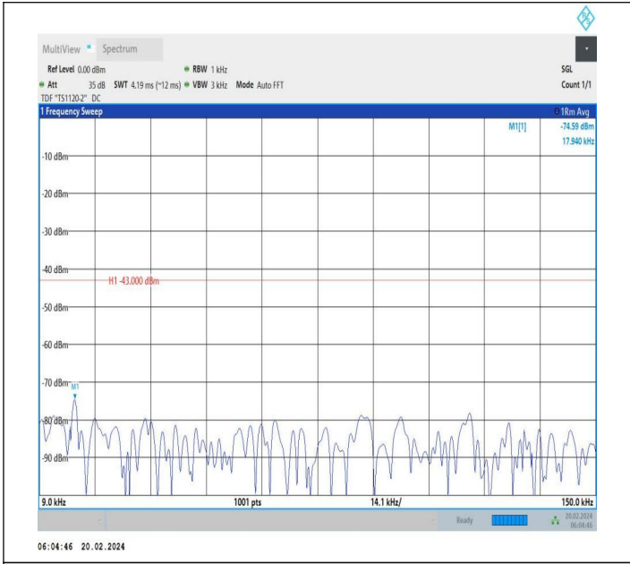
66-66-20MHz-5MHz-QPSK-QPSK-132072-132189-1RB#0-1R B#24-0.009~0.15MHz-PASS
