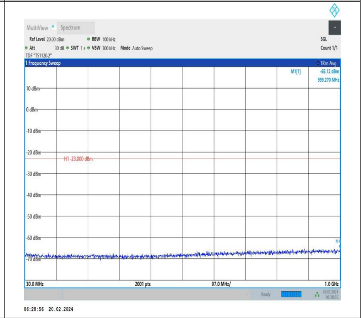
66-66-20MHz-5MHz-QPSK-QPSK-132522-132639-1RB#99-0 RB#0-30~1000MHz-PASS
