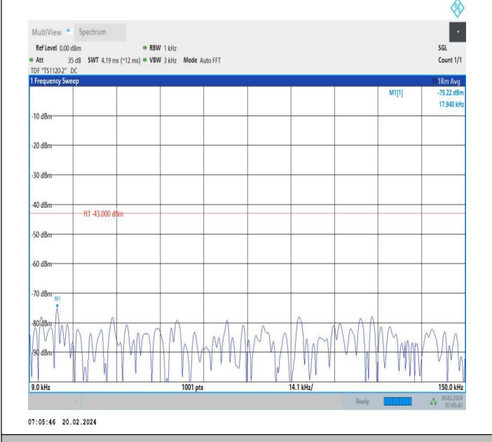
66-66-20MHz-10MHz-QPSK-QPSK-132473-132617-1RB#99-0 RB#0-0.009~0.15MHz-PASS
