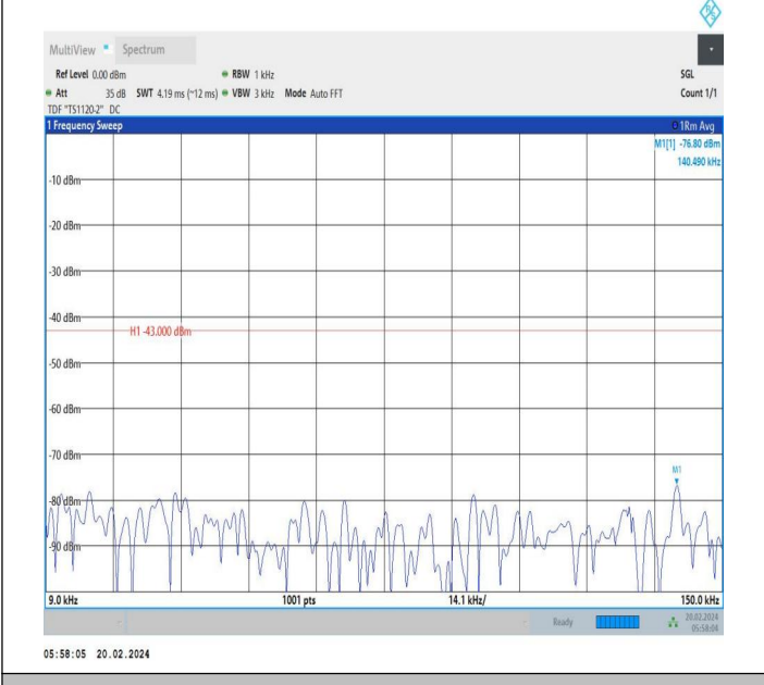
66-66-20MHz-5MHz-QPSK-QPSK-132072-132189-1RB#0-0R B#0-0.009~0.15MHz-PASS
