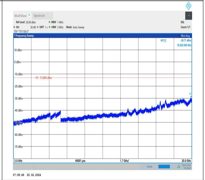
66-66-20MHz-10MHz-QPSK-QPSK-132473-132617-1RB#0-1 RB#49-3000~20000MHz-PASS
