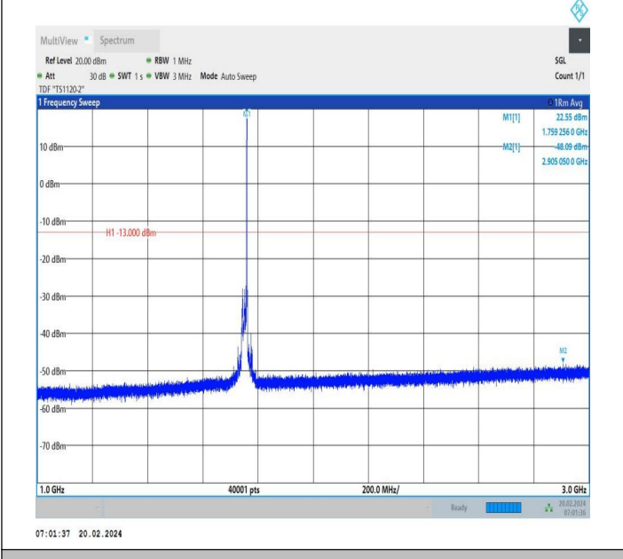
66-66-20MHz-10MHz-QPSK-QPSK-132373-132517-1RB#99-0 RB#0-1000~3000MHz-PASS
