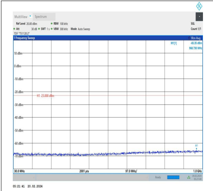
66-66-15MHz-20MHz-QPSK-QPSK-132325-132496-1RB#0-1 RB#99-30~1000MHz-PASS
