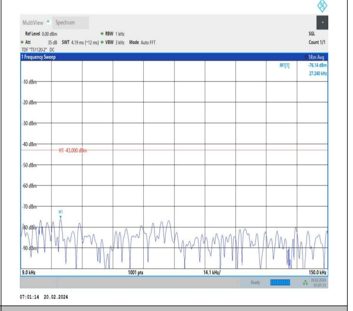
66-66-20MHz-10MHz-QPSK-QPSK-132373-132517-1RB#99-0 RB#0-0.009~0.15MHz-PASS
