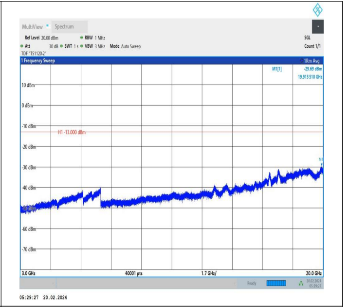
66-66-15MHz-20MHz-QPSK-QPSK-132401-132572-1RB#0-1 RB#99-3000~20000MHz-PASS
