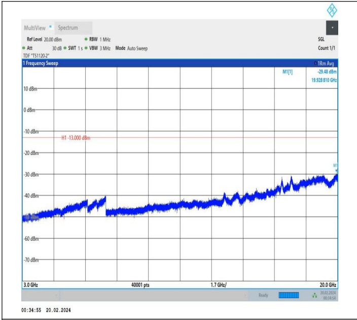
66-66-15MHz-10MHz-QPSK-QPSK-132373-132493-1RB#0-1 RB#49-3000~20000MHz-PASS
