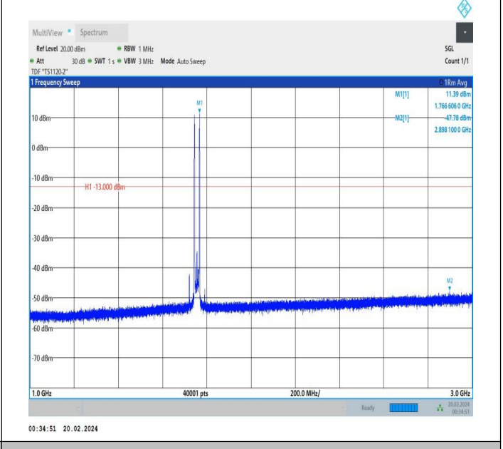
66-66-15MHz-10MHz-QPSK-QPSK-132373-132493-1RB#0-1 RB#49-1000~3000MHz-PASS
