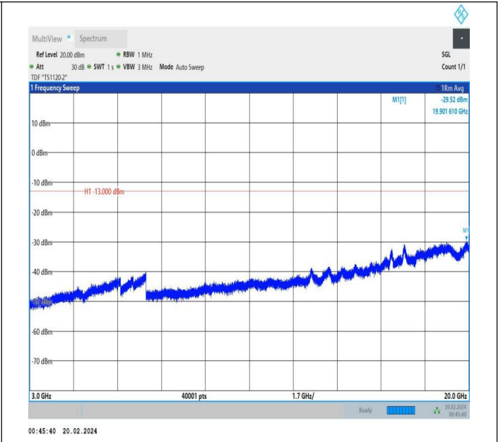
66-66-15MHz-10MHz-QPSK-QPSK-132499-132619-1RB#0-0 RB#0-3000~20000MHz-PASS
