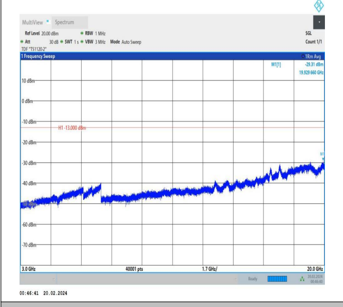
66-66-15MHz-10MHz-QPSK-QPSK-132499-132619-1RB#74-0 RB#0-3000~20000MHz-PASS
