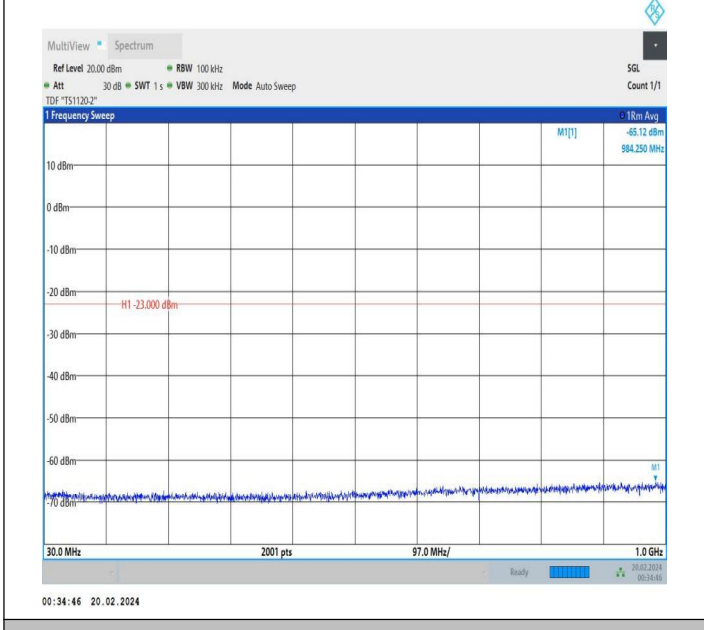
66-66-15MHz-10MHz-QPSK-QPSK-132373-132493-1RB#0-1 RB#49-30~1000MHz-PASS
