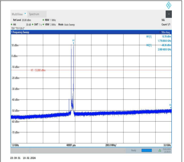
66-66-10MHz-20MHz-QPSK-QPSK-132428-132572-1RB#0-1 RB#99-1000~3000MHz-PASS
