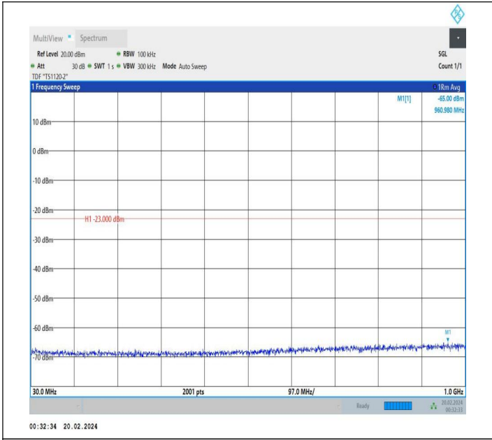
66-66-15MHz-10MHz-QPSK-QPSK-132373-132493-1RB#0-0 RB#0-30~1000MHz-PASS
