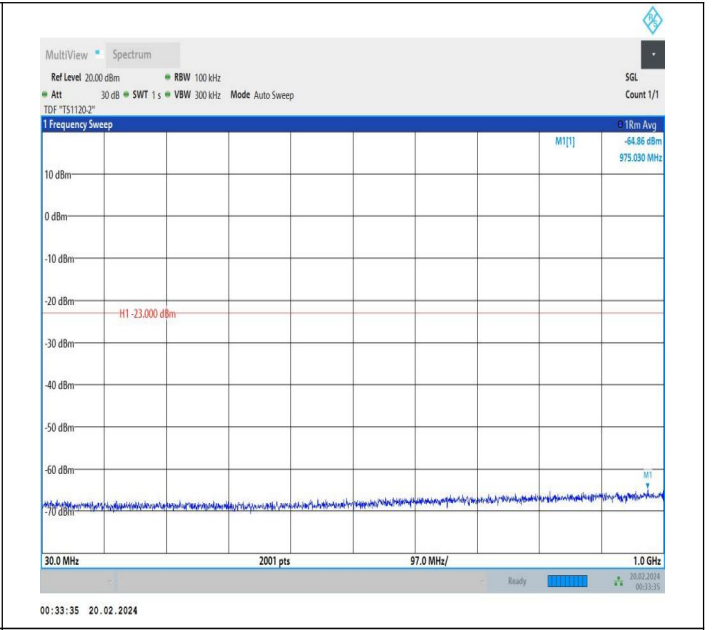
66-66-15MHz-10MHz-QPSK-QPSK-132373-132493-1RB#74-0 RB#0-30~1000MHz-PASS
