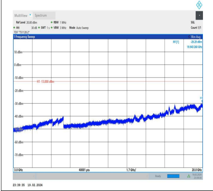
66-66-10MHz-20MHz-QPSK-QPSK-132428-132572-1RB#0-1 RB#99-3000~20000MHz-PASS
