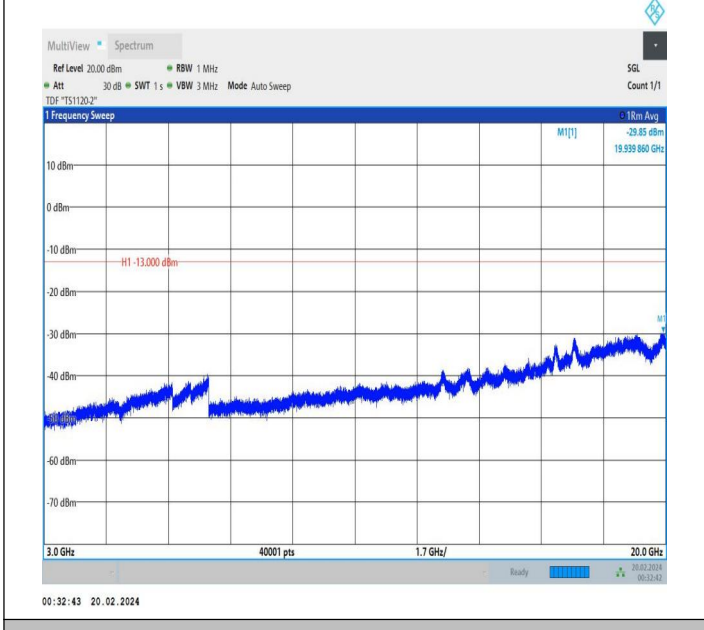
66-66-15MHz-10MHz-QPSK-QPSK-132373-132493-1RB#0-0 RB#0-3000~20000MHz-PASS
