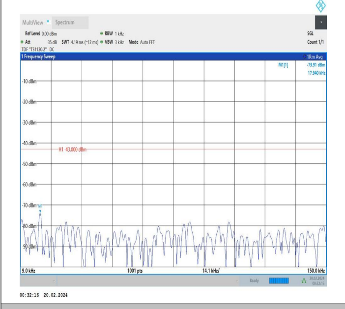
66-66-15MHz-10MHz-QPSK-QPSK-132373-132493-1RB#0-0 RB#0-0.009~0.15MHz-PASS
