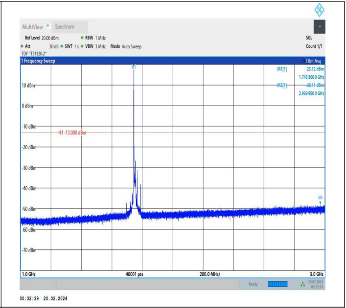
66-66-15MHz-10MHz-QPSK-QPSK-132373-132493-1RB#0-0 RB#0-1000~3000MHz-PASS
