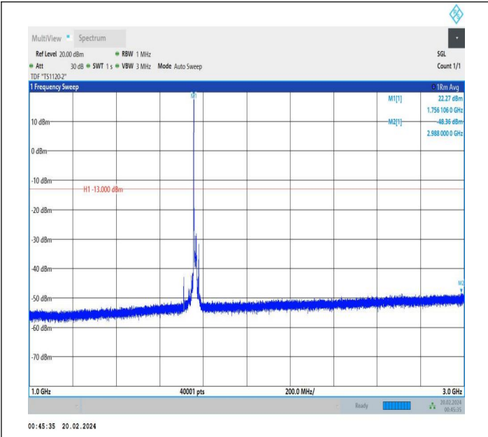
66-66-15MHz-10MHz-QPSK-QPSK-132499-132619-1RB#0-0 RB#0-1000~3000MHz-PASS
