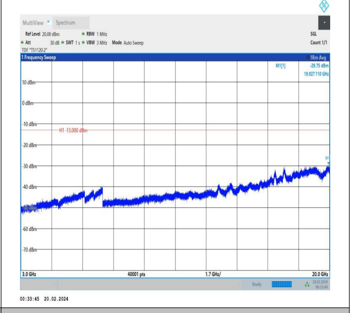
66-66-15MHz-10MHz-QPSK-QPSK-132373-132493-1RB#74-0 RB#0-3000~20000MHz-PASS
