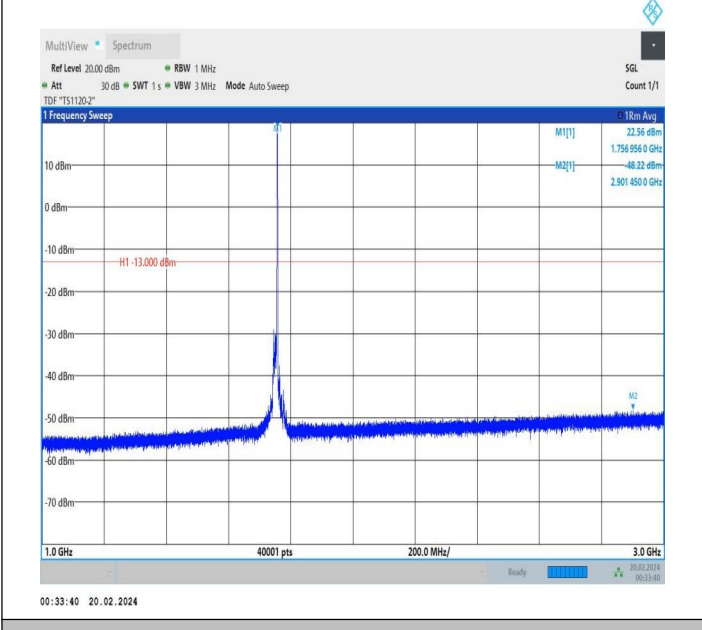
66-66-15MHz-10MHz-QPSK-QPSK-132373-132493-1RB#74-0 RB#0-1000~3000MHz-PASS
