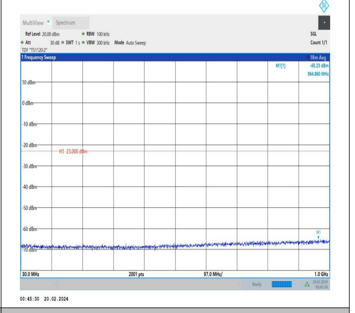
66-66-15MHz-10MHz-QPSK-QPSK-132499-132619-1RB#0-0 RB#0-30~1000MHz-PASS
