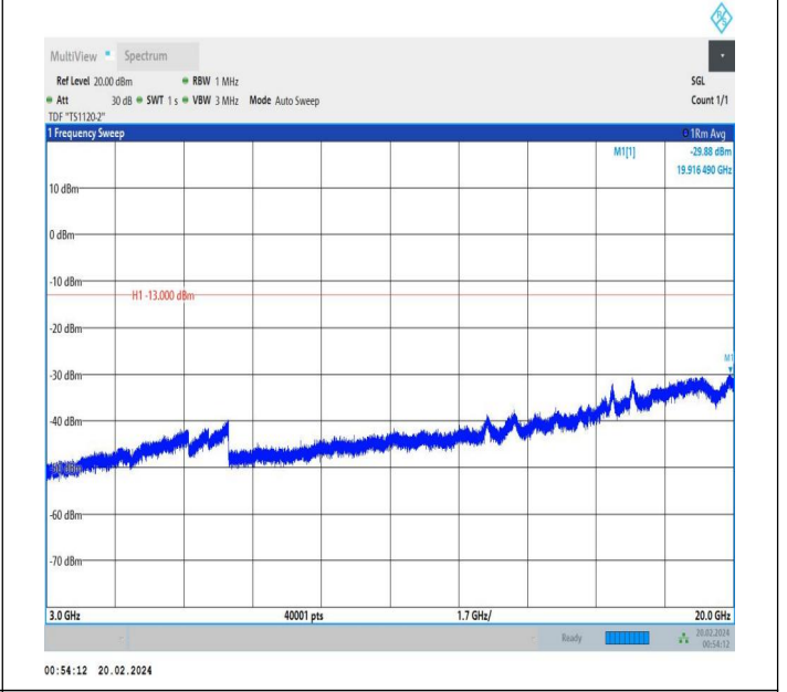
66-66-15MHz-10MHz-QPSK-QPSK-132499-132619-1RB#0-1 RB#49-3000~20000MHz-PASS
