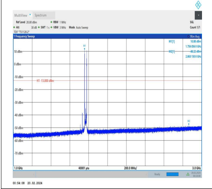
66-66-15MHz-10MHz-QPSK-QPSK-132499-132619-1RB#0-1 RB#49-1000~3000MHz-PASS
