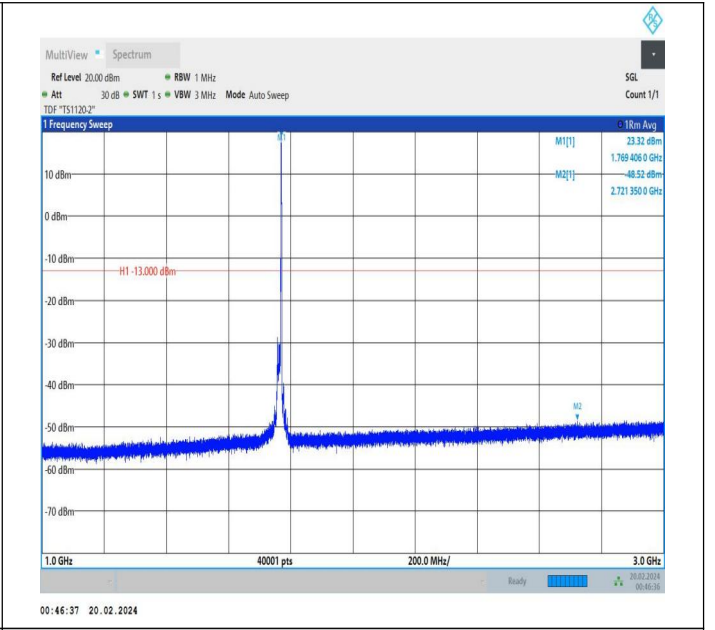
66-66-15MHz-10MHz-QPSK-QPSK-132499-132619-1RB#74-0 RB#0-1000~3000MHz-PASS
