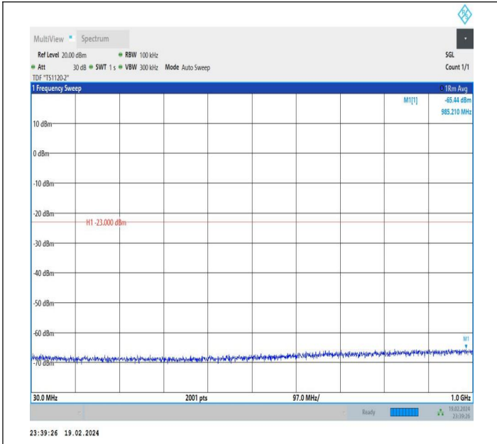
66-66-10MHz-20MHz-QPSK-QPSK-132428-132572-1RB#0-1 RB#99-30~1000MHz-PASS
