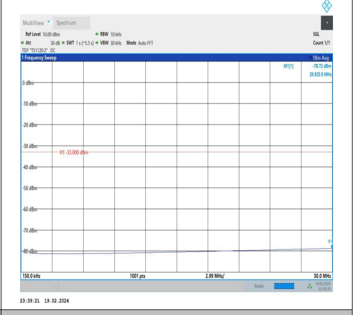
66-66-10MHz-20MHz-QPSK-QPSK-132428-132572-1RB#0-1 RB#99-0.15~30MHz-PASS
