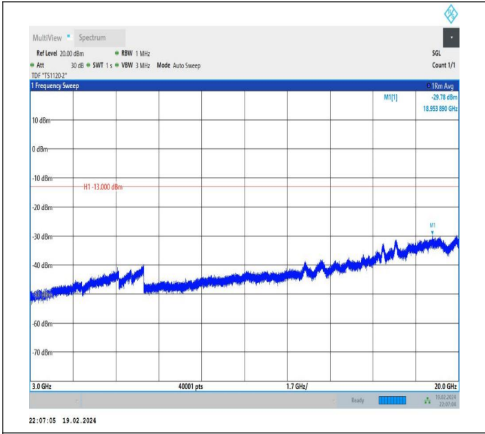
66-66-10MHz-15MHz-QPSK-QPSK-132351-132471-1RB#0-0 RB#0-3000~20000MHz-PASS
