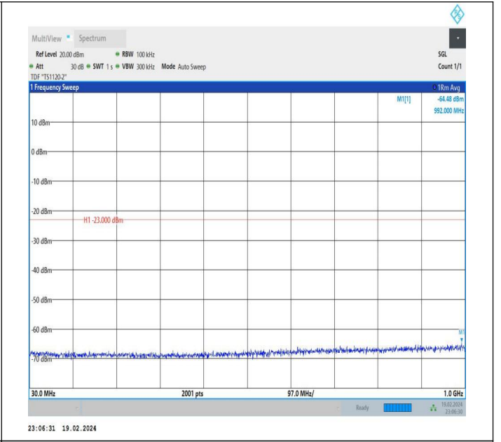
66-66-10MHz-20MHz-QPSK-QPSK-132027-132171-1RB#49-0 RB#0-30~1000MHz-PASS
