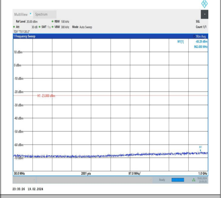
66-66-10MHz-20MHz-QPSK-QPSK-132428-132572-1RB#49-0 RB#0-30~1000MHz-PASS
