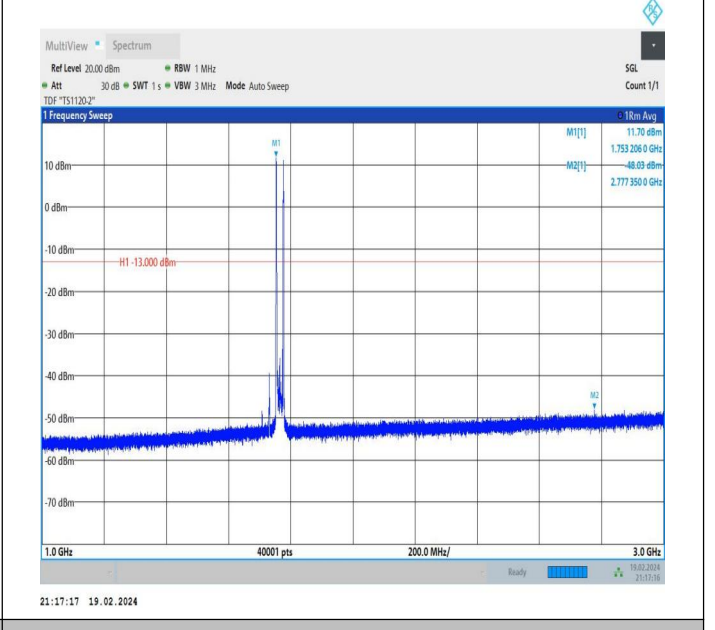
66-66-5MHz-20MHz-QPSK-QPSK-132428-132572-1RB#0-1R B#99-1000~3000MHz-PASS
