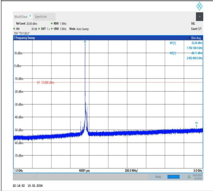
66-66-10MHz-15MHz-QPSK-QPSK-132477-132597-1RB#0-0 RB#0-1000~3000MHz-PASS
