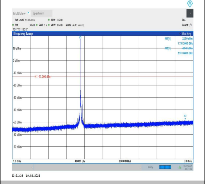
66-66-10MHz-20MHz-QPSK-QPSK-132428-132572-1RB#0-0 RB#0-1000~3000MHz-PASS
