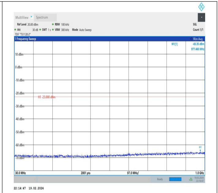
66-66-10MHz-15MHz-QPSK-QPSK-132477-132597-1RB#0-0 RB#0-30~1000MHz-PASS
