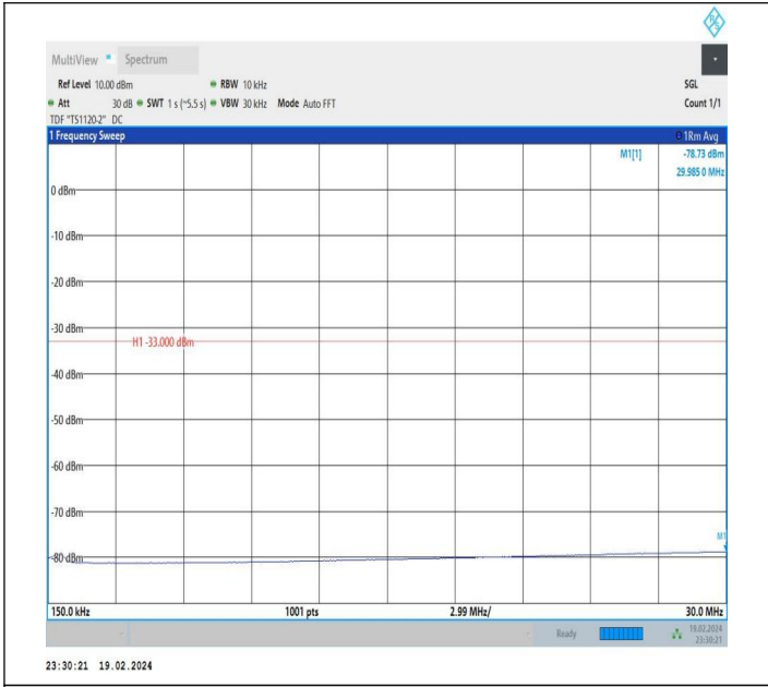
66-66-10MHz-20MHz-QPSK-QPSK-132328-132472-1RB#0-1 RB#99-0.15~30MHz-PASS
