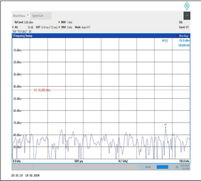
66-66-10MHz-20MHz-QPSK-QPSK-132428-132572-1RB#0-0 RB#0-0.009~0.15MHz-PASS
