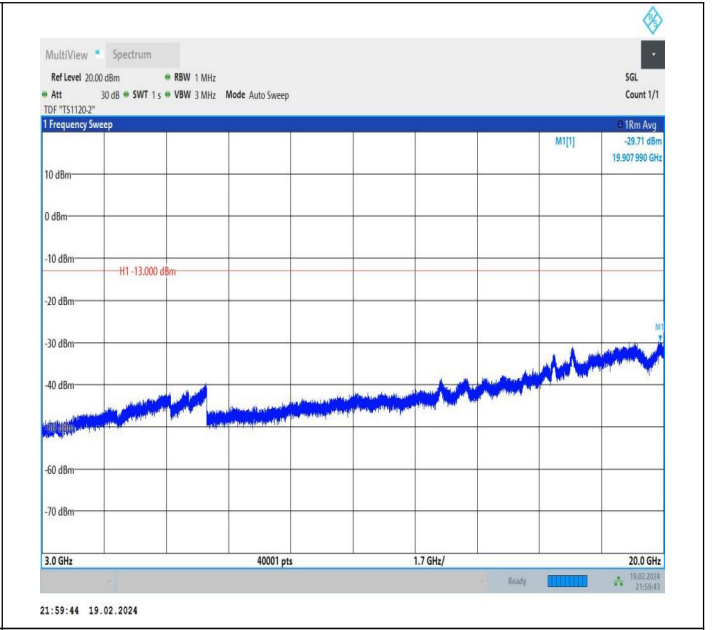
66-66-10MHz-15MHz-QPSK-QPSK-132025-132145-1RB#0-0 RB#0-3000~20000MHz-PASS
