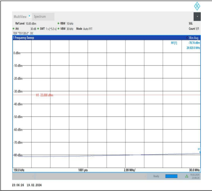
66-66-10MHz-20MHz-QPSK-QPSK-132027-132171-1RB#49-0 RB#0-0.15~30MHz-PASS
