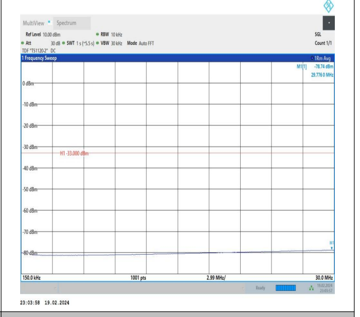
66-66-10MHz-20MHz-QPSK-QPSK-132027-132171-1RB#0-0 RB#0-0.15~30MHz-PASS
