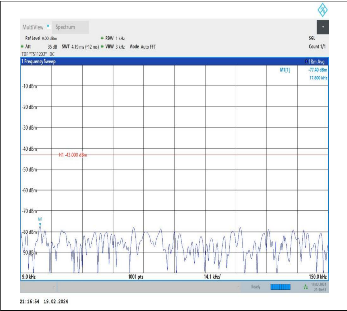
66-66-5MHz-20MHz-QPSK-QPSK-132428-132572-1RB#0-1R B#99-0.009~0.15MHz-PASS
