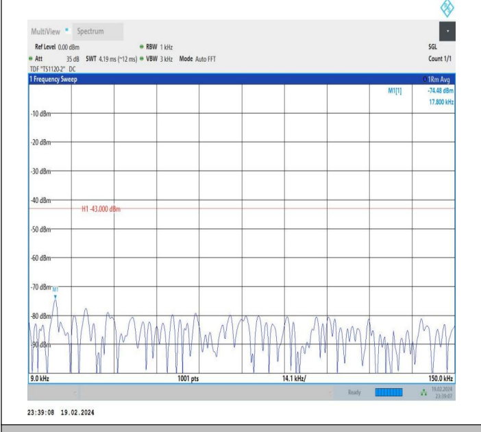
66-66-10MHz-20MHz-QPSK-QPSK-132428-132572-1RB#0-1 RB#99-0.009~0.15MHz-PASS
