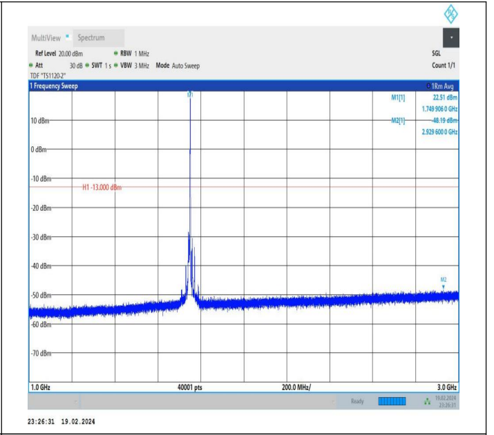
66-66-10MHz-20MHz-QPSK-QPSK-132328-132472-1RB#49-0 RB#0-1000~3000MHz-PASS
