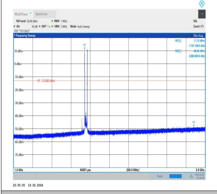
66-66-10MHz-20MHz-QPSK-QPSK-132328-132472-1RB#0-1 RB#99-1000~3000MHz-PASS
