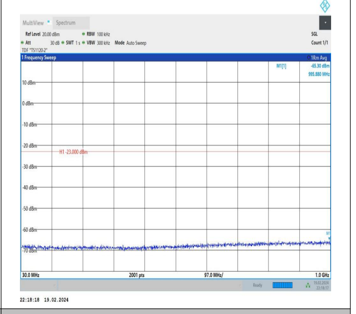
66-66-10MHz-15MHz-QPSK-QPSK-132477-132597-1RB#0-1 RB#74-30~1000MHz-PASS
