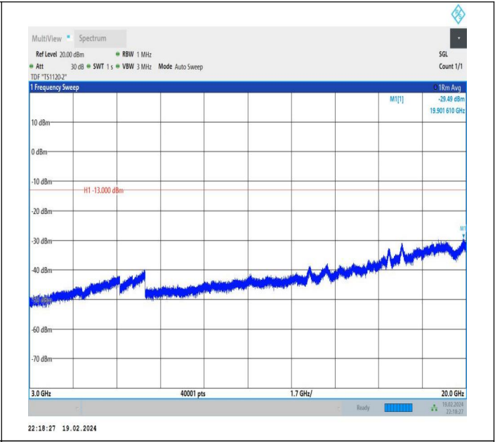
66-66-10MHz-15MHz-QPSK-QPSK-132477-132597-1RB#0-1 RB#74-3000~20000MHz-PASS
