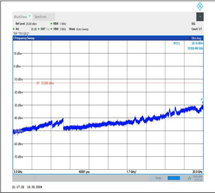
66-66-5MHz-20MHz-QPSK-QPSK-132428-132572-1RB#0-1R B#99-3000~20000MHz-PASS
