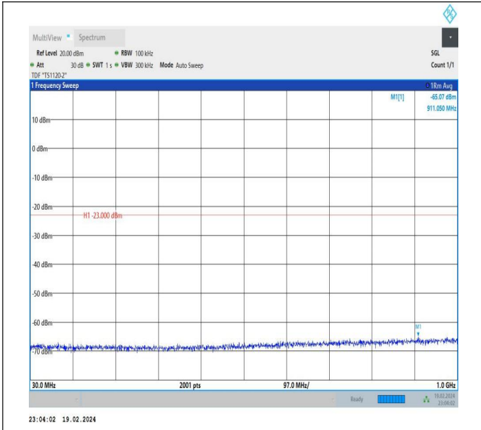
66-66-10MHz-20MHz-QPSK-QPSK-132027-132171-1RB#0-0 RB#0-30~1000MHz-PASS
