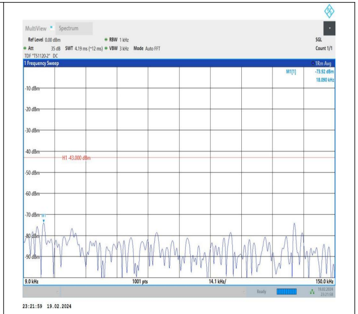
66-66-10MHz-20MHz-QPSK-QPSK-132328-132472-1RB#0-0 RB#0-0.009~0.15MHz-PASS
