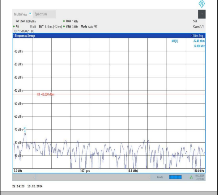
66-66-10MHz-15MHz-QPSK-QPSK-132477-132597-1RB#0-0 RB#0-0.009~0.15MHz-PASS
