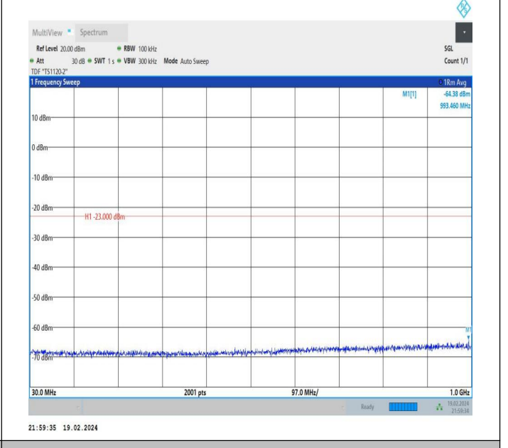
66-66-10MHz-15MHz-QPSK-QPSK-132025-132145-1RB#0-0 RB#0-30~1000MHz-PASS
