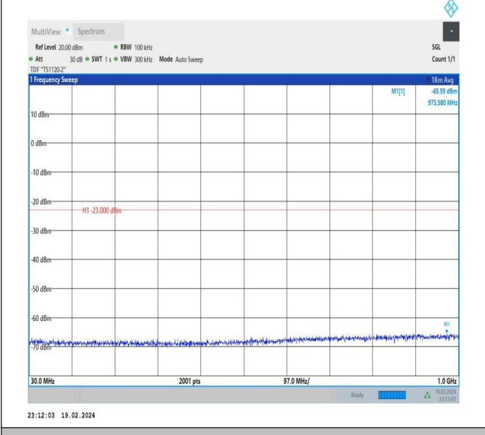
66-66-10MHz-20MHz-QPSK-QPSK-132027-132171-1RB#0-1 RB#99-30~1000MHz-PASS
