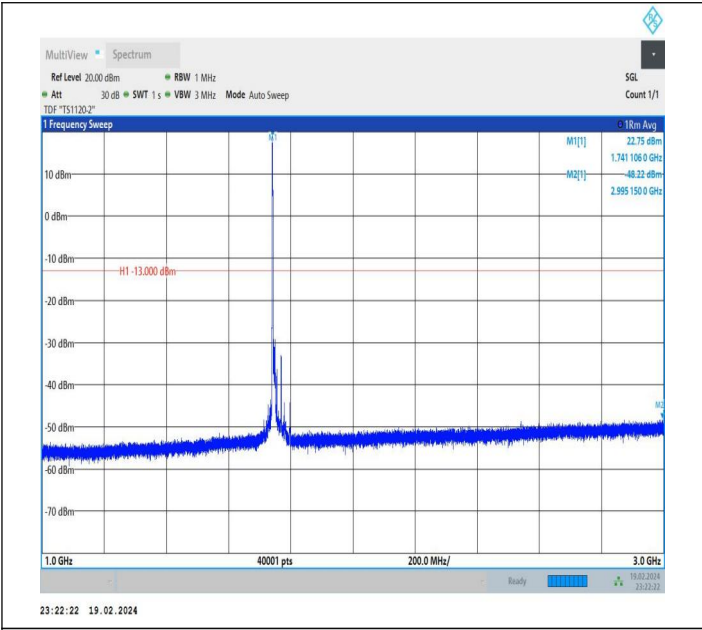
66-66-10MHz-20MHz-QPSK-QPSK-132328-132472-1RB#0-0 RB#0-1000~3000MHz-PASS
