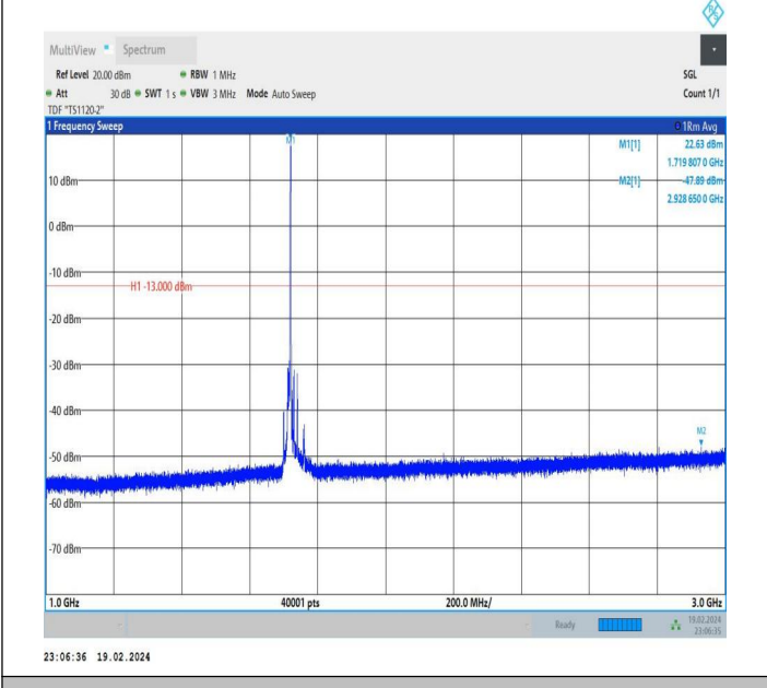
66-66-10MHz-20MHz-QPSK-QPSK-132027-132171-1RB#49-0 RB#0-1000~3000MHz-PASS
