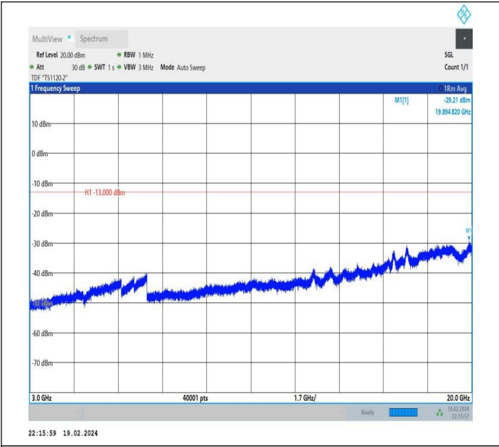
66-66-10MHz-15MHz-QPSK-QPSK-132477-132597-1RB#49-0 RB#0-3000~20000MHz-PASS
