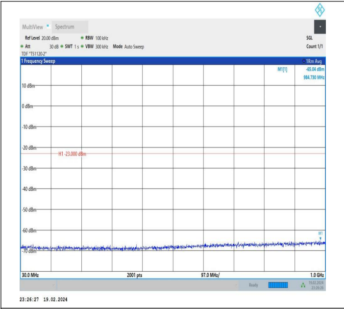
66-66-10MHz-20MHz-QPSK-QPSK-132328-132472-1RB#49-0 RB#0-30~1000MHz-PASS
