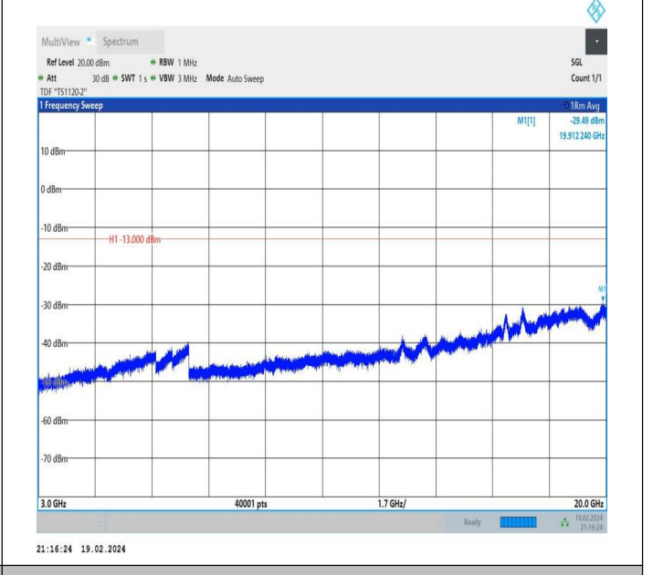
66-66-5MHz-20MHz-QPSK-QPSK-132428-132572-1RB#24-0 RB#0-3000~20000MHz-PASS
