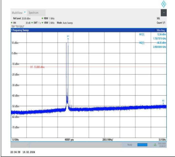
66-66-10MHz-15MHz-QPSK-QPSK-132025-132145-1RB#0-1 RB#74-1000~3000MHz-PASS
