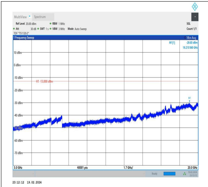
66-66-10MHz-20MHz-QPSK-QPSK-132027-132171-1RB#0-1 RB#99-3000~20000MHz-PASS
