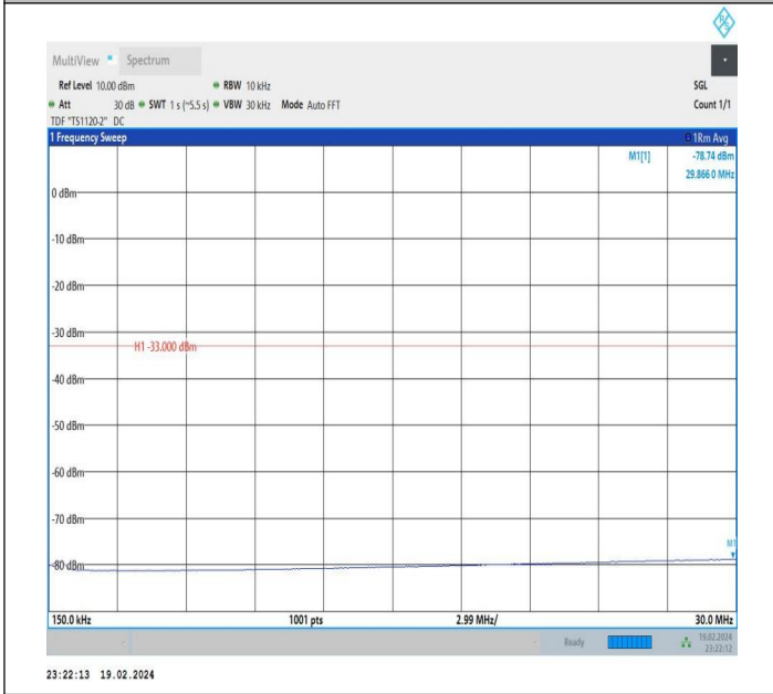
66-66-10MHz-20MHz-QPSK-QPSK-132328-132472-1RB#0-0 RB#0-0.15~30MHz-PASS
