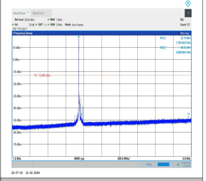
66-66-10MHz-15MHz-QPSK-QPSK-132351-132471-1RB#0-0 RB#0-1000~3000MHz-PASS
