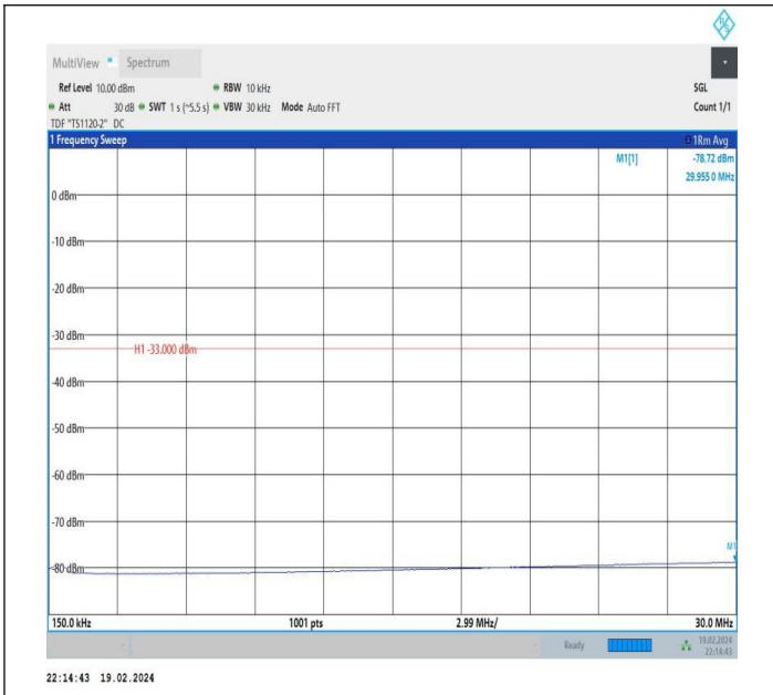
66-66-10MHz-15MHz-QPSK-QPSK-132477-132597-1RB#0-0 RB#0-0.15~30MHz-PASS
