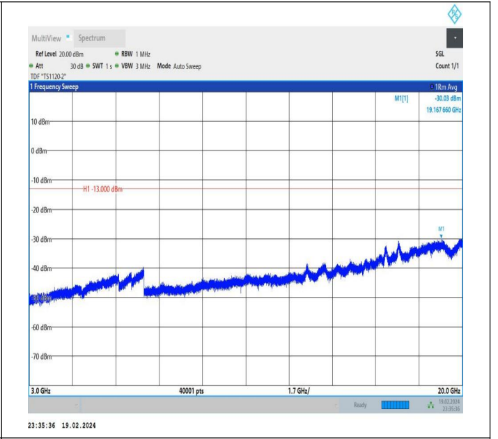
66-66-10MHz-20MHz-QPSK-QPSK-132428-132572-1RB#49-0 RB#0-3000~20000MHz-PASS
