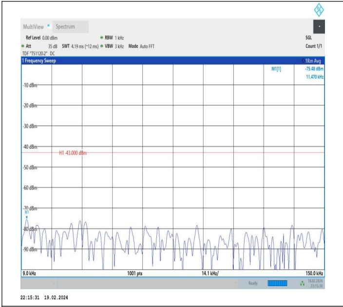
66-66-10MHz-15MHz-QPSK-QPSK-132477-132597-1RB#49-0 RB#0-0.009~0.15MHz-PASS
