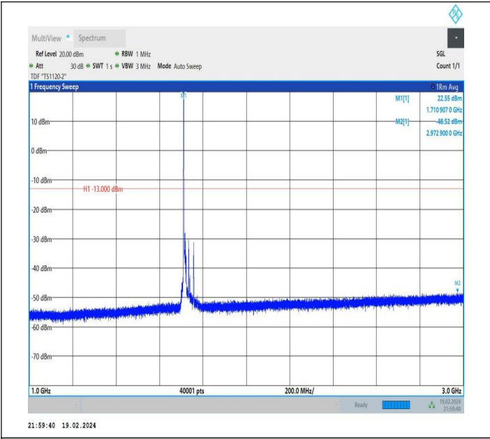
66-66-10MHz-15MHz-QPSK-QPSK-132025-132145-1RB#0-0 RB#0-1000~3000MHz-PASS
