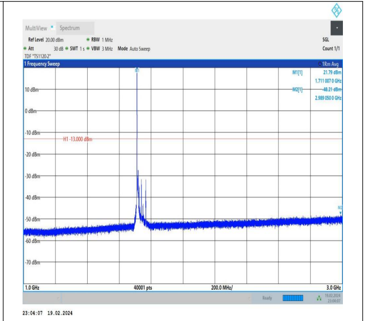
66-66-10MHz-20MHz-QPSK-QPSK-132027-132171-1RB#0-0 RB#0-1000~3000MHz-PASS
