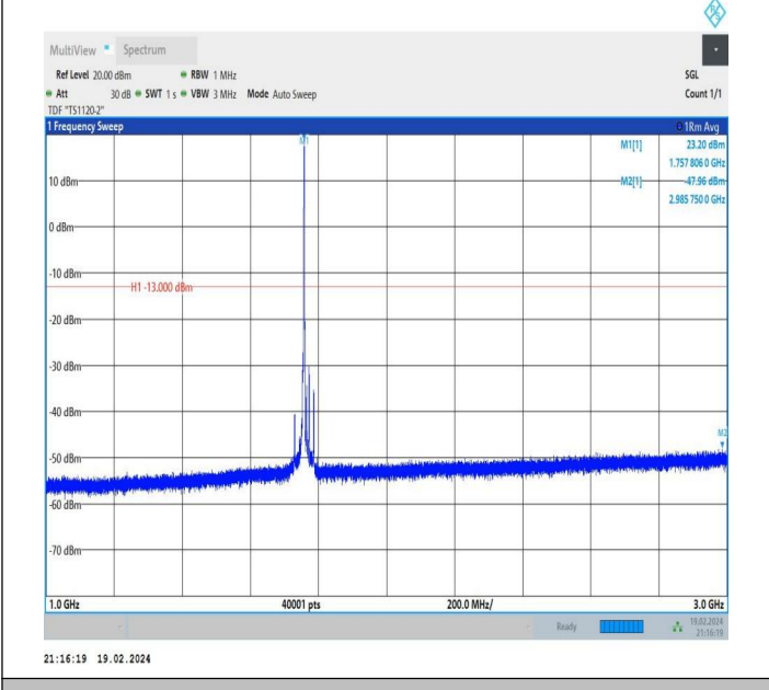
66-66-5MHz-20MHz-QPSK-QPSK-132428-132572-1RB#24-0 RB#0-1000~3000MHz-PASS
