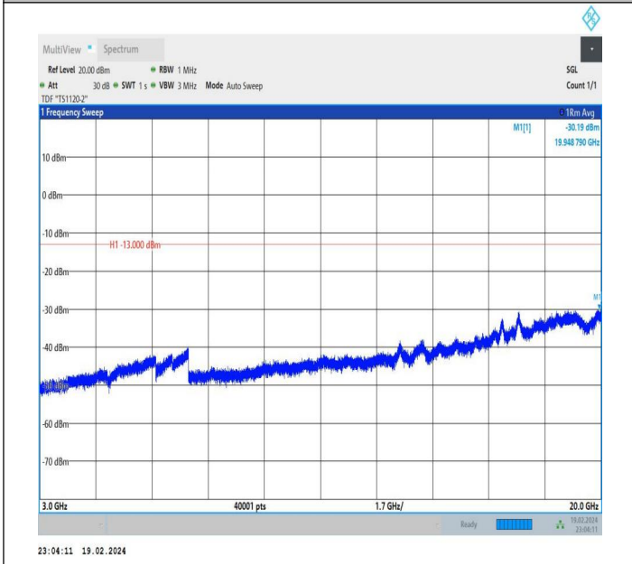
66-66-10MHz-20MHz-QPSK-QPSK-132027-132171-1RB#0-0 RB#0-3000~20000MHz-PASS
