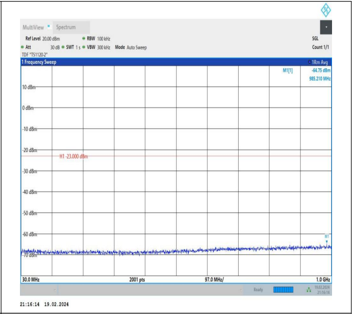
66-66-5MHz-20MHz-QPSK-QPSK-132428-132572-1RB#24-0 RB#0-30~1000MHz-PASS
