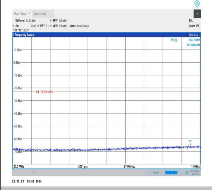
66-66-10MHz-20MHz-QPSK-QPSK-132428-132572-1RB#0-0 RB#0-30~1000MHz-PASS
