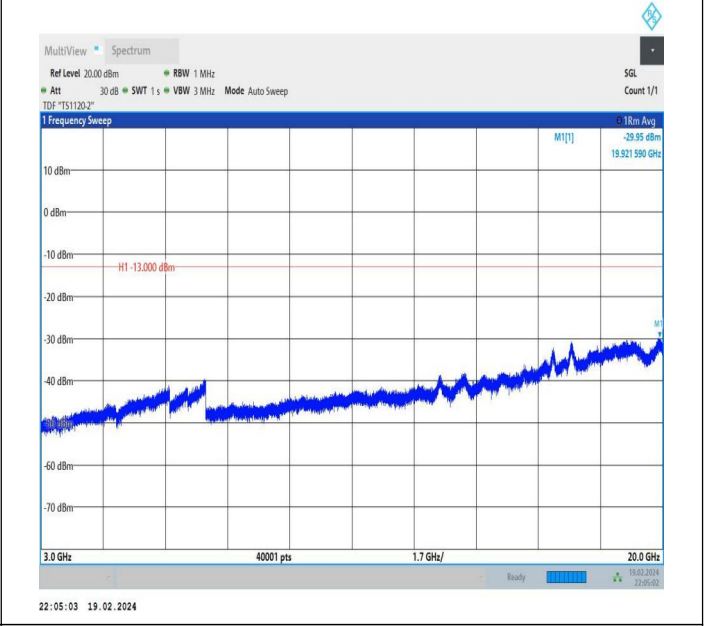
66-66-10MHz-15MHz-QPSK-QPSK-132025-132145-1RB#0-1 RB#74-3000~20000MHz-PASS
