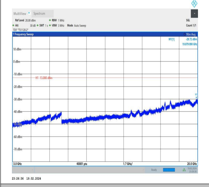
66-66-10MHz-20MHz-QPSK-QPSK-132328-132472-1RB#49-0 RB#0-3000~20000MHz-PASS
