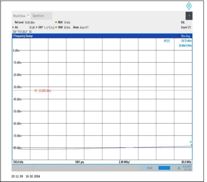
66-66-10MHz-20MHz-QPSK-QPSK-132027-132171-1RB#0-1 RB#99-0.15~30MHz-PASS
