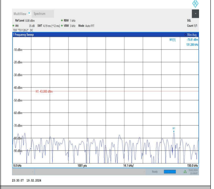
66-66-10MHz-20MHz-QPSK-QPSK-132328-132472-1RB#0-1 RB#99-0.009~0.15MHz-PASS
