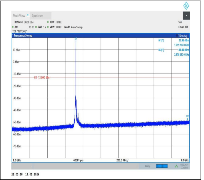
66-66-10MHz-15MHz-QPSK-QPSK-132025-132145-1RB#49-0 RB#0-1000~3000MHz-PASS
