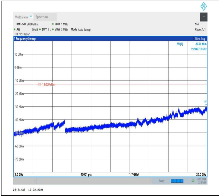
66-66-10MHz-20MHz-QPSK-QPSK-132428-132572-1RB#0-0 RB#0-3000~20000MHz-PASS
