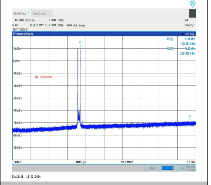
66-66-10MHz-20MHz-QPSK-QPSK-132027-132171-1RB#0-1 RB#99-1000~3000MHz-PASS
