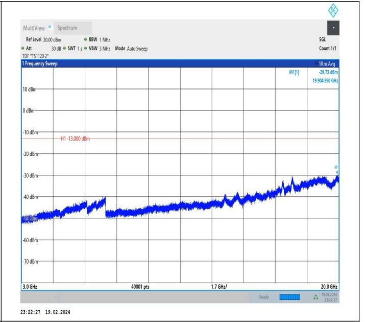
66-66-10MHz-20MHz-QPSK-QPSK-132328-132472-1RB#0-0 RB#0-3000~20000MHz-PASS
