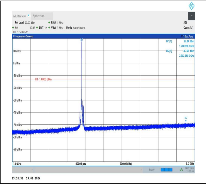
66-66-10MHz-20MHz-QPSK-QPSK-132428-132572-1RB#49-0 RB#0-1000~3000MHz-PASS
