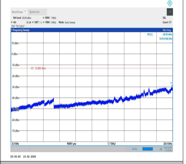
66-66-10MHz-20MHz-QPSK-QPSK-132027-132171-1RB#49-0 RB#0-3000~20000MHz-PASS
