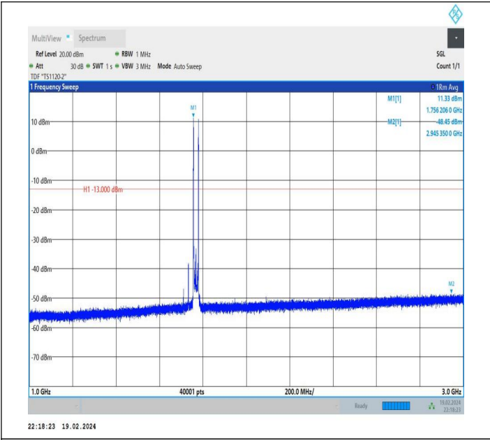
66-66-10MHz-15MHz-QPSK-QPSK-132477-132597-1RB#0-1 RB#74-1000~3000MHz-PASS
