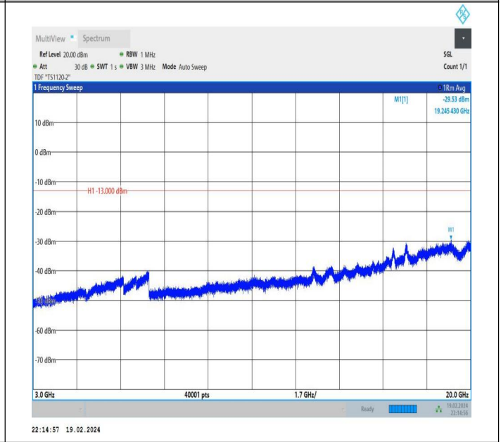
66-66-10MHz-15MHz-QPSK-QPSK-132477-132597-1RB#0-0 RB#0-3000~20000MHz-PASS
