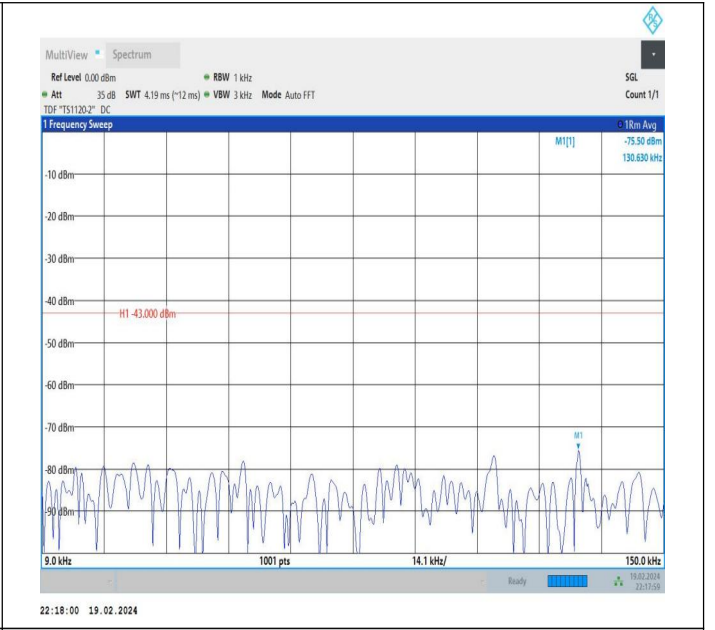
66-66-10MHz-15MHz-QPSK-QPSK-132477-132597-1RB#0-1 RB#74-0.009~0.15MHz-PASS
