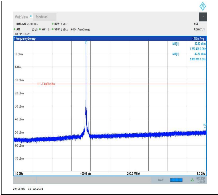
66-66-10MHz-15MHz-QPSK-QPSK-132351-132471-1RB#49-0 RB#0-1000~3000MHz-PASS
