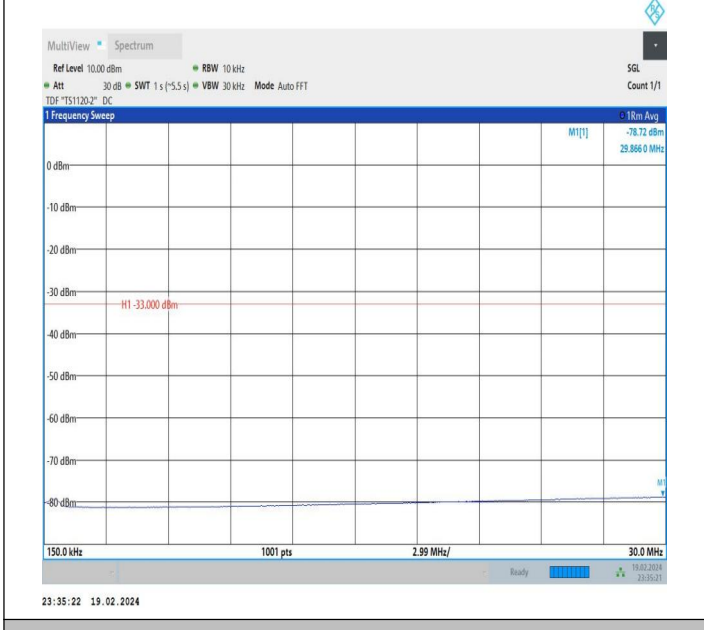
66-66-10MHz-20MHz-QPSK-QPSK-132428-132572-1RB#49-0 RB#0-0.15~30MHz-PASS
