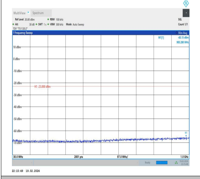
66-66-10MHz-15MHz-QPSK-QPSK-132477-132597-1RB#49-0 RB#0-30~1000MHz-PASS
