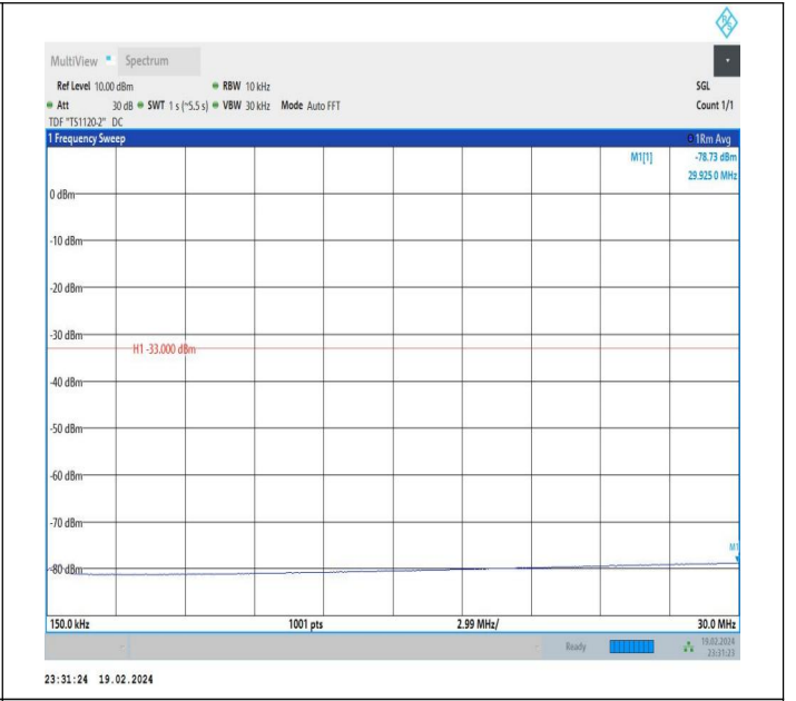
66-66-10MHz-20MHz-QPSK-QPSK-132428-132572-1RB#0-0 RB#0-0.15~30MHz-PASS
