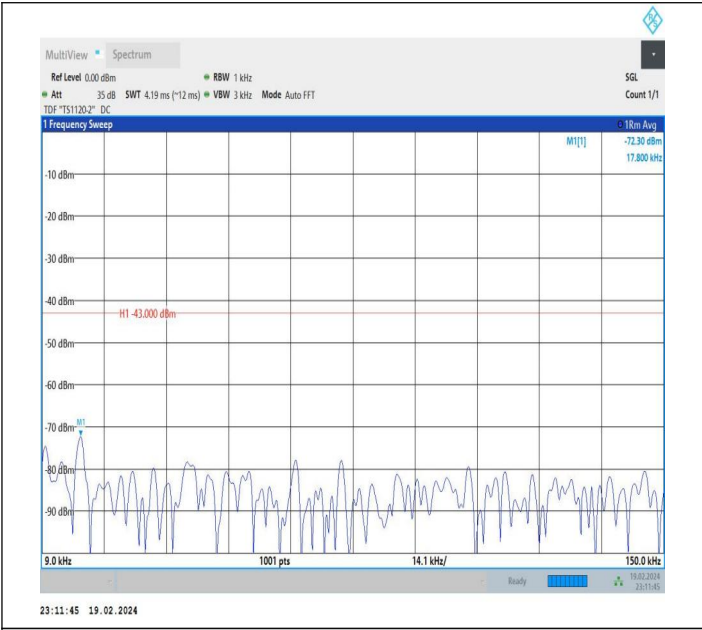
66-66-10MHz-20MHz-QPSK-QPSK-132027-132171-1RB#0-1 RB#99-0.009~0.15MHz-PASS
