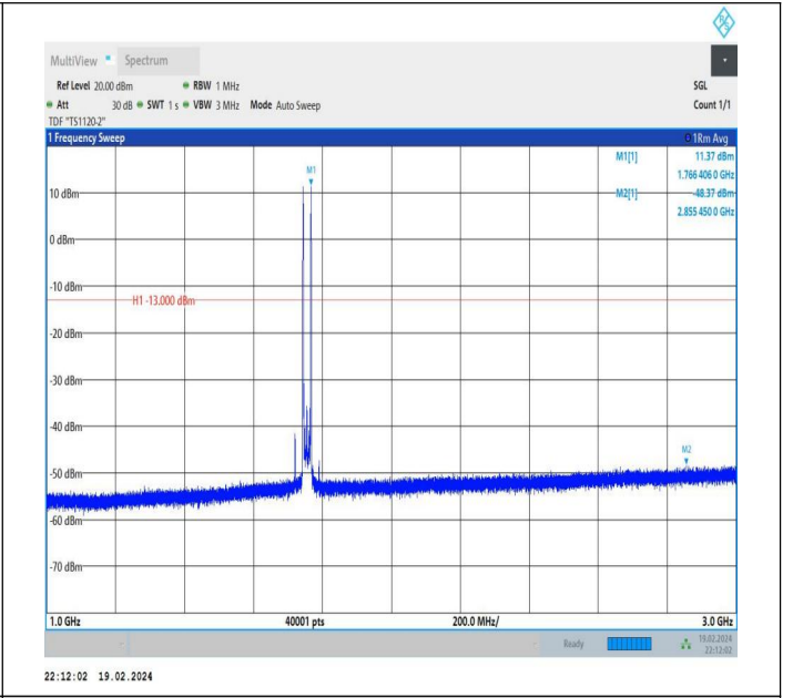
66-66-10MHz-15MHz-QPSK-QPSK-132351-132471-1RB#0-1 RB#74-1000~3000MHz-PASS
