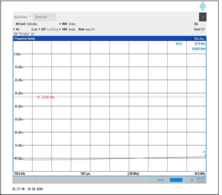
66-66-5MHz-20MHz-QPSK-QPSK-132428-132572-1RB#0-1R B#99-0.15~30MHz-PASS
