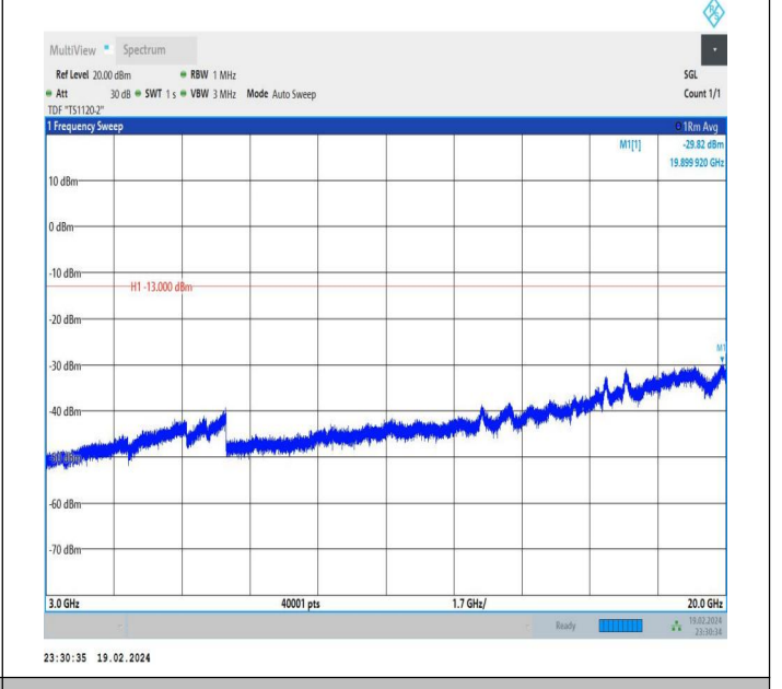
66-66-10MHz-20MHz-QPSK-QPSK-132328-132472-1RB#0-1 RB#99-3000~20000MHz-PASS
