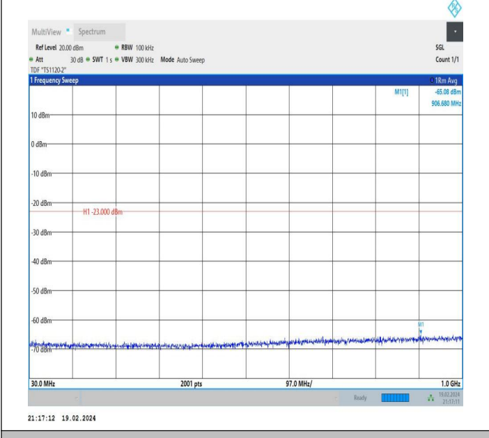
66-66-5MHz-20MHz-QPSK-QPSK-132428-132572-1RB#0-1R B#99-30~1000MHz-PASS
