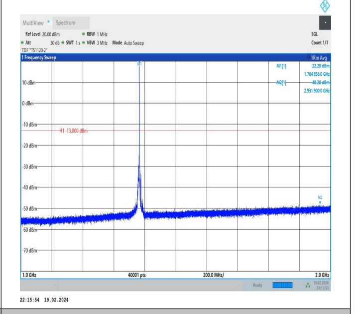
66-66-10MHz-15MHz-QPSK-QPSK-132477-132597-1RB#49-0 RB#0-1000~3000MHz-PASS
