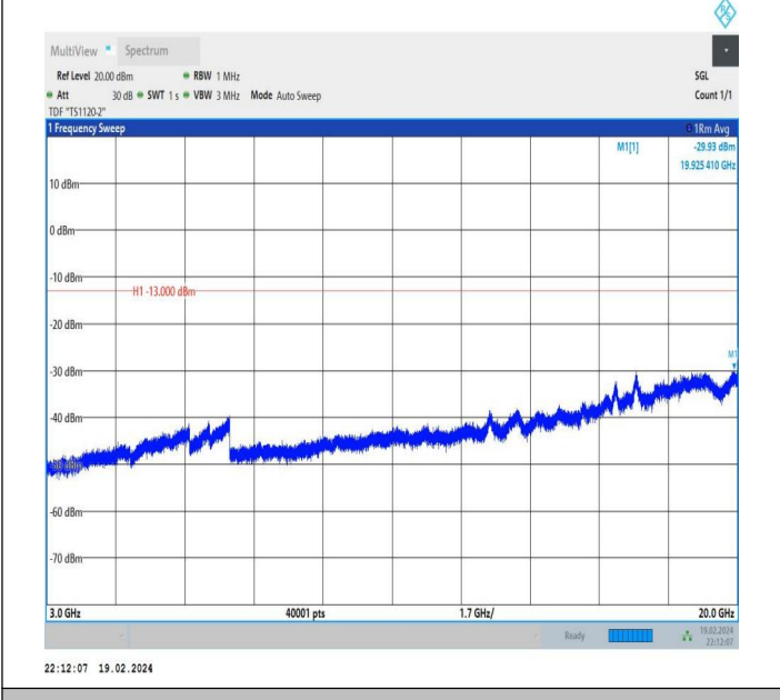
66-66-10MHz-15MHz-QPSK-QPSK-132351-132471-1RB#0-1 RB#74-3000~20000MHz-PASS
