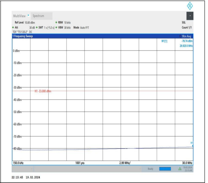
66-66-10MHz-15MHz-QPSK-QPSK-132477-132597-1RB#49-0 RB#0-0.15~30MHz-PASS
