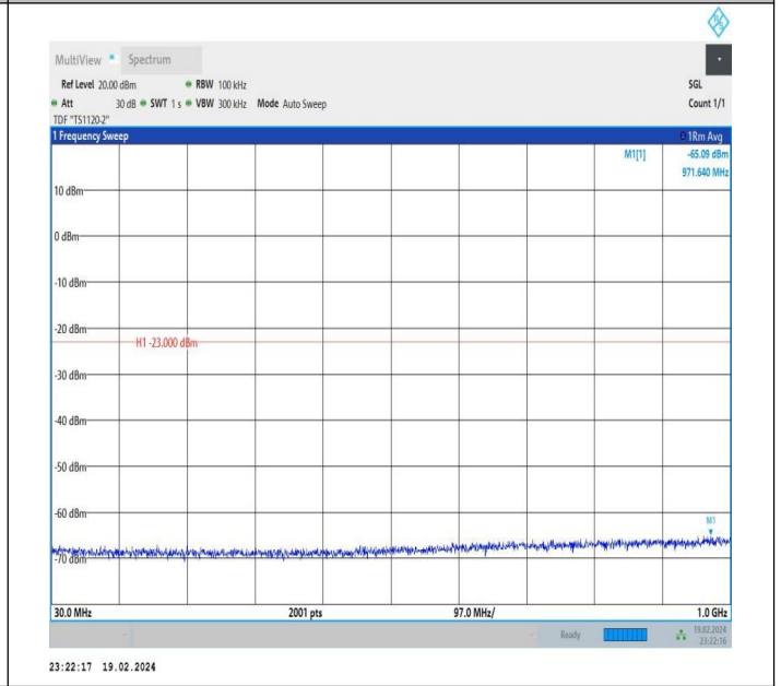
66-66-10MHz-20MHz-QPSK-QPSK-132328-132472-1RB#0-0 RB#0-30~1000MHz-PASS
