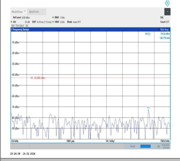
66-66-10MHz-20MHz-QPSK-QPSK-132328-132472-1RB#49-0 RB#0-0.009~0.15MHz-PASS
