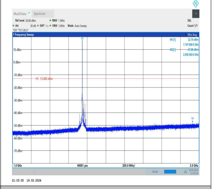
66-66-5MHz-20MHz-QPSK-QPSK-132328-132472-1RB#24-0 RB#0-1000~3000MHz-PASS
