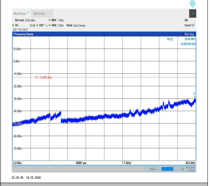
66-66-5MHz-20MHz-QPSK-QPSK-132328-132472-1RB#0-0R B#0-3000~20000MHz-PASS
