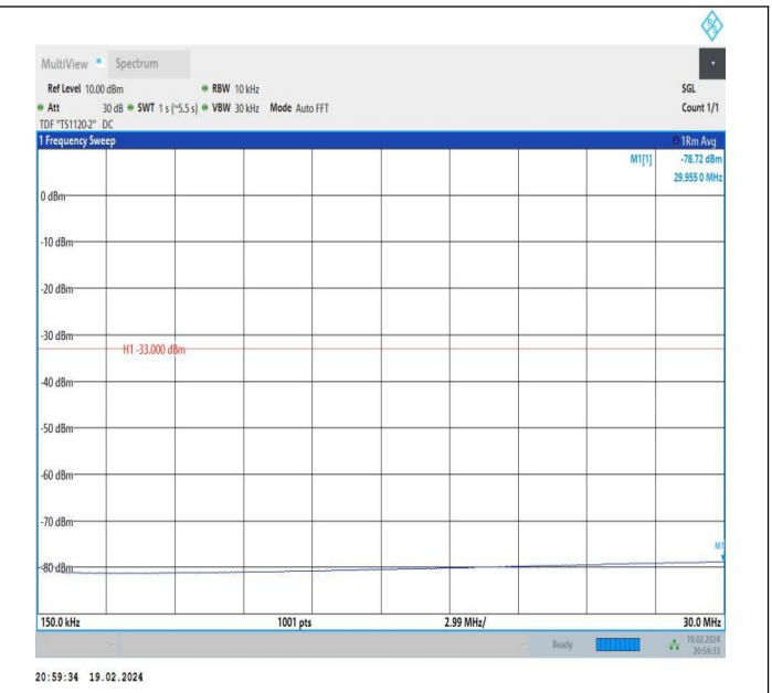
66-66-5MHz-20MHz-QPSK-QPSK-132027-132171-1RB#0-0R B#0-0.15~30MHz-PASS
