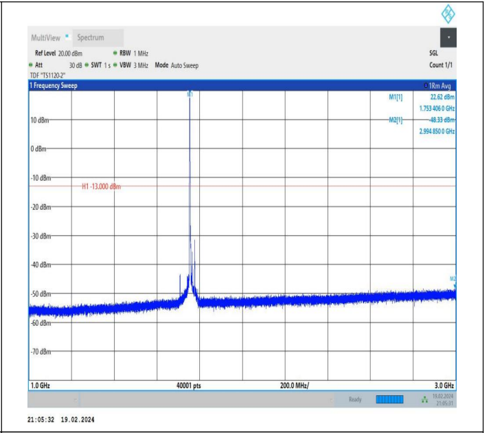
66-66-5MHz-20MHz-QPSK-QPSK-132428-132572-1RB#0-0R B#0-1000~3000MHz-PASS
