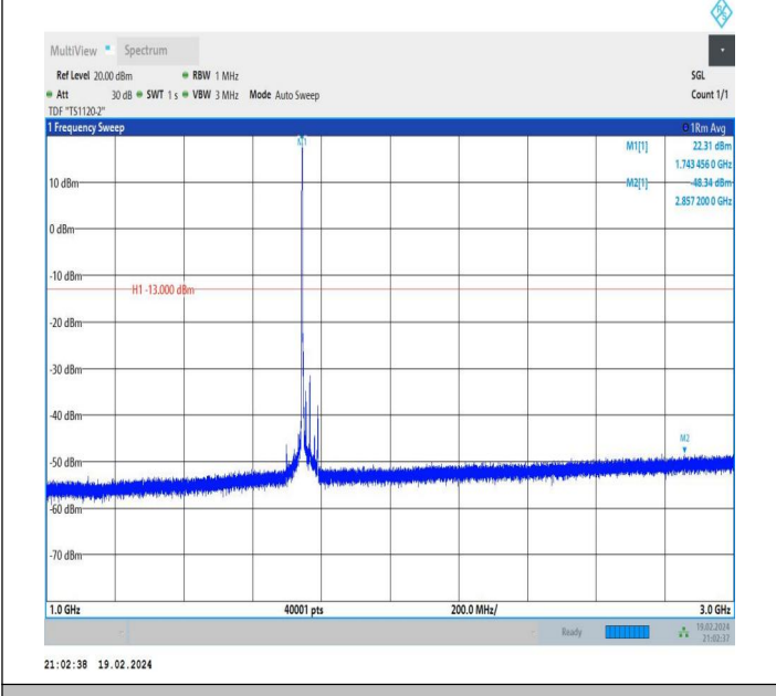
66-66-5MHz-20MHz-QPSK-QPSK-132328-132472-1RB#0-0R B#0-1000~3000MHz-PASS
