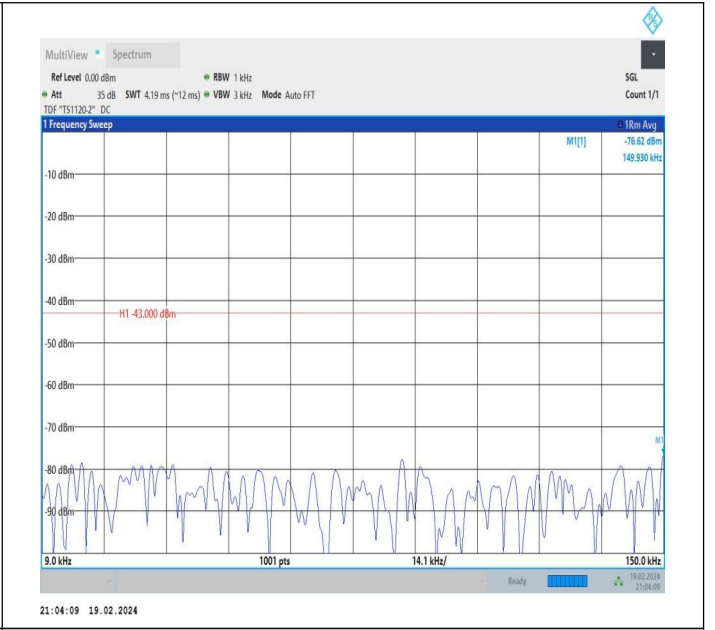
66-66-5MHz-20MHz-QPSK-QPSK-132328-132472-1RB#0-1R B#99-0.009~0.15MHz-PASS
