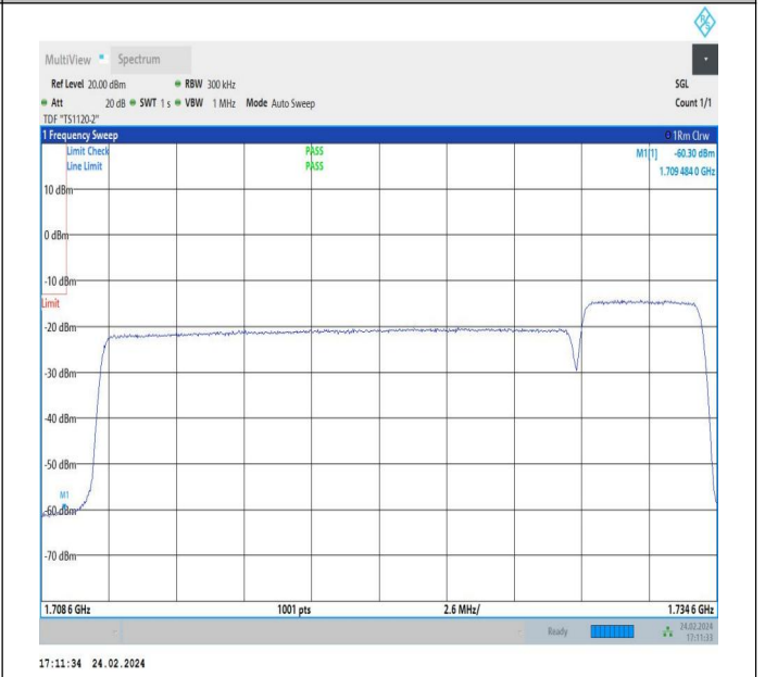
20MHz-5MHz_QPSK@QPSK-QPSK@QPSK_132072-132189_9_100RB#0@100RB#0-25RB#0@25RB#0
