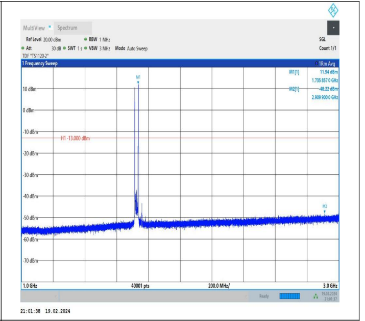
66-66-5MHz-20MHz-QPSK-QPSK-132027-132171-1RB#0-1R B#99-1000~3000MHz-PASS
