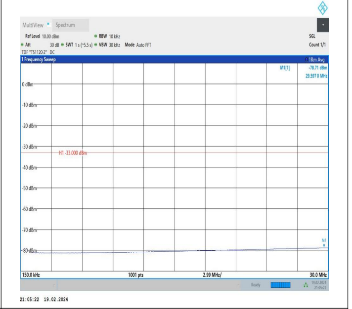
66-66-5MHz-20MHz-QPSK-QPSK-132428-132572-1RB#0-0R B#0-0.15~30MHz-PASS
