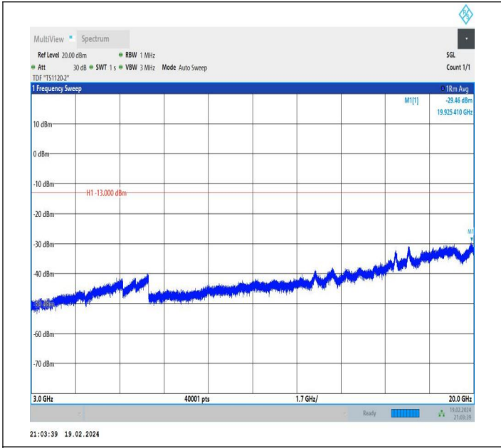
66-66-5MHz-20MHz-QPSK-QPSK-132328-132472-1RB#24-0 RB#0-3000~20000MHz-PASS
