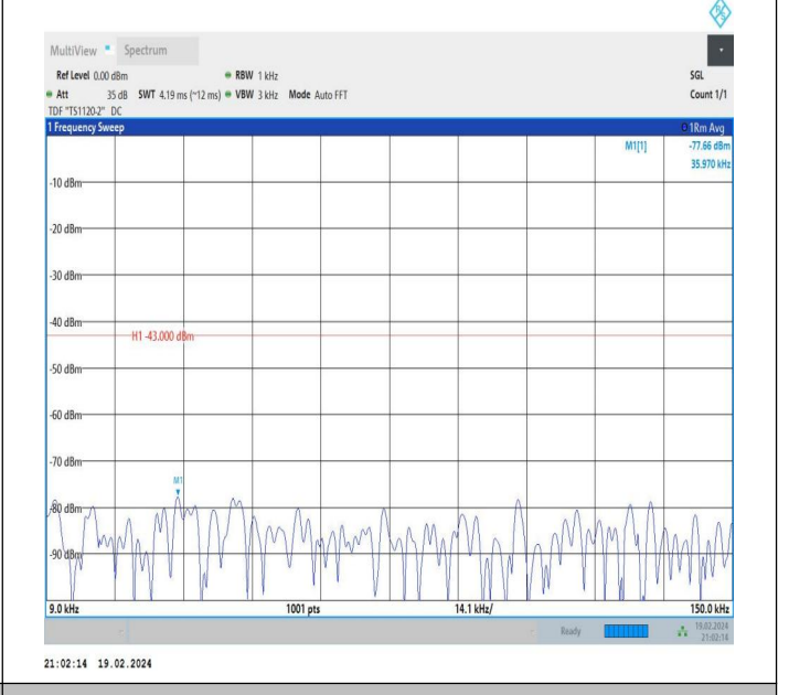
66-66-5MHz-20MHz-QPSK-QPSK-132328-132472-1RB#0-0R B#0-0.009~0.15MHz-PASS
