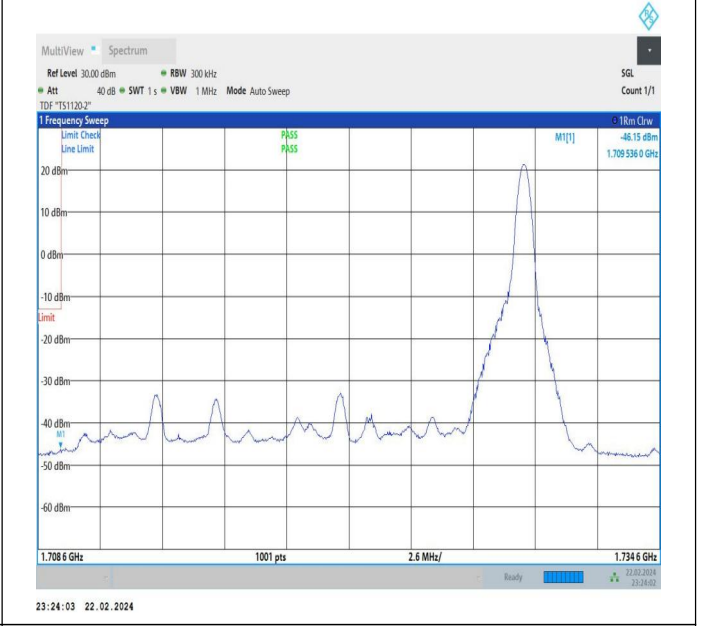
20MHz-5MHz_QPSK@QPSK-QPSK@QPSK_132072-132189_9_1RB#99@100RB#0-0RB#0@25RB#0
