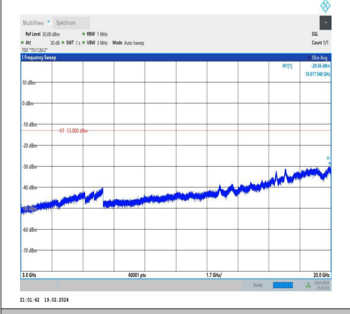
66-66-5MHz-20MHz-QPSK-QPSK-132027-132171-1RB#0-1R B#99-3000~20000MHz-PASS
