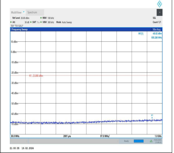
66-66-5MHz-20MHz-QPSK-QPSK-132027-132171-1RB#24-0 RB#0-30~1000MHz-PASS
