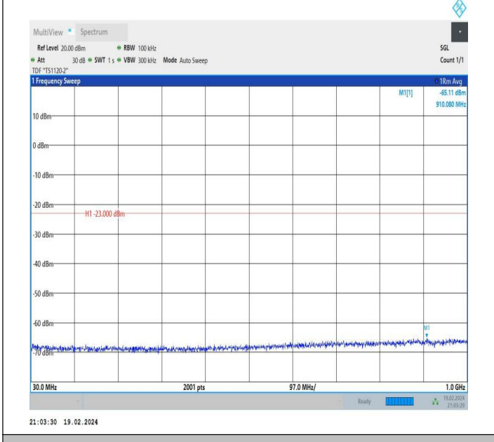
66-66-5MHz-20MHz-QPSK-QPSK-132328-132472-1RB#24-0 RB#0-30~1000MHz-PASS
