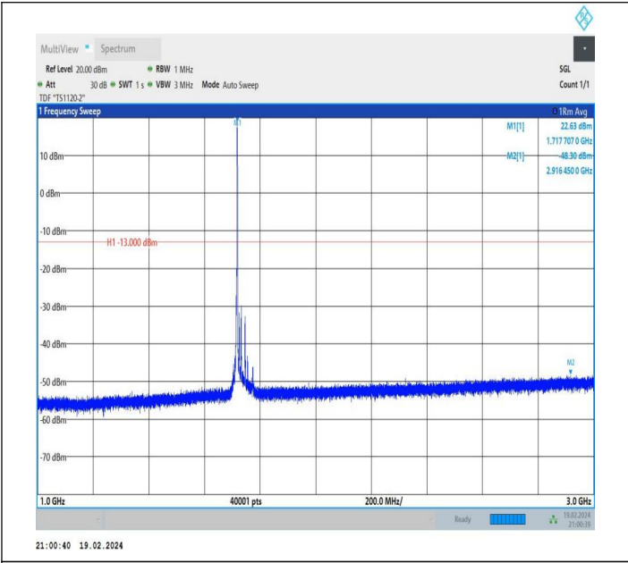
66-66-5MHz-20MHz-QPSK-QPSK-132027-132171-1RB#24-0 RB#0-1000~3000MHz-PASS
