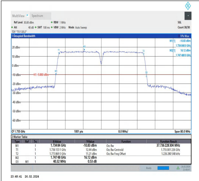
66-66-20MHz-20MHz-QPSK-QPSK-132323-132521-100RB# 0-100RB#0-PASS
