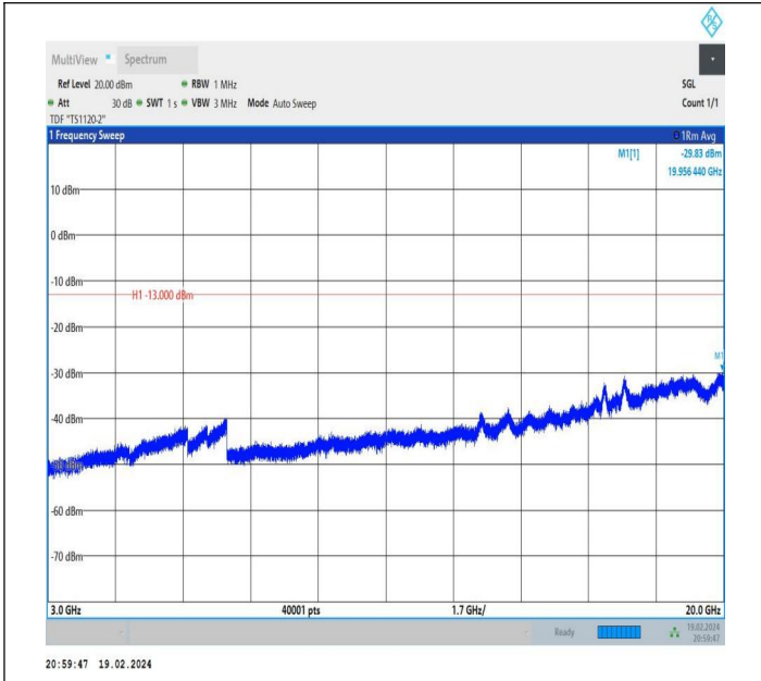
66-66-5MHz-20MHz-QPSK-QPSK-132027-132171-1RB#0-0R B#0-3000~20000MHz-PASS
