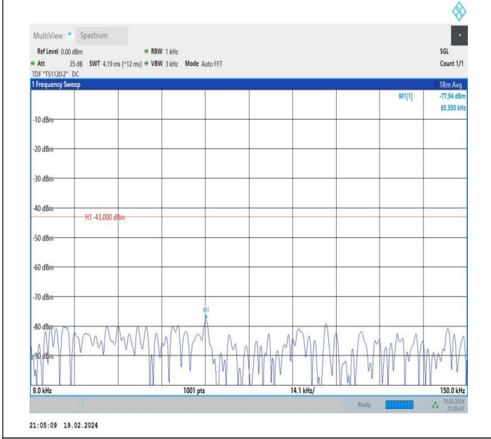
66-66-5MHz-20MHz-QPSK-QPSK-132428-132572-1RB#0-0R B#0-0.009~0.15MHz-PASS
