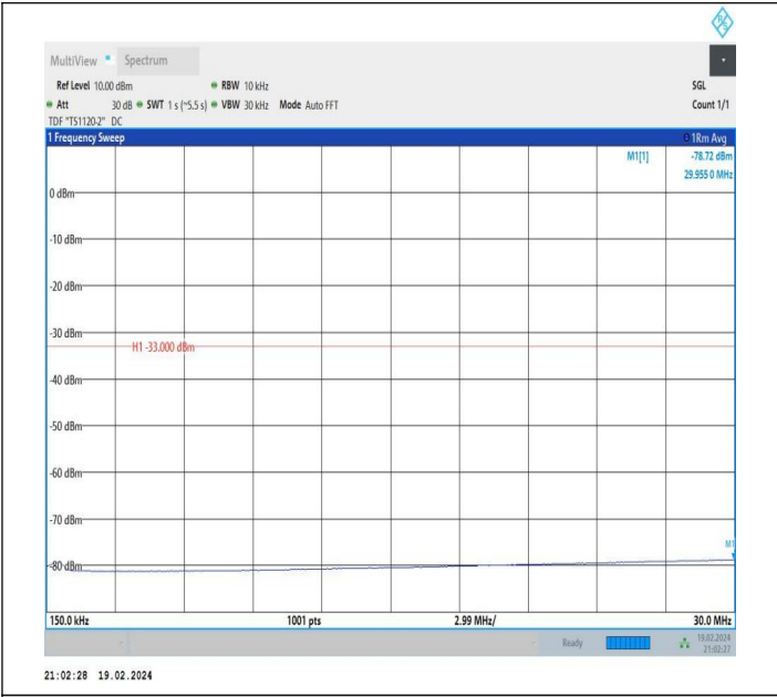
66-66-5MHz-20MHz-QPSK-QPSK-132328-132472-1RB#0-0R B#0-0.15~30MHz-PASS
