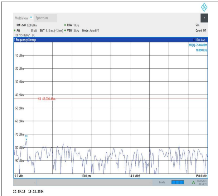
66-66-5MHz-20MHz-QPSK-QPSK-132027-132171-1RB#0-0R B#0-0.009~0.15MHz-PASS
