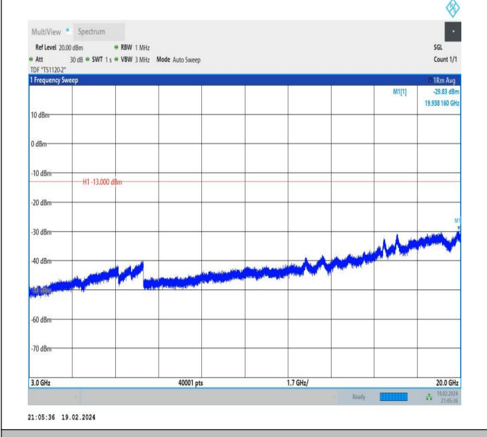
66-66-5MHz-20MHz-QPSK-QPSK-132428-132572-1RB#0-0R B#0-3000~20000MHz-PASS
