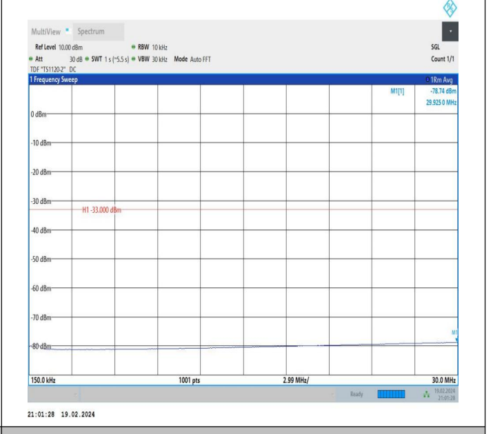
66-66-5MHz-20MHz-QPSK-QPSK-132027-132171-1RB#0-1R B#99-0.15~30MHz-PASS
