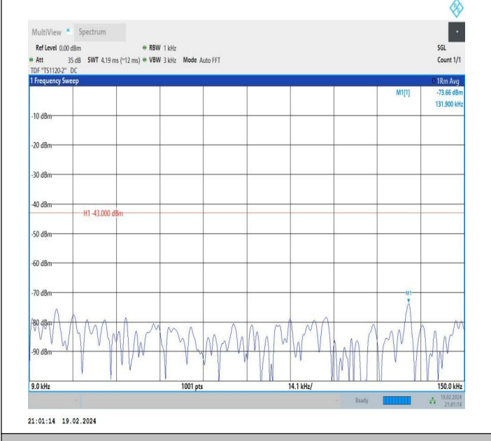
66-66-5MHz-20MHz-QPSK-QPSK-132027-132171-1RB#0-1R B#99-0.009~0.15MHz-PASS
