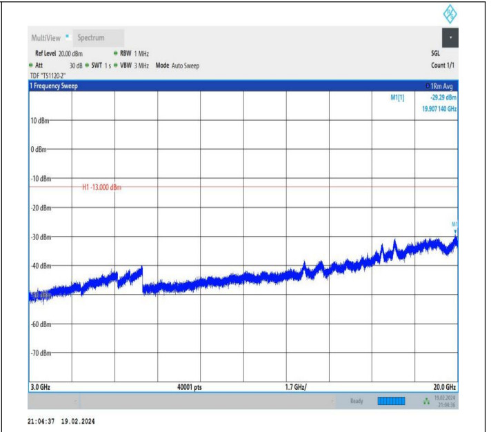
66-66-5MHz-20MHz-QPSK-QPSK-132328-132472-1RB#0-1R B#99-3000~20000MHz-PASS
