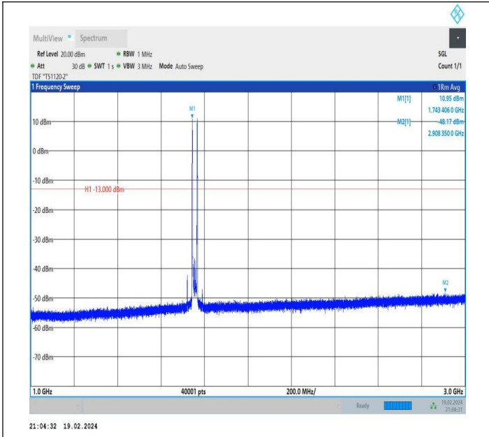
66-66-5MHz-20MHz-QPSK-QPSK-132328-132472-1RB#0-1R B#99-1000~3000MHz-PASS
