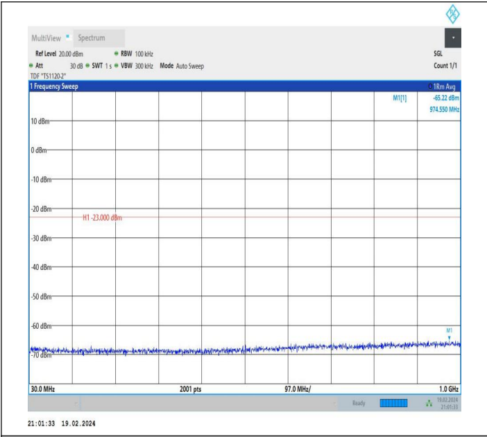
66-66-5MHz-20MHz-QPSK-QPSK-132027-132171-1RB#0-1R B#99-30~1000MHz-PASS
