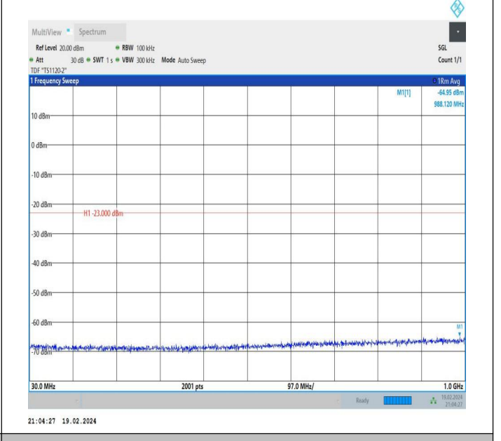
66-66-5MHz-20MHz-QPSK-QPSK-132328-132472-1RB#0-1R B#99-30~1000MHz-PASS
