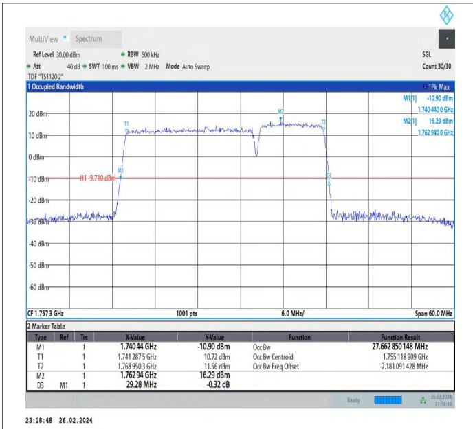
66-66-20MHz-10MHz-QPSK-QPSK-132373-132517-100RB# 0-50RB#0-PASS
