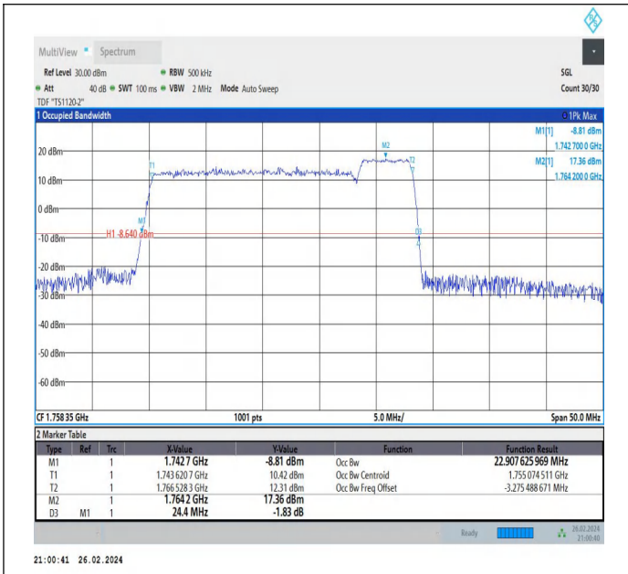
66-66-20MHz-5MHz-QPSK-QPSK-132397-132514-100RB#0-25RB#0-PASS
