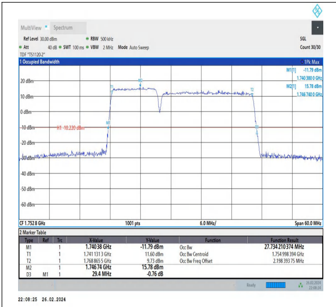
66-66-10MHz-20MHz-QPSK-QPSK-132328-132472-50RB#0-100RB#0-PASS
