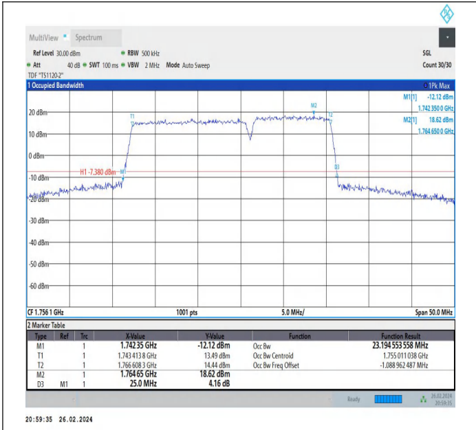
66-66-15MHz-10MHz-QPSK-QPSK-132373-132493-75RB#0-50RB#0-PASS
