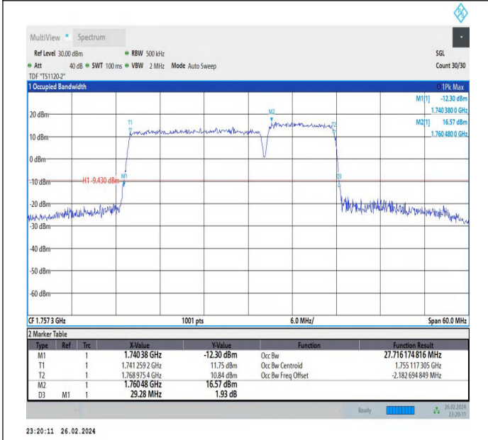
66-66-20MHz-10MHz-64QAM-64QAM-132373-132517-100RB#0-50RB#0-PASS
