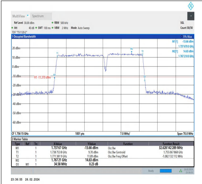
66-66-20MHz-15MHz-QPSK-QPSK-132348-132519-100RB# 0-75RB#0-PASS
