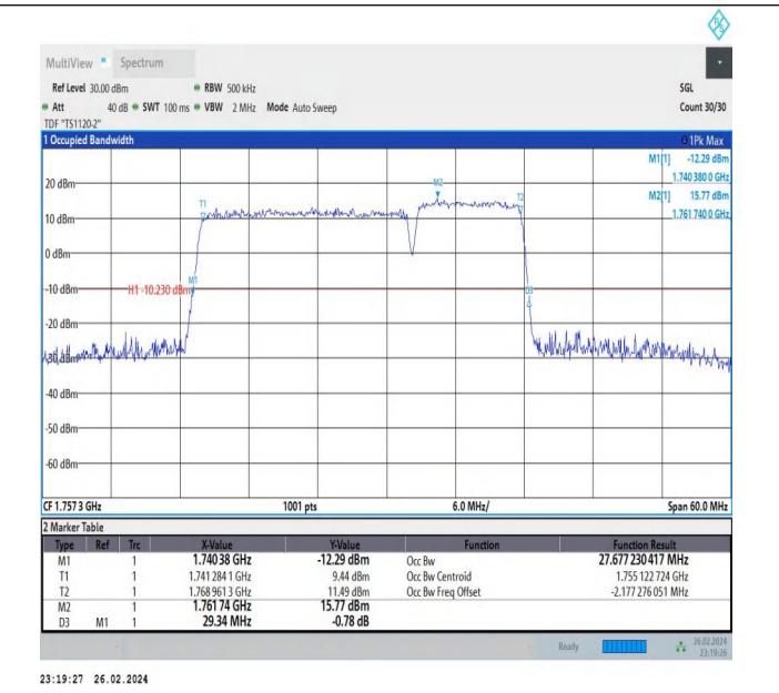
66-66-20MHz-10MHz-16QAM-16QAM-132373-132517-100RB# 0-50RB#0-PASS
