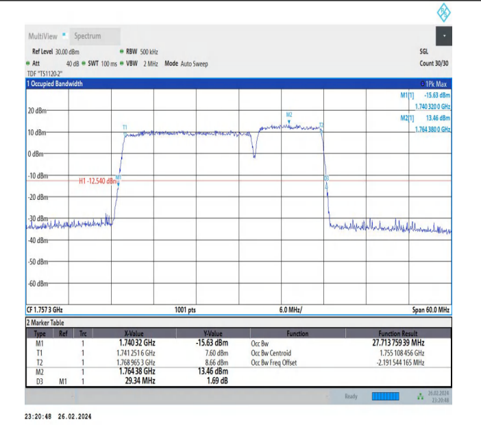
66-66-20MHz-10MHz-256QAM-256QAM-132373-132517-100RB#0-50RB#0-PASS
