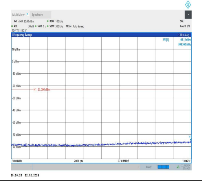
66-66-10MHz-10MHz-QPSK-QPSK-132022-132121-1RB#0-1RB#49-30~1000MHz-PASS
