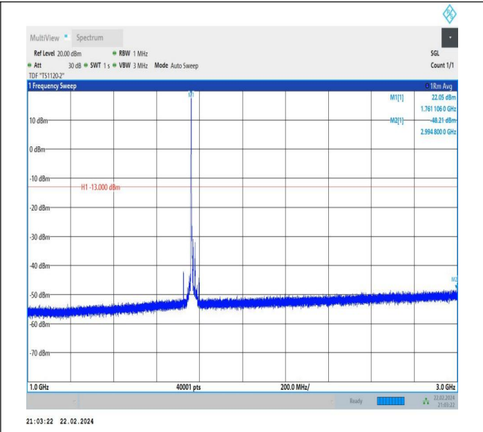
66-66-5MHz-15MHz-QPSK-QPSK-132504-132597-1RB#0-0R B#0-1000~3000MHz-PASS
