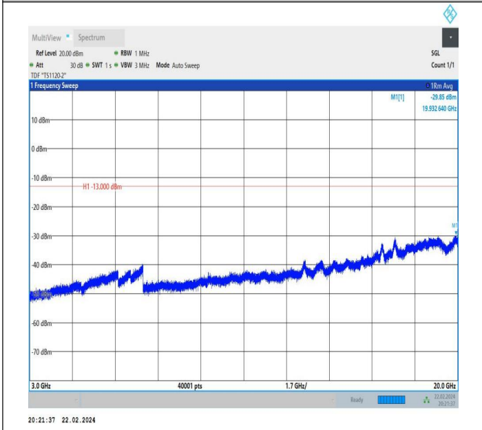
66-66-10MHz-10MHz-QPSK-QPSK-132373-132472-1RB#0-0 RB#0-3000~20000MHz-PASS
