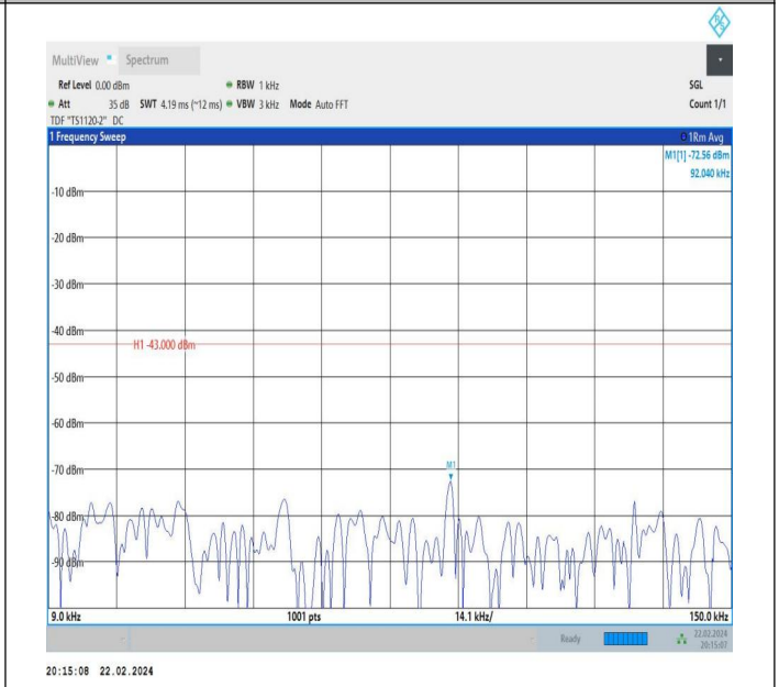
66-66-10MHz-10MHz-QPSK-QPSK-132022-132121-1RB#0-0 RB#0-0.009~0.15MHz-PASS
