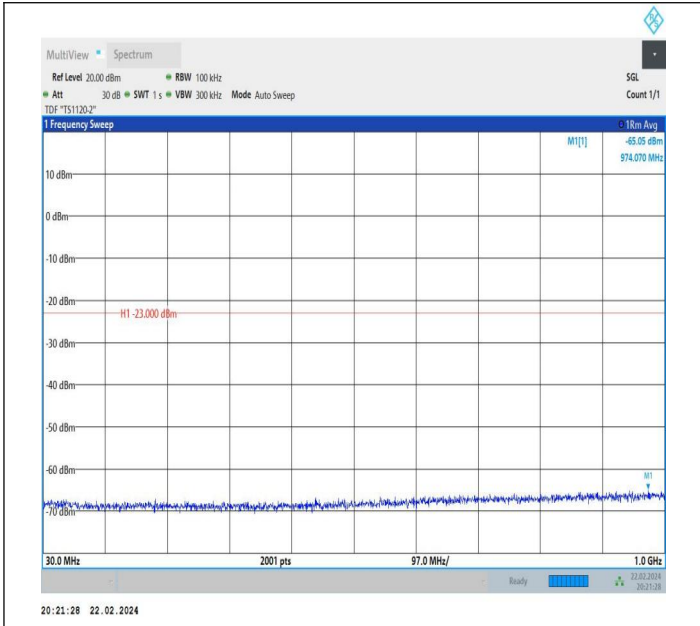
66-66-10MHz-10MHz-QPSK-QPSK-132373-132472-1RB#0-0 RB#0-30~1000MHz-PASS
