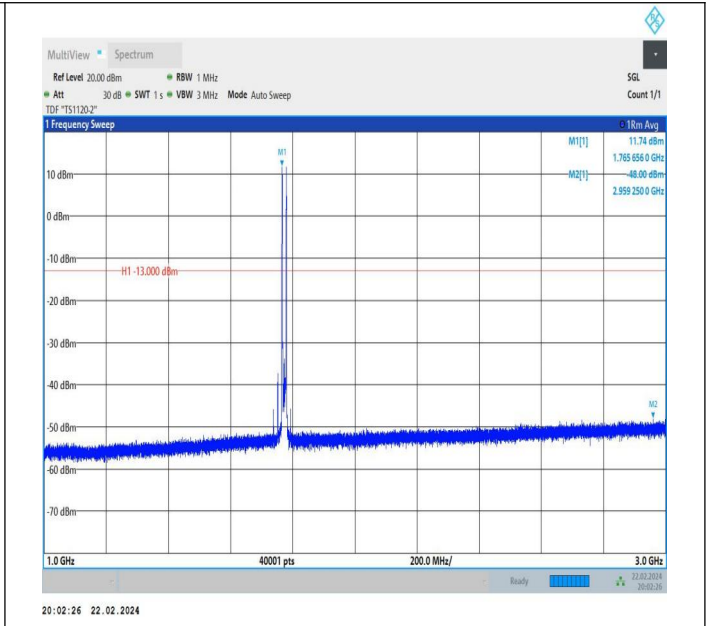
66-66-10MHz-5MHz-QPSK-QPSK-132572-132644-1RB#0-1R B#24-1000~3000MHz-PASS
