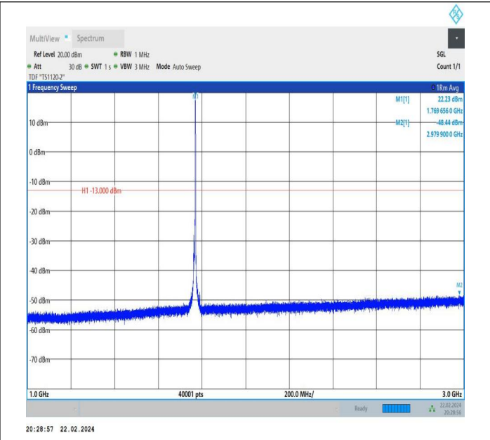
66-66-10MHz-10MHz-QPSK-QPSK-132523-132622-1RB#49-ORB#0-1000~3000MHz-PASS
