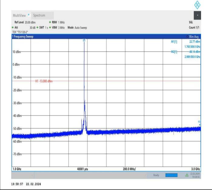
66-66-10MHz-5MHz-QPSK-QPSK-132572-132644-1RB#0-0R B#0-1000~3000MHz-PASS
