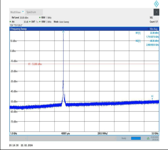
66-66-10MHz-10MHz-QPSK-QPSK-132022-132121-1RB#49-ORB#0-1000~3000MHz-PASS
