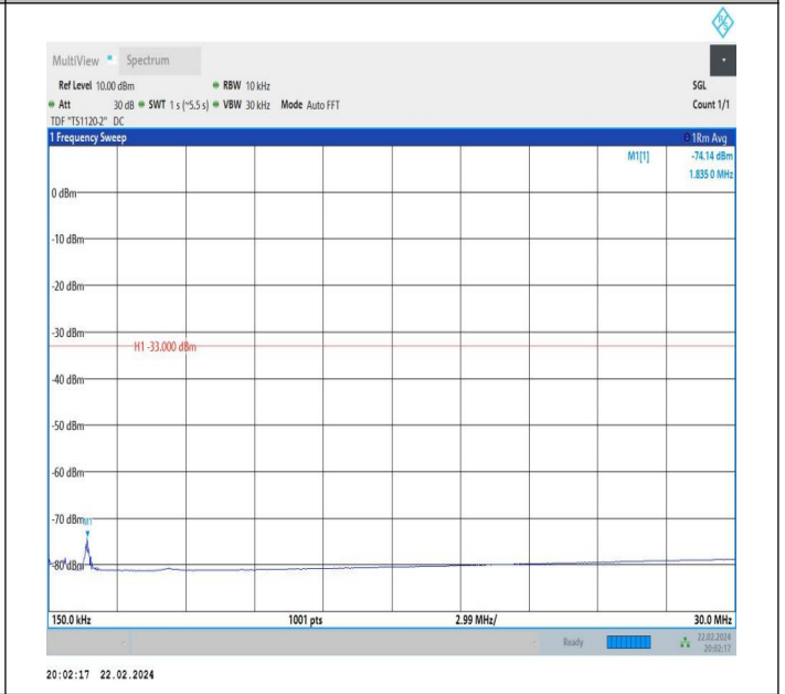
66-66-10MHz-5MHz-QPSK-QPSK-132572-132644-1RB#0-1R B#24-0.15~30MHz-PASS
