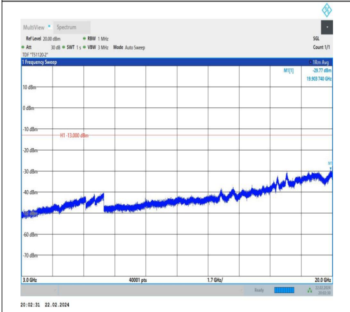
66-66-10MHz-5MHz-QPSK-QPSK-132572-132644-1RB#0-1R B#24-3000~20000MHz-PASS
