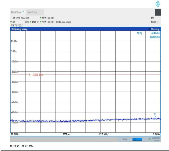
66-66-10MHz-10MHz-QPSK-QPSK-132373-132472-1RB#0-1 RB#49-30~1000MHz-PASS
