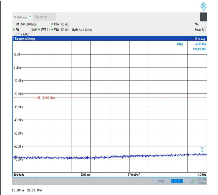
66-66-10MHz-10MHz-QPSK-QPSK-132523-132622-1RB#49-ORB#0-30~1000MHz-PASS
