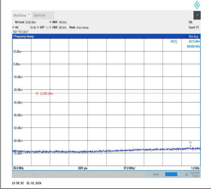
66-66-10MHz-5MHz-QPSK-QPSK-132572-132644-1RB#0-0R B#0-30~1000MHz-PASS
