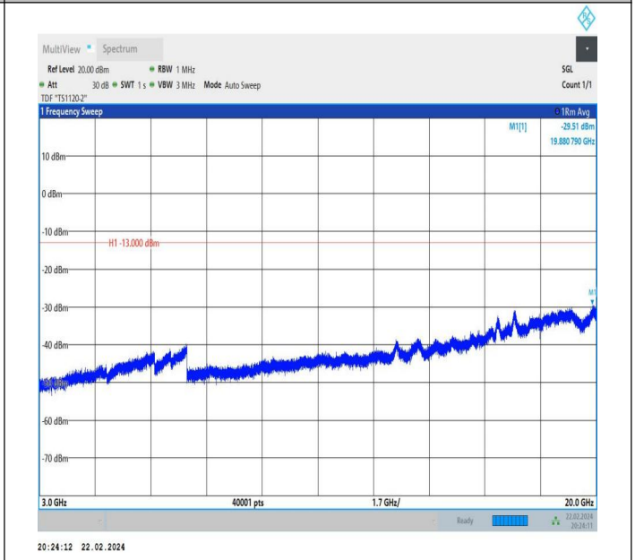
66-66-10MHz-10MHz-QPSK-QPSK-132373-132472-1RB#49-ORB#0-3000~20000MHz-PASS
