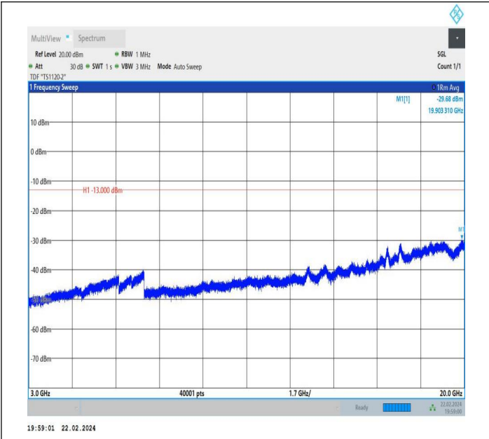
66-66-10MHz-5MHz-QPSK-QPSK-132572-132644-1RB#0-0R B#0-3000~20000MHz-PASS
