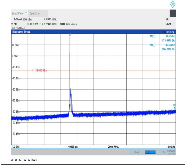
66-66-10MHz-10MHz-QPSK-QPSK-132022-132121-1RB#0-0 RB#0-1000~3000MHz-PASS
