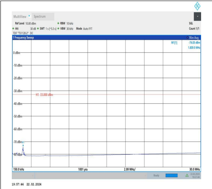
66-66-10MHz-5MHz-QPSK-QPSK-132397-132469-1RB#0-1R B#24-0.15~30MHz-PASS
