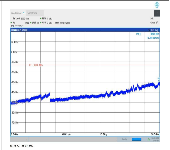
66-66-10MHz-10MHz-QPSK-QPSK-132523-132622-1RB#0-0 RB#0-3000~20000MHz-PASS
