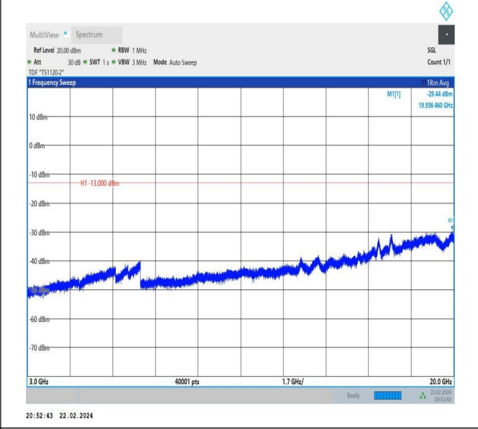
66-66-5MHz-15MHz-QPSK-QPSK-132353-132446-1RB#0-0R B#0-3000~20000MHz-PASS
