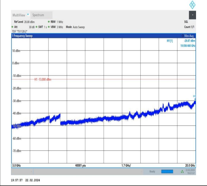
66-66-10MHz-5MHz-QPSK-QPSK-132397-132469-1RB#0-1R B#24-3000~20000MHz-PASS
