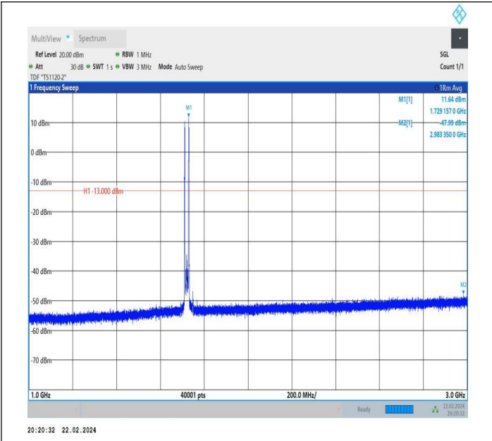
66-66-10MHz-10MHz-QPSK-QPSK-132022-132121-1RB#0-1 RB#49-1000~3000MHz-PASS
