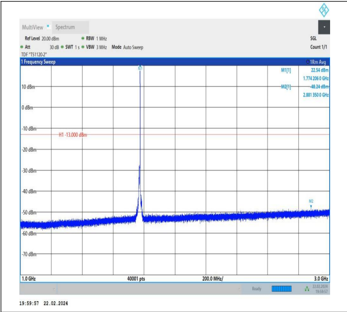
66-66-10MHz-5MHz-QPSK-QPSK-132572-132644-1RB#49-0 RB#0-1000~3000MHz-PASS
