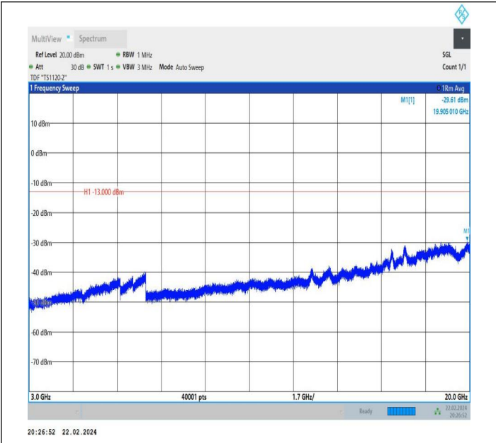
66-66-10MHz-10MHz-QPSK-QPSK-132373-132472-1RB#0-1 RB#49-3000~20000MHz-PASS
