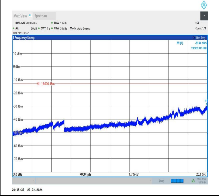
66-66-10MHz-10MHz-QPSK-QPSK-132022-132121-1RB#0-0 RB#0-3000~20000MHz-PASS
