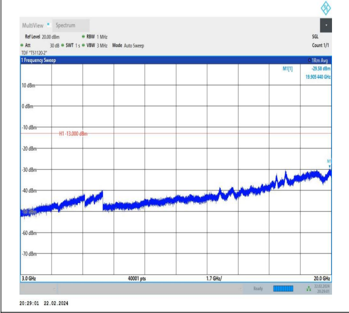
66-66-10MHz-10MHz-QPSK-QPSK-132523-132622-1RB#49-ORB#0-3000~20000MHz-PASS
