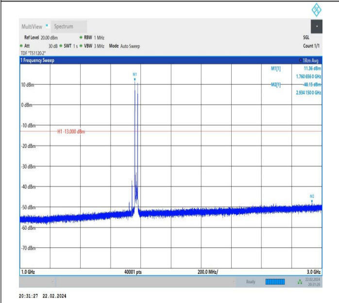
66-66-10MHz-10MHz-QPSK-QPSK-132523-132622-1RB#0-1 RB#49-1000~3000MHz-PASS
