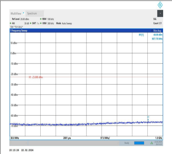
66-66-10MHz-10MHz-QPSK-QPSK-132022-132121-1RB#0-0 RB#0-30~1000MHz-PASS
