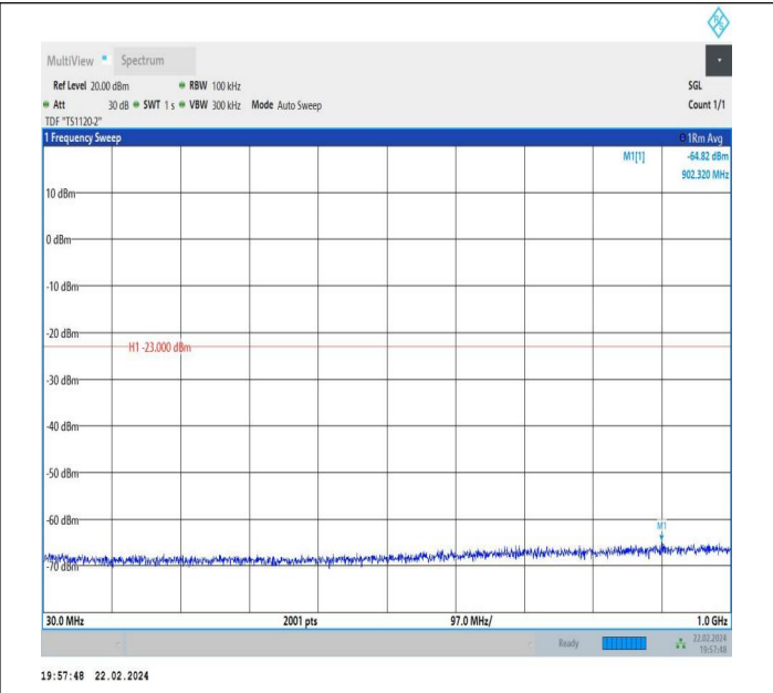
66-66-10MHz-5MHz-QPSK-QPSK-132397-132469-1RB#0-1R B#24-30~1000MHz-PASS
