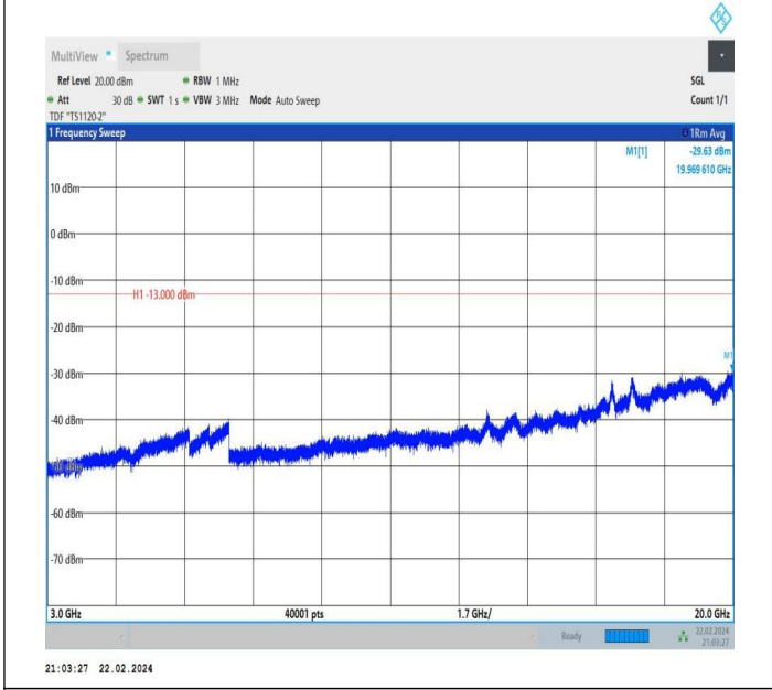
66-66-5MHz-15MHz-QPSK-QPSK-132504-132597-1RB#0-0R B#0-3000~20000MHz-PASS
