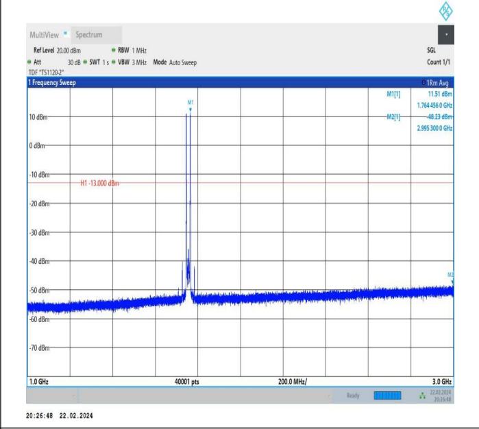
66-66-10MHz-10MHz-QPSK-QPSK-132373-132472-1RB#0-1 RB#49-1000~3000MHz-PASS
