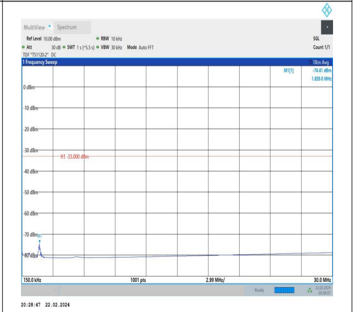
66-66-10MHz-10MHz-QPSK-QPSK-132523-132622-1RB#49- ORB#0-0.15~30MHz-PASS
