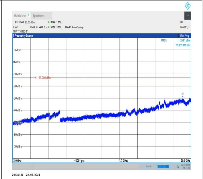
66-66-10MHz-10MHz-QPSK-QPSK-132523-132622-1RB#0-1 RB#49-3000~20000MHz-PASS
