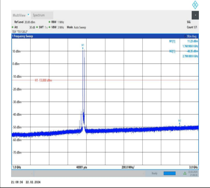
66-66-5MHz-15MHz-QPSK-QPSK-132504-132597-1RB#0-1R B#74-1000~3000MHz-PASS
