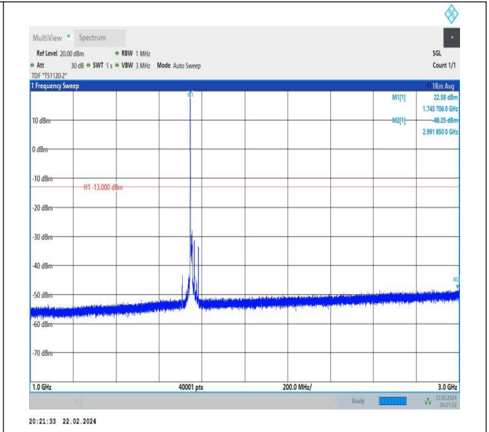
66-66-10MHz-10MHz-QPSK-QPSK-132373-132472-1RB#0-0 RB#0-1000~3000MHz-PASS
