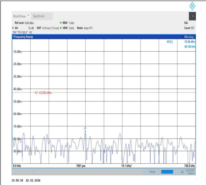
66-66-10MHz-5MHz-QPSK-QPSK-132572-132644-1RB#0-0R B#0-0.009~0.15MHz-PASS
