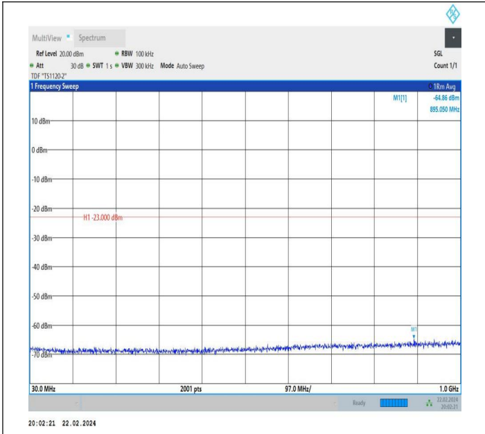
66-66-10MHz-5MHz-QPSK-QPSK-132572-132644-1RB#0-1R B#24-30~1000MHz-PASS
