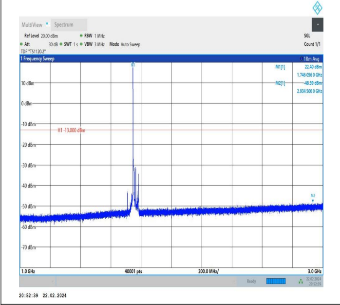
66-66-5MHz-15MHz-QPSK-QPSK-132353-132446-1RB#0-0R B#0-1000~3000MHz-PASS
