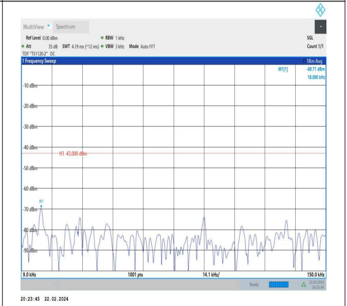
66-66-10MHz-10MHz-QPSK-QPSK-132373-132472-1RB#49- ORB#0-0.009~0.15MHz-PASS
