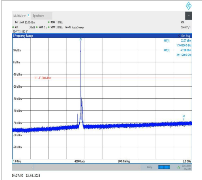
66-66-10MHz-10MHz-QPSK-QPSK-132523-132622-1RB#0-0 RB#0-1000~3000MHz-PASS
