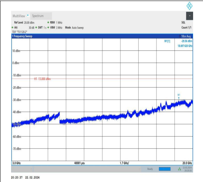
66-66-10MHz-10MHz-QPSK-QPSK-132022-132121-1RB#0-1 RB#49-3000~20000MHz-PASS
