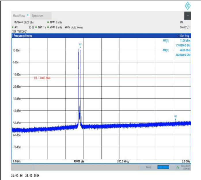
66-66-5MHz-15MHz-QPSK-QPSK-132353-132446-1RB#0-1R B#74-1000~3000MHz-PASS
