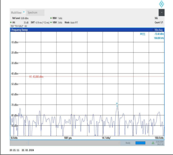
66-66-10MHz-10MHz-QPSK-QPSK-132373-132472-1RB#0-0 RB#0-0.009~0.15MHz-PASS
