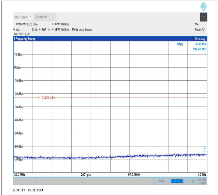
66-66-5MHz-15MHz-QPSK-QPSK-132504-132597-1RB#0-0R B#0-30~1000MHz-PASS
