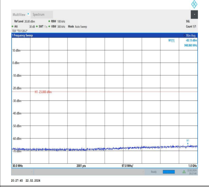
66-66-10MHz-10MHz-QPSK-QPSK-132523-132622-1RB#0-0 RB#0-30~1000MHz-PASS
