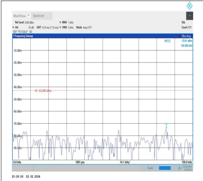
66-66-10MHz-10MHz-QPSK-QPSK-132373-132472-1RB#0-1 RB#49-0.009~0.15MHz-PASS
