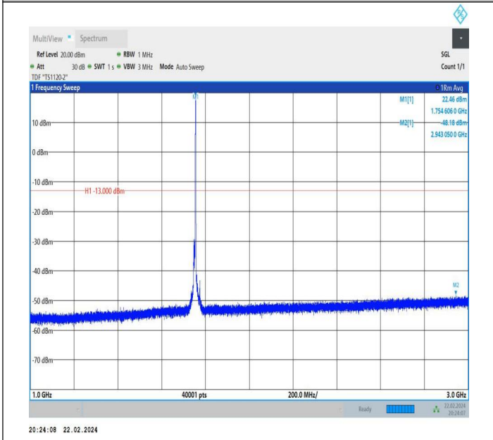
66-66-10MHz-10MHz-QPSK-QPSK-132373-132472-1RB#49-ORB#0-1000~3000MHz-PASS
