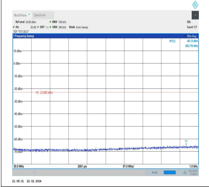
66-66-5MHz-15MHz-QPSK-QPSK-132504-132597-1RB#0-1R B#74-30~1000MHz-PASS
