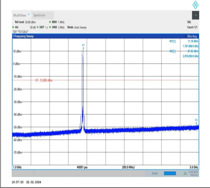
66-66-10MHz-5MHz-QPSK-QPSK-132397-132469-1RB#0-1R B#24-1000~3000MHz-PASS
