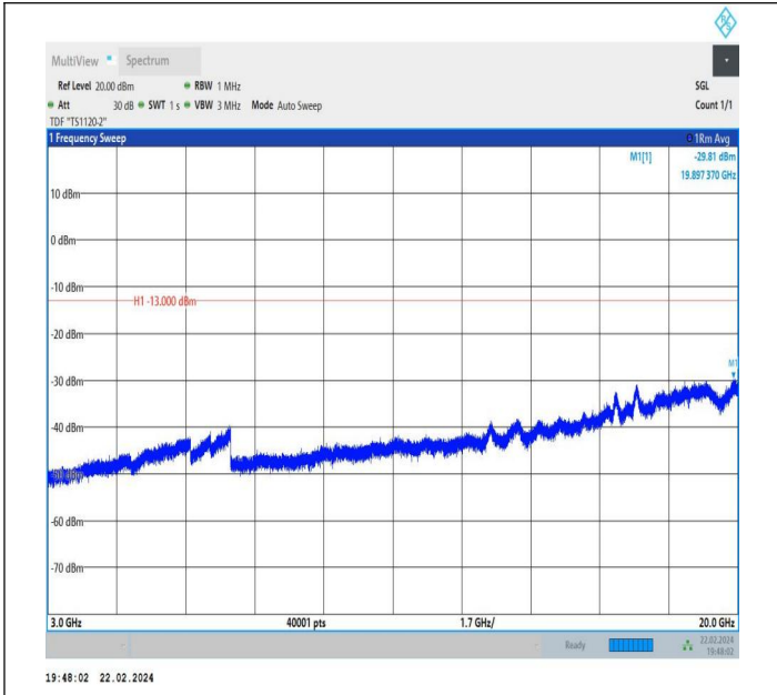
66-66-10MHz-5MHz-QPSK-QPSK-132022-132094-1RB#0-1R B#24-3000~20000MHz-PASS
