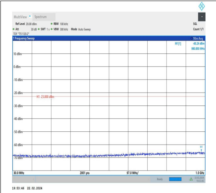
66-66-10MHz-5MHz-QPSK-QPSK-132397-132469-1RB#49-0 RB#0-30~1000MHz-PASS
