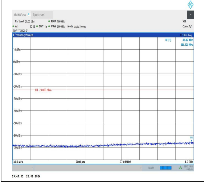
66-66-10MHz-5MHz-QPSK-QPSK-132022-132094-1RB#0-1R B#24-30~1000MHz-PASS
