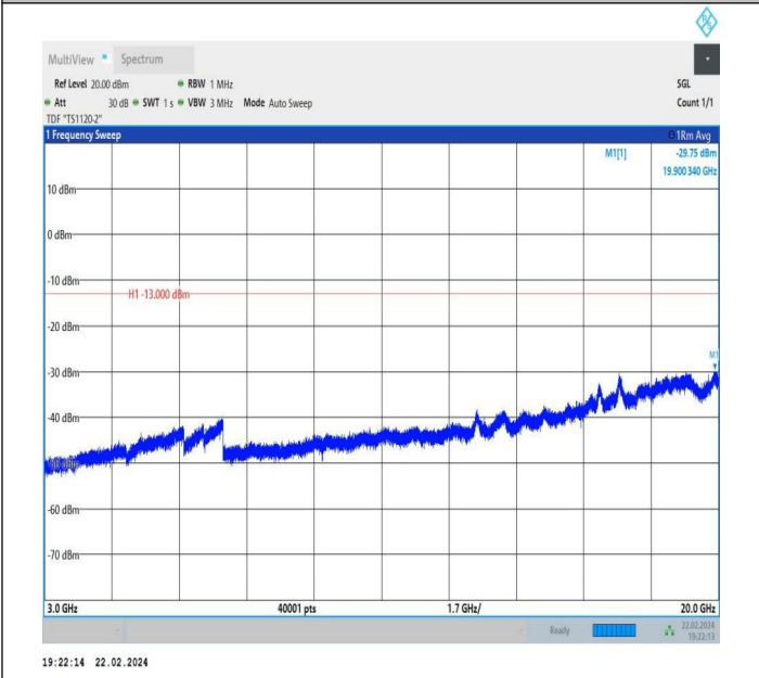
66-66-5MHz-10MHz-QPSK-QPSK-132375-132447-1RB#0-1R B#49-3000~20000MHz-PASS
