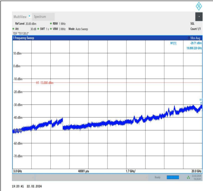
66-66-5MHz-10MHz-QPSK-QPSK-132375-132447-1RB#0-0R B#0-3000~20000MHz-PASS
