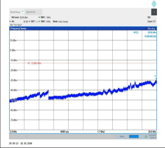
66-66-5MHz-5MHz-QPSK-QPSK-132398-132446-1RB#0-ORB #0-3000~20000MHz-PASS
