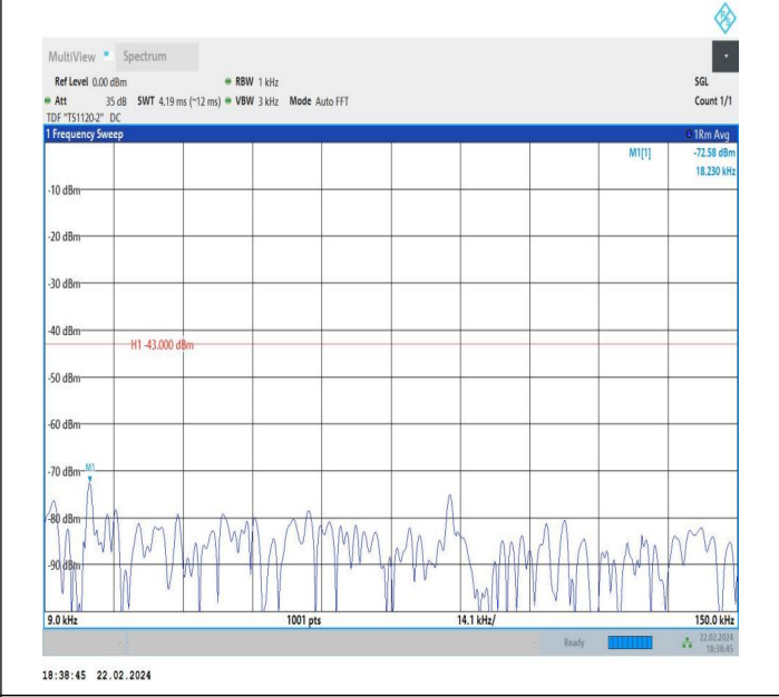
66-66-5MHz-5MHz-QPSK-QPSK-132398-132446-1RB#0-ORB #0-0.009~0.15MHz-PASS
