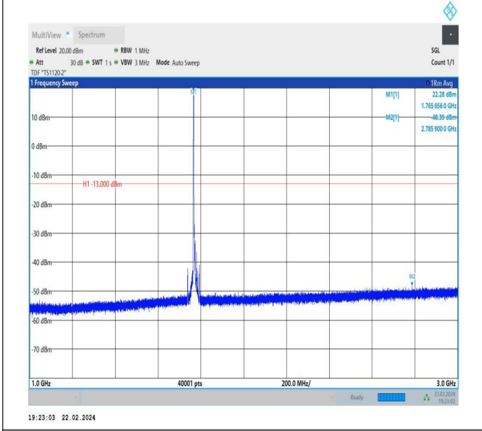
66-66-5MHz-10MHz-QPSK-QPSK-132550-132622-1RB#0-0R B#0-1000~3000MHz-PASS
