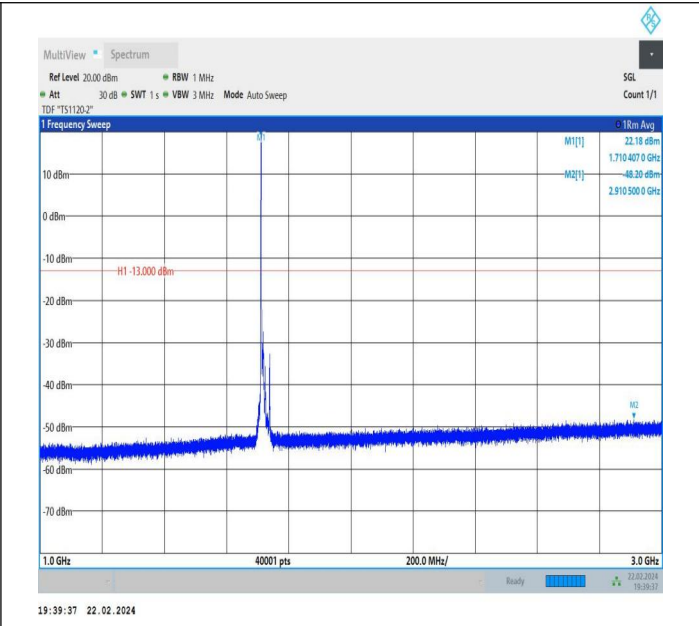
66-66-10MHz-5MHz-QPSK-QPSK-132022-132094-1RB#0-0R B#0-1000~3000MHz-PASS
