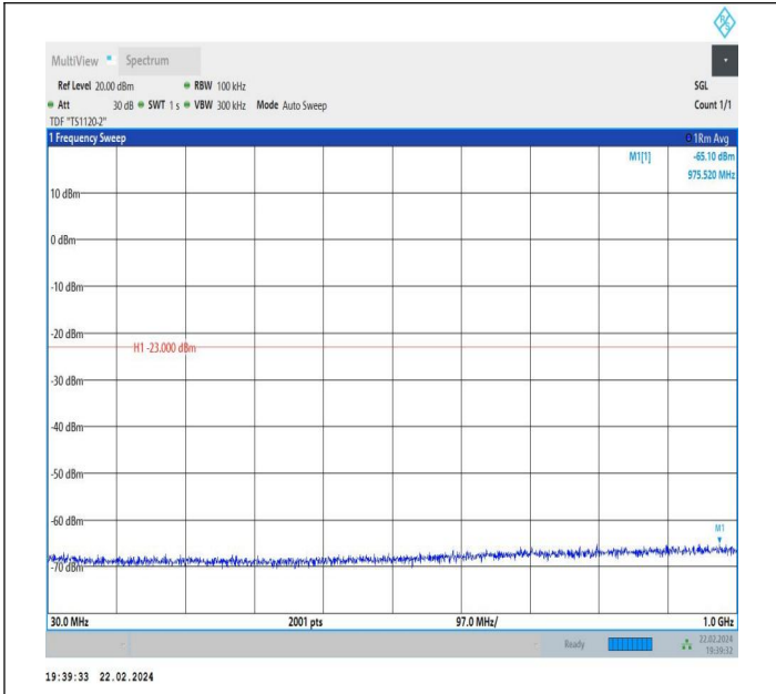
66-66-10MHz-5MHz-QPSK-QPSK-132022-132094-1RB#0-0R B#0-30~1000MHz-PASS
