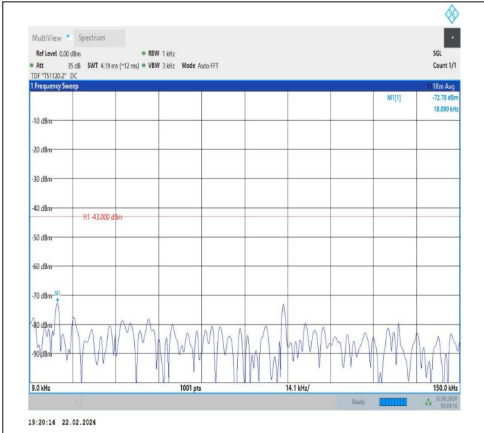
66-66-5MHz-10MHz-QPSK-QPSK-132375-132447-1RB#0-0R B#0-0.009~0.15MHz-PASS
