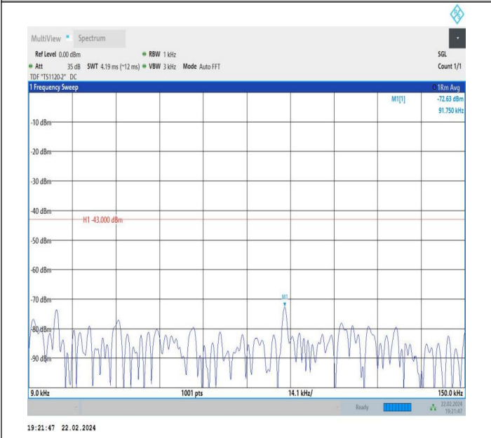
66-66-5MHz-10MHz-QPSK-QPSK-132375-132447-1RB#0-1R B#49-0.009~0.15MHz-PASS
