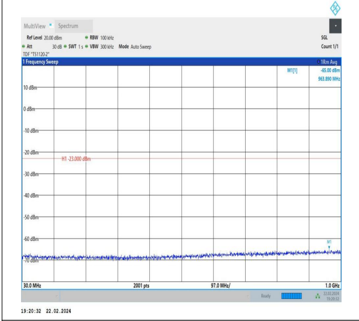
66-66-5MHz-10MHz-QPSK-QPSK-132375-132447-1RB#0-0R B#0-30~1000MHz-PASS
