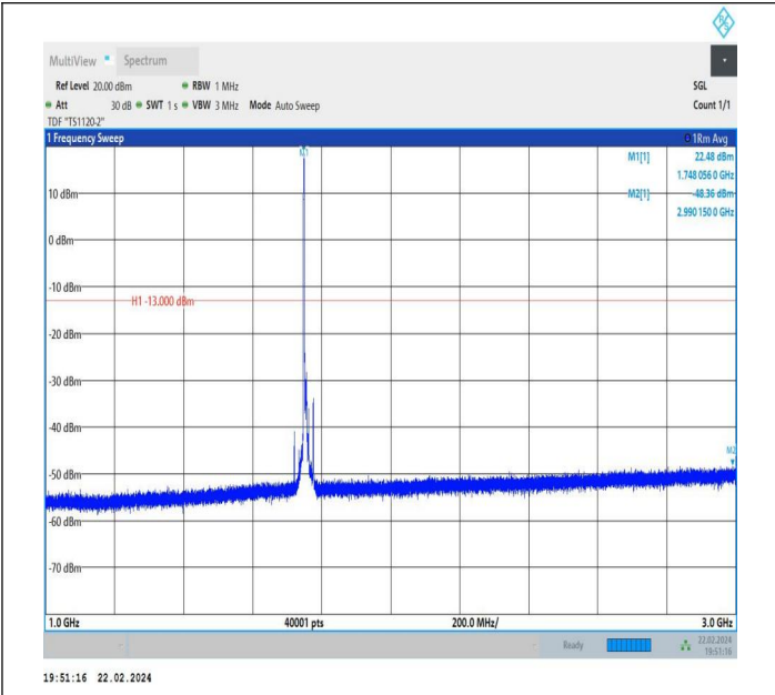
66-66-10MHz-5MHz-QPSK-QPSK-132397-132469-1RB#0-0R B#0-1000~3000MHz-PASS
