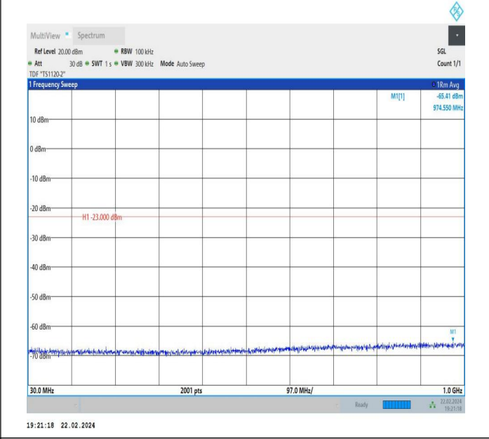
66-66-5MHz-10MHz-QPSK-QPSK-132375-132447-1RB#24-0 RB#0-30~1000MHz-PASS
