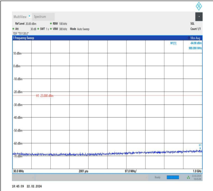
66-66-5MHz-5MHz-QPSK-QPSK-132599-132647-1RB#0-ORB #0-30~1000MHz-PASS
