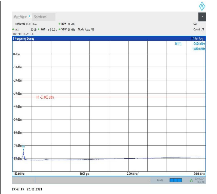
66-66-10MHz-5MHz-QPSK-QPSK-132022-132094-1RB#0-1R B#24-0.15~30MHz-PASS
