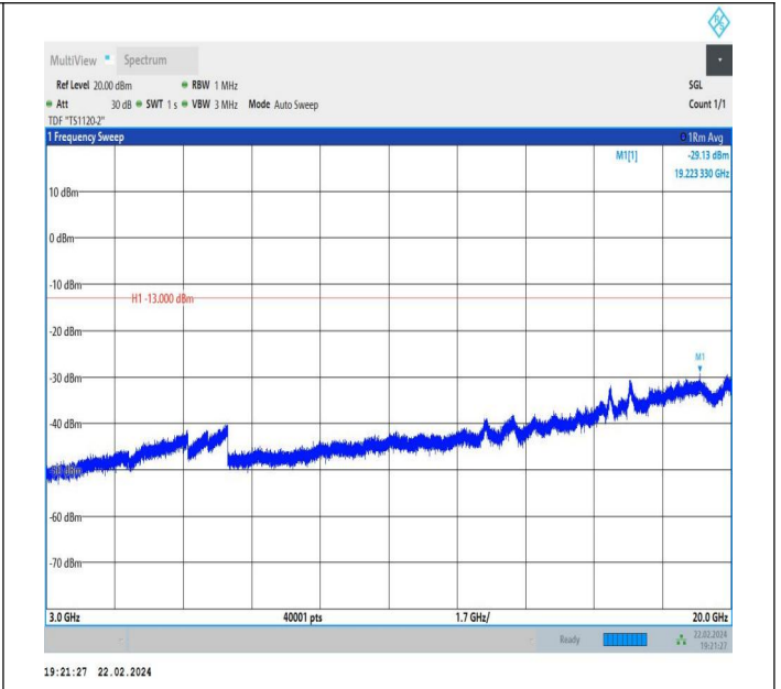
66-66-5MHz-10MHz-QPSK-QPSK-132375-132447-1RB#24-0 RB#0-3000~20000MHz-PASS
