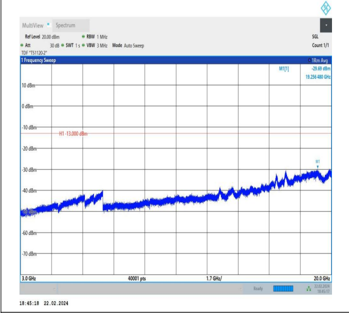
66-66-5MHz-5MHz-QPSK-QPSK-132599-132647-1RB#0-ORB #0-3000~20000MHz-PASS
