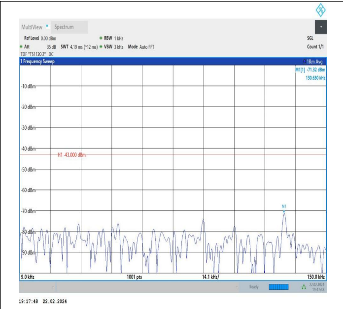
66-66-5MHz-10MHz-QPSK-QPSK-132000-132072-1RB#0-0R B#0-0.009~0.15MHz-PASS
