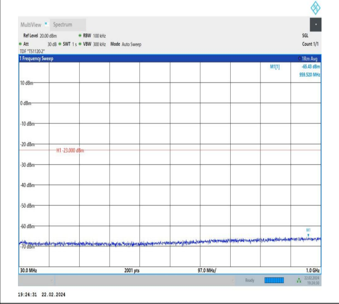
66-66-5MHz-10MHz-QPSK-QPSK-132550-132622-1RB#0-1R B#49-30~1000MHz-PASS
