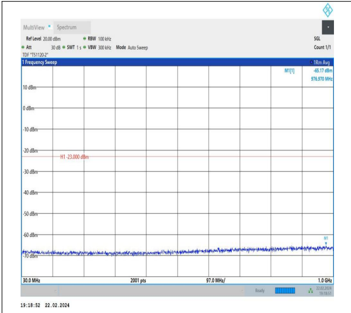
66-66-5MHz-10MHz-QPSK-QPSK-132000-132072-1RB#24-0 RB#0-30~1000MHz-PASS
