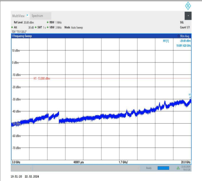
66-66-10MHz-5MHz-QPSK-QPSK-132397-132469-1RB#0-0R B#0-3000~20000MHz-PASS
