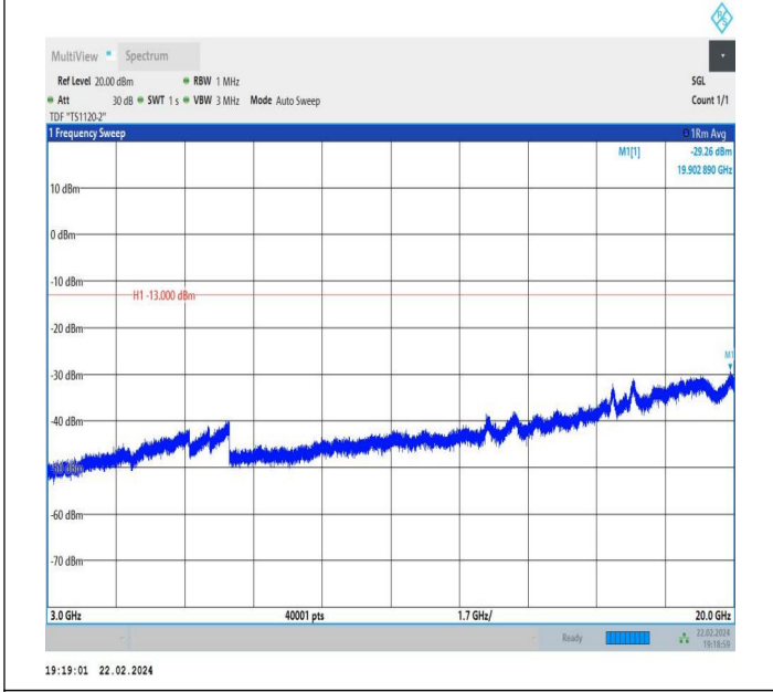
66-66-5MHz-10MHz-QPSK-QPSK-132000-132072-1RB#24-0 RB#0-3000~20000MHz-PASS
