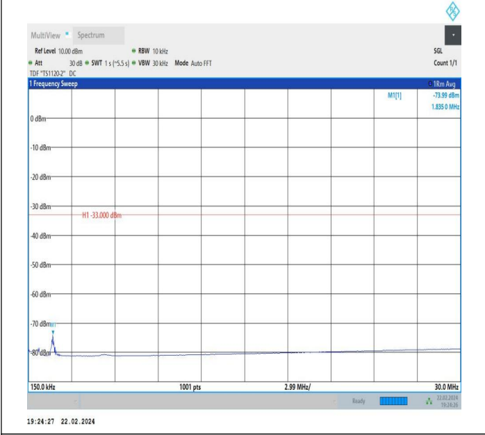
66-66-5MHz-10MHz-QPSK-QPSK-132550-132622-1RB#0-1R B#49-0.15~30MHz-PASS
