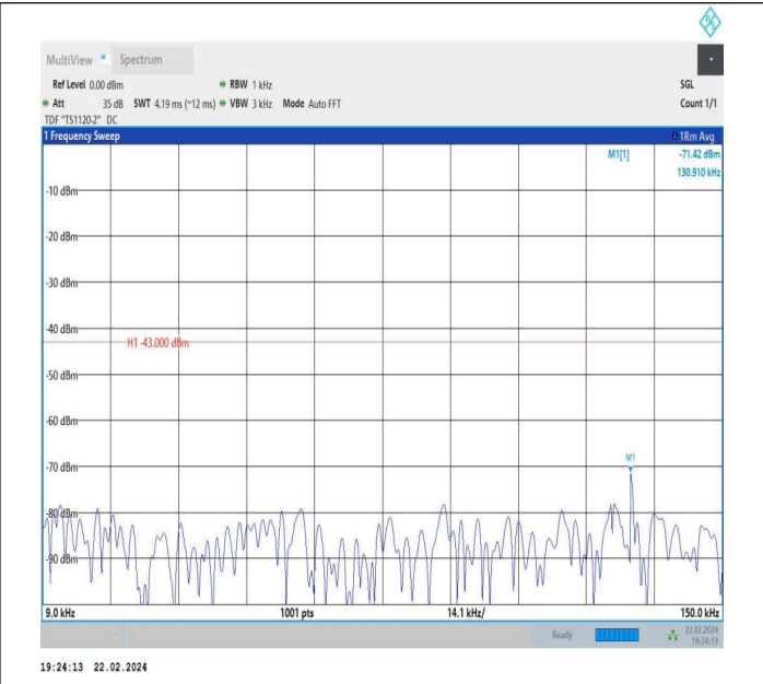
66-66-5MHz-10MHz-QPSK-QPSK-132550-132622-1RB#0-1R B#49-0.009~0.15MHz-PASS
