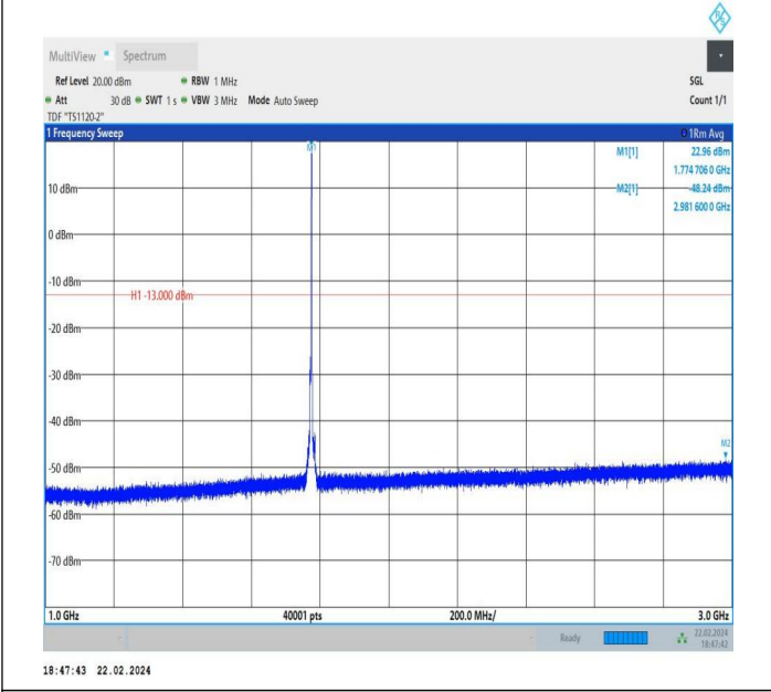
66-66-5MHz-5MHz-QPSK-QPSK-132599-132647-1RB#24-0R B#0-1000~3000MHz-PASS
