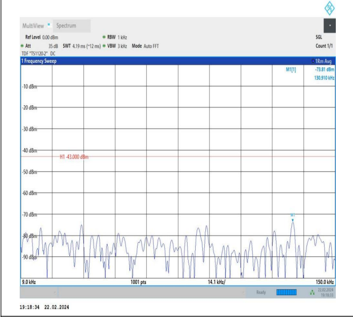
66-66-5MHz-10MHz-QPSK-QPSK-132000-132072-1RB#24-0 RB#0-0.009~0.15MHz-PASS
