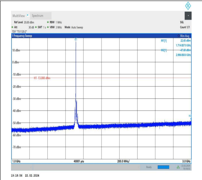
66-66-5MHz-10MHz-QPSK-QPSK-132000-132072-1RB#24-0 RB#0-1000~3000MHz-PASS
