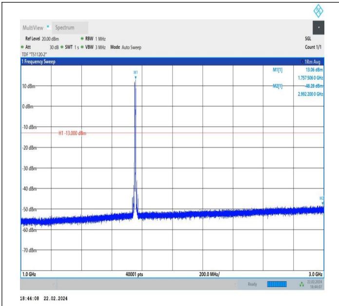
66-66-5MHz-5MHz-QPSK-QPSK-132398-132446-1RB#0-1RB #15-1000~3000MHz-PASS
