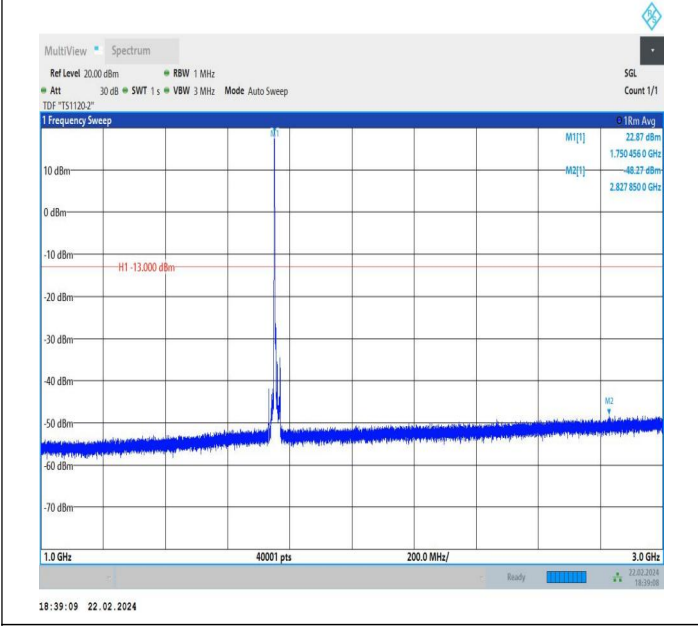
66-66-5MHz-5MHz-QPSK-QPSK-132398-132446-1RB#0-ORB #0-1000~3000MHz-PASS
