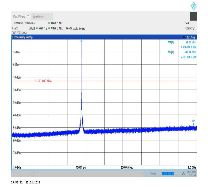
66-66-10MHz-5MHz-QPSK-QPSK-132397-132469-1RB#49-0 RB#0-1000~3000MHz-PASS
