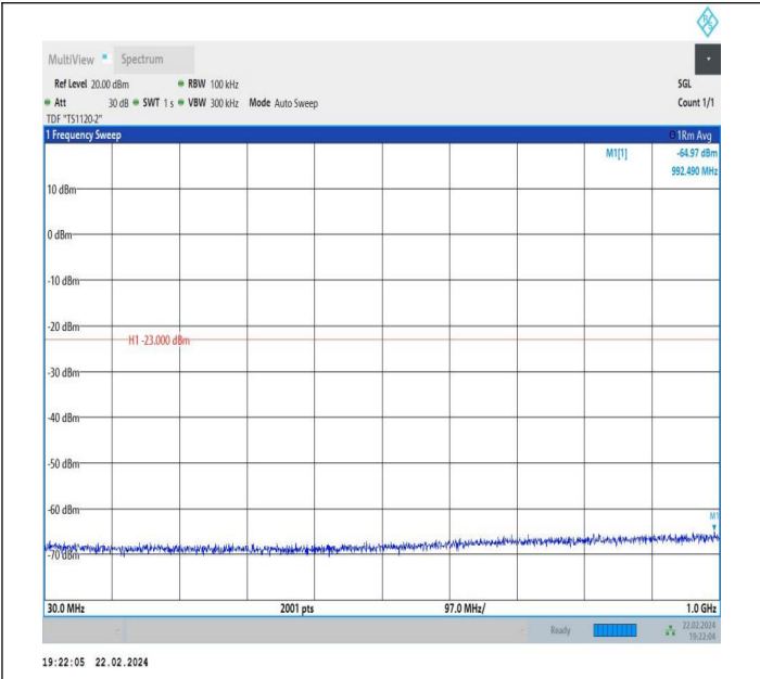
66-66-5MHz-10MHz-QPSK-QPSK-132375-132447-1RB#0-1R B#49-30~1000MHz-PASS
