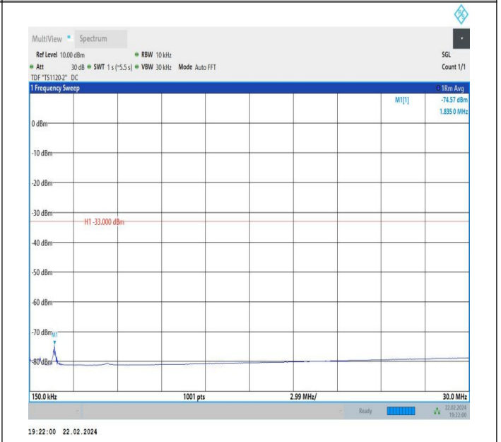
66-66-5MHz-10MHz-QPSK-QPSK-132375-132447-1RB#0-1R B#49-0.15~30MHz-PASS
