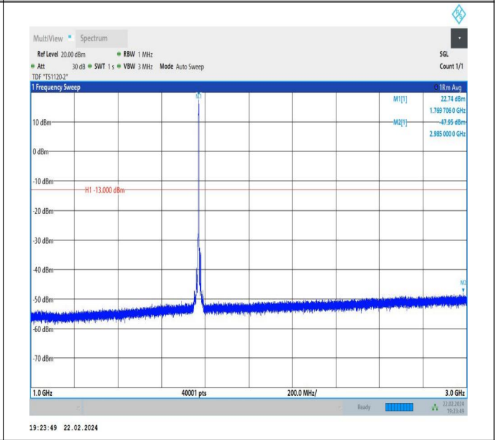
66-66-5MHz-10MHz-QPSK-QPSK-132550-132622-1RB#24-0 RB#0-1000~3000MHz-PASS
