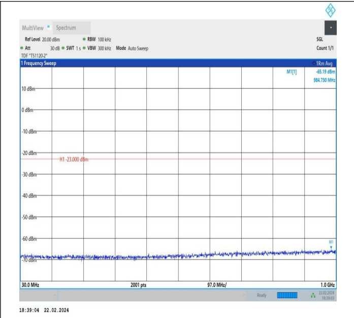
66-66-5MHz-5MHz-QPSK-QPSK-132398-132446-1RB#0-ORB #0-30~1000MHz-PASS
