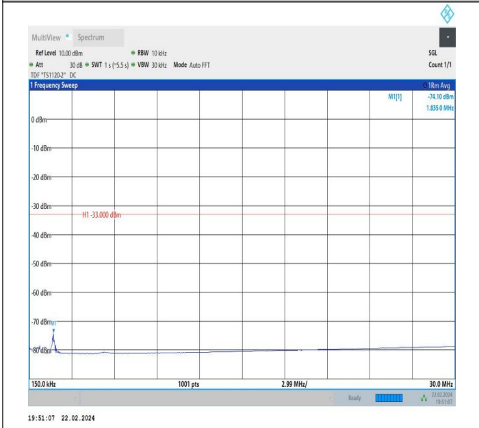
66-66-10MHz-5MHz-QPSK-QPSK-132397-132469-1RB#0-0R B#0-0.15~30MHz-PASS
