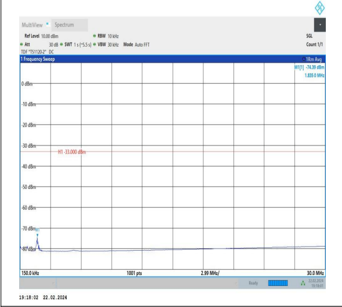
66-66-5MHz-10MHz-QPSK-QPSK-132000-132072-1RB#0-0R B#0-0.15~30MHz-PASS
