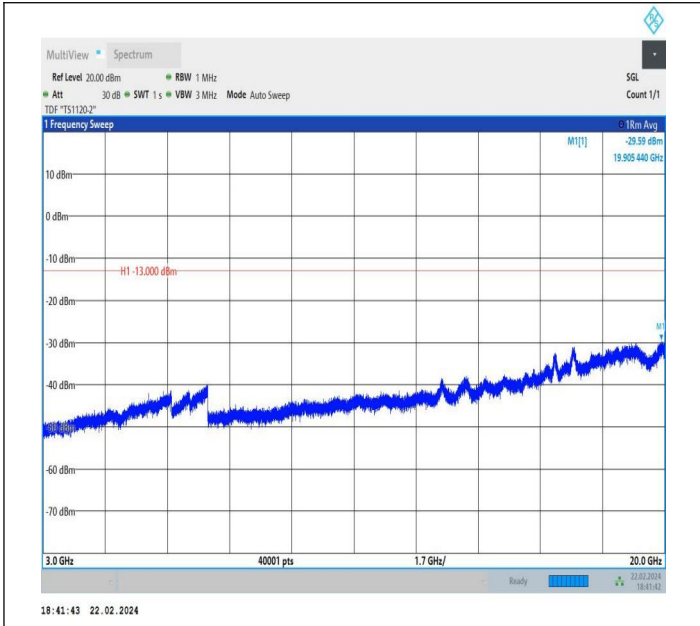
66-66-5MHz-5MHz-QPSK-QPSK-132398-132446-1RB#24-0R B#0-3000~20000MHz-PASS
