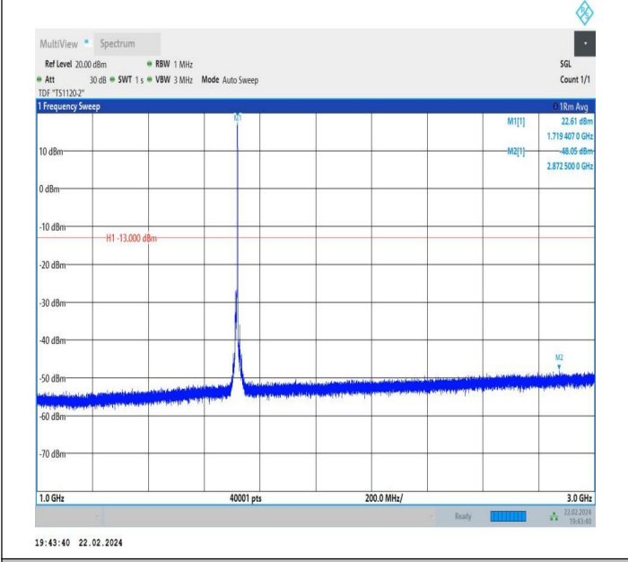
66-66-10MHz-5MHz-QPSK-QPSK-132022-132094-1RB#49-0 RB#0-1000~3000MHz-PASS
