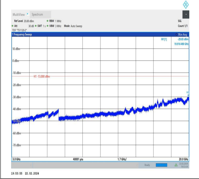
66-66-10MHz-5MHz-QPSK-QPSK-132397-132469-1RB#49-0 RB#0-3000~20000MHz-PASS
