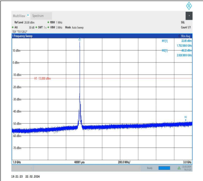
66-66-5MHz-10MHz-QPSK-QPSK-132375-132447-1RB#24-0 RB#0-1000~3000MHz-PASS
