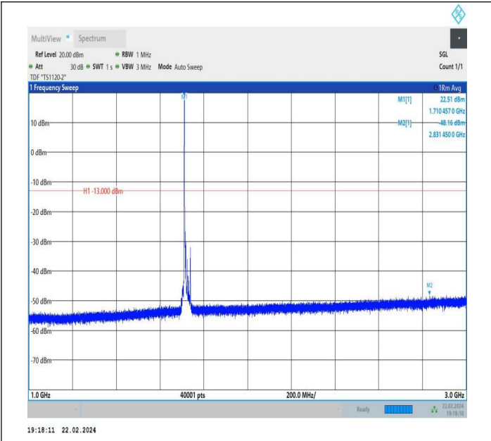
66-66-5MHz-10MHz-QPSK-QPSK-132000-132072-1RB#0-0R B#0-1000~3000MHz-PASS
