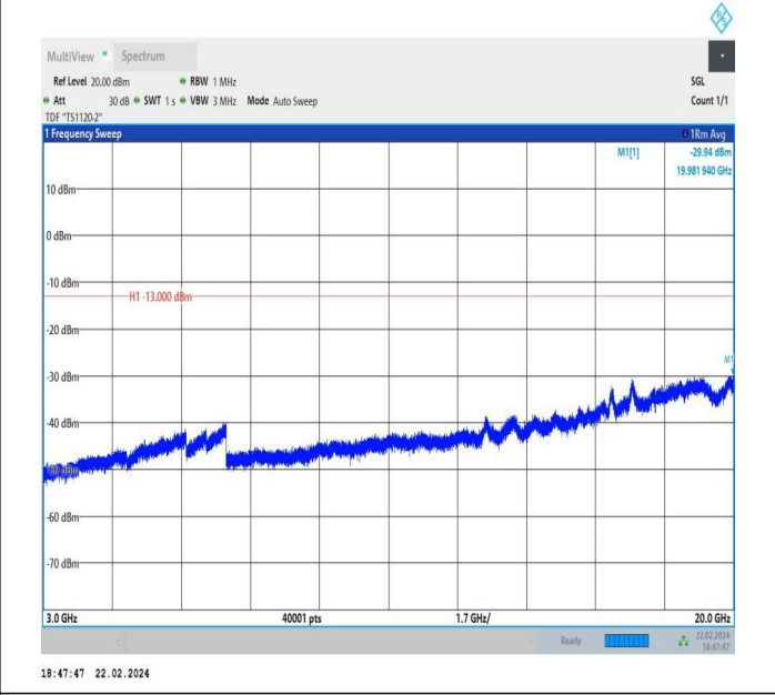
66-66-5MHz-5MHz-QPSK-QPSK-132599-132647-1RB#24-0R B#0-3000~20000MHz-PASS
