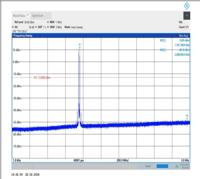
66-66-5MHz-10MHz-QPSK-QPSK-132375-132447-1RB#0-1R B#49-1000~3000MHz-PASS
