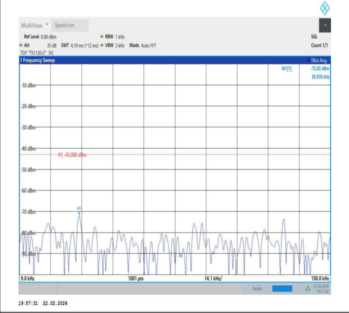
66-66-10MHz-5MHz-QPSK-QPSK-132397-132469-1RB#0-1R B#24-0.009~0.15MHz-PASS
