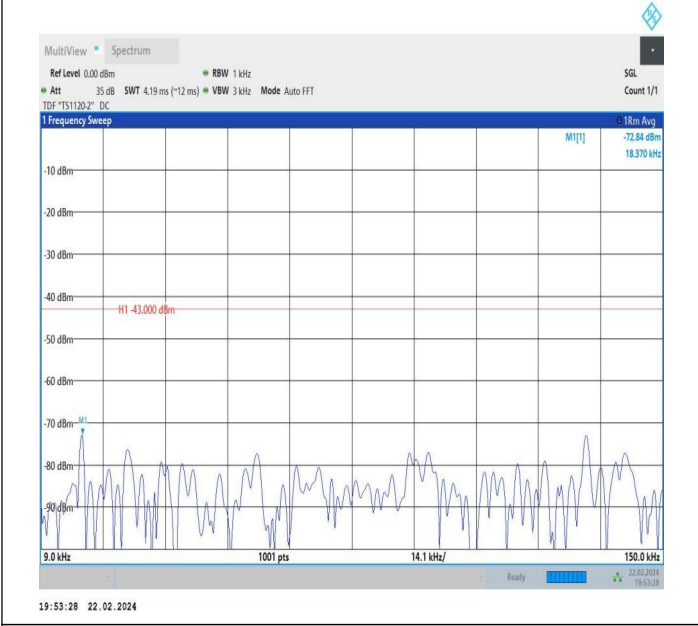
66-66-10MHz-5MHz-QPSK-QPSK-132397-132469-1RB#49-0 RB#0-0.009~0.15MHz-PASS
