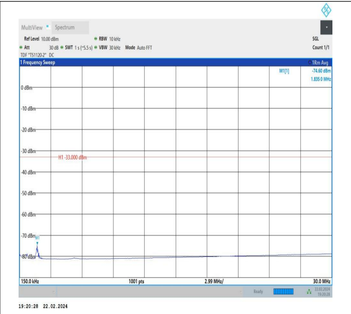
66-66-5MHz-10MHz-QPSK-QPSK-132375-132447-1RB#0-0R B#0-0.15~30MHz-PASS
