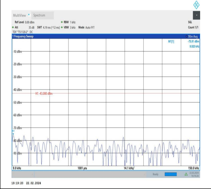
66-66-5MHz-10MHz-QPSK-QPSK-132000-132072-1RB#0-1R B#49-0.009~0.15MHz-PASS
