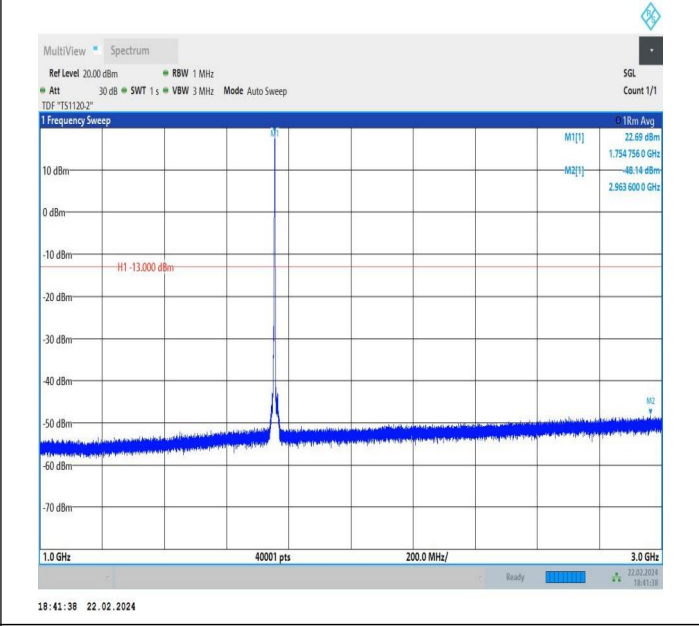
66-66-5MHz-5MHz-QPSK-QPSK-132398-132446-1RB#24-0R B#0-1000~3000MHz-PASS
