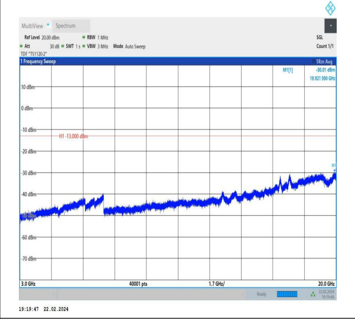
66-66-5MHz-10MHz-QPSK-QPSK-132000-132072-1RB#0-1R B#49-3000~20000MHz-PASS
