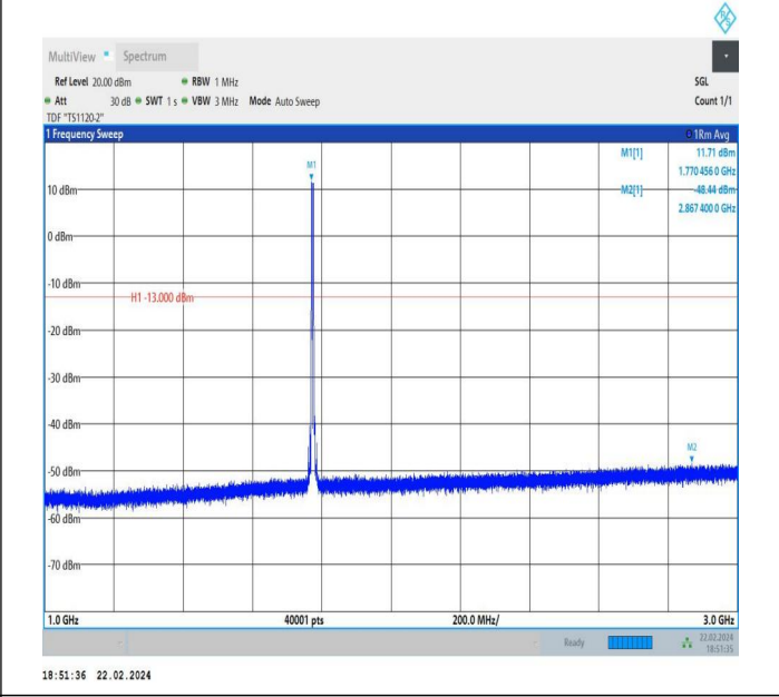
66-66-5MHz-5MHz-QPSK-QPSK-132599-132647-1RB#0-1RB #15-1000~3000MHz-PASS
