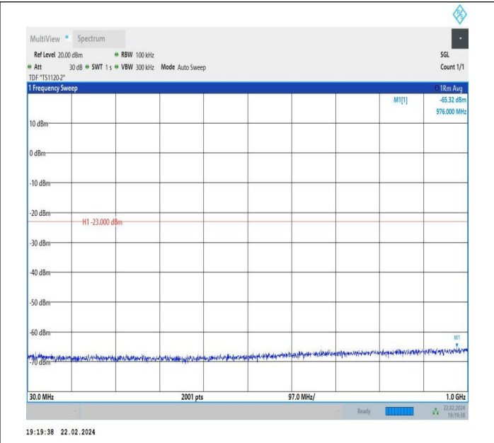
66-66-5MHz-10MHz-QPSK-QPSK-132000-132072-1RB#0-1R B#49-30~1000MHz-PASS
