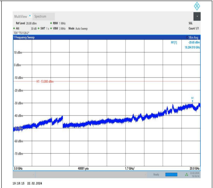
66-66-5MHz-10MHz-QPSK-QPSK-132000-132072-1RB#0-0R B#0-3000~20000MHz-PASS
