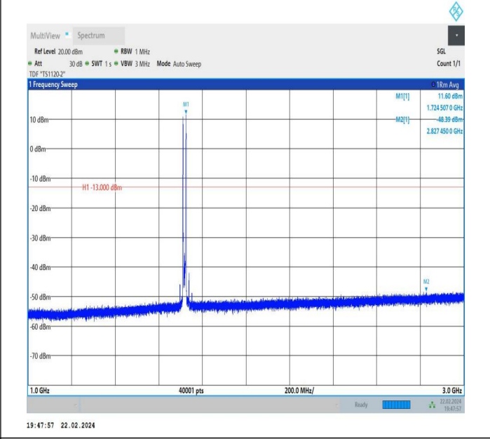
66-66-10MHz-5MHz-QPSK-QPSK-132022-132094-1RB#0-1R B#24-1000~3000MHz-PASS
