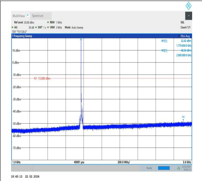
66-66-5MHz-5MHz-QPSK-QPSK-132599-132647-1RB#0-ORB #0-1000~3000MHz-PASS
