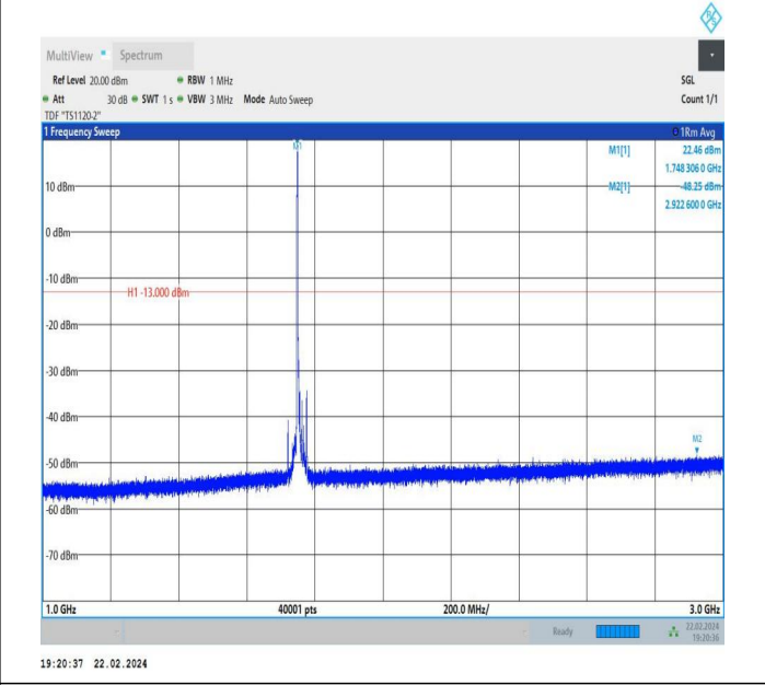
66-66-5MHz-10MHz-QPSK-QPSK-132375-132447-1RB#0-0R B#0-1000~3000MHz-PASS
