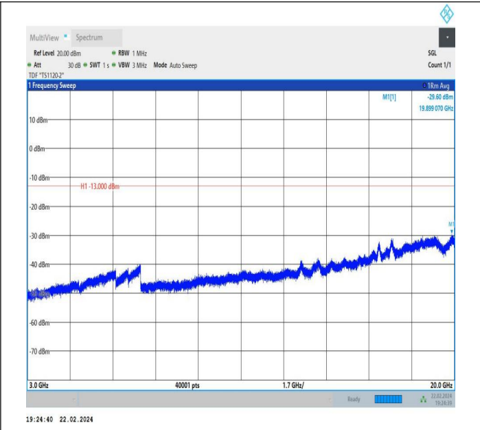
66-66-5MHz-10MHz-QPSK-QPSK-132550-132622-1RB#0-1R B#49-3000~20000MHz-PASS
