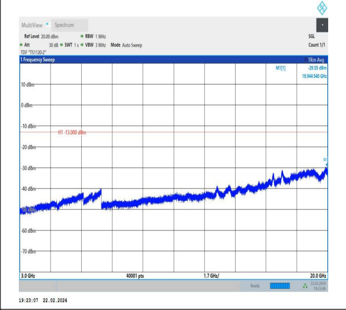
66-66-5MHz-10MHz-QPSK-QPSK-132550-132622-1RB#0-0R B#0-3000~20000MHz-PASS
