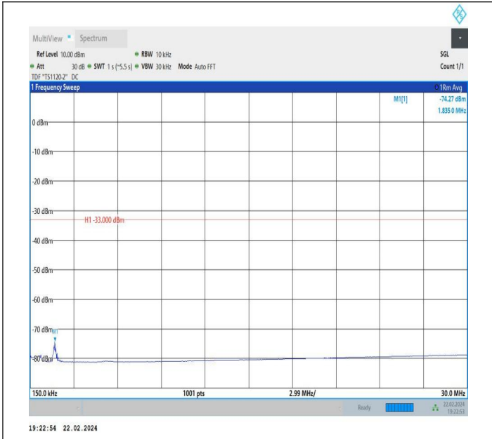
66-66-5MHz-10MHz-QPSK-QPSK-132550-132622-1RB#0-0R B#0-0.15~30MHz-PASS
