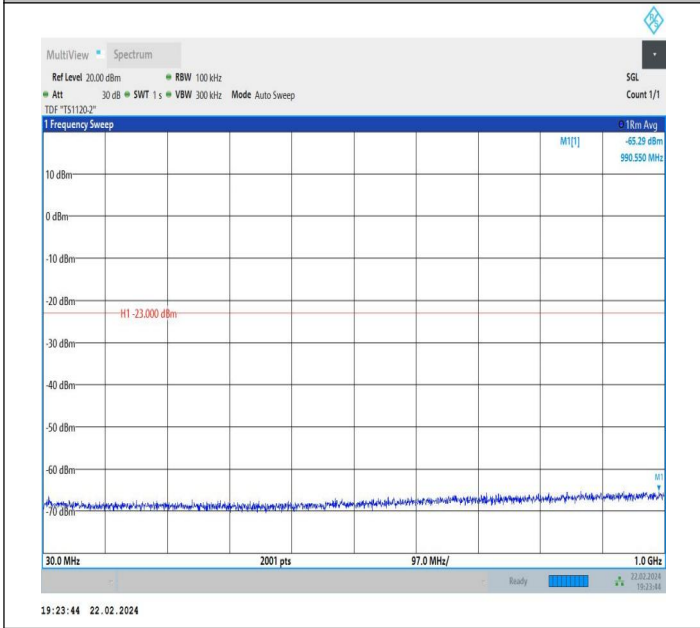
66-66-5MHz-10MHz-QPSK-QPSK-132550-132622-1RB#24-0 RB#0-30~1000MHz-PASS
