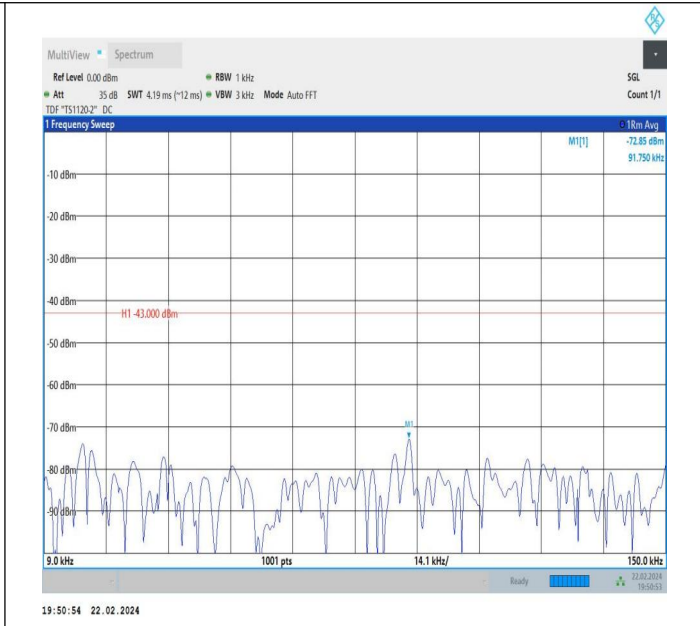
66-66-10MHz-5MHz-QPSK-QPSK-132397-132469-1RB#0-0R B#0-0.009~0.15MHz-PASS
