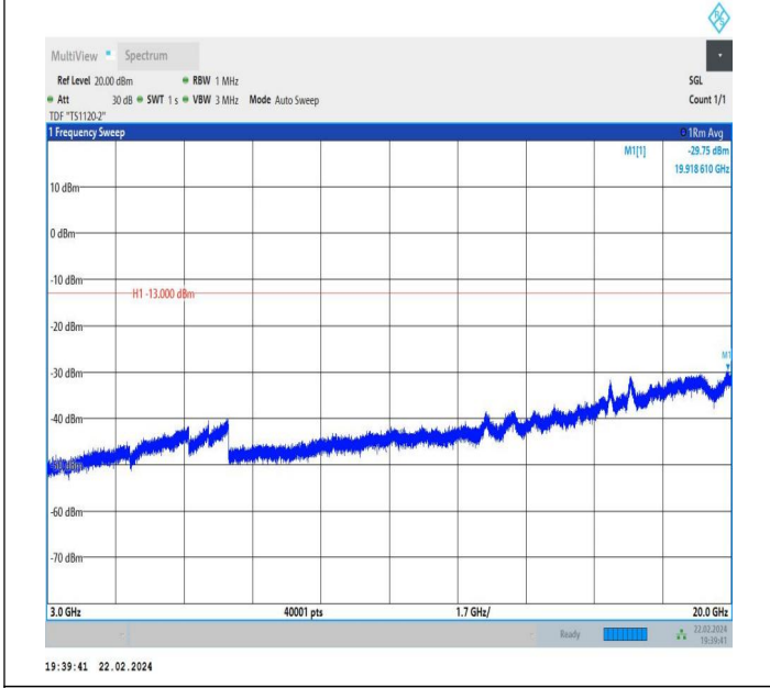
66-66-10MHz-5MHz-QPSK-QPSK-132022-132094-1RB#0-0R B#0-3000~20000MHz-PASS
