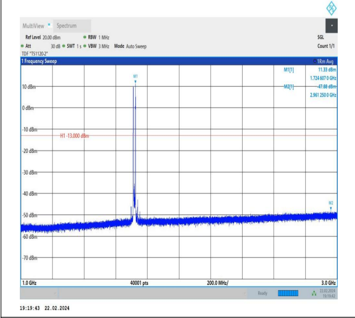
66-66-5MHz-10MHz-QPSK-QPSK-132000-132072-1RB#0-1R B#49-1000~3000MHz-PASS
