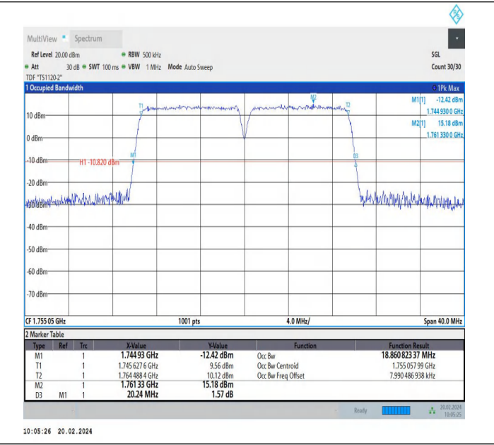
66-66-10MHz-10MHz-16QAM-16QAM-132373-132472-50RB#0-50RB#0-PASS
