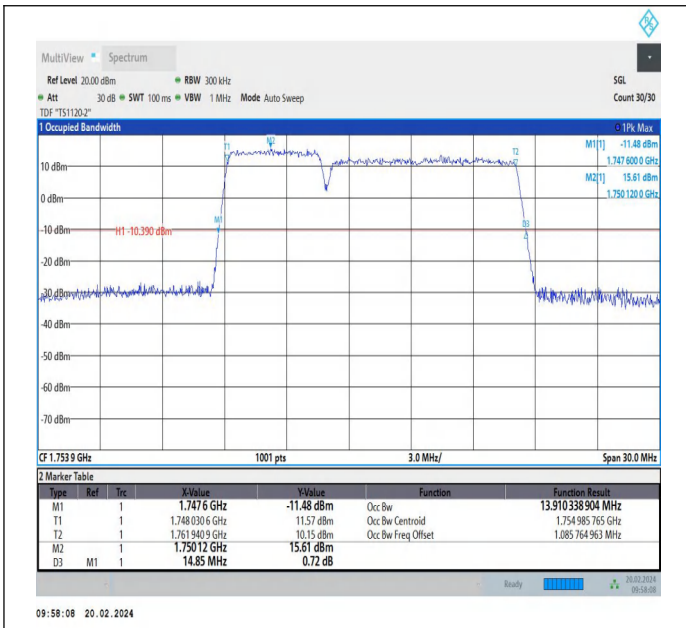
66-66-5MHz-10MHz-QPSK-QPSK-132375-132447-25RB#0-5 ORB#0-PASS
