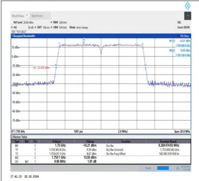
66-66-5MHz-5MHz-QPSK-QPSK-132398-132446-25RB#0-25 RB#0-PASS
