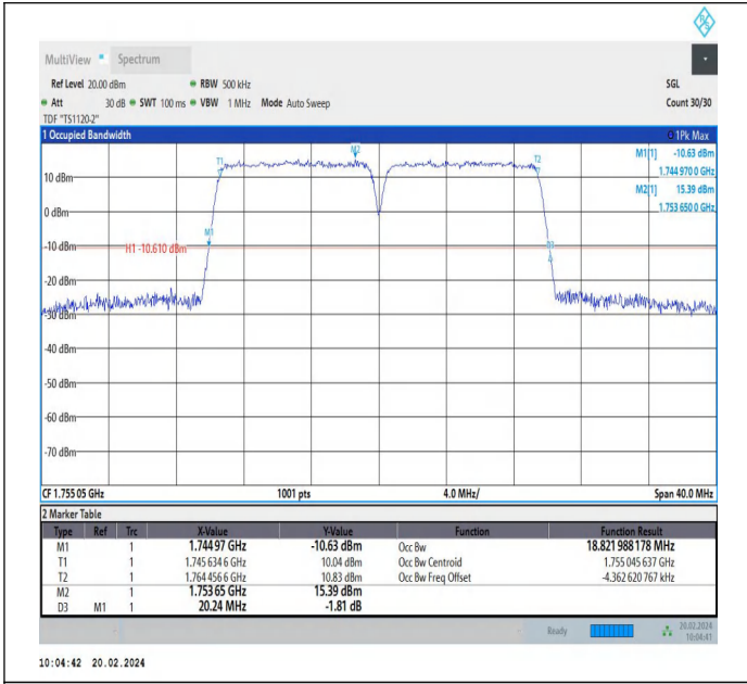
66-66-10MHz-10MHz-QPSK-QPSK-132373-132472-50RB#0-50RB#0-PASS
