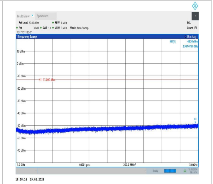
5-5-10MHz-5MHz-QPSK-QPSK-20500-20572-1RB#0-0RB#0-1 000~3000MHz-PASS
