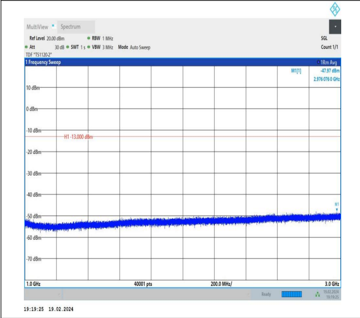
5-5-10MHz-10MHz-QPSK-QPSK-20476-20575-1RB#0-0RB#0-1000~3000MHz-PASS
