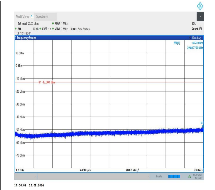
5-5-5MHz-10MHz-QPSK-QPSK-20528-20600-1RB#24-0RB#0-1000~3000MHz-PASS
