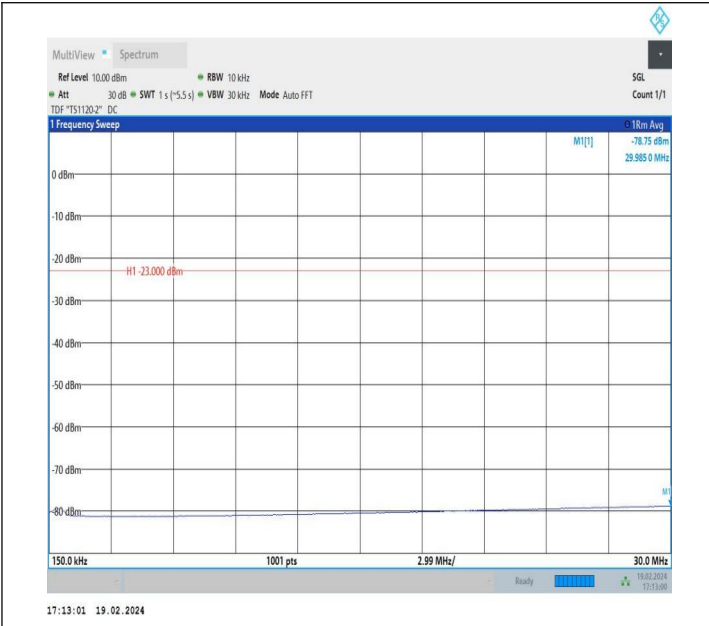
5-5-5MHz-3MHz-QPSK-QPSK-20425-20464-1RB#0-1RB#15-0. 15~30MHz-PASS
