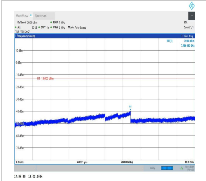
5-5-5MHz-10MHz-QPSK-QPSK-20528-20600-1RB#0-0RB#0-3 000~10000MHz-PASS
