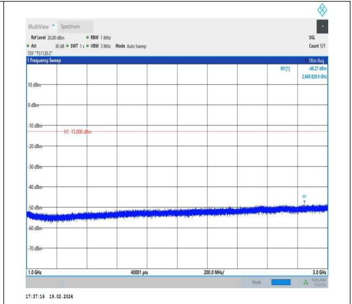
5-5-5MHz-10MHz-QPSK-QPSK-20428-20500-1RB#0-0RB#0-1 000~3000MHz-PASS
