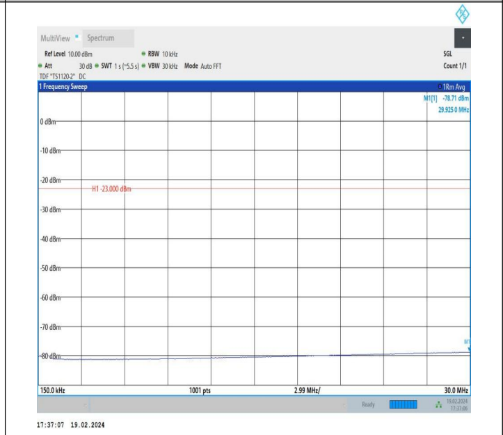
5-5-5MHz-10MHz-QPSK-QPSK-20428-20500-1RB#0-0RB#0-0. 15~30MHz-PASS
