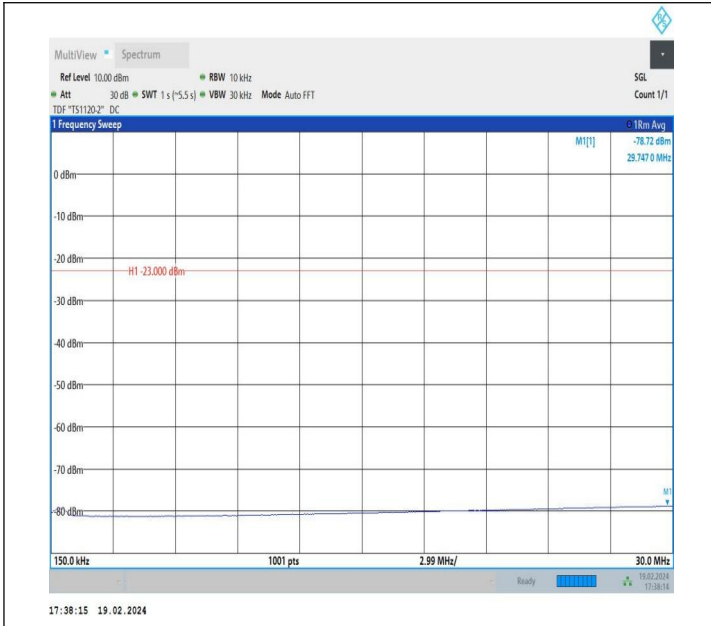
5-5-5MHz-10MHz-QPSK-QPSK-20428-20500-1RB#24-0RB#0- 0.15~30MHz-PASS
