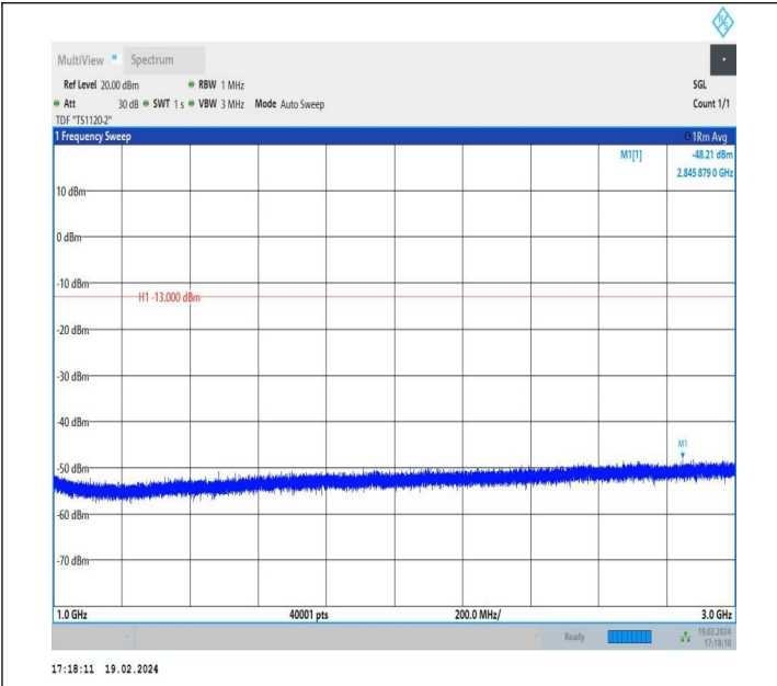
5-5-5MHz-3MHz-QPSK-QPSK-20595-20634-1RB#0-1RB#15-1 000~3000MHz-PASS
