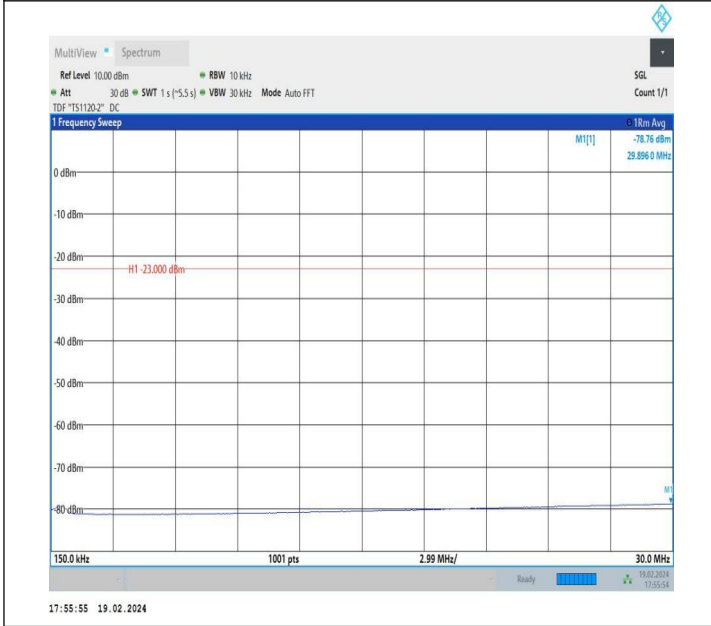
5-5-5MHz-10MHz-QPSK-QPSK-20528-20600-1RB#24-0RB#0- 0.15~30MHz-PASS
