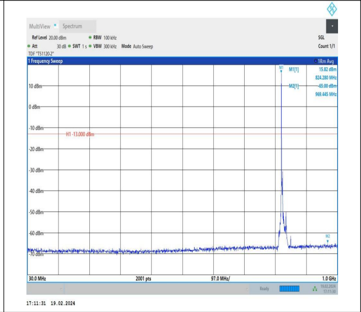
5-5-5MHz-3MHz-QPSK-QPSK-20425-20464-1RB#0-0RB#0-30 ~1000MHz-PASS
