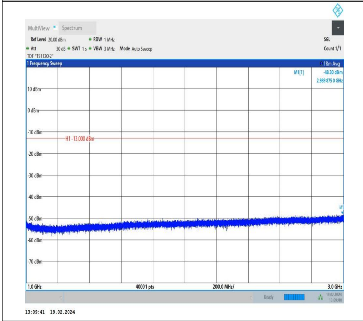
5-5-3MHz-5MHz-QPSK-QPSK-20501-20540-1RB#0-0RB#0-10 00~3000MHz-PASS
