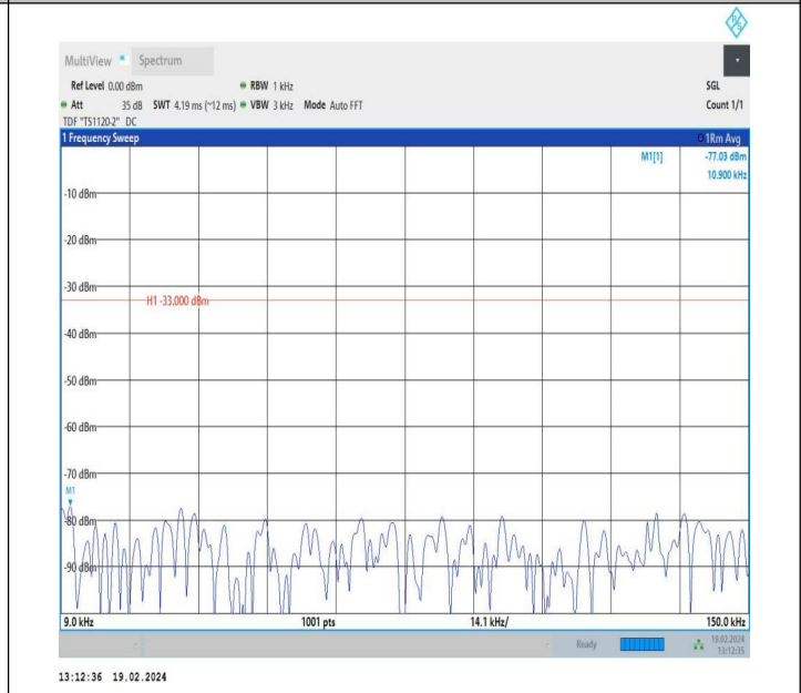
5-5-3MHz-5MHz-QPSK-QPSK-20586-20625-1RB#14-0RB#0-0. 009~0.15MHz-PASS
