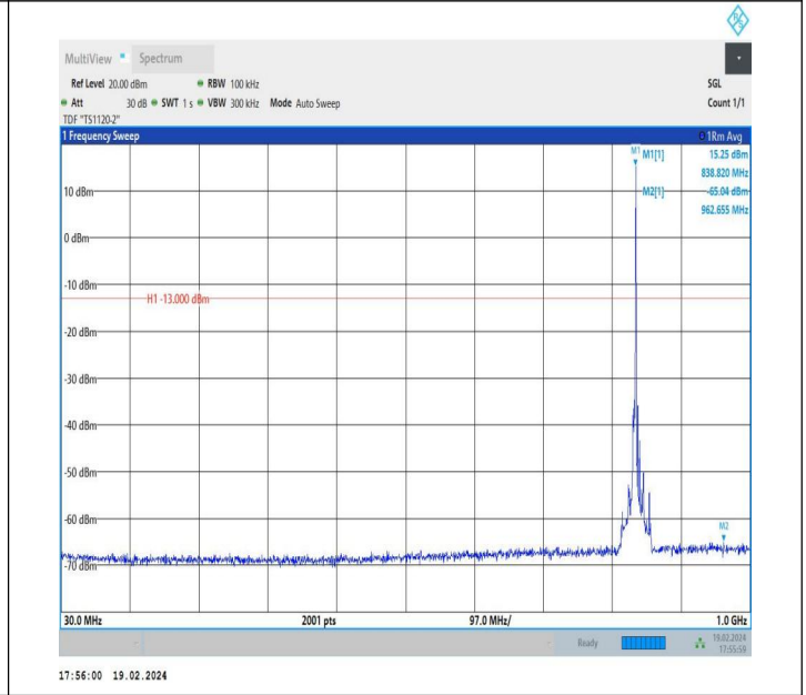
5-5-5MHz-10MHz-QPSK-QPSK-20528-20600-1RB#24-0RB#0- 30~1000MHz-PASS
