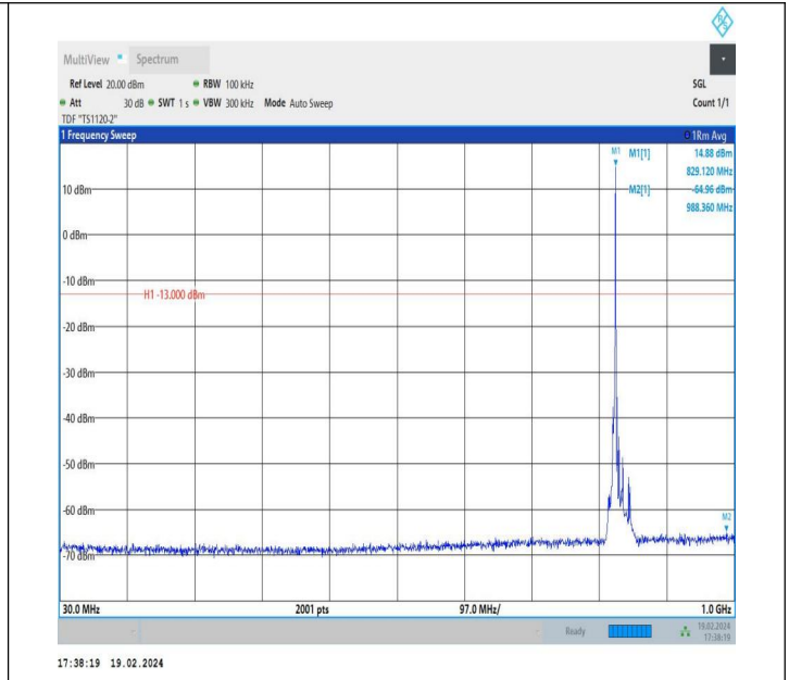
5-5-5MHz-10MHz-QPSK-QPSK-20428-20500-1RB#24-0RB#0- 30~1000MHz-PASS
