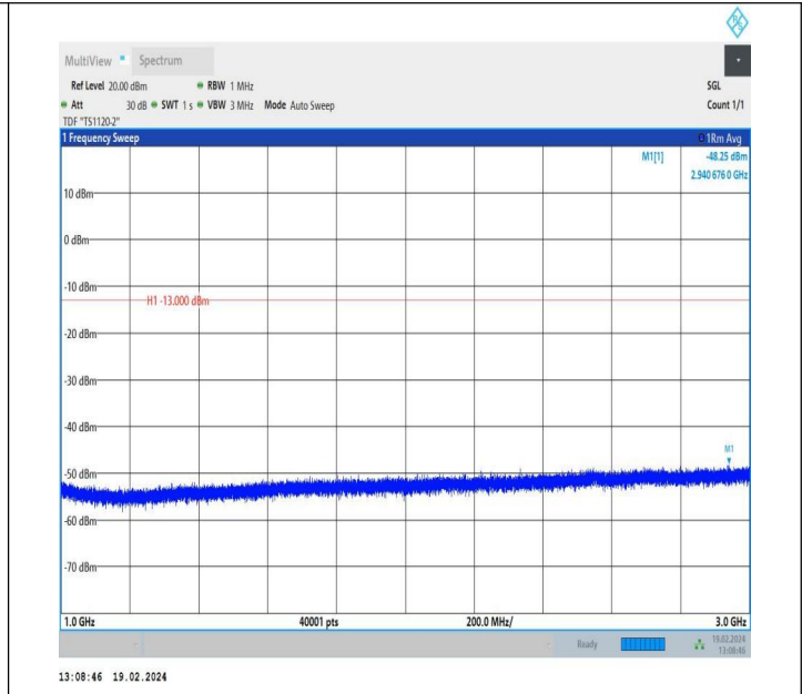
5-5-3MHz-5MHz-QPSK-QPSK-20416-20455-1RB#0-1RB#24-1 000~3000MHz-PASS
