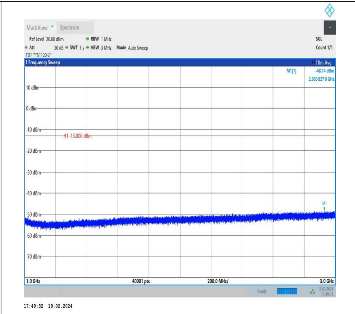
5-5-5MHz-10MHz-QPSK-QPSK-20478-20550-1RB#24-0RB#0-1000~3000MHz-PASS
