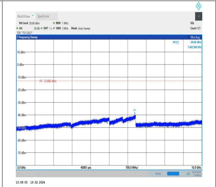
5-5-3MHz-5MHz-QPSK-QPSK-20416-20455-1RB#14-0RB#0-3 000~10000MHz-PASS
