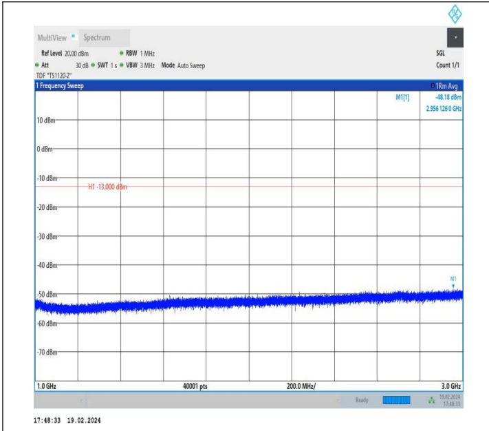
5-5-5MHz-10MHz-QPSK-QPSK-20478-20550-1RB#0-0RB#0-1 000~3000MHz-PASS
