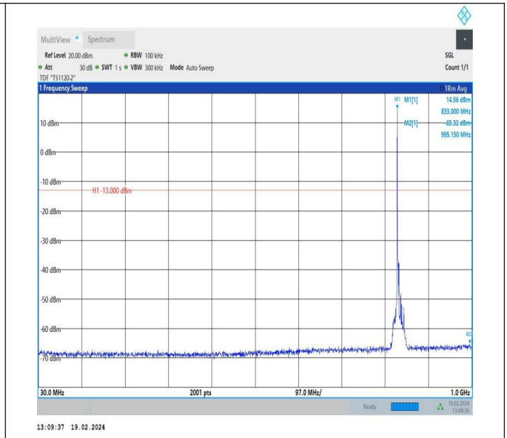
5-5-3MHz-5MHz-QPSK-QPSK-20501-20540-1RB#0-0RB#0-30 ~1000MHz-PASS
