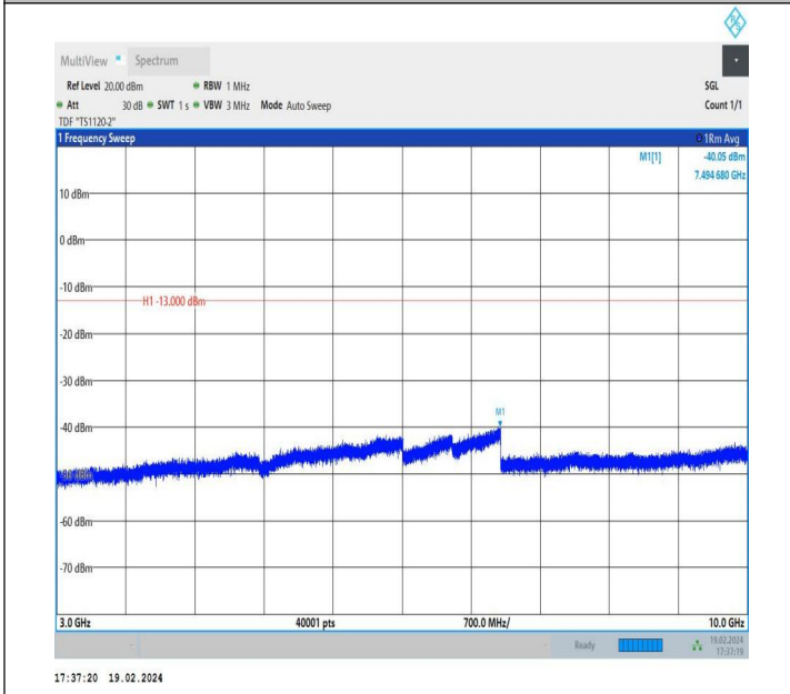
5-5-5MHz-10MHz-QPSK-QPSK-20428-20500-1RB#0-0RB#0-3 000~10000MHz-PASS
