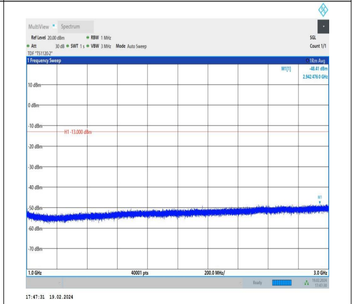
5-5-5MHz-10MHz-QPSK-QPSK-20428-20500-1RB#0-1RB#49- 1000~3000MHz-PASS
