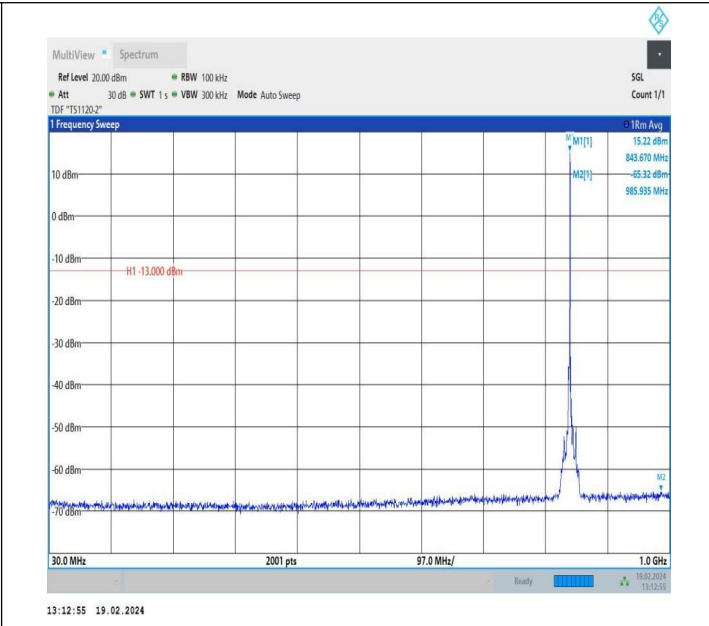
5-5-3MHz-5MHz-QPSK-QPSK-20586-20625-1RB#14-0RB#0-3 0~1000MHz-PASS
