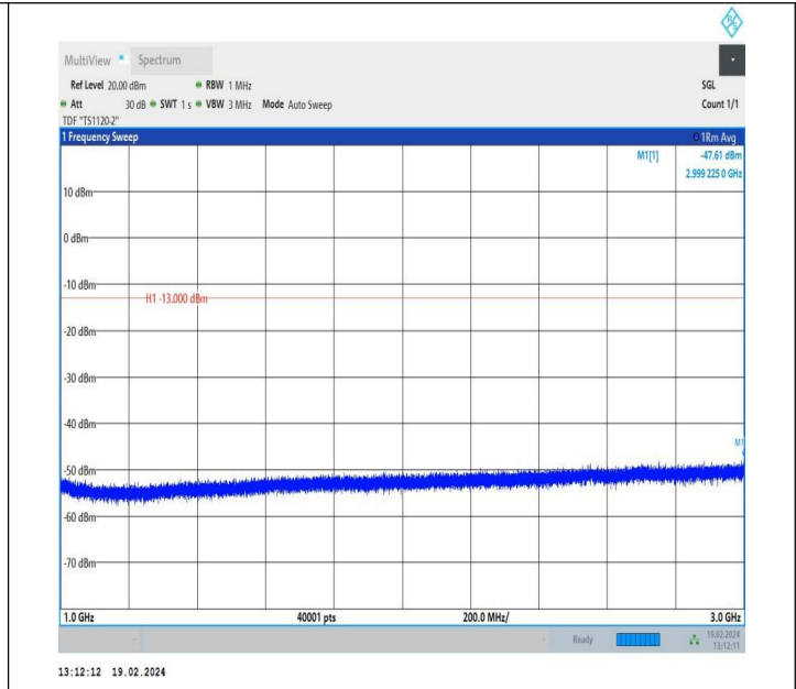
5-5-3MHz-5MHz-QPSK-QPSK-20586-20625-1RB#0-0RB#0-10 00~3000MHz-PASS
