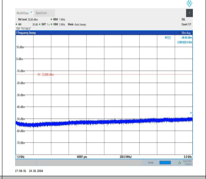
5-5-5MHz-10MHz-QPSK-QPSK-20528-20600-1RB#0-0RB#0-1.000~3000MHz-PASS
