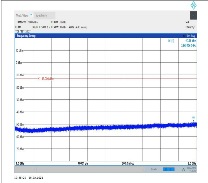
5-5-5MHz-10MHz-QPSK-QPSK-20428-20500-1RB#24-0RB#0- 1000~3000MHz-PASS
