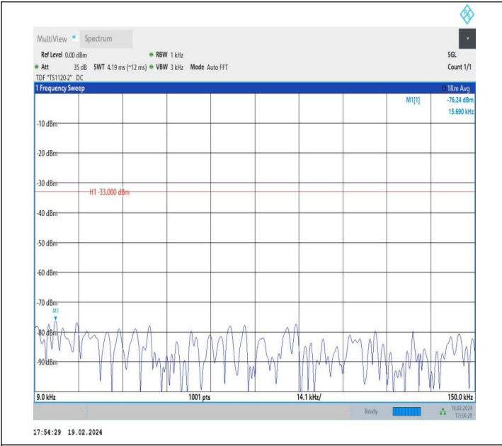
5-5-5MHz-10MHz-QPSK-QPSK-20528-20600-1RB#0-0RB#0-0.009~0.15MHz-PASS
