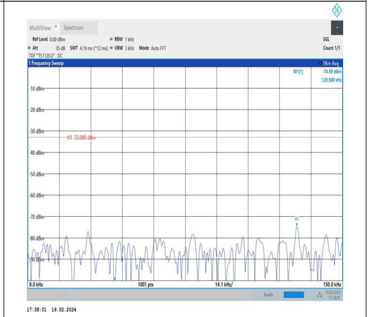
5-5-5MHz-10MHz-QPSK-QPSK-20428-20500-1RB#24-0RB#0- 0.009~0.15MHz-PASS
