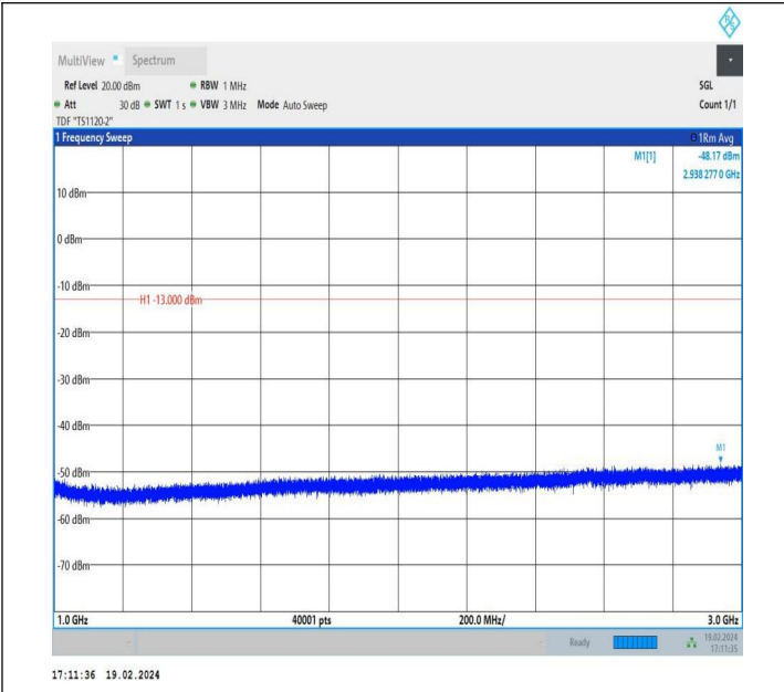
5-5-5MHz-3MHz-QPSK-QPSK-20425-20464-1RB#0-ORB#0-10 00~3000MHz-PASS
