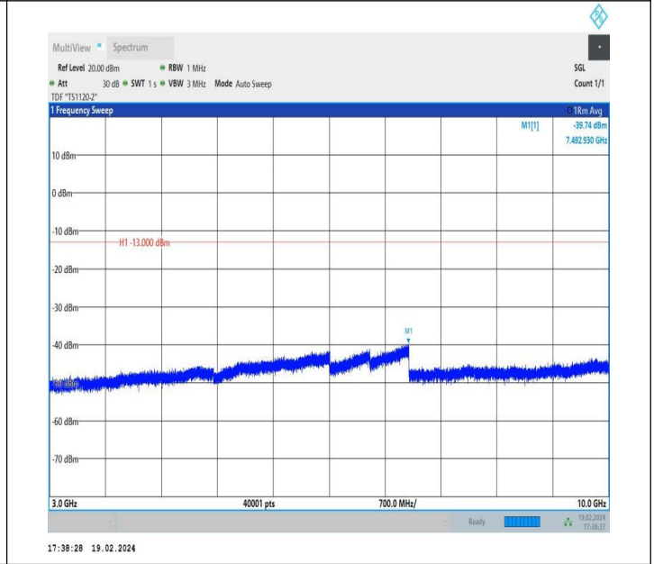
5-5-5MHz-10MHz-QPSK-QPSK-20428-20500-1RB#24-0RB#0- 3000~10000MHz-PASS
