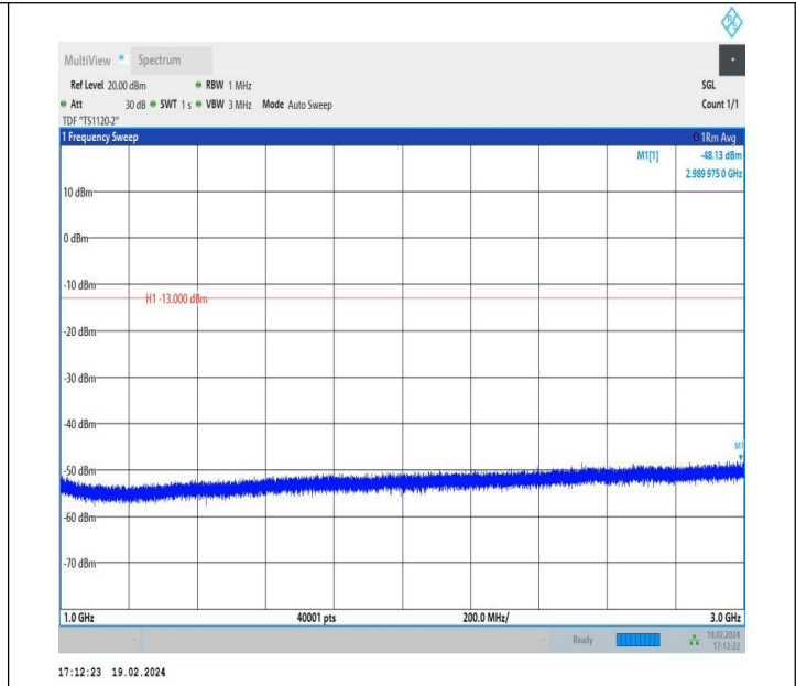
5-5-5MHz-3MHz-QPSK-QPSK-20425-20464-1RB#24-0RB#0-1 000~3000MHz-PASS
