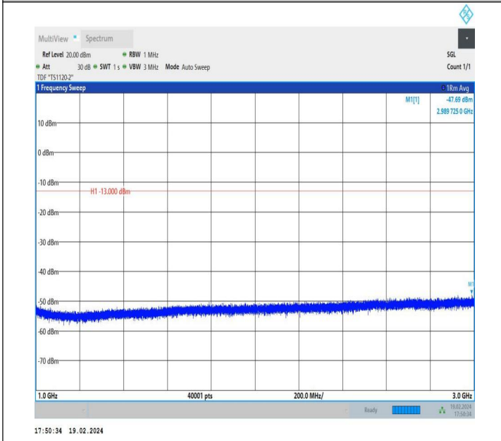
5-5-5MHz-10MHz-QPSK-QPSK-20478-20550-1RB#0-1RB#49- 1000~3000MHz-PASS
