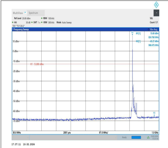
5-5-5MHz-10MHz-QPSK-QPSK-20428-20500-1RB#0-0RB#0-3 0~1000MHz-PASS
