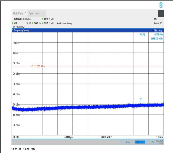
5-5-3MHz-5MHz-QPSK-QPSK-20416-20455-1RB#14-0RB#0-1 000~3000MHz-PASS
