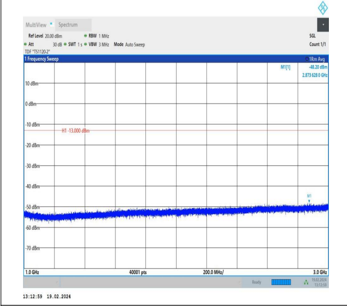
5-5-3MHz-5MHz-QPSK-QPSK-20586-20625-1RB#14-0RB#0-1 000~3000MHz-PASS
