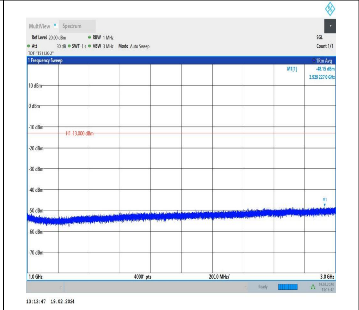
5-5-3MHz-5MHz-QPSK-QPSK-20586-20625-1RB#0-1RB#24-1 000~3000MHz-PASS
