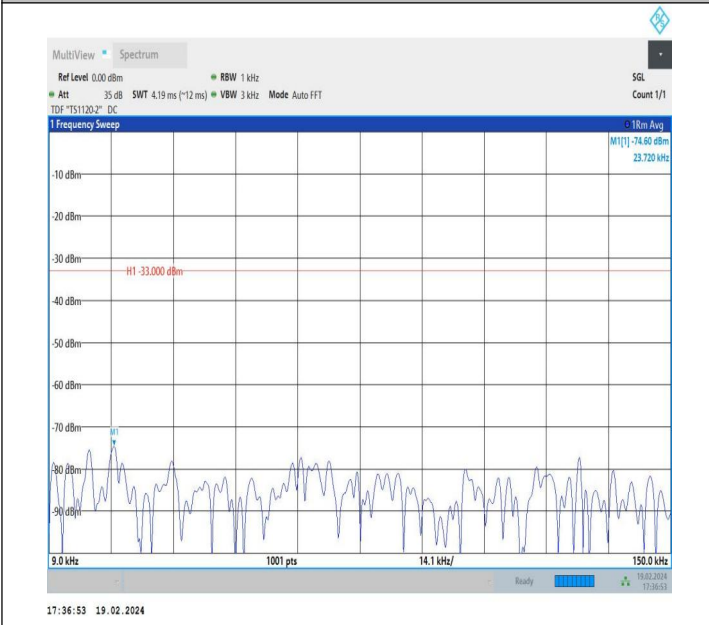
5-5-5MHz-10MHz-QPSK-QPSK-20428-20500-1RB#0-0RB#0-0. 009~0.15MHz-PASS
