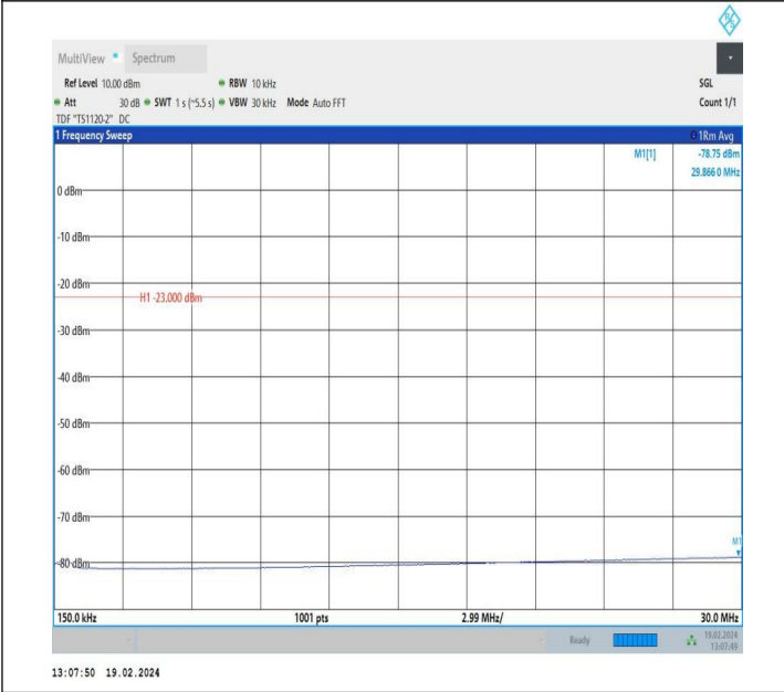
5-5-3MHz-5MHz-QPSK-QPSK-20416-20455-1RB#14-0RB#0-0. 15~30MHz-PASS
