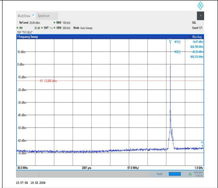
5-5-3MHz-5MHz-QPSK-QPSK-20416-20455-1RB#14-0RB#0-3 0~1000MHz-PASS
