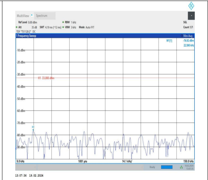
5-5-3MHz-5MHz-QPSK-QPSK-20416-20455-1RB#14-0RB#0-0. 009~0.15MHz-PASS
