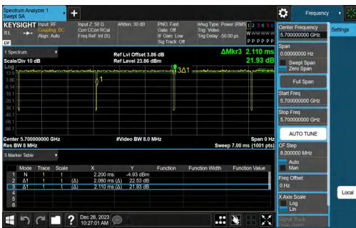
NTNV-11A-Ant0-5720
