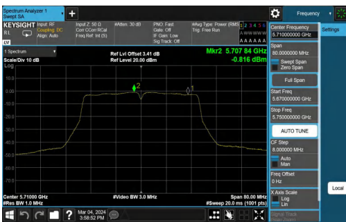
11N40SISO-Ant0-5710_UNII-3-PASS
