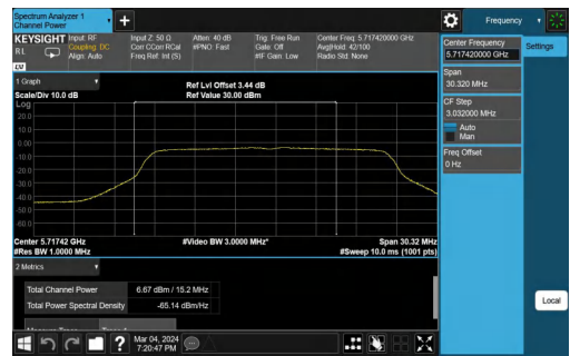
11AC20SISO-Ant1-5720_UNII-3-TPC_H-PASS
