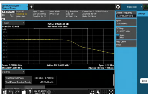
11AC20MIMO-Ant0-5720_UNII-3-TPC_L-PASS
