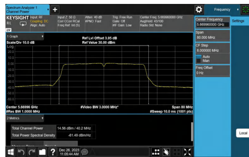
11N40SISO-Ant1-5670-TPC_H-PASS
