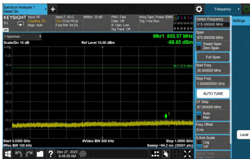
BLE_1M-Ant0-2440-30~1000-PASS
