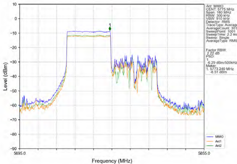
802.11ax(HE80) MCH 5775MHz RU484 Left MIMO NTVN
