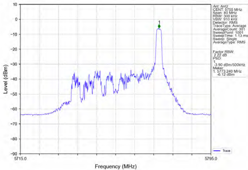
802.11ax(HE40) LCH 5755MHz RU26 Right MIMO NTVN
