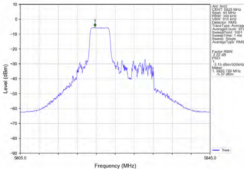
802.11ax(HE20) HCH 5825MHz RU52 Mid Ant2 NTN
