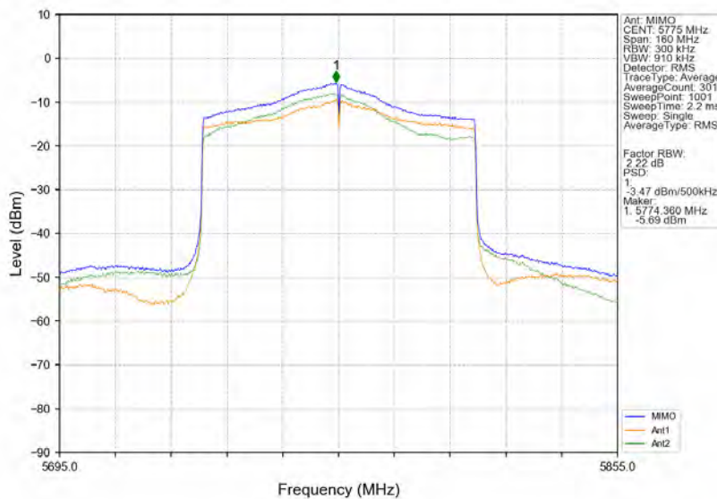
802.11ax(HE80)_MCH_5775MHz_RU996_Left_MIMO_NTNV
