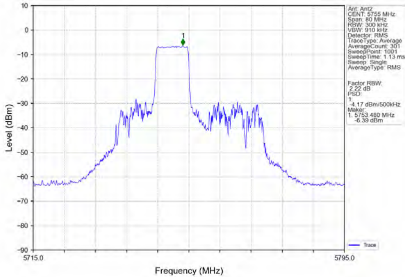
802.11ax(HE40) LCH 5755MHz RU106 Mid Ant2 NTN
