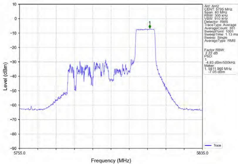
802.11ax(HE40) HCH 5795MHz RU106 Right MIMO NTVN
