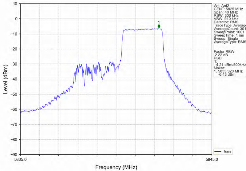
802.11ax(HE20) HCH 5825MHz RU106 Right MIMO NTVN
