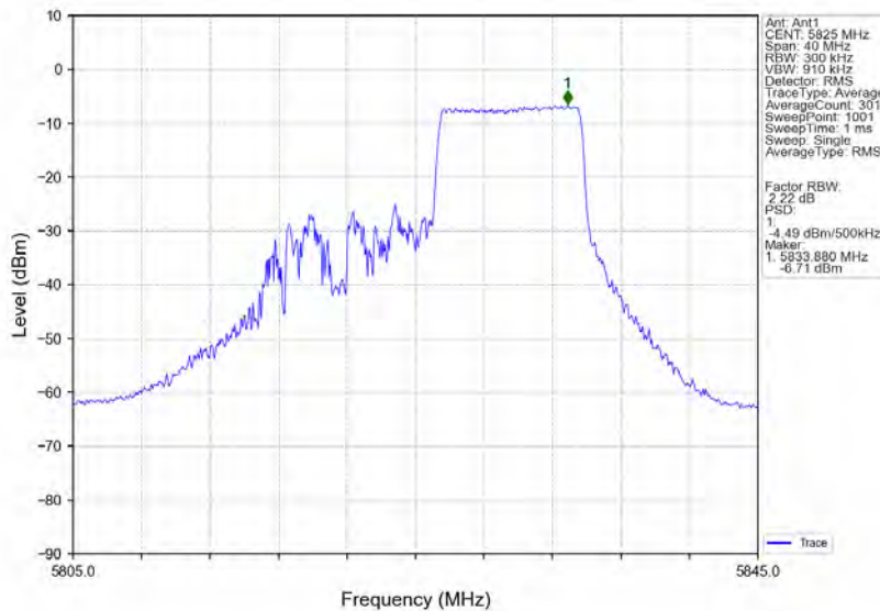
802.11ax(HE20) HCH 5825MHz RU106 Right Ant1 NTV
