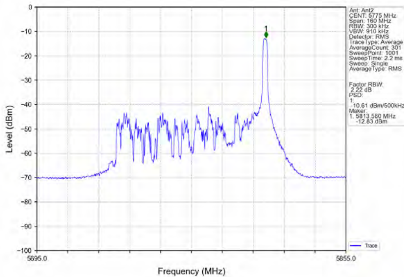
802.11ax(HE80) MCH 5775MHz RU26 Right MIMO NTVN
