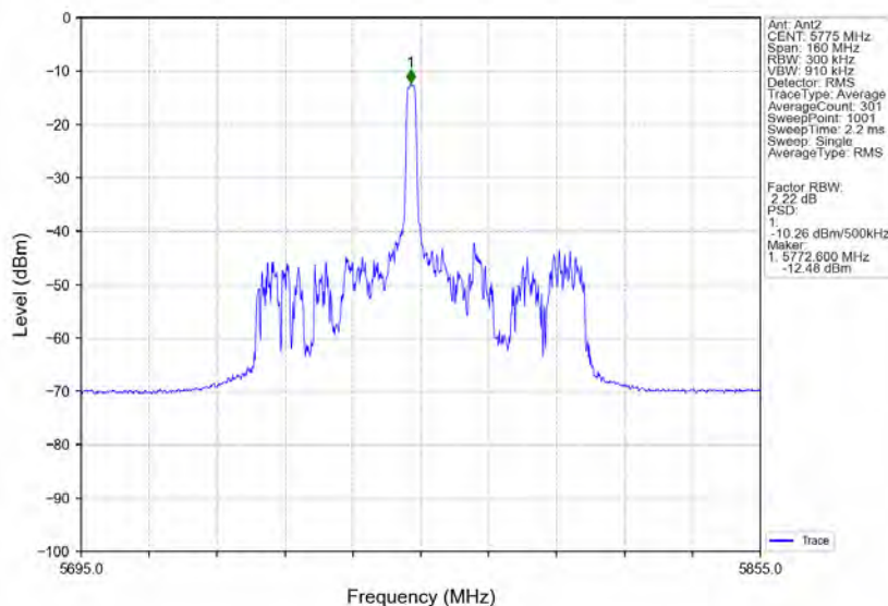
802.11ax(HE80) MCH_5775MHz RU26 Mid Ant2 NTN
