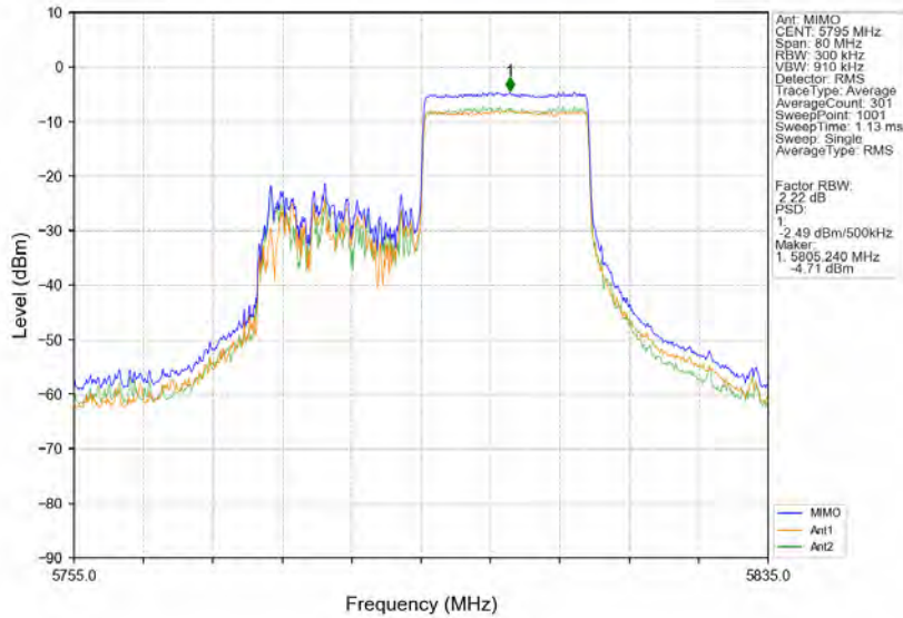
802.11ax(HE40) HCH 5795MHz RU242 Right MIMO NTVN
