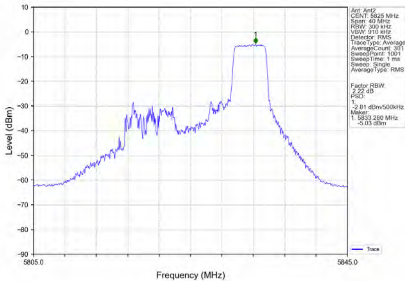
802.11ax(HE20) HCH 5825MHz RU52 Right MIMO NTVN
