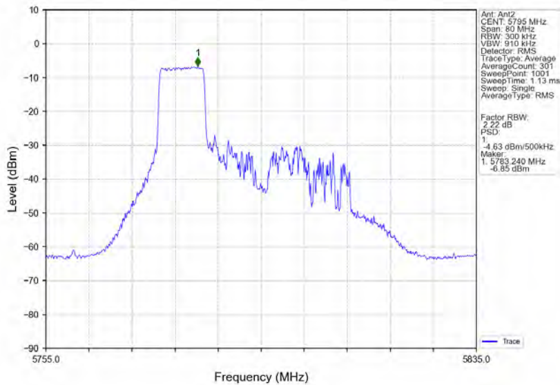
802.11ax(HE40) HCH 5795MHz RU106 Left MIMO NTVN
