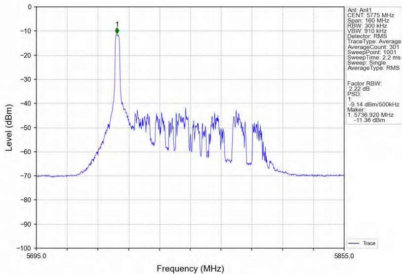
802.11ax(HE80) MCH 5775MHz RU26 Left Ant1 NTN
