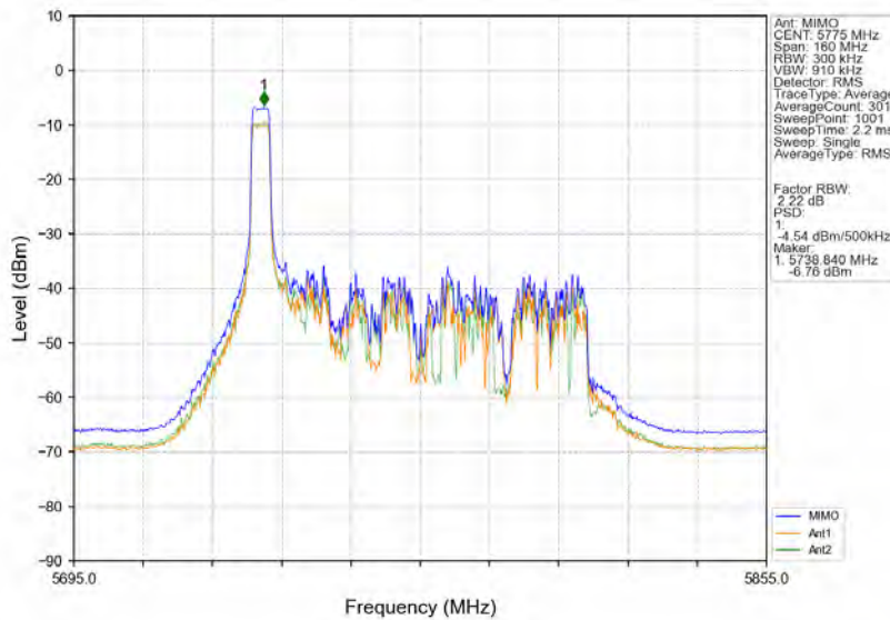
802.11ax(HE80) MCH 5775MHz RU52 Mid Ant1 NTNv
