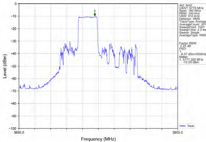
802.11ax(HE80) MCH 5775MHz RU242 Mid MIMO NTVN
