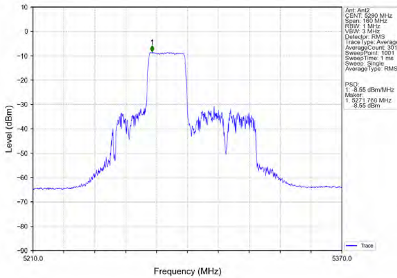
802.11ax(HE80) MCH 5290MHz RU242 Mid MIMO NTVN
