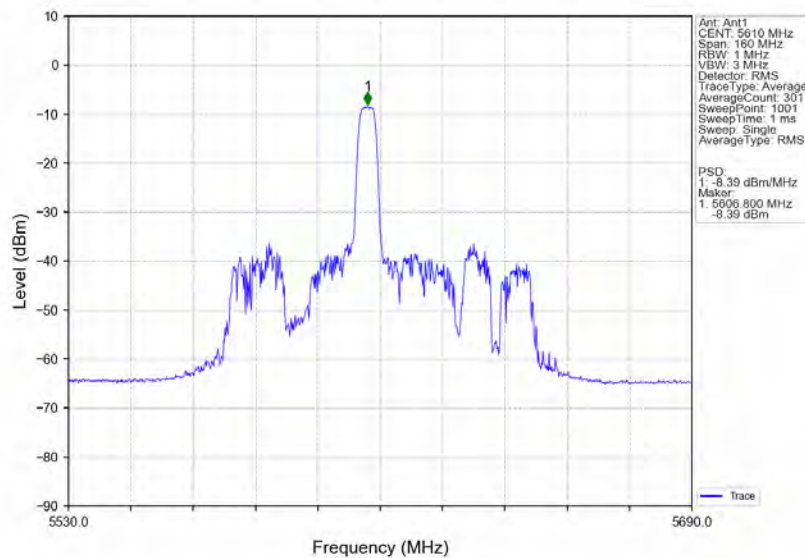
802.11ax(HE80) HCH 5610MHz RU52 Mid Ant1 NTN
