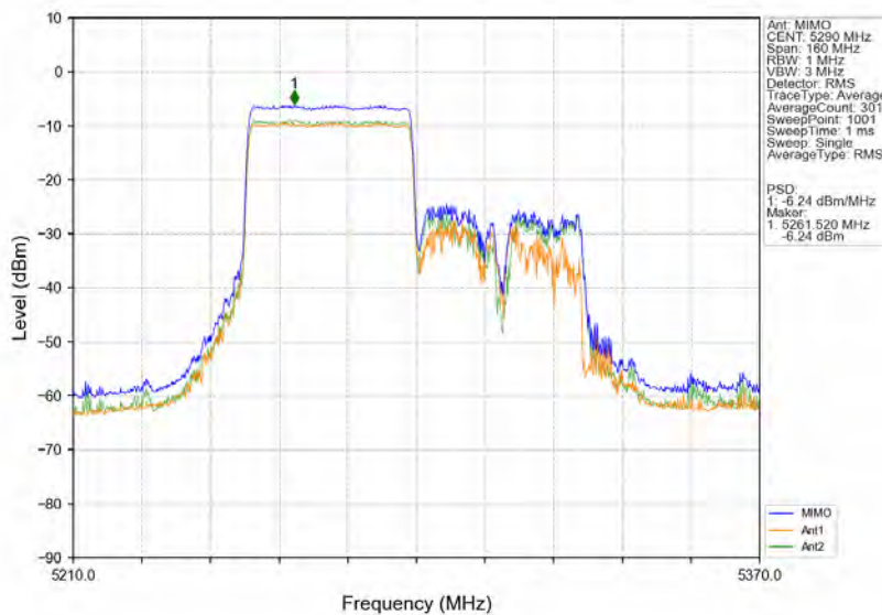
802.11ax(HE80) MCH 5290MHz RU484 Left MIMO NTN
