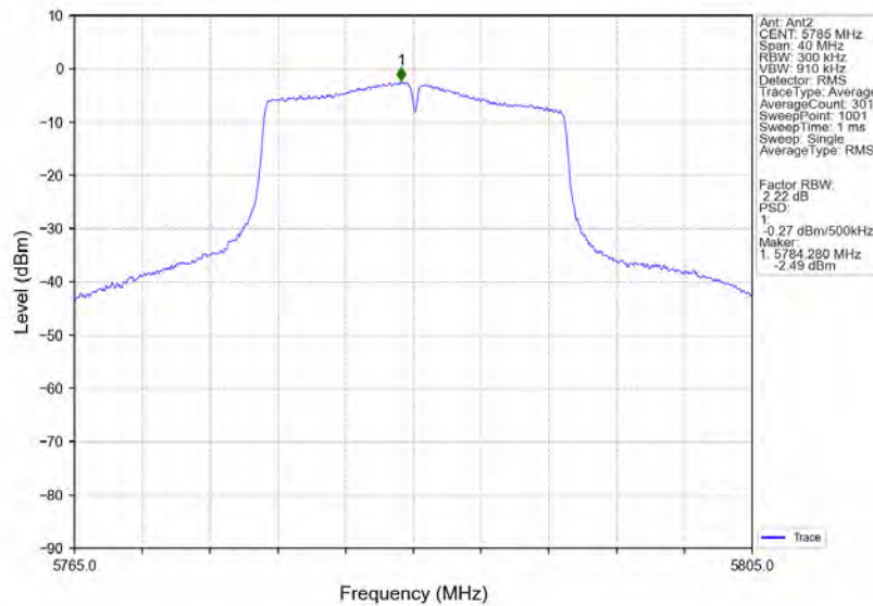
802.11ac(VHT20) MCH 5785MHz MIMO NTV
