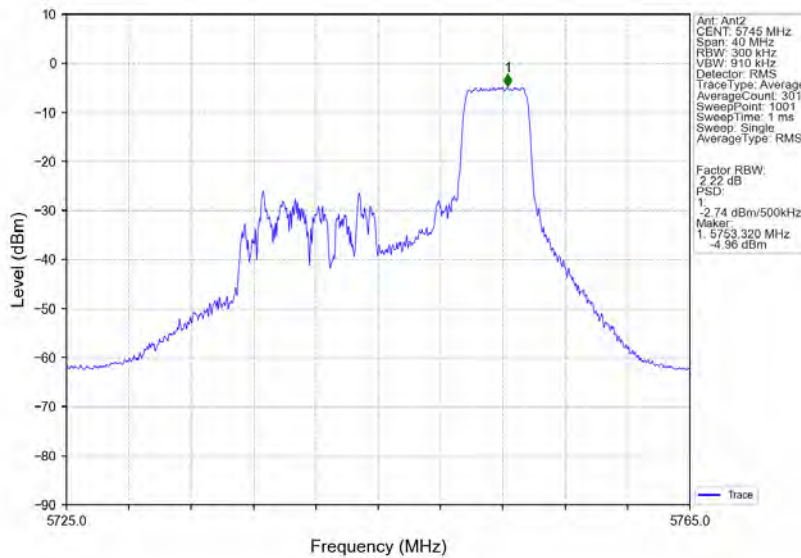
802.11ax(HE20) LCH 5745MHz RU52 Right MIMO NTVN
