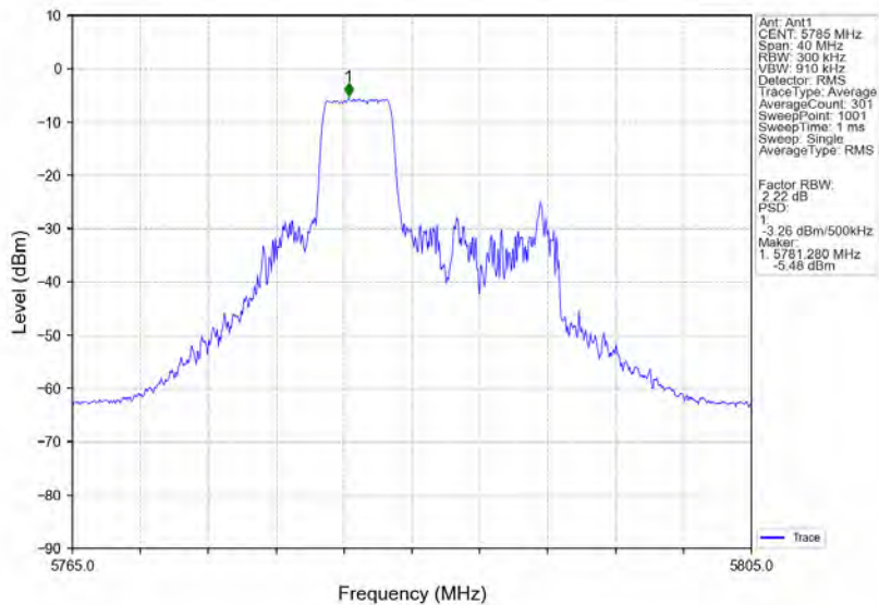
802.11ax(HE20) MCH 5785MHz RU52 Mid Ant1 NTN
