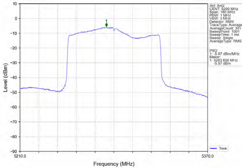
802.11ax(HE80)_MCH_5290MHz_RU996_Left_MIMO_NTNV
