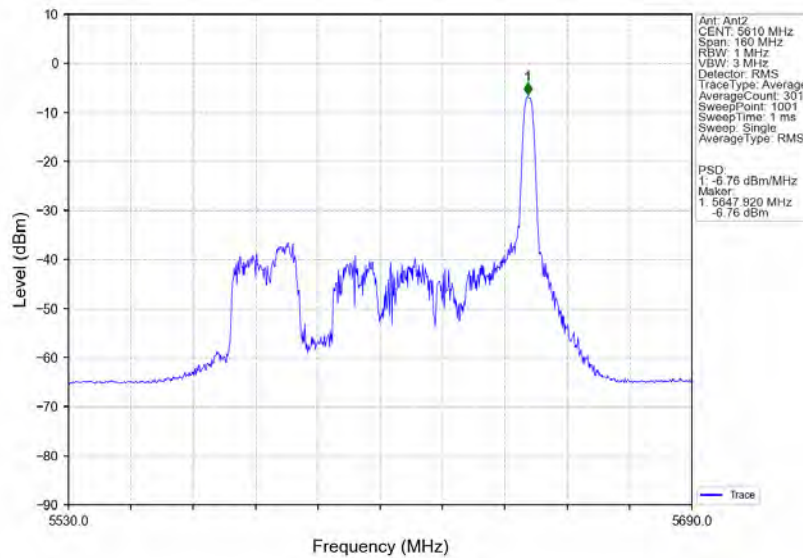
802.11ax(HE80) HCH 5610MHz RU26 Right MIMO NTVN
