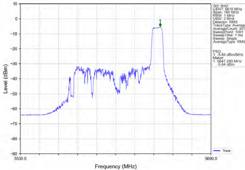
802.11ax(HE80) HCH 5610MHz RU106 Right MIMO NTVN
