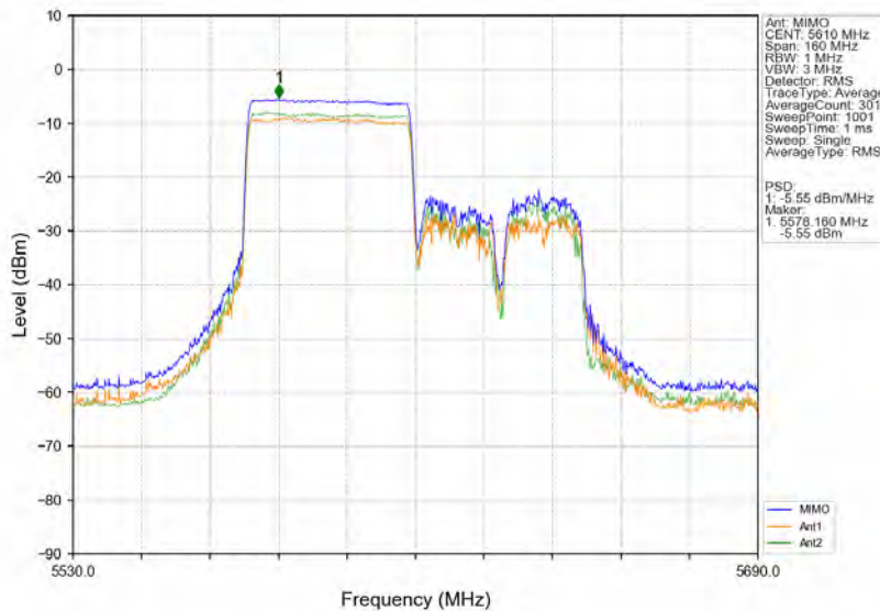
802.11ax(HE80) HCH 5610MHz RU484 Left MIMO NTVN
