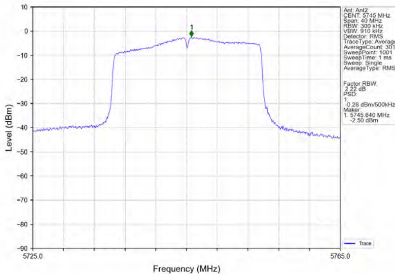
802.11ax(HE20) LCH 5745MHz RU242 Left Ant2 NTN
