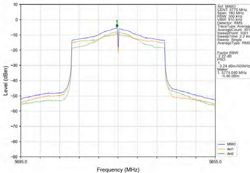
802.11ac(VHT80) MCH 5775MHz MIMO NTV
