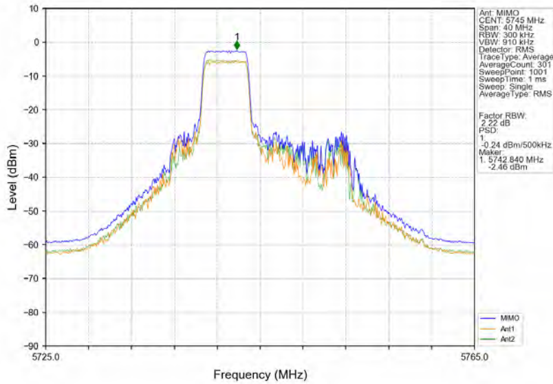
802.11ax(HE20) LCH 5745MHz RU52 Right Ant1 NTN
