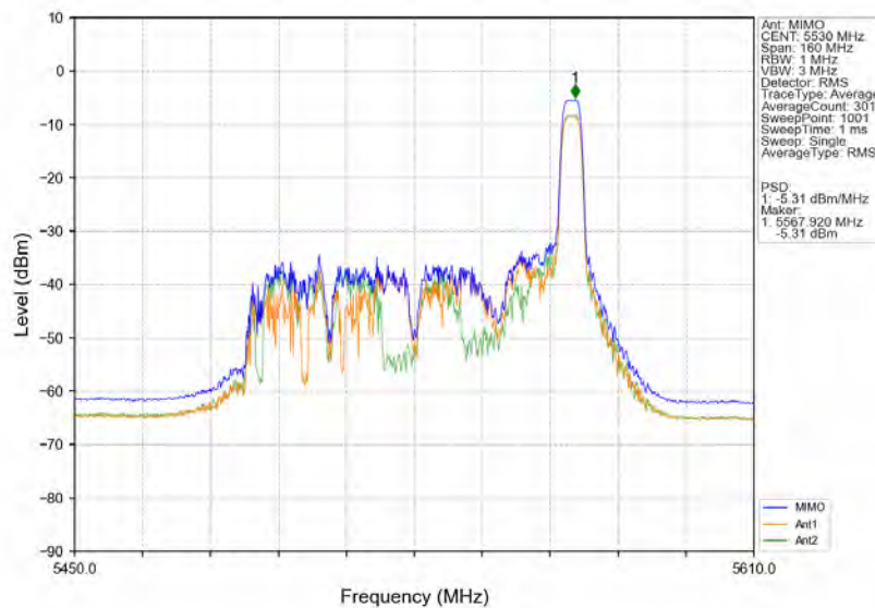
802.11ax(HE80) LCH 5530MHz RU52 Right MIMO NTNv
