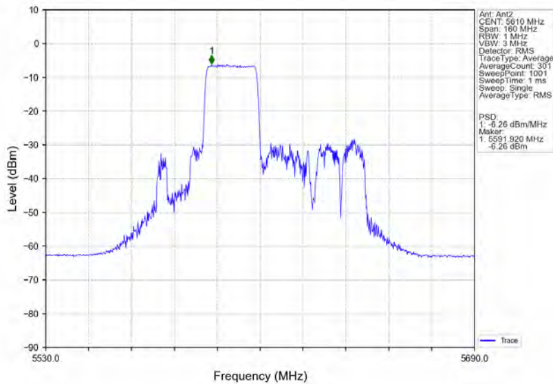
802.11ax(HE80) HCH 5610MHz RU242 Mid MIMO NTVN
