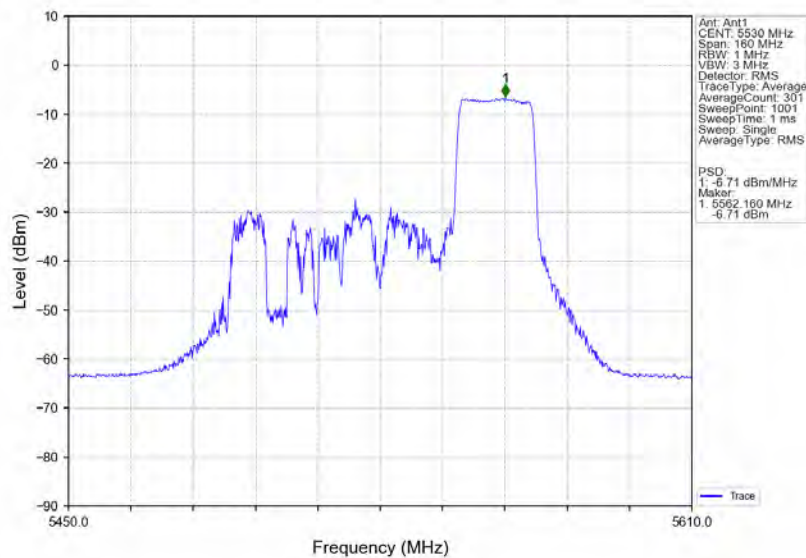
802.11ax(HE80) LCH 5530MHz RU242 Right Ant1 NTV
