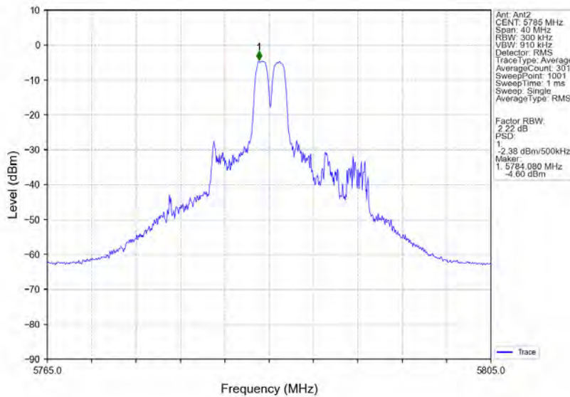
802.11ax(HE20) MCH 5785MHz RU26 Right MIMO NTVN
