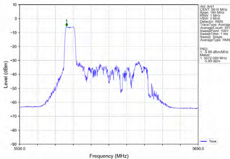
802.11ax(HE80) HCH 5610MHz RU106 Left Ant1 NTN
