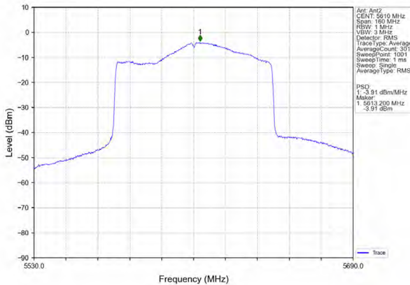
802.11ax(HE80) HCH 5610MHz RU996 Left MIMO NTVN
