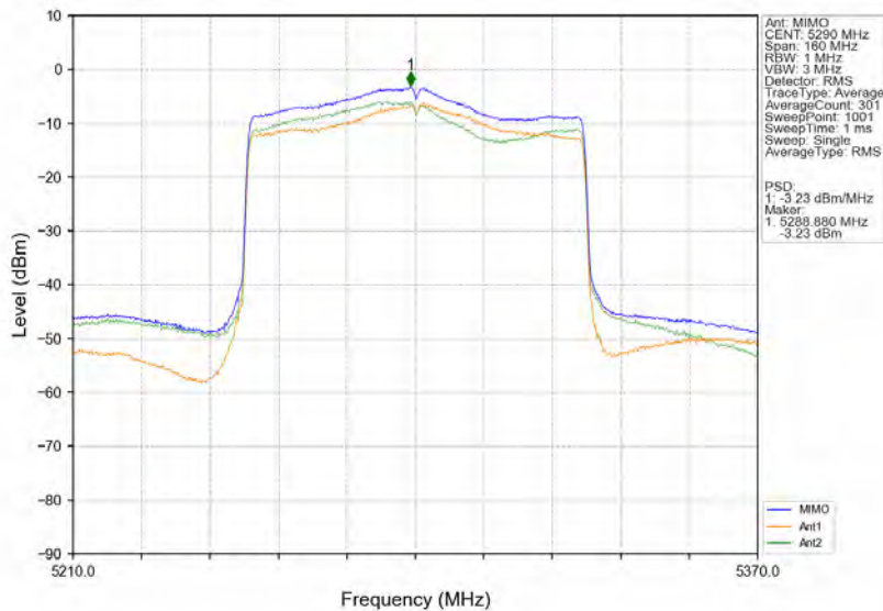
802.11ax(HE80)_MCH_5290MHz_RU996_Left_MIMO_NTNV
