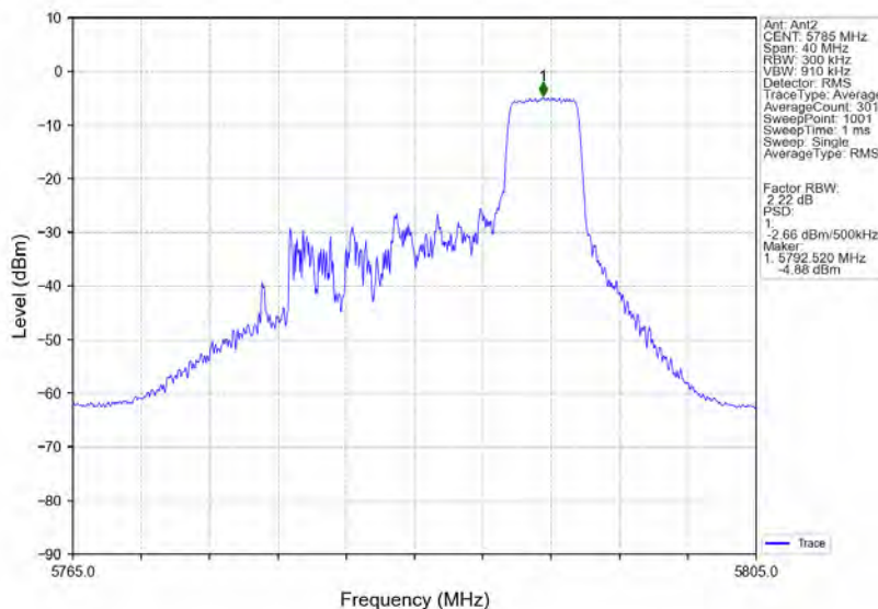
802.11ax(HE20) MCH 5785MHz RU52 Right Ant2 NTNv
