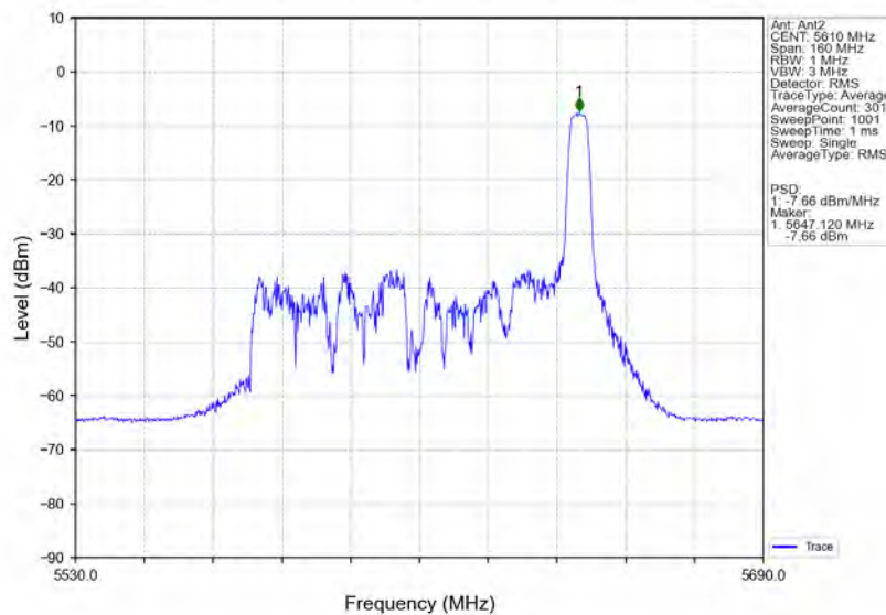
802.11ax(HE80) HCH 5610MHz RU52 Right Ant2 NTN
