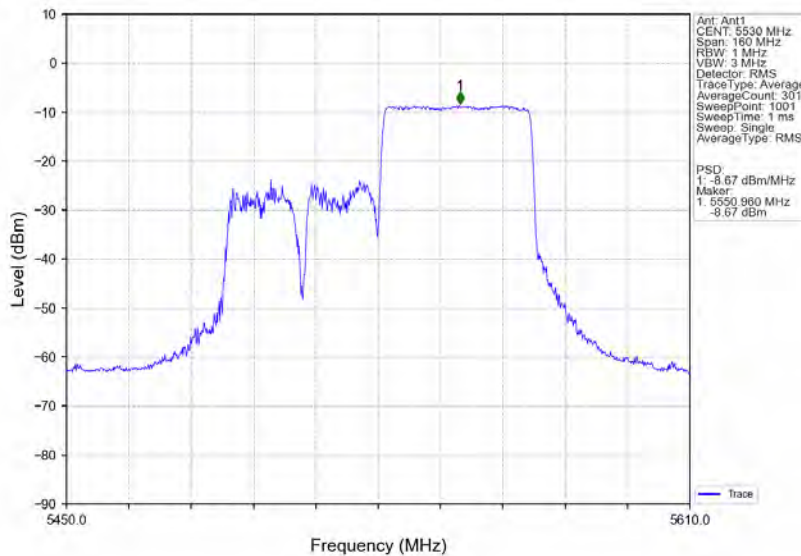
802.11ax(HE80) LCH 5530MHz RU484 Right Ant1 NTV
