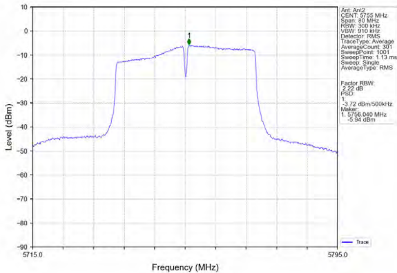
802.11ac(VHT40) LCH 5755MHz MIMO NTVN
