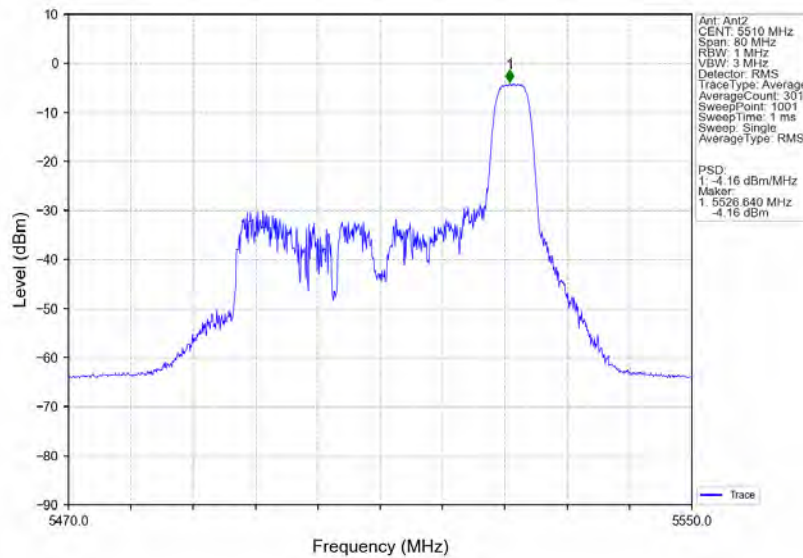
802.11ax(HE40) LCH 5510MHz RU52 Right MIMO NTVN
