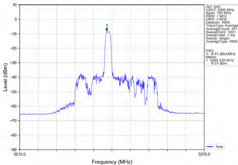
802.11ax(HE80) MCH 5290MHz RU52 Mid Ant1 NTN
