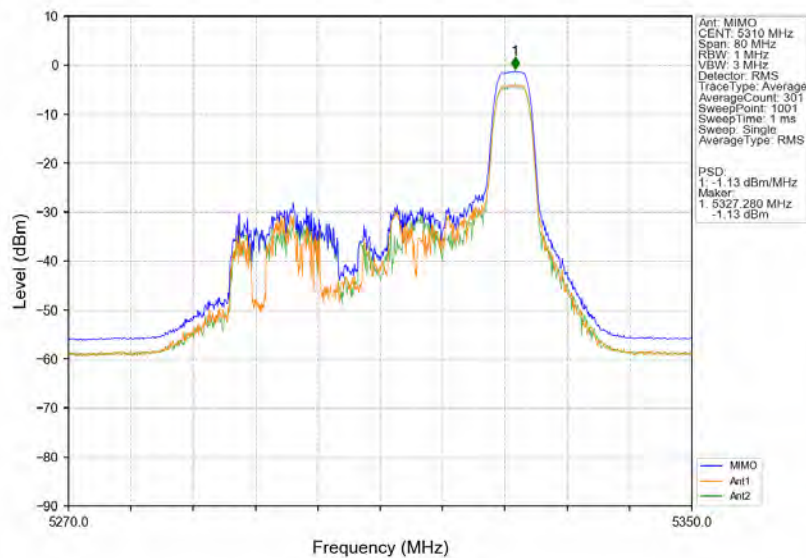
802.11ax(HE40) HCH 5310MHz RU52 Right MIMO NTN
