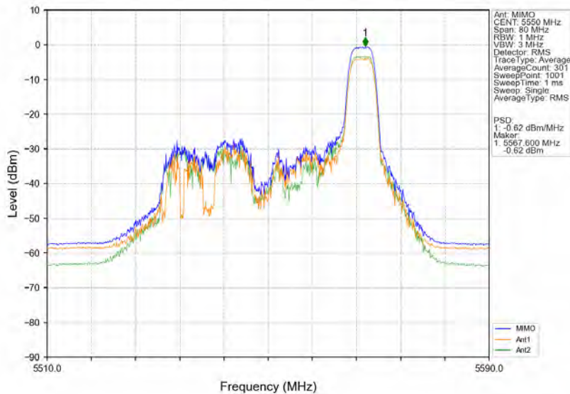
802.11ax(HE40) MCH 5550MHz RU52 Right MIMO NTVN
