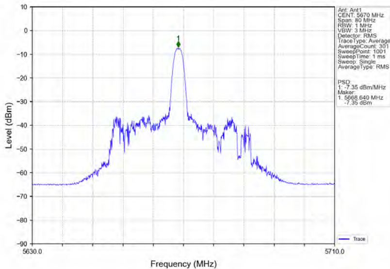
802.11ax(HE40) HCH 5670MHz RU26 Mid_Ant1 NTN
