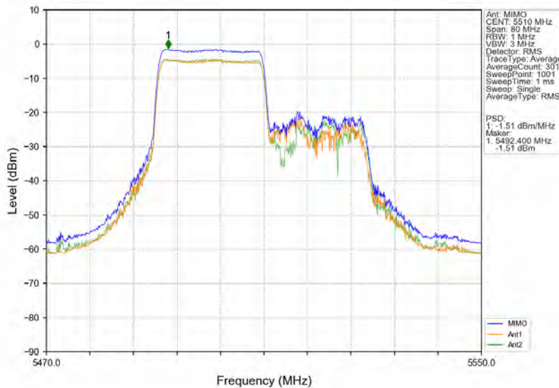
802.11ax(HE40) LCH 5510MHz RU242 Left MIMO NTVN
