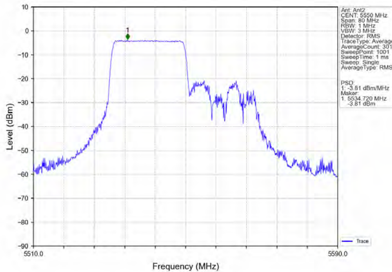
802.11ax(HE40) MCH 5550MHz RU242 Left MIMO NTNv
