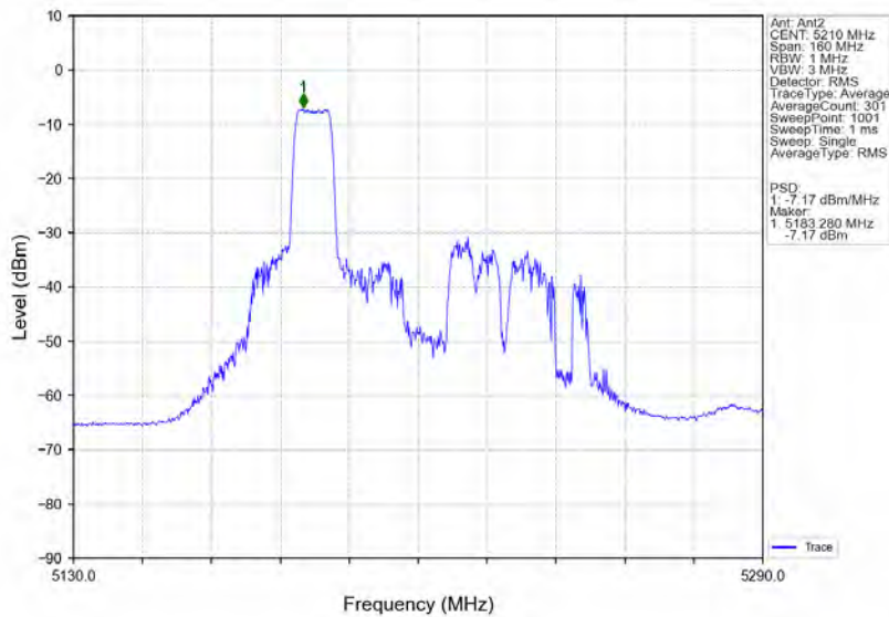
802.11ax(HE80) MCH 5210MHz RU106 Mid MIMO NTVN
