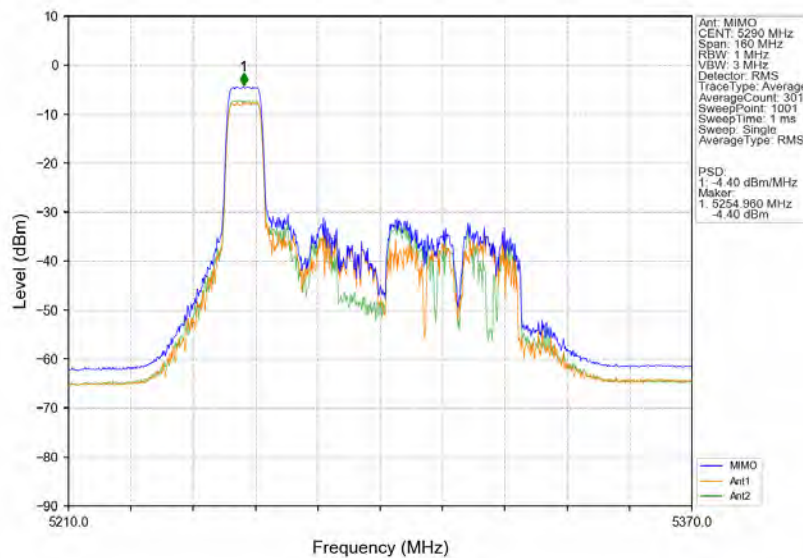
802.11ax(HE80) MCH 5290MHz RU106 Left MIMO NTVN
