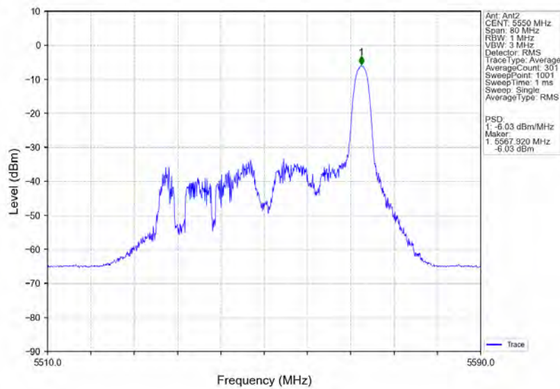
802.11ax(HE40) MCH 5550MHz RU26 Right Ant2 NTNv
