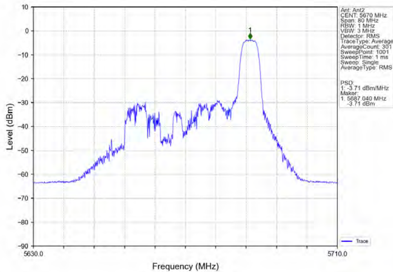
802.11ax(HE40) HCH 5670MHz RU52 Right MIMO NTVN
