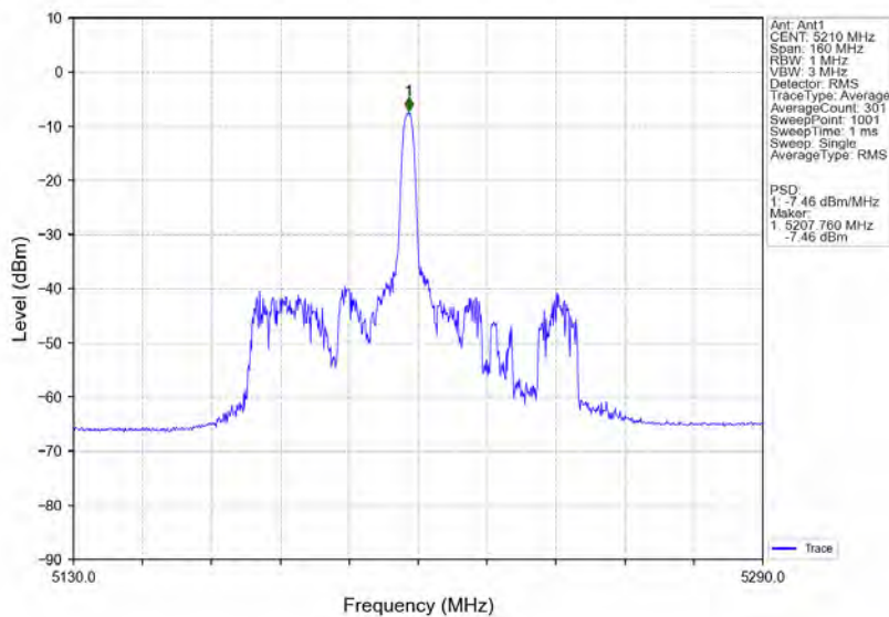
802.11ax(HE80) MCH 5210MHz RU26 Mid Ant1 NTN
