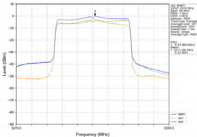
802.11ax(HE40) HCH 5310MHz RU484 Left MIMO NTVN
