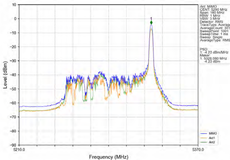
802.11ax(HE80) MCH 5290MHz RU26 Right MIMO NTVN
