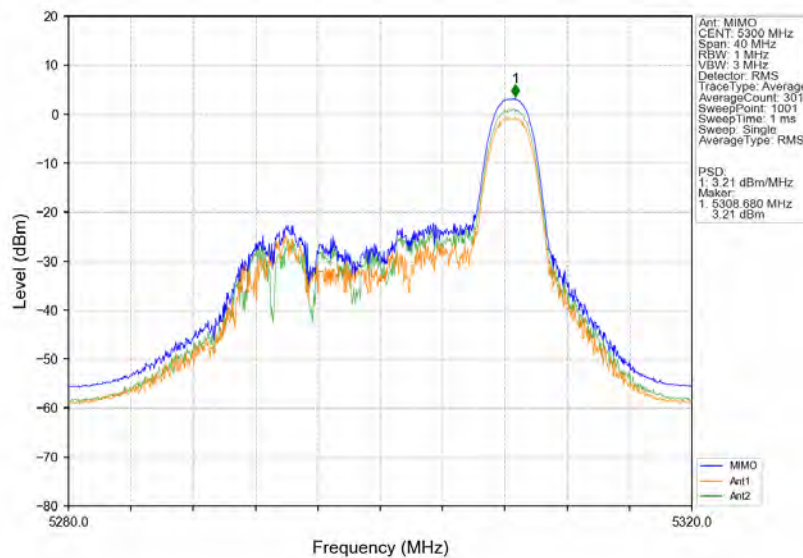
802.11ax(HE20) MCH 5300MHz RU26 Right MIMO NTVN
