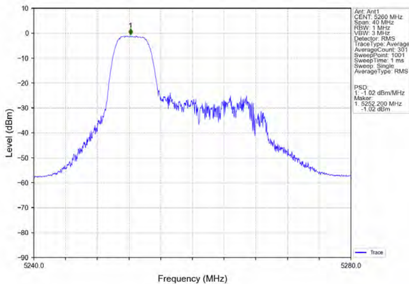
802.11ax(HE20) LCH 5260MHz RU52 Left Ant1 NTN
