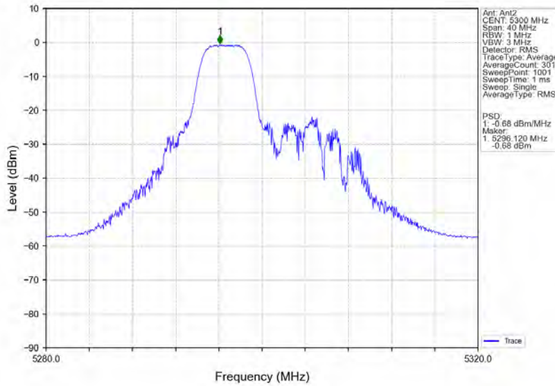
802.11ax(HE20) MCH 5300MHz RU52 Mid MIMO NTN
