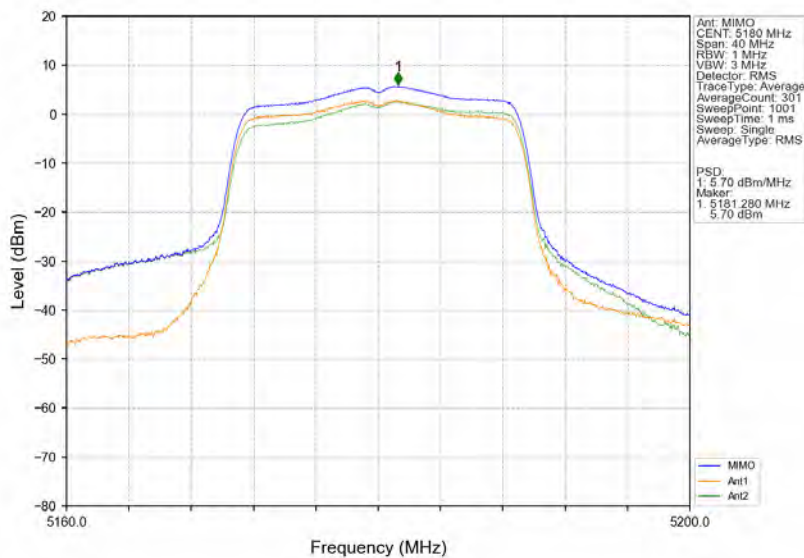
802.11ac(VHT20) LCH 5180MHz MIMO NTV
