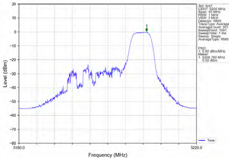
802.11ax(HE20) MCH 5200MHz RU52 Right Ant1 NTN
