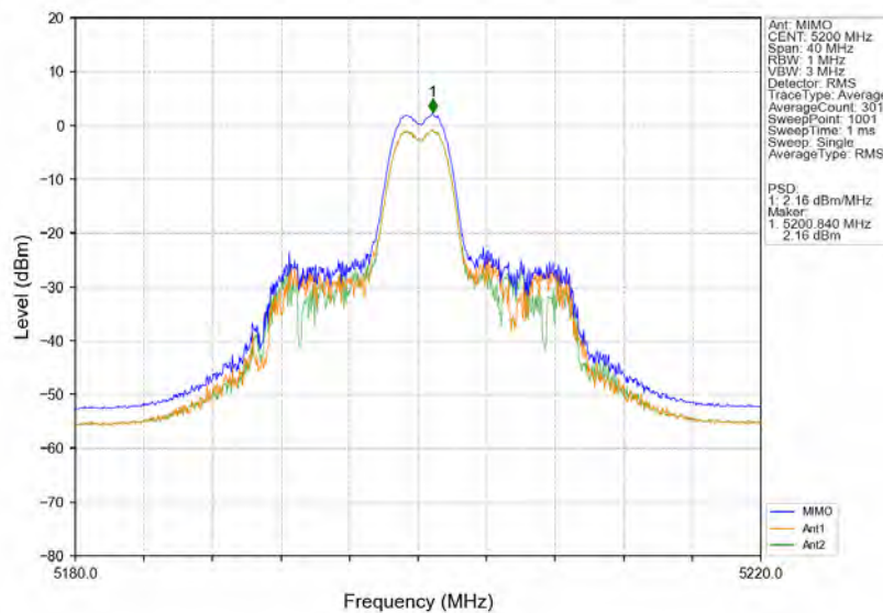
802.11ax(HE20) MCH 5200MHz RU26 Mid MIMO NTN
