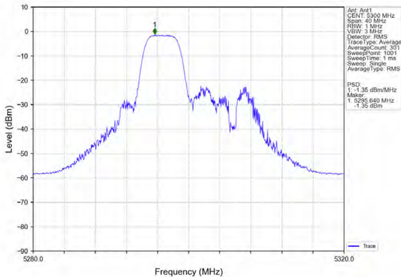
802.11ax(HE20) MCH 5300MHz RU52 Mid Ant1 NTN
