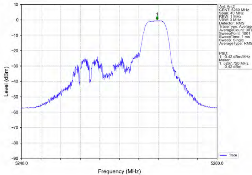
802.11ax(HE20) LCH 5260MHz RU52 Right MIMO NTN
