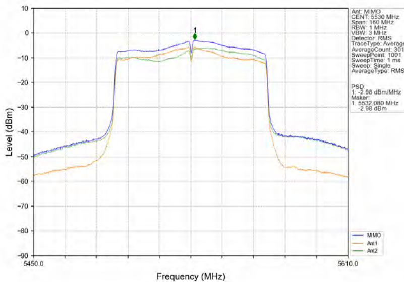
802.11ac(VHT80) LCH 5530MHz MIMO NTV
