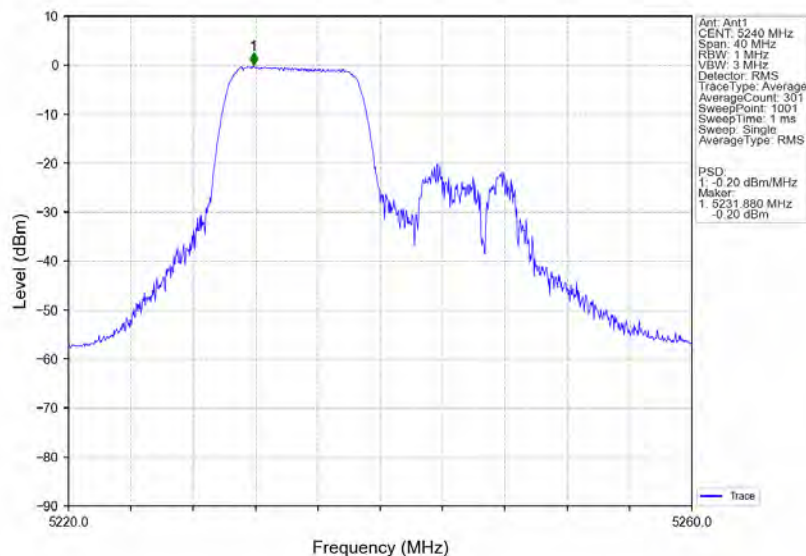
802.11ax(HE20) HCH 5240MHz RU106 Left Ant1 NTN
