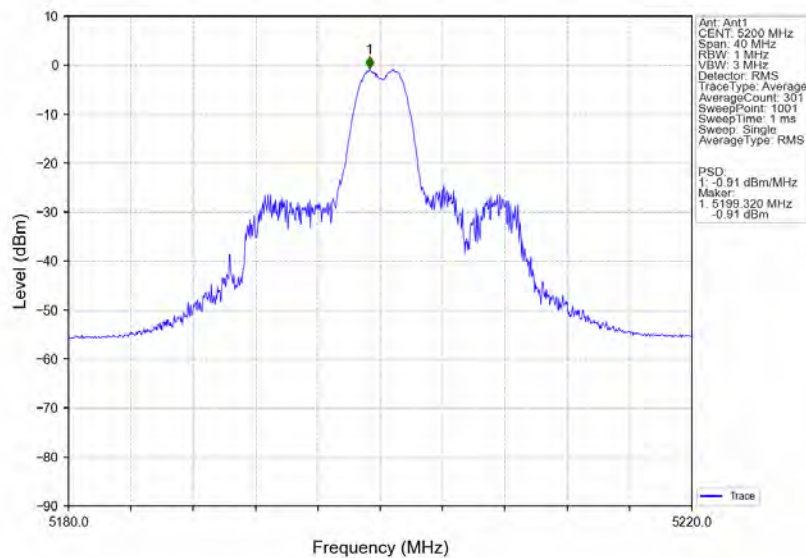
802.11ax(HE20) MCH 5200MHz RU26 Mid Ant1 NTN
