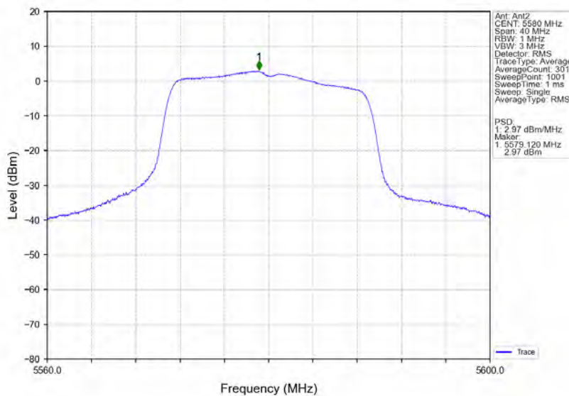
802.11n(HT20) MCH 5580MHz Ant2 NTVN
