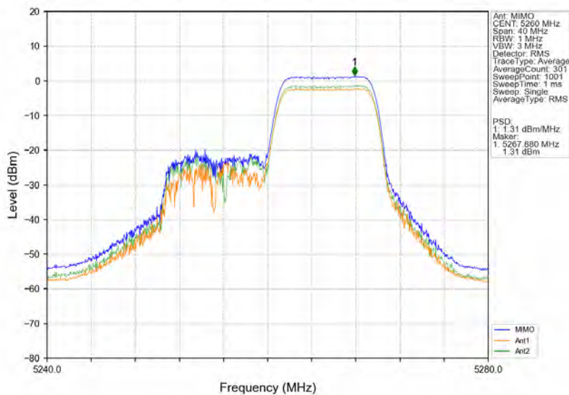
802.11ax(HE20) LCH 5260MHz RU106 Right MIMO NTVN
