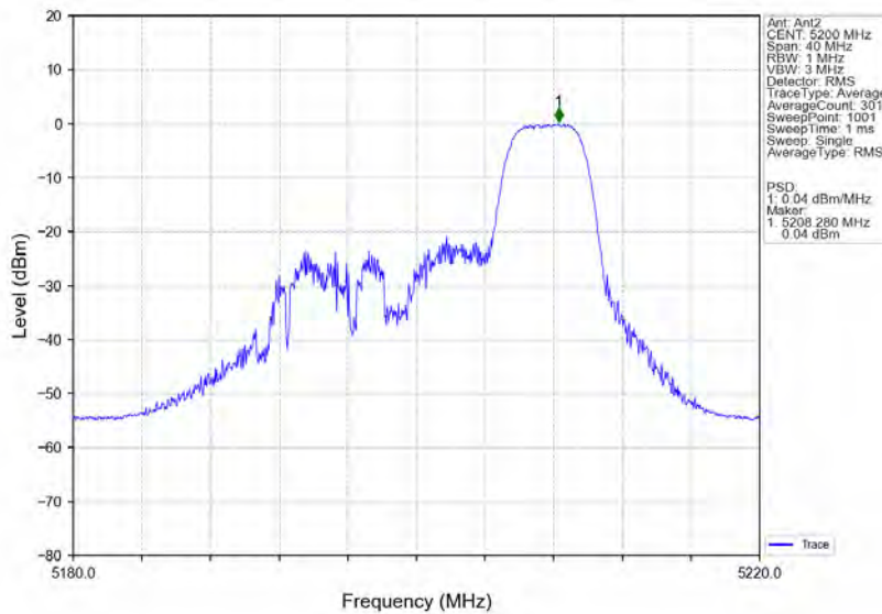
802.11ax(HE20) MCH 5200MHz RU52 Right MIMO NTVN
