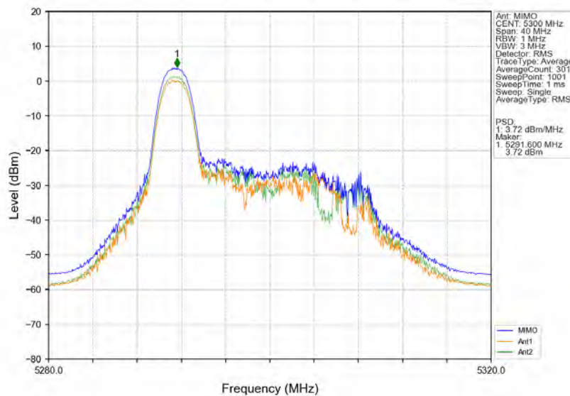
802.11ax(HE20) MCH 5300MHz RU26 Left MIMO NTN
