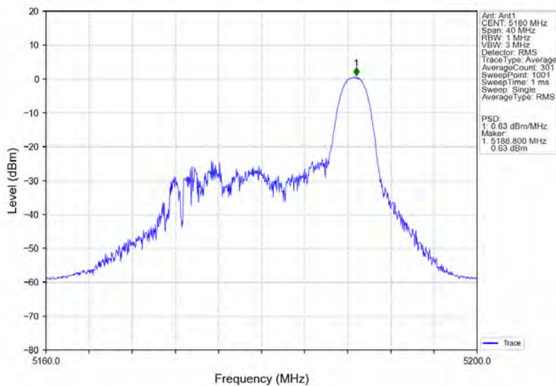
802.11ax(HE20) LCH 5180MHz RU26 Right Ant1 NTN
