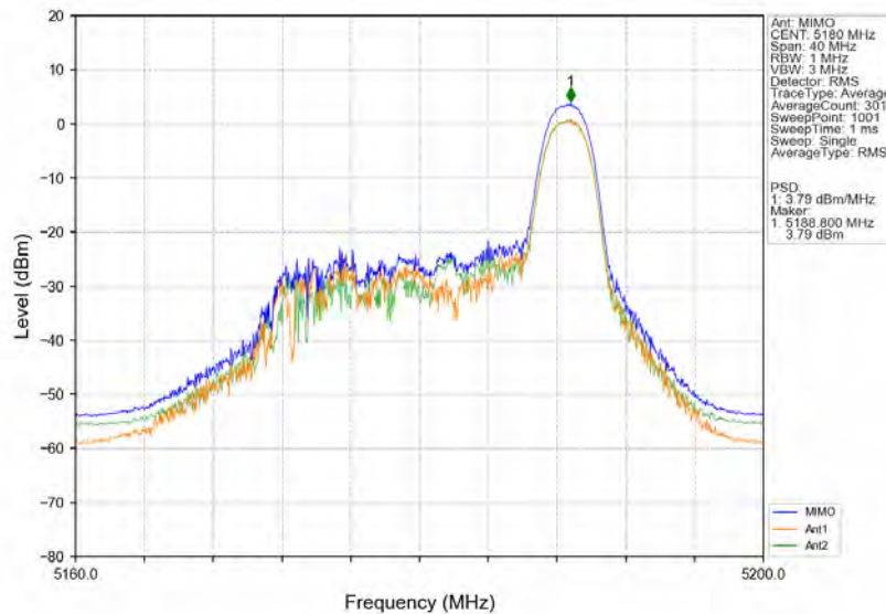
802.11ax(HE20) LCH 5180MHz RU26 Right MIMO NTN
