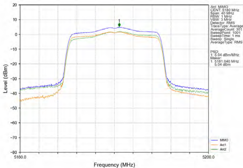
802.11ax(HE20) LCH 5180MHz RU242 Left MIMO NTN
