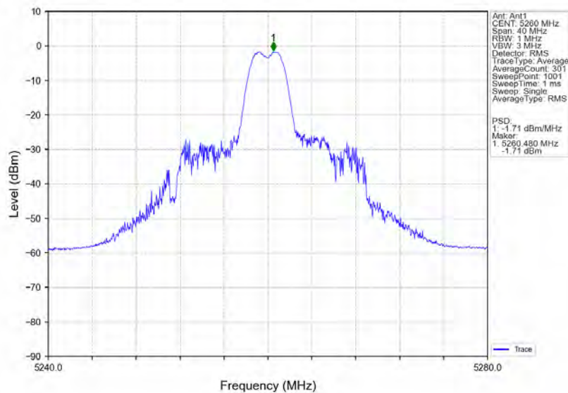
802.11ax(HE20) LCH 5260MHz RU26 Mid Ant1 NTN
