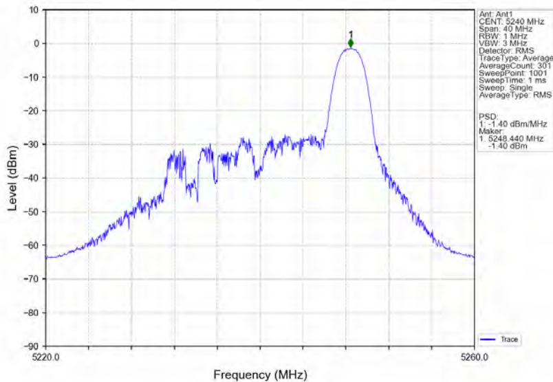
802.11ax(HE20) HCH 5240MHz RU26 Right Ant1 NTN
