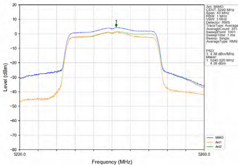
802.11ax(HE20) HCH 5240MHz RU242 Left MIMO NTN
