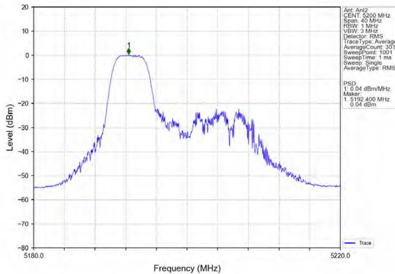
802.11ax(HE20) MCH 5200MHz RU52 Left MIMO NTN
