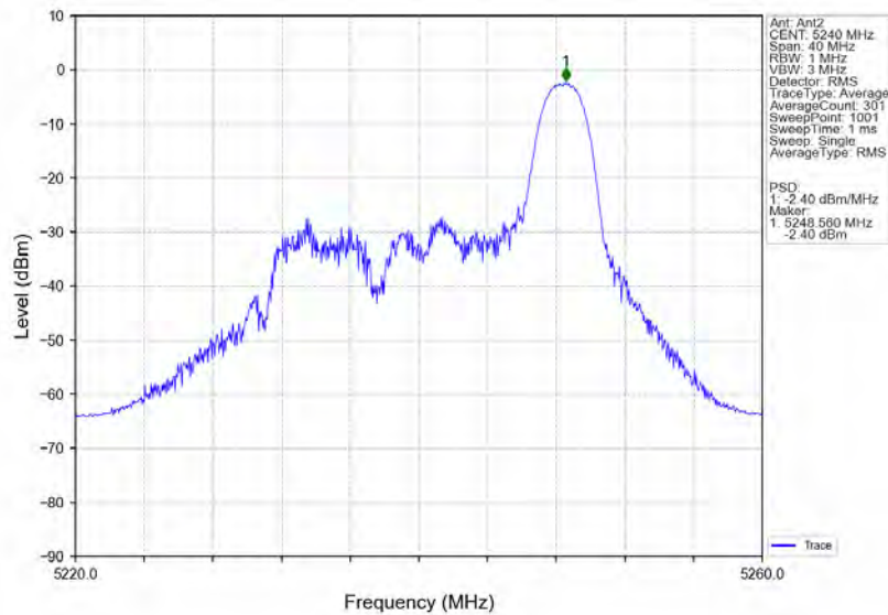
802.11ax(HE20) HCH 5240MHz RU26 Right MIMO NTVN
