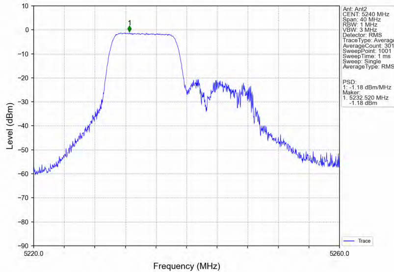
802.11ax(HE20) HCH 5240MHz RU106 Left MIMO NTN
