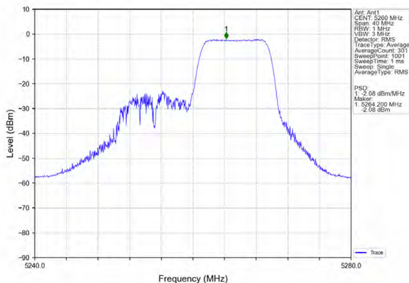
802.11ax(HE20) LCH 5260MHz RU106 Right Ant1 NTV
