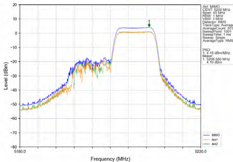
802.11ax(HE20) MCH 5200MHz RU106 Right MIMO NTN
