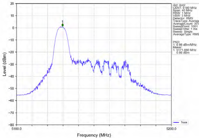
802.11ax(HE20) LCH 5180MHz RU26 Left MIMO NTN
