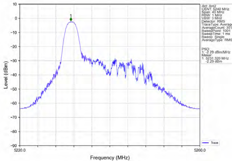
802.11ax(HE20) HCH 5240MHz RU26 Left MIMO NTN
