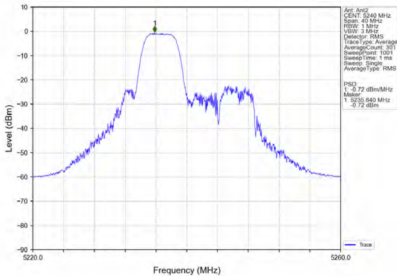
802.11ax(HE20) HCH 5240MHz RU52 Mid MIMO NTN
