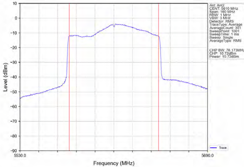
802.11ax(HE80) HCH 5610MHz RU996 Left Ant2 NTN
