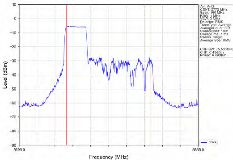
802.11ax(HE80) MCH 5775MHz RU242 Left Ant2 NTN
