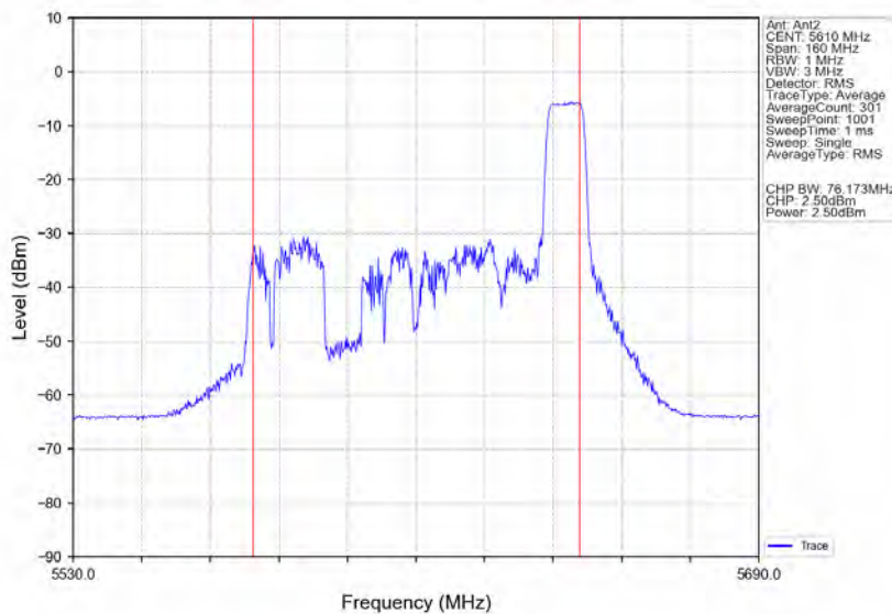
802.11ax(HE80) HCH 5610MHz RU106 Right Ant2 NTV
