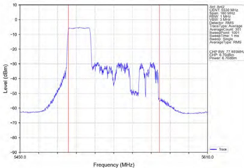
802.11ax(HE80) LCH 5530MHz RU242 Left Ant2 NTN
