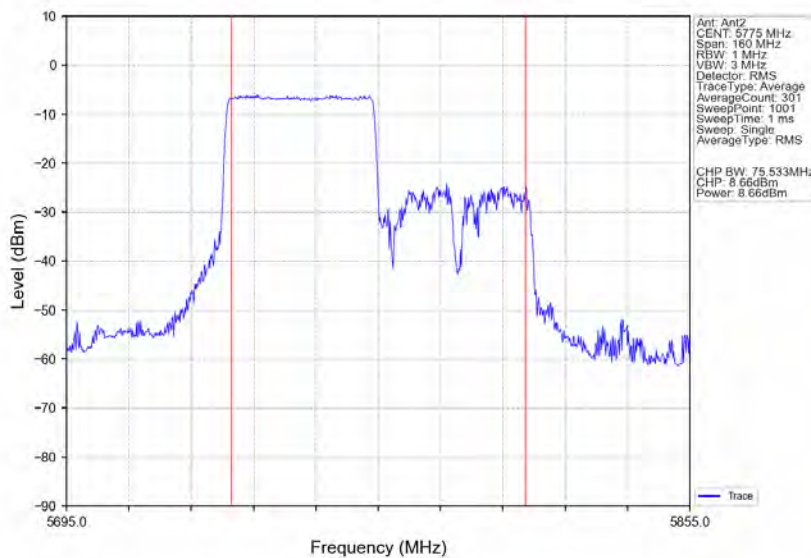
802.11ax(HE80) MCH 5775MHz RU484 Left Ant2 NTN
