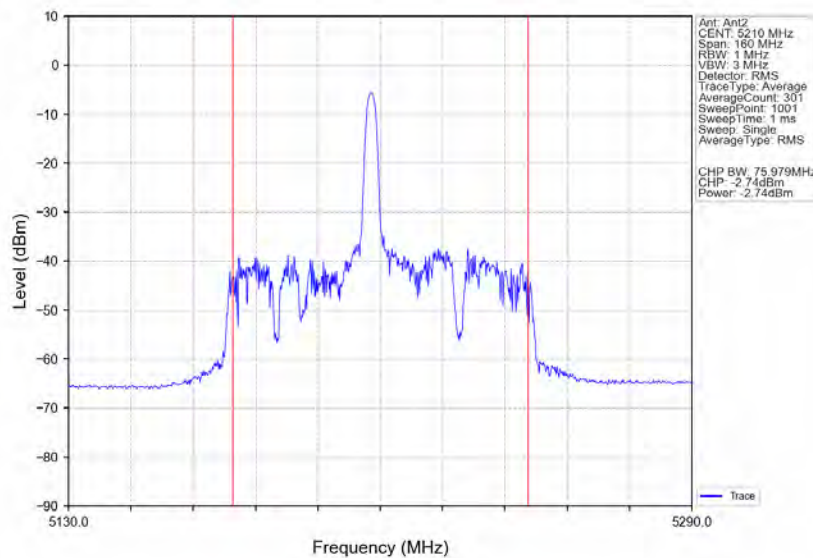
802.11ax(HE80) MCH 5210MHz RU26 Mid Ant2 NTN
