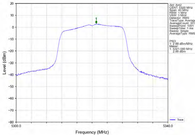
802.11a HCH 5320MHz MIMO NTN
