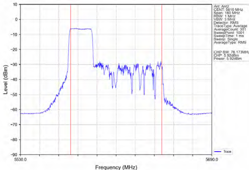
802.11ax(HE80) HCH 5610MHz RU242 Left Ant2 NTNv
