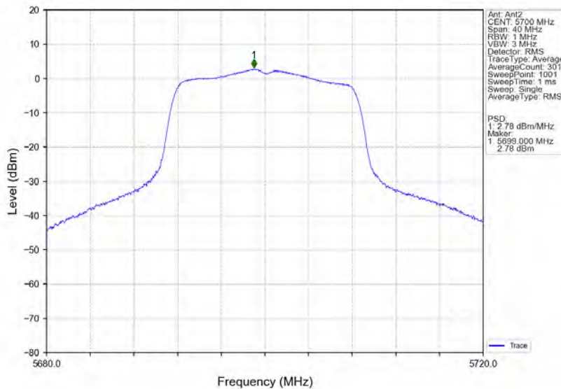
802.11a_HCH_5700MHz_Ant2_NTNV
