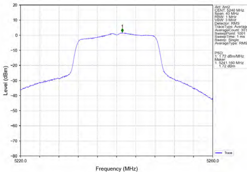
802.11a_HCH_5240MHz_Ant2_NTNV
