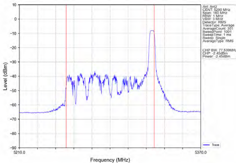
802.11ax(HE80) MCH 5290MHz RU52 Right Ant2 NTNv
