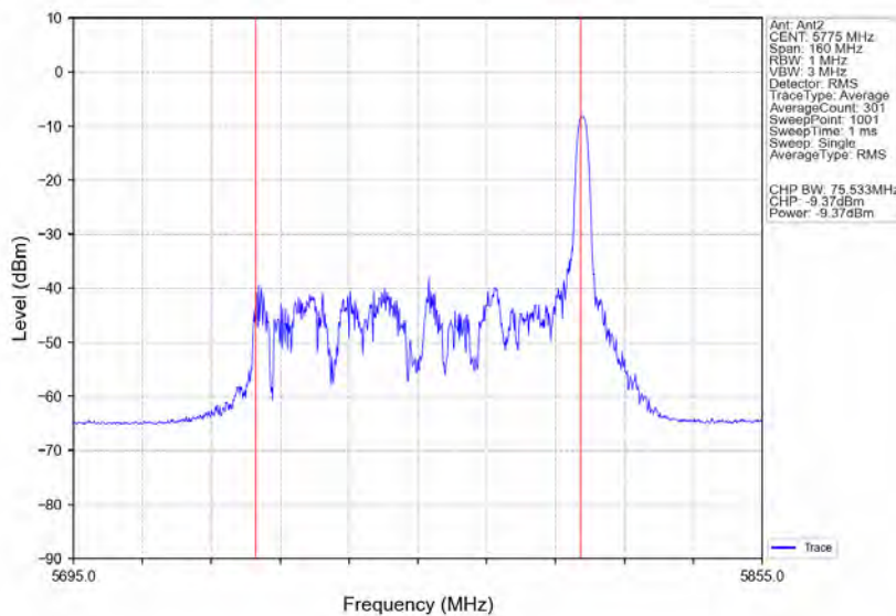
802.11ax(HE80) MCH 5775MHz RU26 Right Ant2 NTNv
