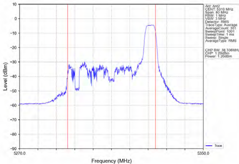
802.11ax(HE40) HCH 5310MHz RU52 Right Ant2 NTN
