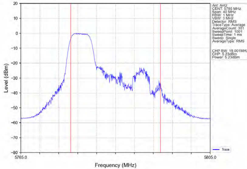
802.11ax(HE20) MCH_5785MHz RU52 Left Ant2 NTN
