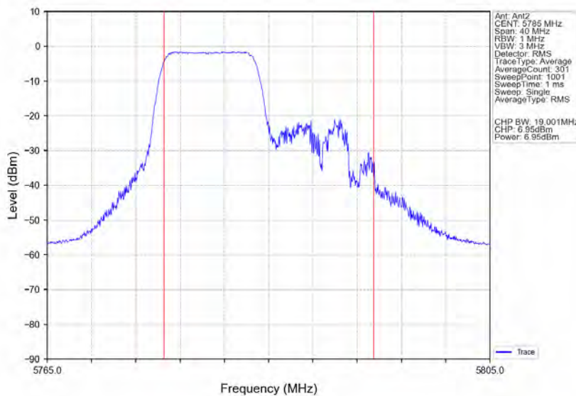
802.11ax(HE20) MCH 5785MHz RU106 Left Ant2 NTN
