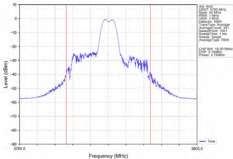
802.11ax(HE20) MCH 5785MHz RU26 Right Ant2 NTN
