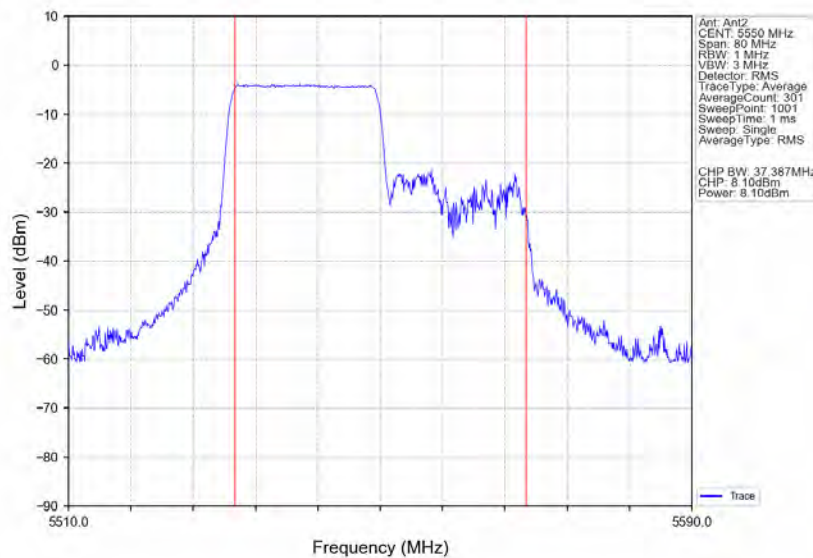
802.11ax(HE40) MCH 5550MHz RU242 Left Ant2 NTN
