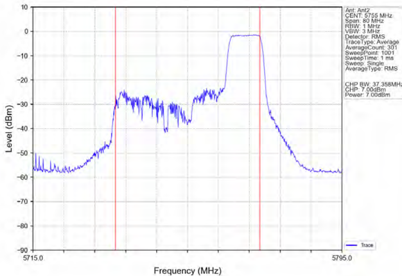
802.11ax(HE40) LCH 5755MHz RU106 Right Ant2 NTV
