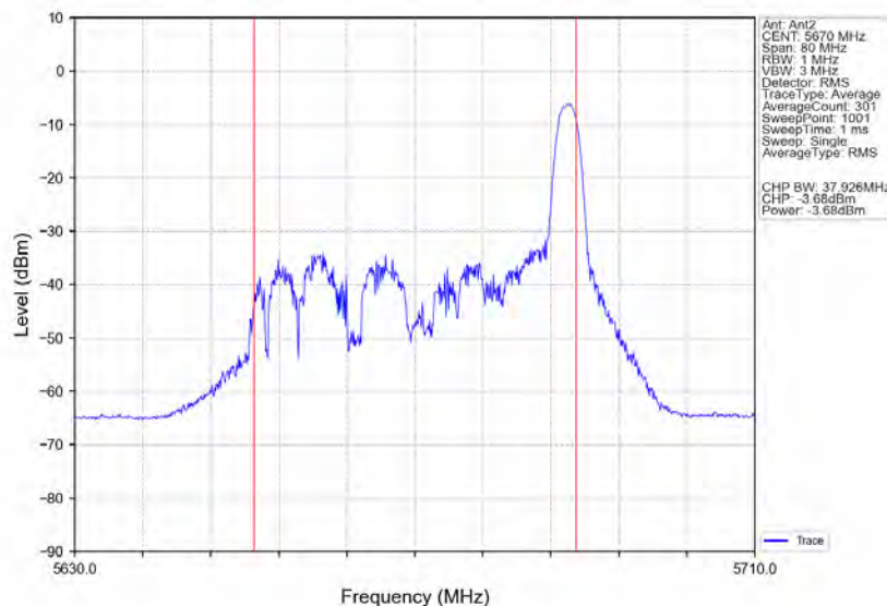
802.11ax(HE40) HCH 5670MHz RU26 Right Ant2 NTN
