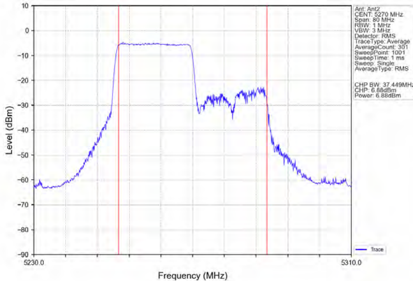
802.11ax(HE40) LCH 5270MHz RU242 Left Ant2 NTN
