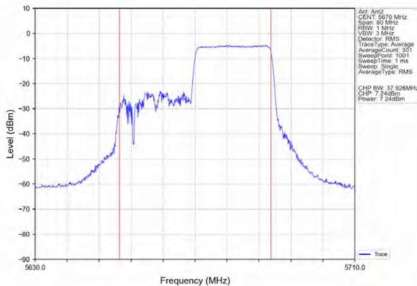
802.11ax(HE40) HCH 5670MHz RU242 Right Ant2 NTV
