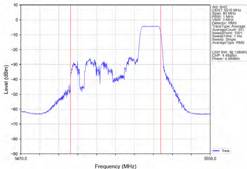
802.11ax(HE40) LCH 5510MHz RU106 Right Ant2 NTV
