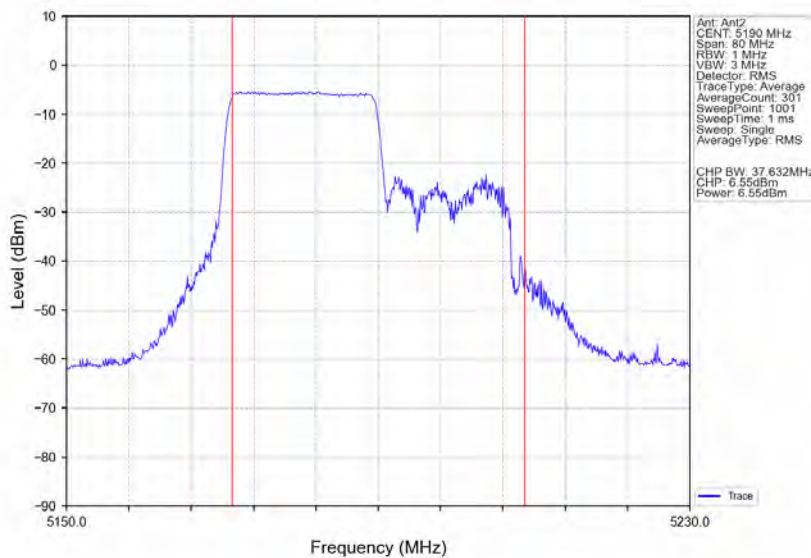
802.11ax(HE40) LCH 5190MHz RU242 Left Ant2 NTN
