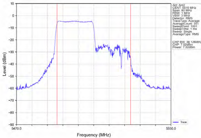
802.11ax(HE40) LCH 5510MHz RU242 Left Ant2 NTN
