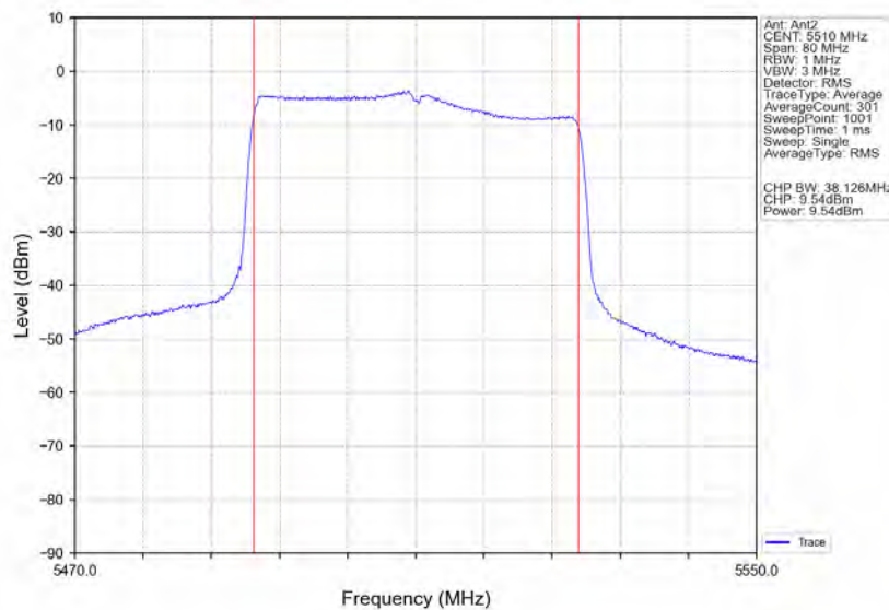
802.11ax(HE40) LCH 5510MHz RU484 Left Ant2 NTN
