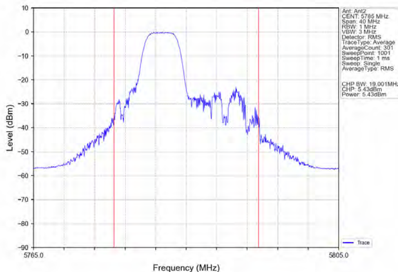
802.11ax(HE20) MCH_5785MHz RU52 Mid Ant2 NTN
