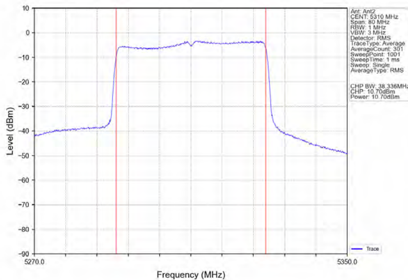
802.11ax(HE40) HCH 5310MHz RU484 Left Ant2 NTNv
