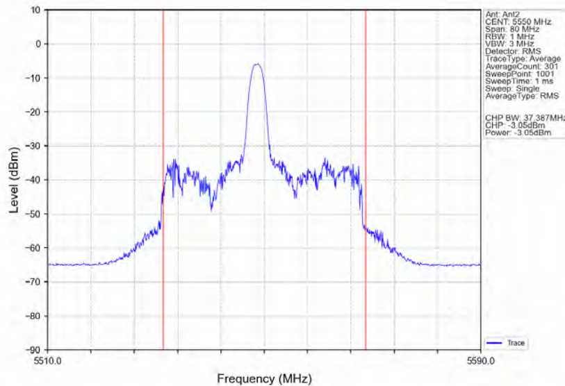
802.11ax(HE40) MCH 5550MHz RU26 Mid Ant2 NTN
