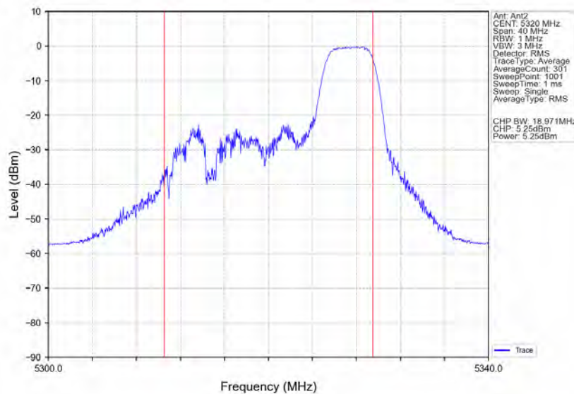
802.11ax(HE20) HCH 5320MHz RU52 Right Ant2 NTN
