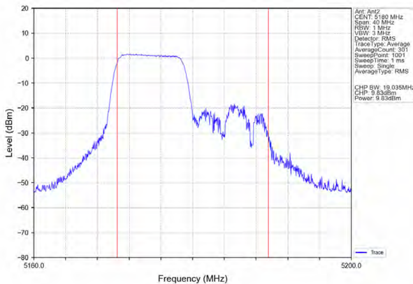
802.11ax(HE20) LCH 5180MHz RU106 Left Ant2 NTN
