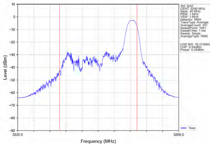
802.11ax(HE20) HCH 5240MHz RU26 Right Ant2 NTN
