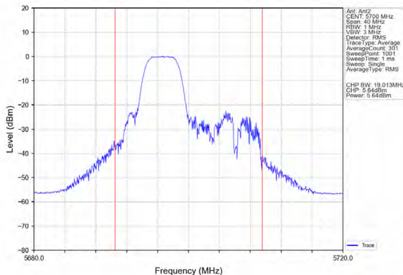
802.11ax(HE20) HCH 5700MHz RU52 Mid Ant2 NTN
