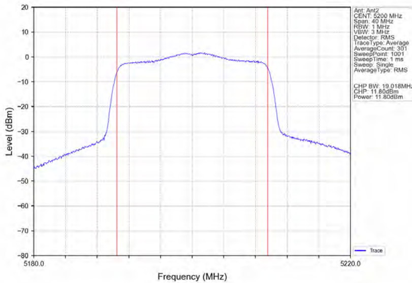
802.11ax(HE20) MCH 5200MHz RU242 Left Ant2 NTN
