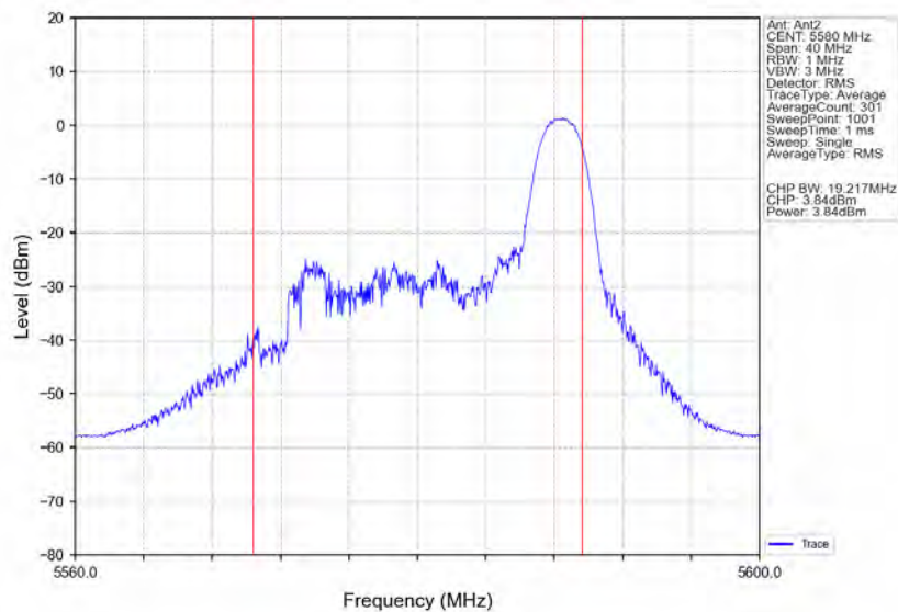
802.11ax(HE20) MCH 5580MHz RU26 Right Ant2 NTN
