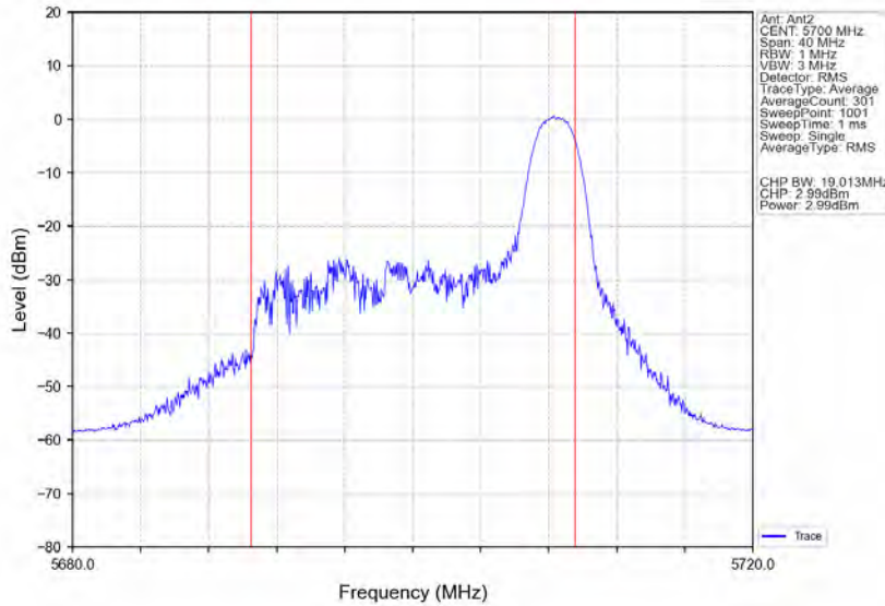
802.11ax(HE20) HCH 5700MHz RU26 Right Ant2 NTN
