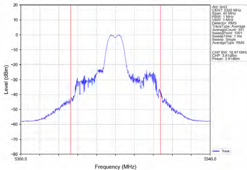
802.11ax(HE20) HCH 5320MHz RU26 Mid Ant2 NTN
