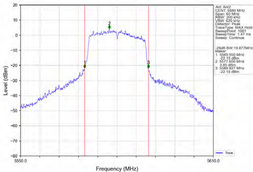
802.11n(HT20) MCH 5580MHz Ant2 NTVN
