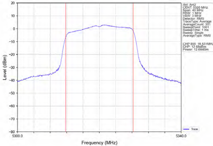
802.11a_HCH_5320MHz_Ant2_NTNV
