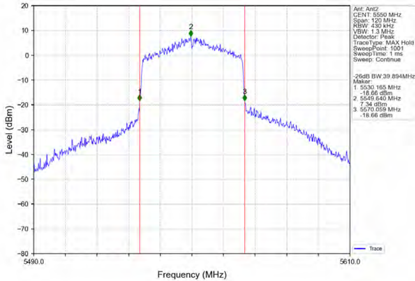
802.11ax(HE40) MCH 5550MHz RU484 Left Ant2 NTNv
