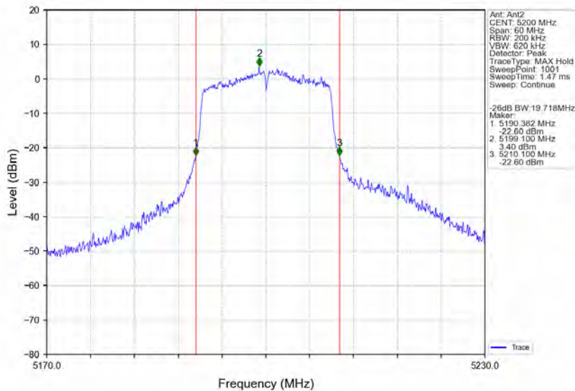
802.11n(HT20) MCH 5200MHz Ant2 NTVN
