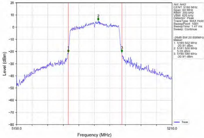
802.11ax(HE20) LCH 5180MHz RU242 Left Ant2 NTNv
