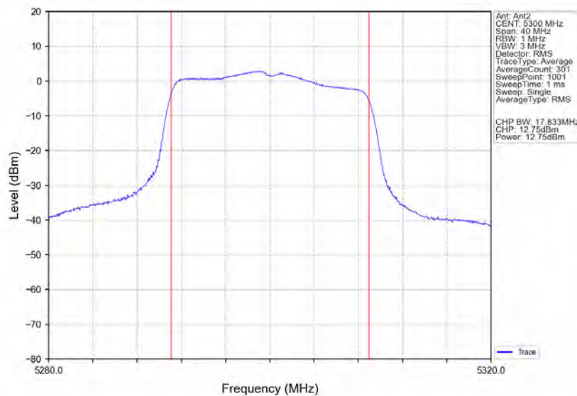
802.11n(HT20) MCH 5300MHz Ant2 NTVN
