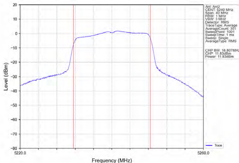
802.11a_HCH_5240MHz_Ant2_NTNV
