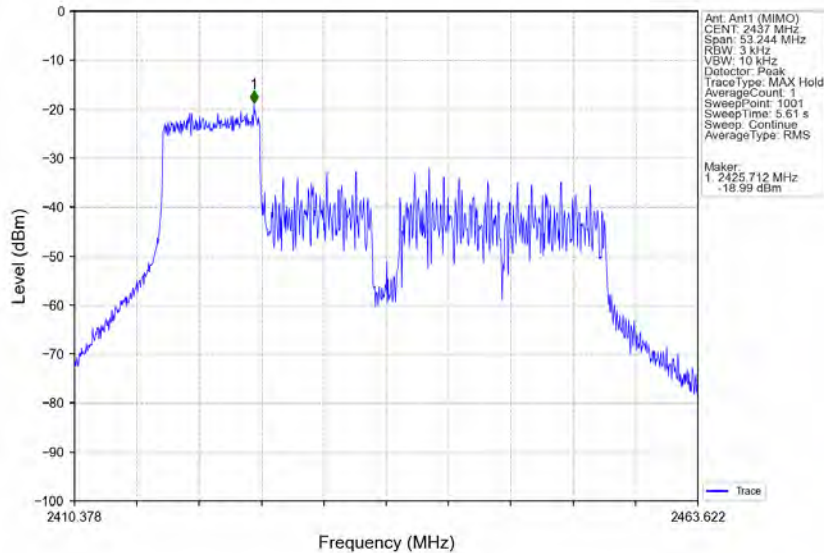
802.11ax(HE40) MCH 2437MHz RU106 Left Ant1 (MIMO) NTN
