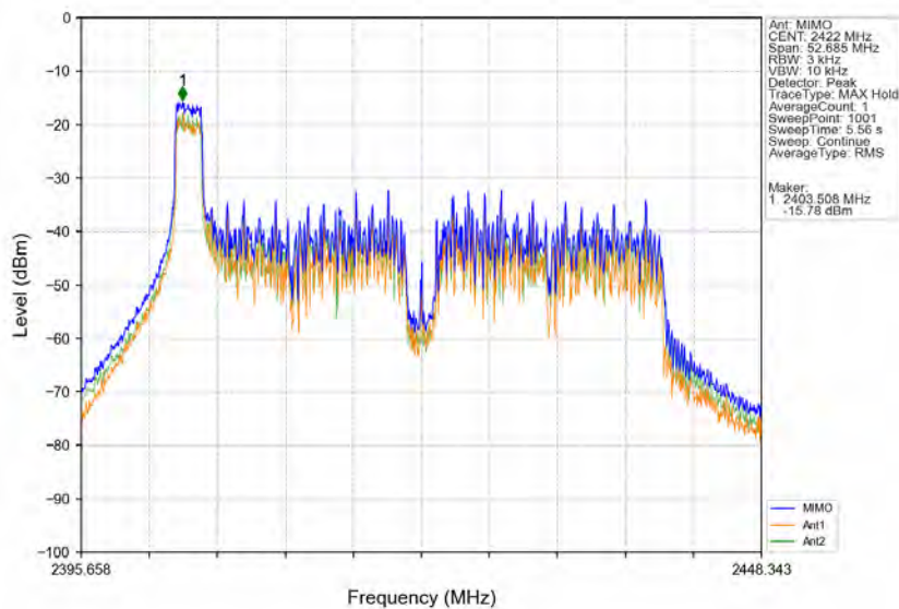
802.11ax(HE40) LCH 2422MHz RU26 Left MIMO NTN
