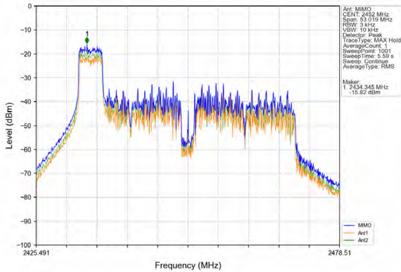
802.11ax(HE40) HCH 2452MHz RU52 Mid Ant1 (MIMO) NTN
