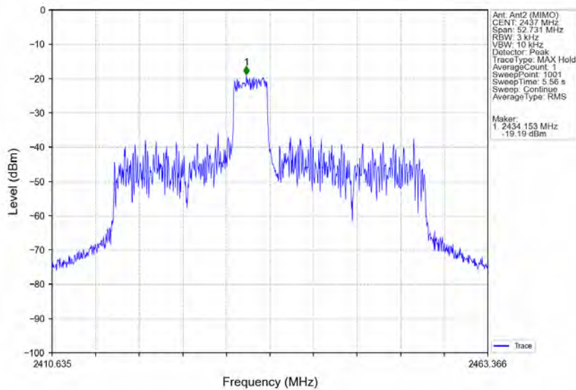
802.11ax(HE40) MCH 2437MHz RU52 Mid MIMO NTVN
