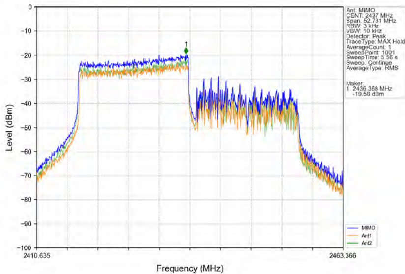
802.11ax(HE40) MCH_2437MHz_RU242_Right_Ant1(MIMO)_NTNV
