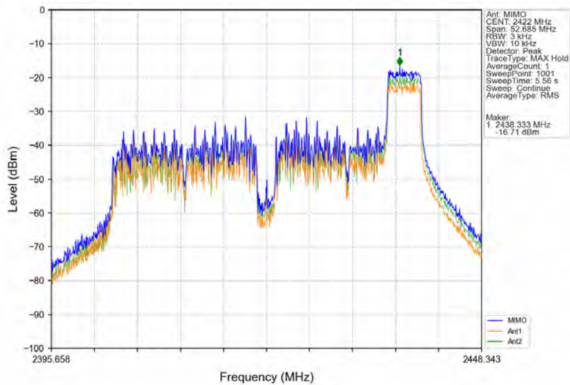
802.11ax(HE40) LCH 2422MHz RU106 Left Ant1 (MIMO) NTV
