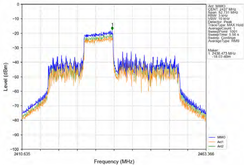
802.11ax(HE40) MCH_2437MHz_RU106_Right_Ant1(MIMO)_NTNV
