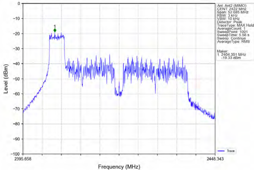
802.11ax(HE40) LCH 2422MHz RU52 Left Ant2 (MIMO) NTVN
