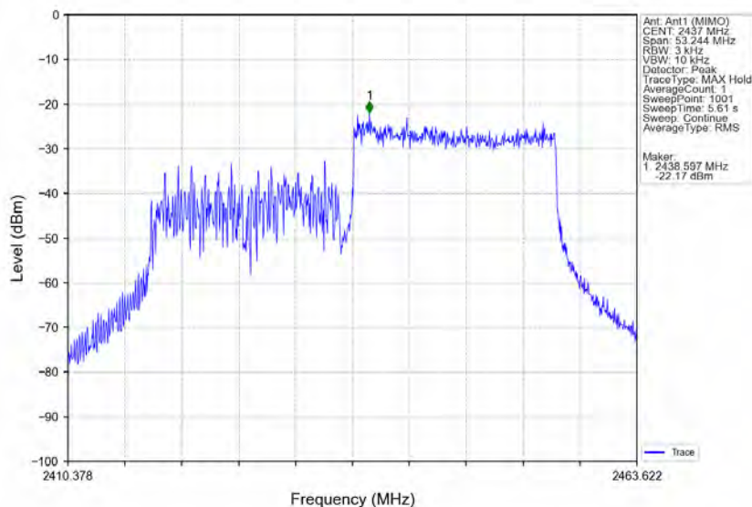
802.11ax(HE40) MCH_2437MHz_RU242_Right_Ant1(MIMO)_NTNV
